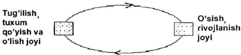
19-rasm. Bir marta borib kelish sxemasi
