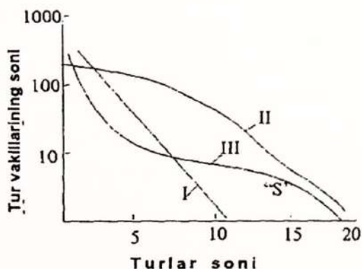
22-rasm. Turning har xilligini ko'rsatuvchi sxema (20 turga 1000 ta tur vakili; original)
