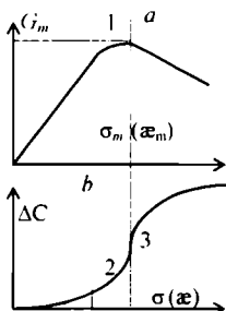
24.14-chizma. O'tkazuvchanlik aktiv qismining (a) va bo'g'in sig'imining (b) elektr o'tkazuvchanlikka bog'liqligi. 1-past o'tkazuvchanlik sohasi; 2-sinish nuqtasi; 3-o'rta nuqta
