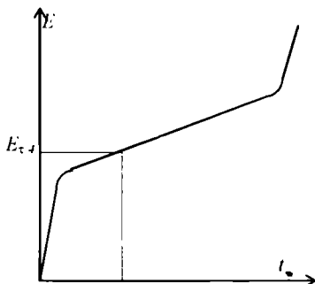
23.15-chizma. Xronopotensioqramma
