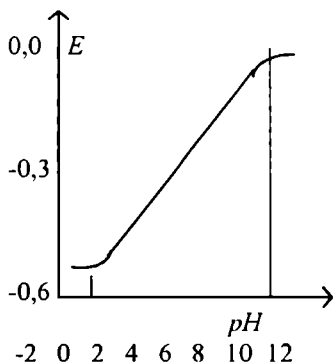
21.2-chizma. Shisha elektrod potentsialining pH ga bog'liqligi
