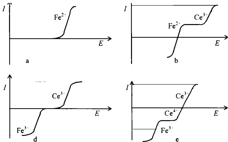
20.9-chizma. Kimyoviy reaksiyalarning natijasida voltamper egri chiziqlarining o'zgarishi
