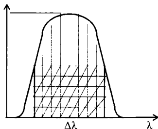
25.5-chizma. Spektr chizig'i va uning yarim kengligi
