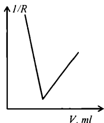
24.4-chizma. Kuchli kislotani ishqor eritmasi bilan titrlash egri chizig'i
