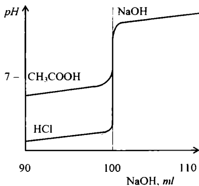
15.5-chizma. Kuchli (HCl) va kuchsiz ( CH_3COOH ) kislotalarni titrlash egri chiziqlari
