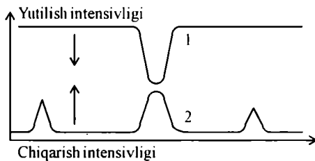
26.5-chizma. Atom-absorbtsion spektroskopiyada chiqarish va yutilish spektrlari:
