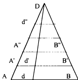
24.16-chizma. Uch tarkibiy qisimli sistemalarda moddalar tarkibi o'zgarishi qonuniyatlari
