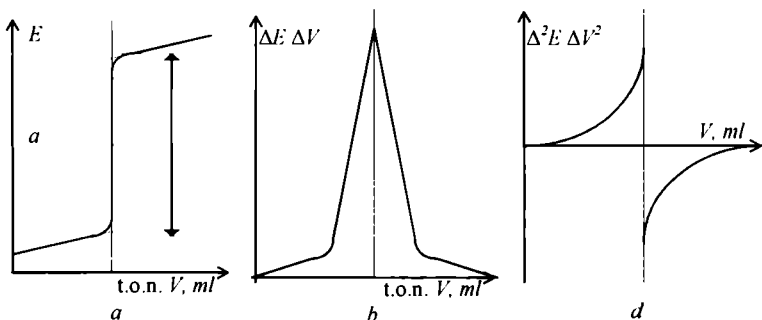
21.7-chizma. Potentsiometrik titrlash egri chiziqlarining ko'rinishi: a -integral; b -differensial; d -ikkinchi tartibli hosila
