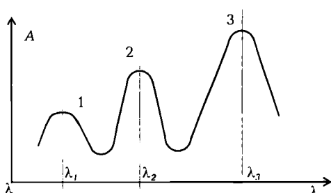
27.3-chizma. Bir necha yutilish yo'lakiga ega bo'lgan moddaning spektri
