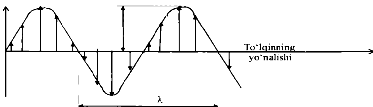
25.1-chizma. Monoxromatik nurlanish oqimining to‘lqin uzunligi ( \lambda ) va amplitudasi ( a )
