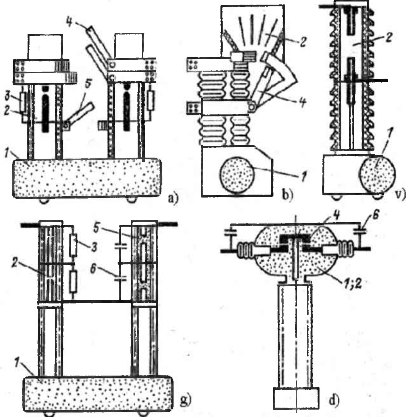
8.21-rasm Havoli uzgichlarining konstruktiv sxemalari: a, b – katta nominal tokka mo'ljallangan uzgich; d – 35 kVli ochiq qurilmalardagi uzgich; e – 110 kVli ochiq qurilmalardagi uzgich; 1 – siqilgan havoli rezervuar; 2 – yoy so'ndiruvchi kamera; 3 – shuntlovchi rezistor; 4 – bosh kontaktlar; 5 – ajratkich; 6 – sig'imli kuchlanish bo'lgichi.
