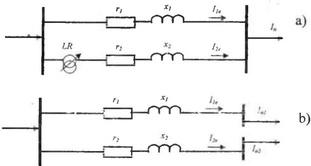
9.4-rasm. Tenglashtiruvchi kontur toklarini kompensatsiyalash: a – liniya rostagich transformatorining transformatsiyalash koeffitsiyentini rostlash orqali; b– konturni ochish orqali.
