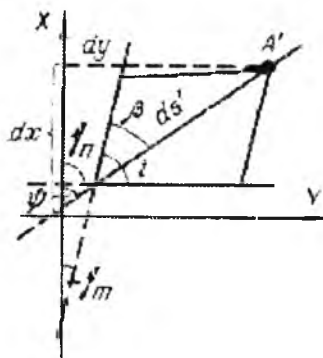
6-rasm. Proyeksiyada azimutni tasvirlash
