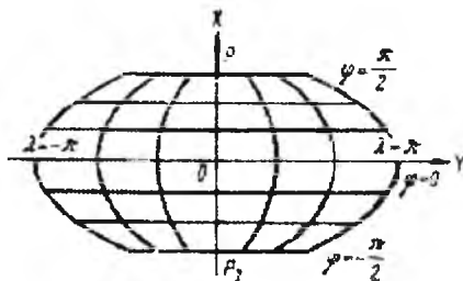
42-rasm. Psevdosilindrik proyeksiyalar koordinatalari tizimi
