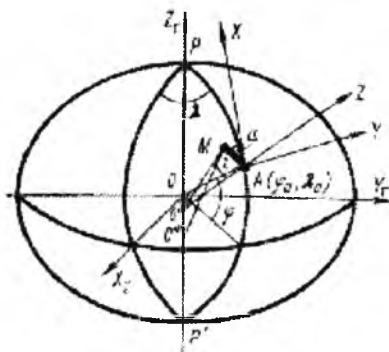
1-rasm. Geosentrik va toposentrik fazoviy koordinatalar tizimlari
