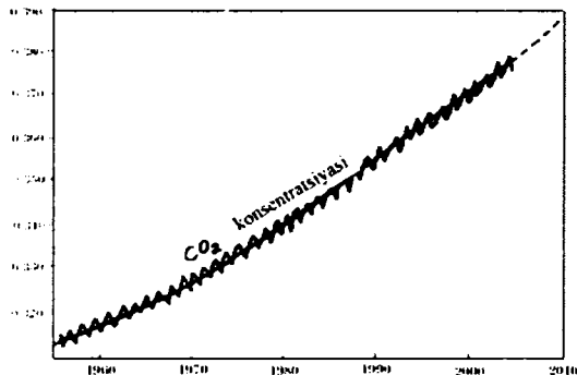
9-rasm. Turli xil qazilma yonilg'ilardan (ko'mir, neft, tabiiy gaz) foydalanish natijasida atmosfera havosi tarkibida karbonat anhidridining oshib borishi (Manba: Keeling, Whorf, Wohlon va Wan der Plich, 1995).
