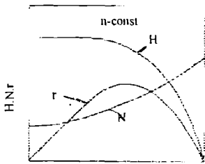
3.4-rasm. Markazdan qochma nasosning ish xarakteristikasi.
