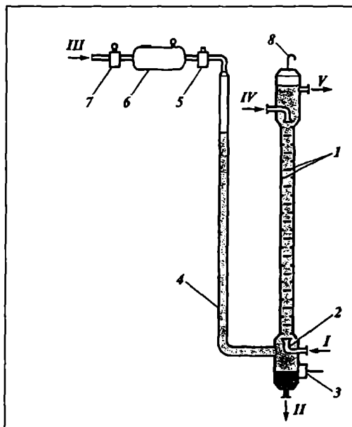
17.11 - rasm. Pulsatsiyali ekstraktorning sxemasi: 1–kontakt moslamalari; 2–taqsimlagich; 3–fazalarning ajralish yuzasini nazorat qilish sistemasi; 4–pulsatsion quvur; 5–pulsator; 6–qalqon idish; 7–saqlovchi klapan; 8–havo chiqargich. Oqimlar: I–yengil faza; II–rafinat; III–havo yoki azot; IV–og‘ir faza; V–ekstrakt.
