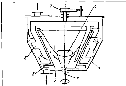
8.9-rasm. Aylanuvchi konusli aralashtirish uskunasi sxemasining sxemasini: 1-qobiq; 2-val; 3-konus; 4-oynak; 5-parrakli aralashtirgich; 6-rama; 7-to'xtatish uchun moslama.
