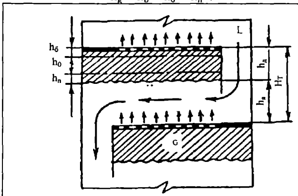
17.14-rasm. Tirgovich balandligini va tarelkalar orasidagi masofani aniqlash.
