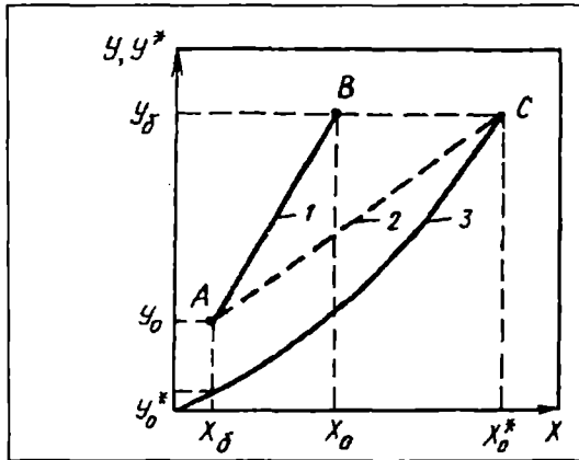
14.2-rasm. Absorbsiya jarayonining ish va muvozanat chiziqlari: 1—absorbentning sarfi L bo'lganidagi ish chizig'i; 2—absorbentning sarfi L_{min} bo'lgandagi ish chizig'i; 3—muvozanat chizig'i Y^* = f(x) .
