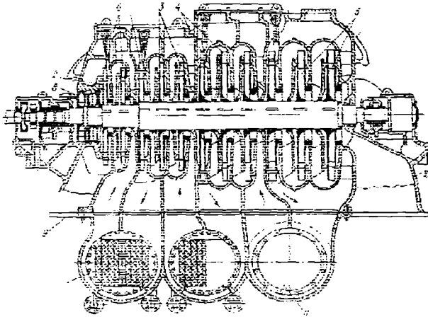
3.21- rasm. Ko'p bosqichli turbokompressor:
