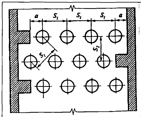
11.8-rasm. Quvurlarning konveksiya kamerasida joylanish sxemasi.
