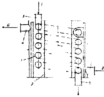
10.9-rasm. Zmeevikli issiqlik almashgich: 1–zmeevik; 2–qobiq; 3,4–patrubkalar; I, II–issiqlik tashuvchi agentlar.
