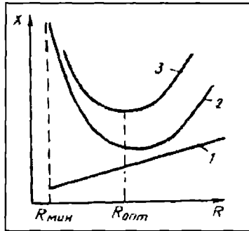
13.11-rasm. Flegma sonining maqbul qiymatini aniqlashga doir: 1–qurilmani ishlatish bilan bog'liq bo'lgan sarflar; 2–kapital xarajatlar; 3–umumiy xarajatlar.
