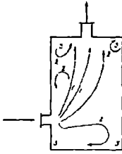
2.12-rasm. Ichi bo'sh uskunadagi oqimlar sxemasi: 1,2-harakat traektoriyasi; 3-harakatsizlik sohasi.
