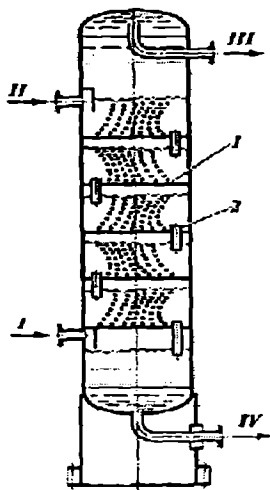
17.10 - rasm. Elaksimom tarelkali ekstraktorning sxemasi: 1—elaksimom tarelka; 2—quyilish patrubkasi. Oqimlar: I—xomashyo; II—erituvchi; III—rafinat eritmasi; IV—ekstrakt eritmasi.
