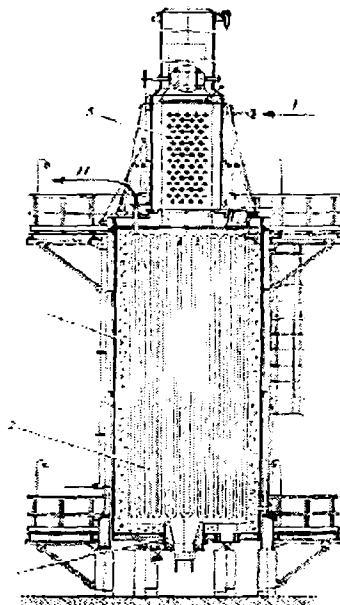
11.5-rasm. SS rusumidagi quvurli pech sxemasi: 1—gorelka; 2—radiant quvurlari zmeevigi; 3—karkas; 4—futerovka; 5—konveksiya quvurlari zmeevigi; Oqimlar: I—mahsulotning kirishi; II—mahsulotning chiqishi. va chiqishi pechning yuqorigi qismida amalga oshiriladi.
