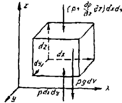
2.5-rasm. Harakatdagi suyuqlikning Eylerni tenglamasini aniqlashga doir.
