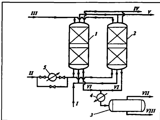
16.4-rasm. Ikkita adsorberli adsorbsion qurilma sxemasi: 1,2—adsorberlar; 3—suv ajratgich; 4—sovitgich; 5—isitgich. Oqimlar: I—dastlabki gaz; II—quritish va sovitish uchun havo; III—desorbsiya uchun sugʻi; IV—desorberlardan chiqayotgan havo; V—quruq gaz; VI—bugʻlar, suv va adsorbat aralashmasi; VII—adsorbat; VIII—suv.
