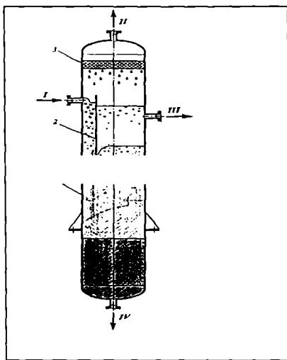
4.4-rasm. Gazoseparator – suv ajratgichning sxemasi: I–qobiq; 2–to'siq; 3–qaytargich. Oqimlar: I–aralashma; II–gaz; III–benzin; IV–suv.
