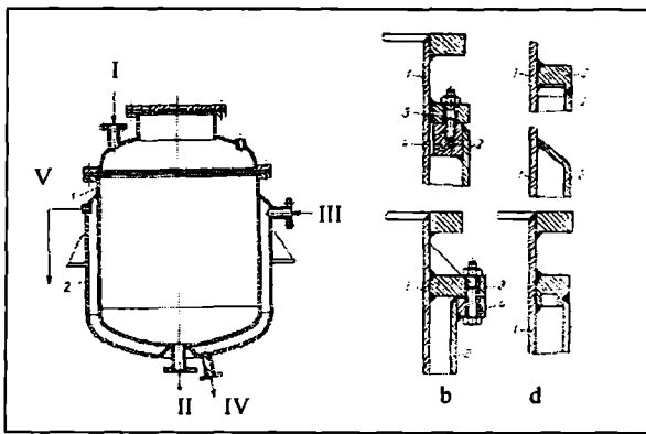
10.12-rasm. G'ilofli issiqlik almashgich(a) va g'ilofni uskunaga biriktirish usullari (b—flanes yordamida; d—payvandlash yo'li bilan): 1—idishlarning qobiqlari; 2—isituvchi g'iloflar; 3—halqalar; 4—flaneslar. Oqimlar: I—sovuq suyuqlik; II—issiq suyuqlik; III—bug'; IV—kondensat; V—havo.
