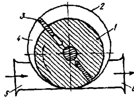
3.10- rasm. Plastinkali nasos: 1 – rotor; 2 – qobiq; 3 – plastinalar; 4 – boʻshliq; 5 – soʻruvchi trubka; 6 – uzatuvchi patrubkasi.
