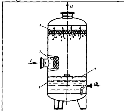
2.14-rasm. To'rli gazsepartori:
