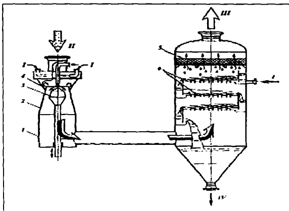
4.15-rasm. «Kox» firmasi gaz tozalash qurilmasining sxemasi: 1–Venturi quvuri; 2–diffuzor; 3–boshqaruvchi konus; 4–konfuzor; 5–to‘rli qaytargich (demister); 6–klapanli tarelkalar. Oqimlar: I–suv; II–dastlabki gaz; III–tozalangan gaz; IV–chiqindilar.
