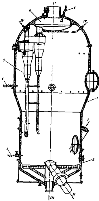
21.6 rasm. Changsimon katalizatorli regeneratori:
