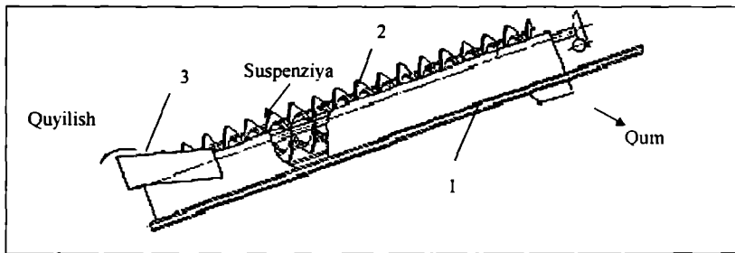
8.4-rasm. Spiralli sinflash uskunasining sxemasi: 1—tog'ora; 2—spiral; 3—to'siq.
