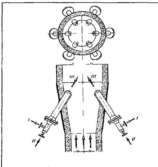
21.9- rasm. Reaktor liftining pastki qismiga «Atomax» soplosini o'rnatish sxemasi: Oqimlar: I—xomashyo; II—suv bug'i; III—bug'-xomashyo aralashmasi.
