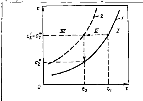
19.1-rasm. Muvozanat va to'yiinish konsentratsiyalarining haroratdan bog'liqligi:
