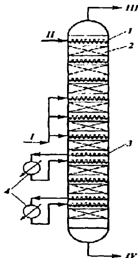
17.9 -rasm. Nasadkali ekstraksion kolonnaning sxemasi: 1—taqsimlovchi tarelka; 2—nasadka qatlarni; 3—bo'g'iq tarelka; 4—oraliq sovitgichlar. Oqimlar: I—xomashyo; II—erituvchi; 3—rafinat eritmasi; ekstrakt eritmasi.
