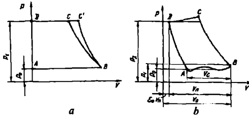
3.26-rasm. Bir bosqichli porshenli kompressorning indikator diagrammasi:
