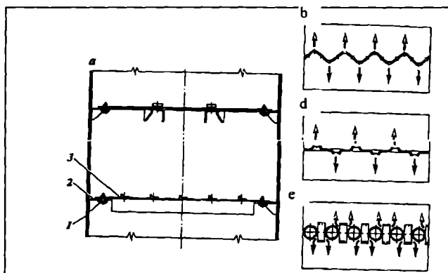
15.7-rasm. Ag‘darilma rusumidagi tarelkalarining sxemalari: a—panjarali tarelka; b—to‘lqinsimon elakli tarelka; d—tirqishlarining chetlari egilgan panjarali tarelka; e—qat-qat burma lenta bilan ta‘minlangan quvurli-panjarali tarelka; 1—kolonna qobig‘i; 2—tayanch halqasi; 3—tarelka seksiyasi.
