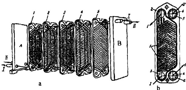
10.10-rasm. Plastinali issbiqlik almashgich: a) qurilmaning sxemasi: A,B – bosh plitalar; 1-5–qat-qat burma qilingan plastinalar; I, II –issiqlik tashuvchi agentlar;b) plastinaning tuzilishi; 1,4–rezinali qistirmalar; 2,3-I–suyuqlik uchun teshiklar; 5,6-II–suyuqlik uchun teshiklar.
