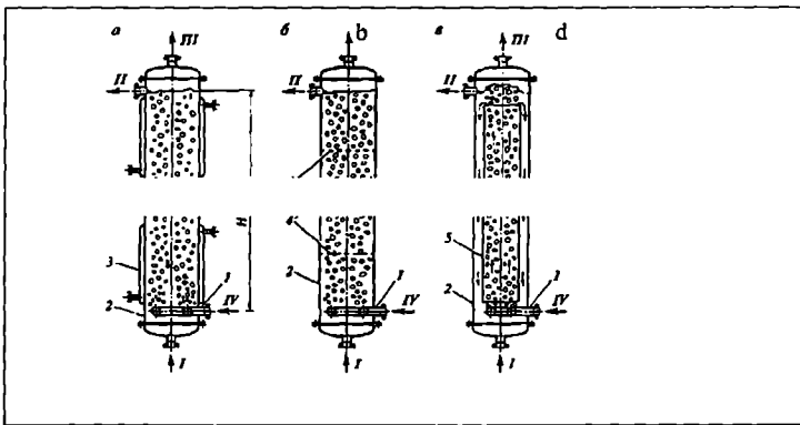
5.3-rasm. Barbotajli aralastirgichli uskunalarning sxemalari: a—ichi bo'sh; b—seksiyali; d—gazliftli; 1—barbotoer; 2—qobiq; 3—sovitish g'illofi; 4—seksiya hosil qiluvchi to'siqlar; 5—sirkulatsiya quvuri. Oqimlar: I—dastlabki suyuqlik; II—chiqayotgan suyuqlik; III—chiqayotgan gaz; IV—kirayotgan gaz.
