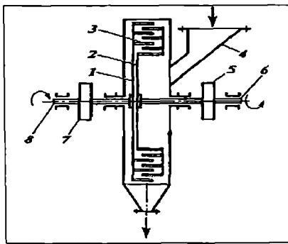
7.6-rasm. Dezintegratorning tuzilish sxemasi: 1,2—disklar; 3—zarba beruvchi paleslar; 4—yuklovchi voronka; 5,7—shkivlar; 6,8—vallar.
