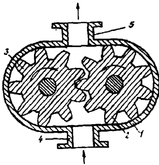
3.9- rasm. Shesterniyali nasos: 1-qobiq; 2, 3-bir-biriga ilashgan ishli shesterniyalar; 4 – soʻruvchi patrubka; 5 – haydash trubka.
