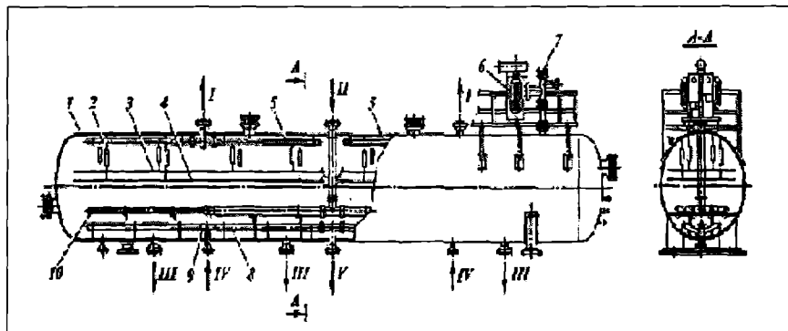
2.11-rasm. Gorizontaal elektrodehidrator EG200-10:
