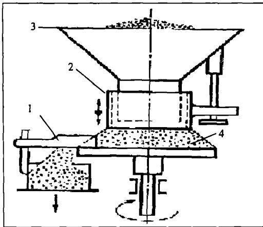
8.7-rasm. Tarekali ta'minlagichning sxemasi: 1-bur.luvchi pichoq; 2-manjeta(qadama eng); 3-qabul qiluvchi bunker; 4-tarelka.
