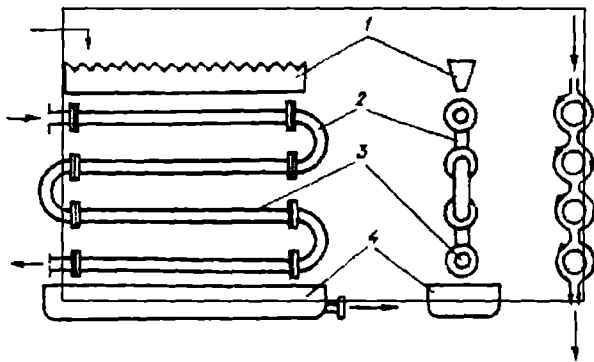
10.8-rasm. Namlanuvchi issiqlik almashgich: 1–tarnov; 2–tirsak; 3–quvur; 4–yig‘gich; I va II – issiqlik tashuvchi agentlar.
