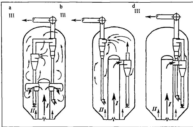
21.7-rasm. Reaktor lifti uchun neft mahsulotlaridan katalizatorni ajratib olish uskunalarining turlari:
