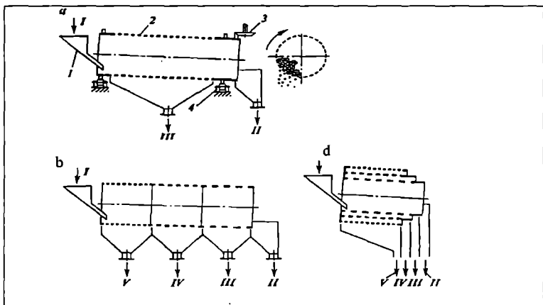
8.2-rasm. Barabanli sim g'alvirli uskunalarining sxemalari: a–bitta g'alvirli: 1–dastlabki materialni berish uchun tarnov; 2–baraban; 3–uzatma moslamasi; 4–tayanch roligi; b–g'alvirlarning ketma-ket joylanishi; d–g'alvirlarning markaziy o'qqa parallel joylanishi. Oqimlar: I–dastlabki material; II–katta o'lchamli fraksiya; III,IV,V–zarrachalarning o'lchami kichrayib boradigan fraksiyalar.
