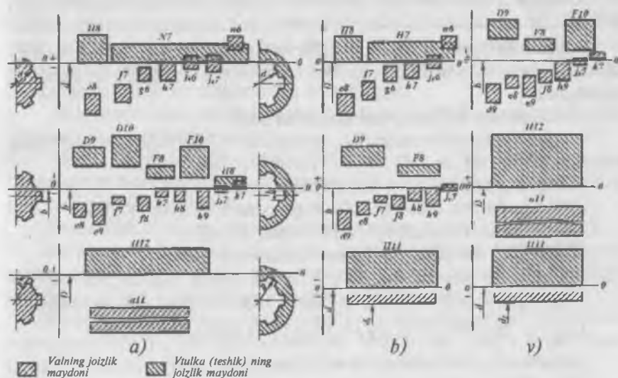
31-rasm. Shliksali vallar va vtulkalar joizlik maydonlarining joylashish sxemasi. a) ichki-d diametr; b) tashqi-D diametr; v) tishlar yon tomoni-b bo'yicha markazlashtirish.
