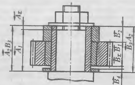
57 – rasm. Ko‘paytirilgan o‘lchamlar zanjiri.
