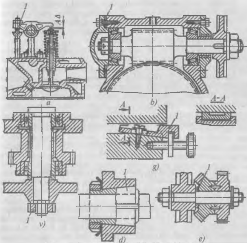
62-rasm. Kompensatordan foydalanishga oid misollar.
