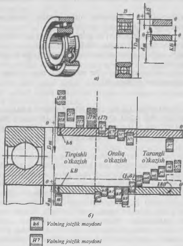
27-rasm. Podshinik halqalari joizlik maydonining joylashish sxemasi.
