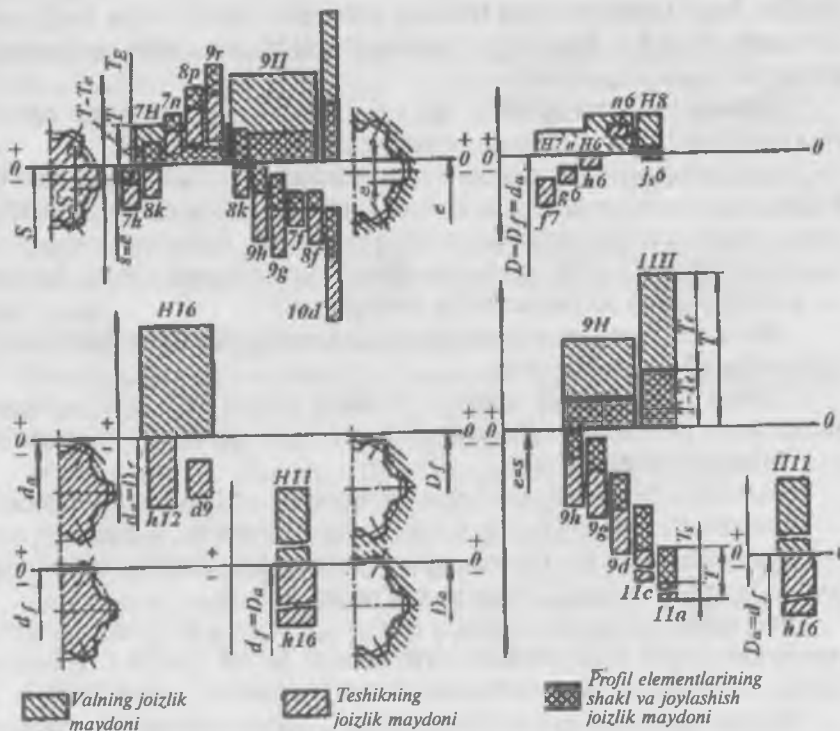
32-rasm. Evolventali shlitsali val va vtulkalarning asosiy parametrlari, joizlik maydonlarining joylashish sxemasi.
