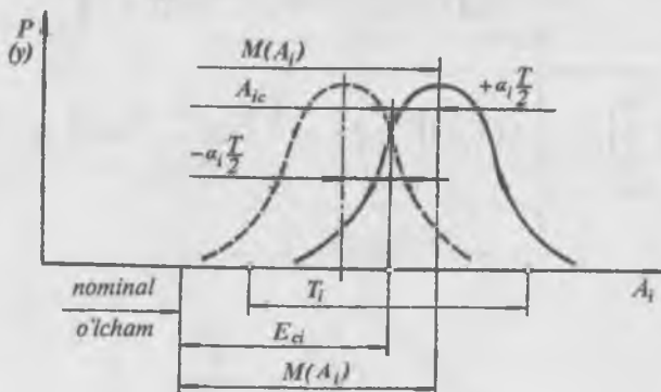
61 – rasm. Joizlik maydoni markazi bilan matematik kutilishning mos tushmaslik koeffitsientini aniqlash.
