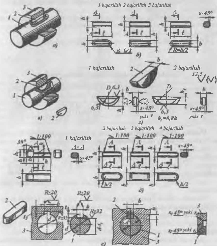
28-rasm. Shponkali birikma va uning turlari.
