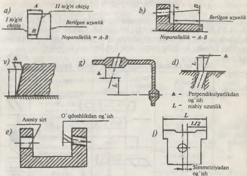
6-rasm. O'qlar va sirtlar joylashishining og'ish turlari.
