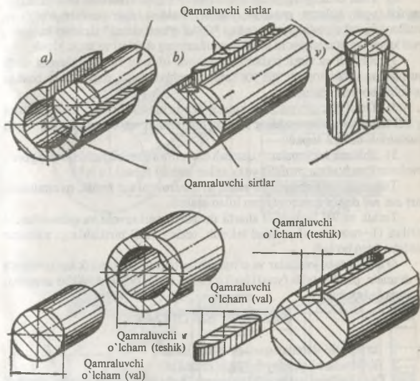
1-rasm. Qamrovchi va qamraluvchi detallar va o'lchamlar.
