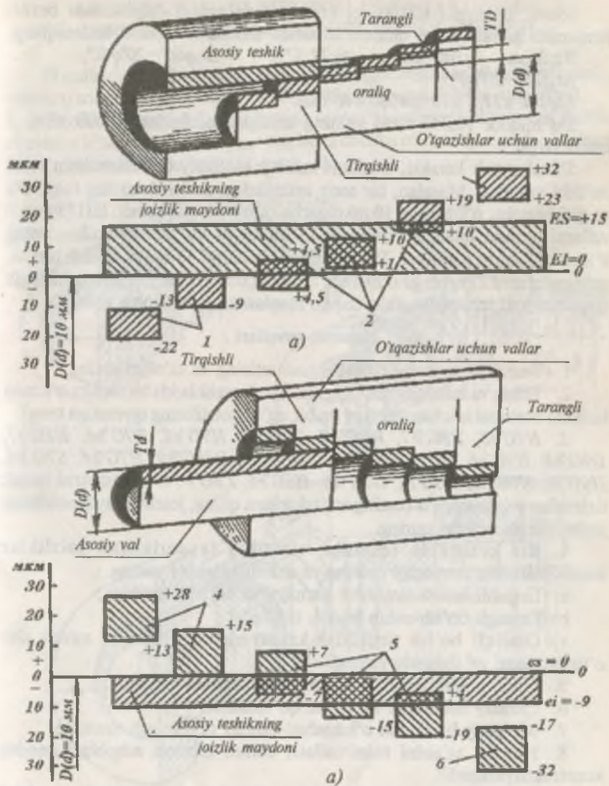
11-rasm. Teshiklar va vallar tizimida o'iqazishlarning joylashishi. a) — teshiklar tizimi. b) — vallar tizimi.
