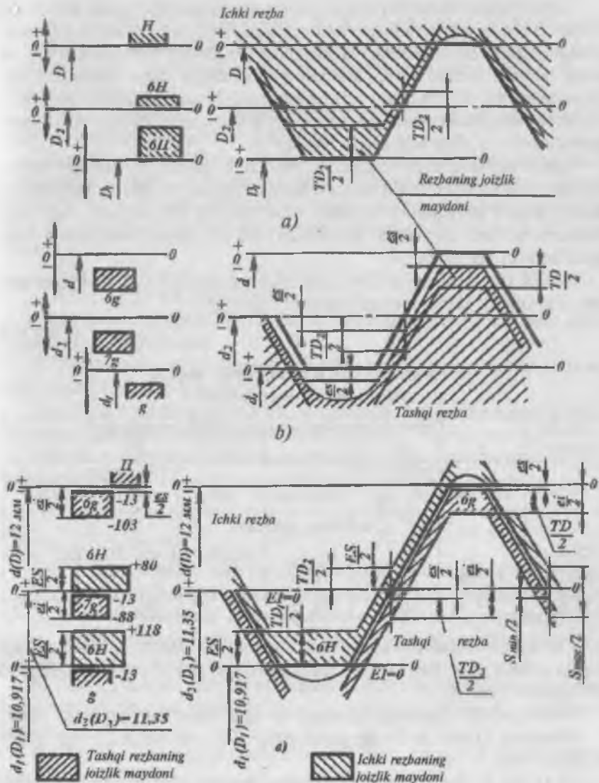
37-rasm. Metrik rezba joizlik maydonlarining joylashish sxemasi, a-ichki, b-tashqi rezbalar uchun, v-tirqishli o'qazishlar bo'yicha birikkan rezbali detallar.
