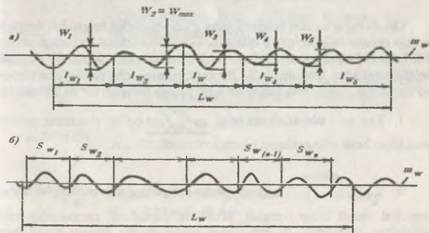
9-rasm. Sirtning to'liqligi.
