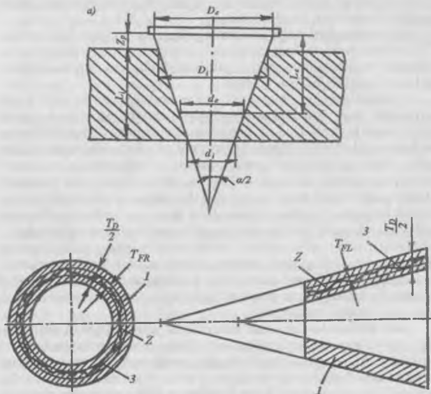
26-rasm. Konusli birikmalarning a) o'lchamlari, b) joylik maydonining joylashishi.
