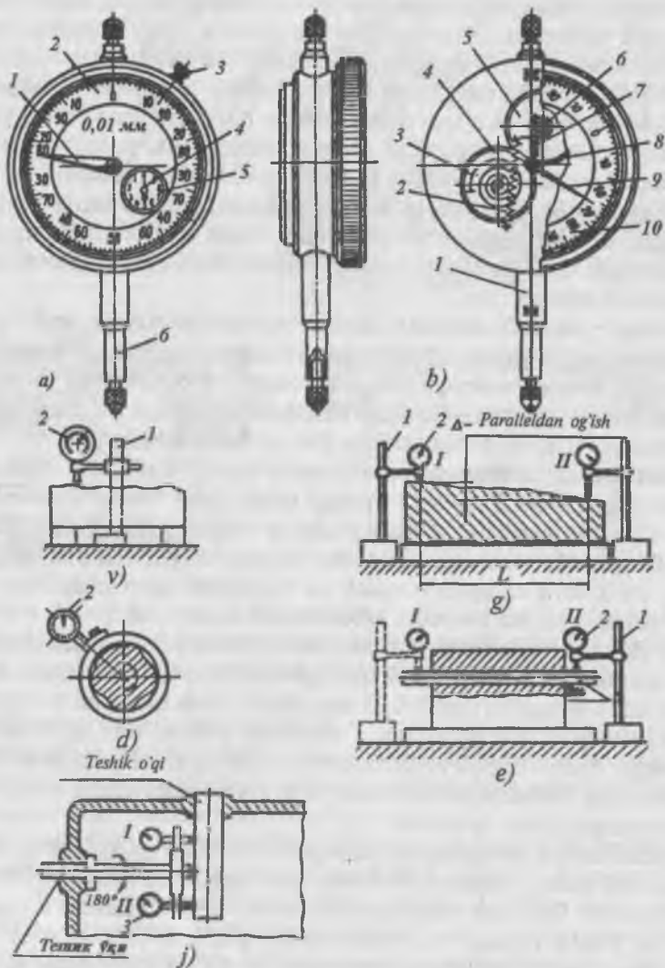
68-rasm. Soat tipidagi indikator (a) va uning tuzilishi (b), chizqlikdan (v), parallellikdan (g), dumaloqlikdan (d), tekislikka nisbatan o'qning parallelligidan (e), o'qlarning perpendikulyarligidan (j) va ishlarni o'lashga doir misollar.
