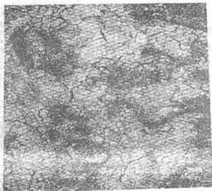
5.52-rasm. O'rta dona strukturali ohaktosh, qayta kristallangan kalsit qoldig'i bilan (to'q kulrang). Nikol. II. kattal. 21.
