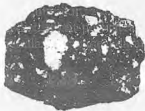
4.80-rasm. Bazalt-porfirit.
