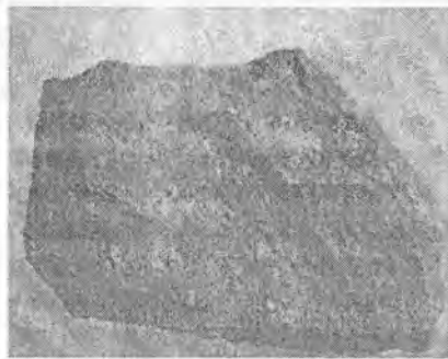
4.49-rasm. Liparit.
