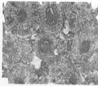
5.47-rasm. G'ovak teksturali yirik oolimli ohaktosh. G'ovakning ko'p qismi kalsit bilan to'ldirilgan. Eotsen, Turkiston yarusi. Shimoliy Farg'ona. Nikol. I1; kattal. 40. A.I.Osipov koli.
