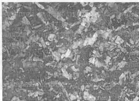
4.25-rasm. Allotriomorf donali struktura. Nikollar +
