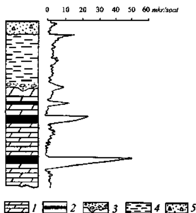
15-rasm. Burg'i qudug'ining gamma karotaj diagrammasi. 1-mergellar; 2-donador fosforit qatlamlari; 3-g'uddali fosforitlar; 4-gillar; 5-to'rtlamchi davr yotqiziqari.
