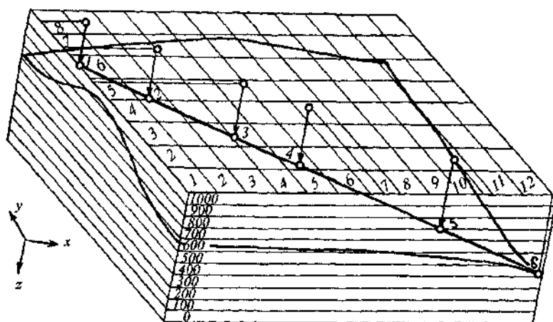
132-rasm. Qiyshiq burchakli aksonometrik proyeksiyali parallelepipedning ko'rinishi. 1-6 yer yorig'i bo'yicha olingan tayanch nuqtalari va ularning koordinatalari yordamida blok-diagrammaga tushirish tartibi. Parallelepipedning yon tomonlarida gorizontal tekisliklarning sathi ko'rsatilgan.
