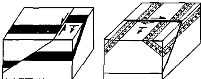
89-rasm. Siljima strukturalarni qiya yotgan qatlamlar va burmali strukturalar yordamida aniqlash.
