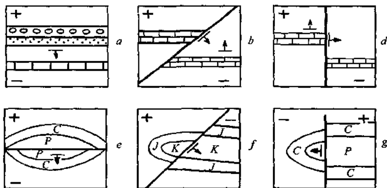
72-rasm. Uzilma struktura turlari: a, e-bo'ylama; b, f-diagonal va d, g-ko'ndalang uzilmalar.
