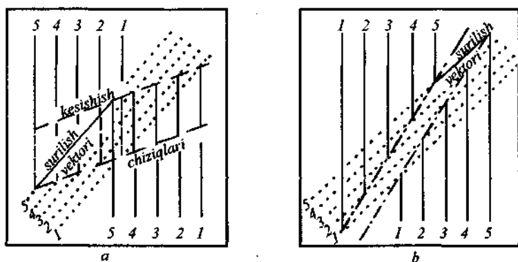
98-rasm. Qiya yotgan tayanch gorizonti va surilish yuzasi yotish chiziqlarining proyeksiyalari orasidagi burchak 90^\circ dan kichik (a) va katta (b) bo'lganda siljima strukturalarning planda ko'rinishi.
