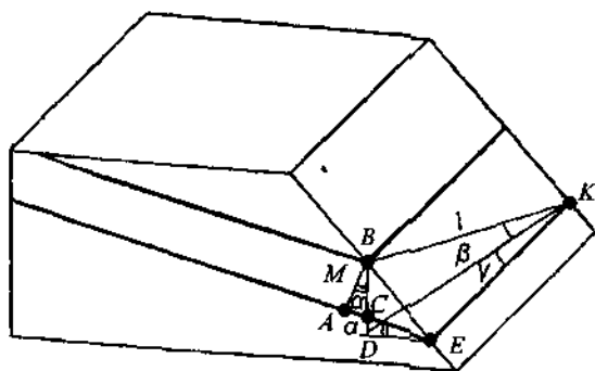
46-rasm. Qatlamning yotishi va relyef qiyaligi bir tomonga yo'nalganda (qatlamning yotish burchagi relyef qiyaligidan kichik bo'lganda) qatlamning haqiqiy qalinligini aniqlash.
