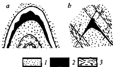
121-rasm. Egarsimon ma'dan shakllari (Velikiy, 1961): a-odatdagi, b-soxta "egar".
