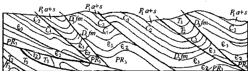
80-rasm. Pog'onali ustsurtimlarlar tizimining kesmada ko'rinishi.
