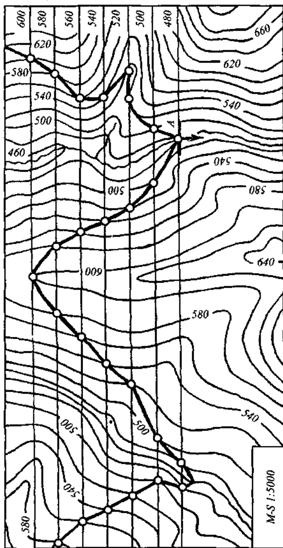
41-rasm. Yotish elementlari orqali qatlam chegaralarini xaritada tushirish.
