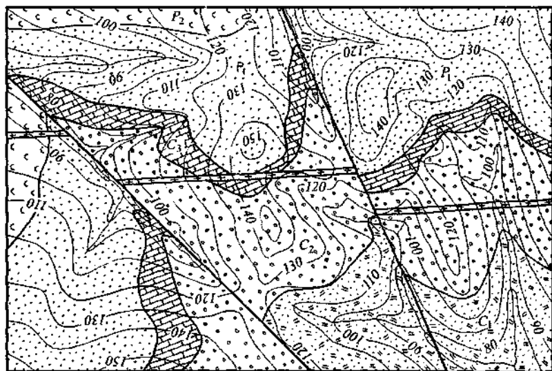
100-rasm. Surilmali yer yoriqlari rivojlangan maydonning geologik xaritasi. C_1 -quyi karbon tuf yotqiziqarlari, C_2 -o'rta karbon gravelitlari, C_3 -yuqori karbon ohaktoshlari, P_1 -quyi perm qumtoshlari, P_2 -yuqori perm effuzivlari. Surilmali yer yoriqlari yo'g'on gora chiziqlar bilan tasvirlangan.
