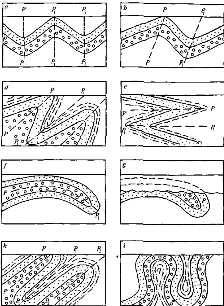
52-rasm. Burmali struktura turlari: a-simmetrik, b-asimmetrik, d-to'ntarilgan qiya, e-yotuvchi, f va g - sho'ng'uvchi, h-izoklinal, i-yelpig'ichsimon burma; PP, P 1 P 1 va P 2 P 2 -burmalarning o'q chiziqlari (A.Ye.Mixaylov bo'yicha).
