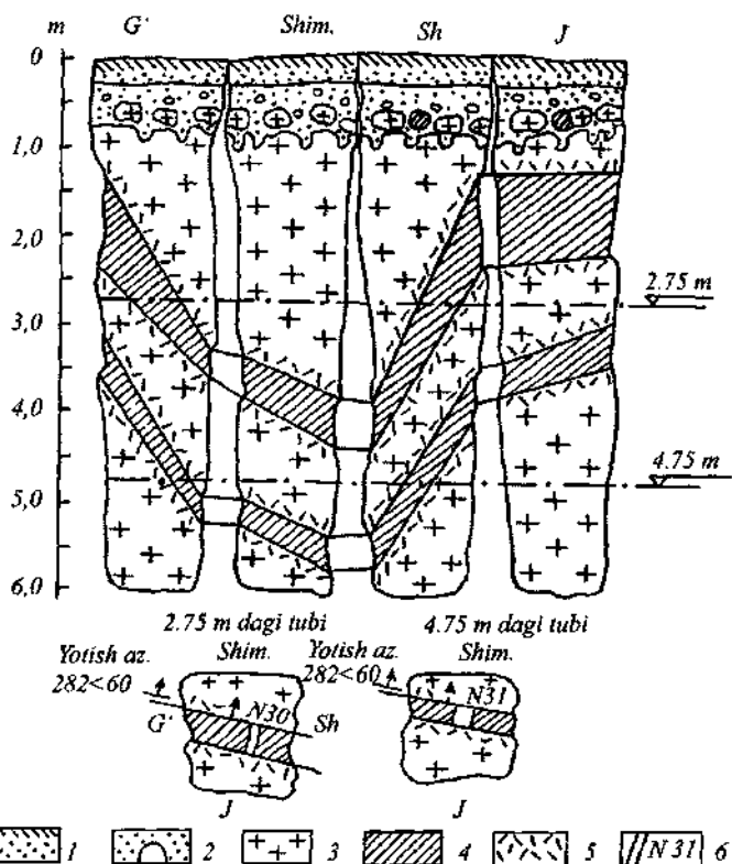
139-rasm. Shurfni hujjatlash namunasi. 1-delyuvial qoplama jinslar; 2-elyuviy jinslari; 3-magmatik jinslar; 4-o'zgargan zonalar; 5-kontakt o'zgarishi; 6-namuna olingan joylar.
