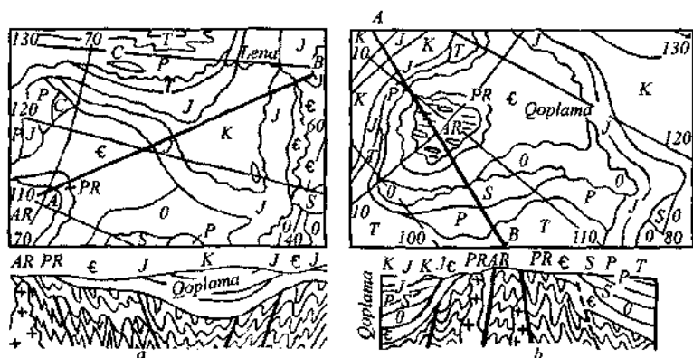
136-rasm. Platformalarning yirik struktura shakllari:
