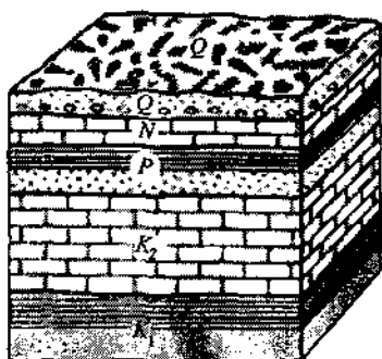
29-rasm. Qatlamlarning birlamchi gorizontal yotishi.
