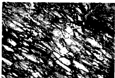
116-rasm. Metamorfik jinslarda konglomerat g'o'laklarning cho'zilganligi.
