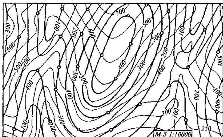
126-rasm. Burg'i quduqlaridan olingan ma'lumotlarga asoslanib tuzilgan struktura xaritasining umumiy ko'rinishi.
