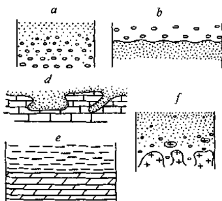
21-rasm. Qatlamlarning biridan ikkinchisiga o'tish holatlari: a-asta-sekin, b-to'qinsimon, d-cho'ntaksimon, f-keskin, e-tub jinslarning (granit) nurashi tufayli qoplama jinslarga aylanishi.
