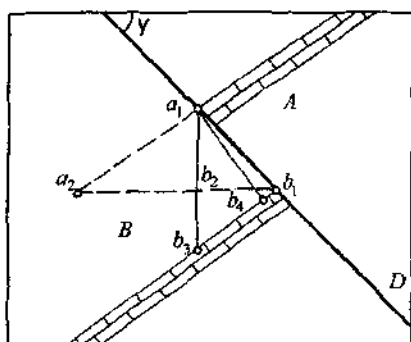
75-rasm. Aksuzilma strukturaning elementlari.
