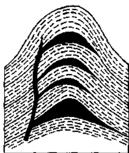
109-rasm. Antiklinal burma yadrosidagi fakolitlar (A.E.Mixaylov bo'yicha).
