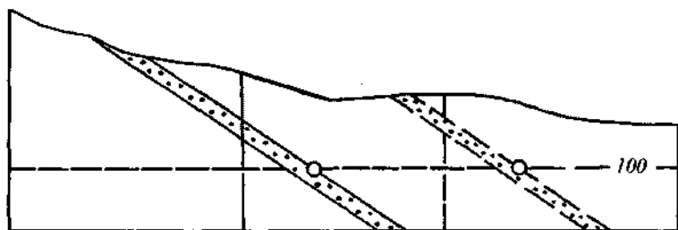
94-rasm. Ikki devordagi geologik vaziyatlarni bir kesmaga tushirish orqali siljimaning haqiqiy surilish amplitudasini aniqlash.
