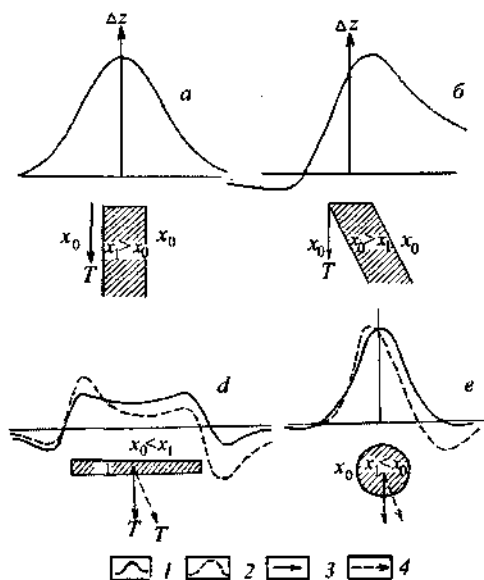
11-rasm. Mahalliy tanalar ustidagi magnetimetrik godograflar: a-vertikal qatlam ustidagi; b-qiya yotgan qatlam ustidagi; d-gorizontaal yotgan qatlam ustidagi va e-shar ustidagisi. 1-vertikal magnitlanishdagi \Delta Z chizmasi; 2-qiya magnitlanishdagi \Delta Z chizmasi; 3- magnitlanayotgan maydon vektor yo'nalishi.
