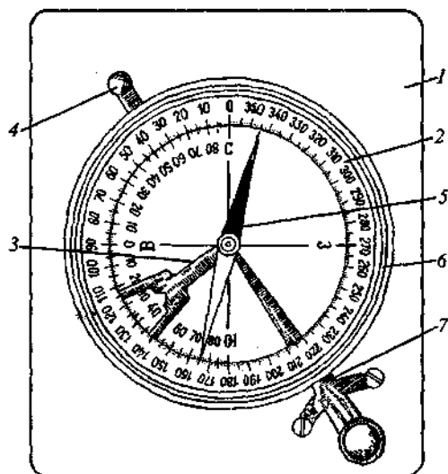
34-rasm. Tog' kompassi. 1-kompass asosi; 2-limbl kompass qutisi; 3-klinometr; 4-klinometri mahkamlash mexanizmi; 5-magnit mili; 6-qoplovchi oynani tutib turuvchi prujina; 7-magnit milini mahkamlash mexanizmi.
