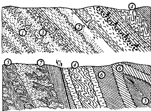
117-rasm. Kuchsiz metamorflashgan qatlamlarning to'ntarilganligini aniqlash belgilari: a-qattam ritmiyligi, 2-simmetrik to'lg'in ryabi, 3-qurish yoriqlari va tosh kemiruvchilar izlari, 4-oqish teksturalari, 5-budinaj, 6-klivaj, 7-migmatitlar (V.N.Pavlinov bo'yicha).
