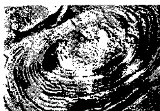
65-rasm. Aerofotosuratlarda burmalı strukturalarning tasviri: a-periklinal, b-sinklinal, d-periklinal va sentriklinal, e-braxiformali sinklinal (V.N.Pavlinov bo'yicha).
