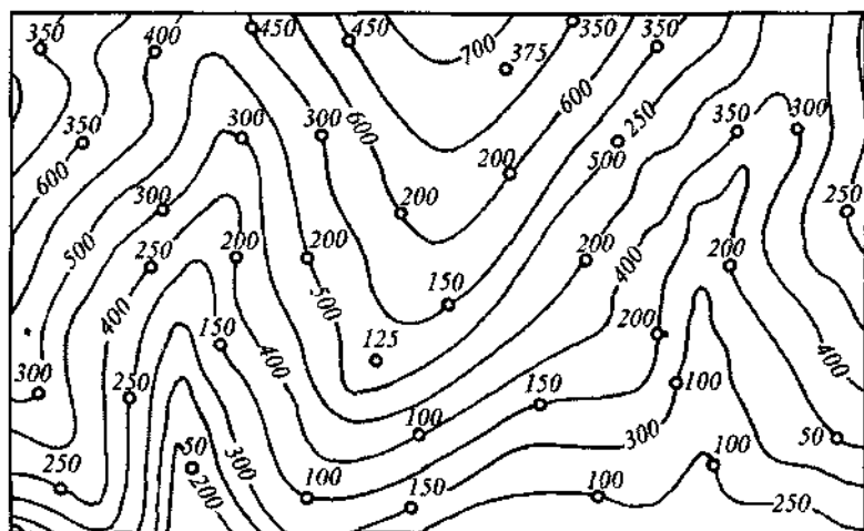
124-rasm. Burg'i quduqlari qazilgan maydonning topografik xartasi. Xaritada burg'i quduqlarining o'rni va tayanch gorizonti yuzasigacha bo'lgan vertikal chuqurtigi ko'rsatilgan.
