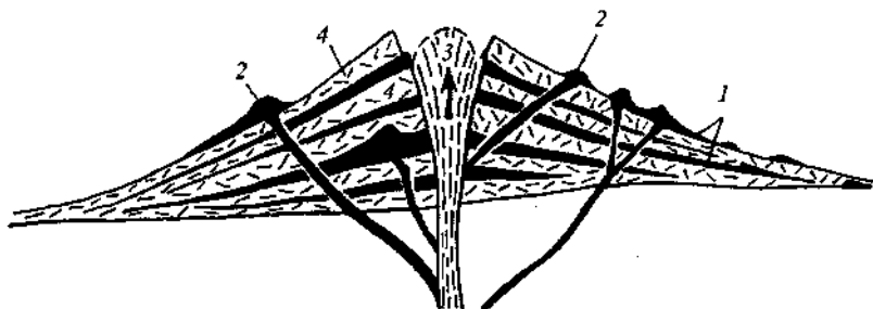
111-rasm. Markaziy tipdagi vulqon konusining vertikal kesmasi. 1-lavalalar; parazit vulqonlarning markazi; 3-ekstruziv gumbaz; 4-piroklastik jinslarning qatlamlari (E.E.Milanovskiy bo'yicha).
