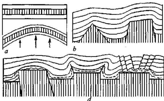
61-rasm. Shtampli burmalarning hosil bo'lish mexanizmi: a-qattiq blokning ko'tarilishi, b-qoplama yotqiziqqlarning cho'zilishi va uzilishi, d-ko'ndalang burilish natijasida hosil bo'lgan blokli va shtampli burmalar (A.Ye.Mixaylov bo'yicha).
