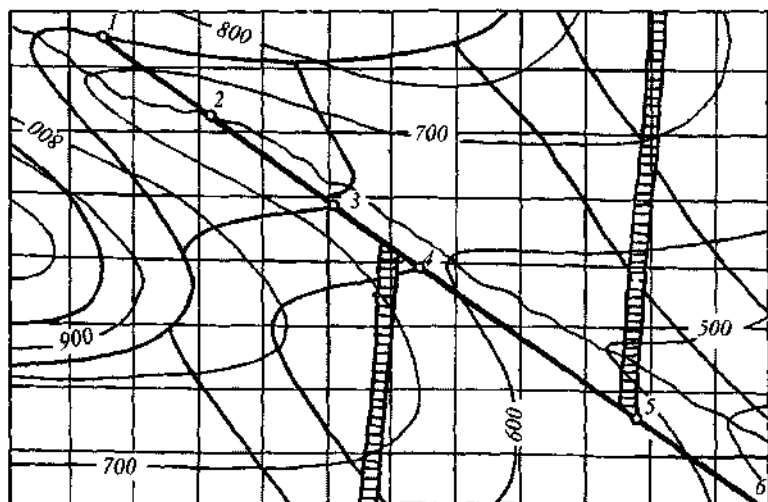
131-chizma. Blok-diagramma tuzilishi kerak bo'lgan geologik xaritaning umumiy ko'rinishi.
