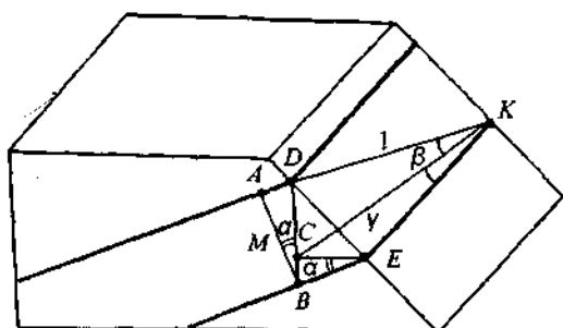
45-rasm. Qatlamning yotishi va relyef qiyaligi qarama-qarshi tomonga yoʻnalganda qatlamning haqiqiy qalinligini aniqlash. M - qatlamning haqiqiy qalinligi, l - qatlamning koʻrinarli qalinligi, \alpha - qatlamning yotish burchagi, \beta - relyefning kesma yoʻnalishidagi qiyalik burchagi, \gamma - qatlamning yoʻnalish chizigʻi bilan kesma chizigʻi orasidagi burchak.
