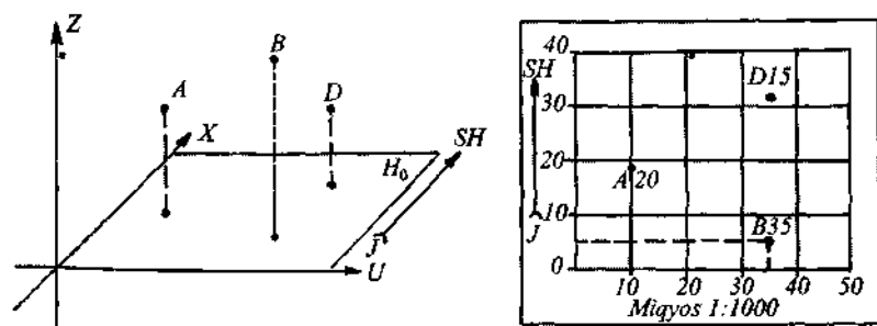
7-rasm. Fazoviy nuqtalarni proyeksiyalash.
