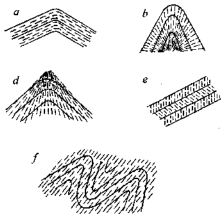
66-rasm. Klivaj xilari: a-qatlamlanishga parallel, kesuvchi klivajlar: b-yelpig'ichsimon; d-teskari yelpig'ichsimon; e-S simon; f-parallel oqish klivajlari (A. Ye. Mixaylov bo'yicha).
