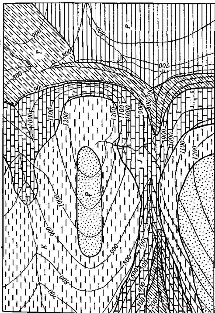
48-rasm. Qatlamlarning qiya yotishi (geologik xarita). 1-Perm yotqiziqchilari (gillar), 2-trias mergellari, 3-yura ohaktoshlari, 4-bo'y alevrolitlari, 5-paleogen qumtoshlari.
