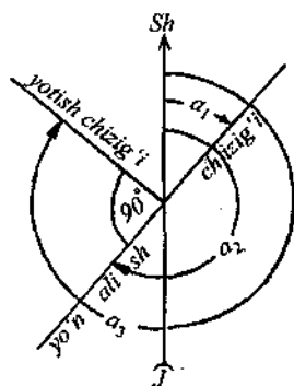
33-rasm. Planda qatlamning yotish elementlari orasidagi munosabat. a_1 va a_2 - yo'nalish chizig'ining azimutlari, a_3 - yotish chizig'ining azimuti.
