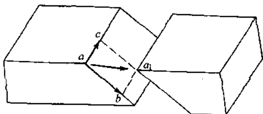
78-rasm. Uzilma-siljima aralash strukturaning ko'rinishi va uning elementlari: aa_1 - blokning harakat yo'nalishi, ac - yer yorig'ining yo'nalish chizig'i, ab - uning yotish burchagi.
