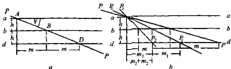
40-rasm. Qatlam qadamini aniqlovchi qurilma. \gamma - qatlamning yotish burchagi, RR-qatlamning vertikal kesmadagi holati, aa, bb, dd - gorizont tekisliklar, h-gorizont tekisliklar orasidagi vertikal masofa, A, B, D - gorizont tekisliklar bilan qatlam yuzasining kesishish nuqtalar, m - qatlam qadami.
