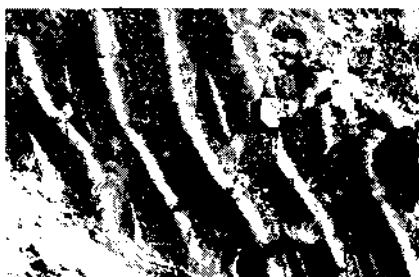
24-rasm. Qatlamning ustki yuzasidagi simmetrik to'lqin ryabi.
