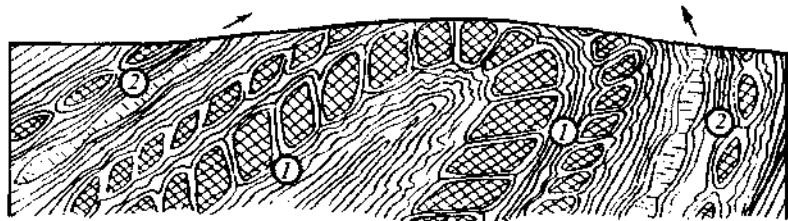
67-rasm. Budinajlarning xillari: 1-sinish budinajlari, 2-to'ntarilgan burmada uzilish budinajlari (A.Ye.Mixaylov bo'yicha).
