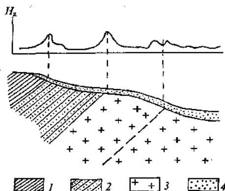
14-rasm. Geologik kesma ustidagi radiokip chizmasi (A.D.Frolov bo'yicha) 1-slanéslar, 2-rogoviklar; 3-granitlar; 4-to'rtlamchi davr yotqiziqdari.
