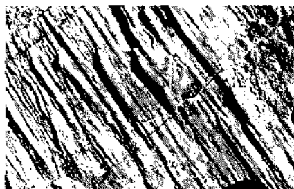
25-rasm. Qatlarning ostki yuzasidagi yuvilish izlarining aks tasviri.
