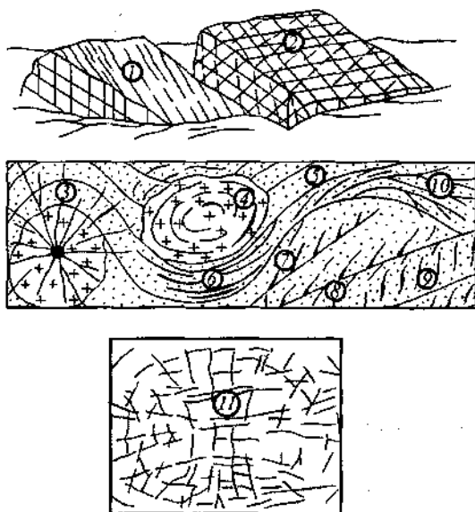
65-rasm. Darzlik xillari va ularning majmualari: 1-qatorli darzliklar; 2-darzliklar tizmasi. Darzlik xillari: 3-radial; 4-konsentrik; 5-kulissimon; 6-marjondek tizilgan (ikki kulisli qator); 7-yon tomonli darzliklar; 8-patsimon; 9-narvonli; 10-“ot dumi”; 11-“toshbaqa struktura“ (A.Ye.Mixaylov bo‘yicha).
