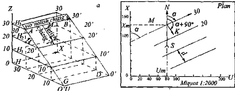
9-rasm. Fazoviy tekislikni proyeksiyalash (a) va uni planda tasvirlash (b).
