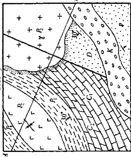
A-B yiqilish bo'yicha geologik kesma
