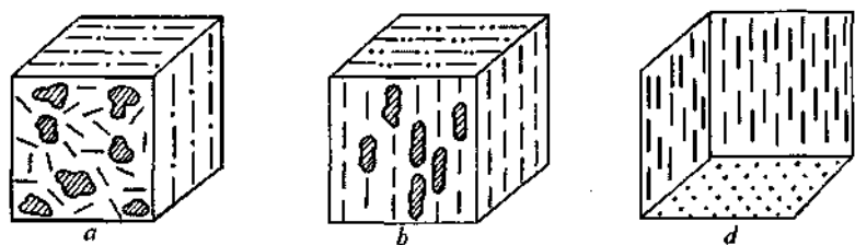
113-rasm. Metamorfik jinslarning teksturasi: a-parallel-slansli; b-chiziqli; d-parallel-chiziqli yoki chiziqli (G.I.Sokratov bo'yicha).
