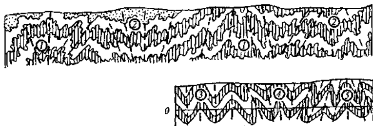
135-rasm. Burmali strukturalar kombinatsiyasi: 1-antiklinoriy; 2-sinklinoriy. Vergent shakllari: 3-konvergentli; 4-divergentli; 5-antivergentli (V.N.Pavlinov bo'yicha).
