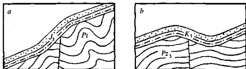
58-rasm. Muvofig (a) va nomuvofig (b) fleksuralar.
