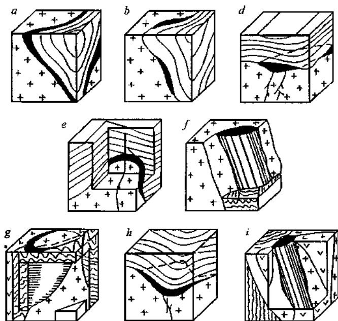
118-rasm. Geologik kontaktlardagi maʼdan shakllari (Korolev, Shextman, 1965): a-maʼdanli qatlam; b-qatlamsimon maʼdan; d-tasmasimon; e-gumbazsimon; f-ustunsimon; g-oʻrab turuvchi; h-togʻorasimon; i-daykali ustunsimon maʼdan tanasi.
