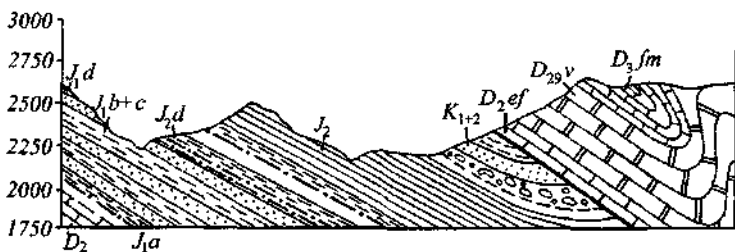
6- rasm. Geologik kesmaning umumiy ko'rinishi.
