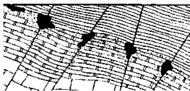
123-rasm. Minerallashtgan ohaktoshlardagi uyasimon ma'danlar (Smirnov, 1969).
