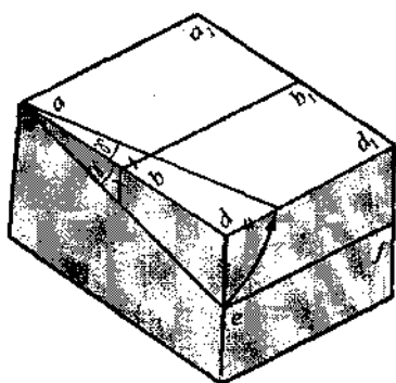
37-rasm. Qatlamning xaritada yotish burchagini aniqlash. a-a , qatlamning yo'nalish chizig'i, b-b , va d-d , 1 - qatlam yo'nalish chiziqlarining gorizont tekislikdagi proyeksiyalari, a-e - qatlamning yotish chizig'i, a-d - yotish chizig'ining gorizont tekislikdagi proyeksiyasi, \alpha - qatlamning yotish burchagi, \alpha_1 - yotish burchagining gorizont tekislikka ko'chirilgan vaziyati, aef - qatlamning o'zaro perpendikulyar vertikal tekisliklardagi o'rni.
