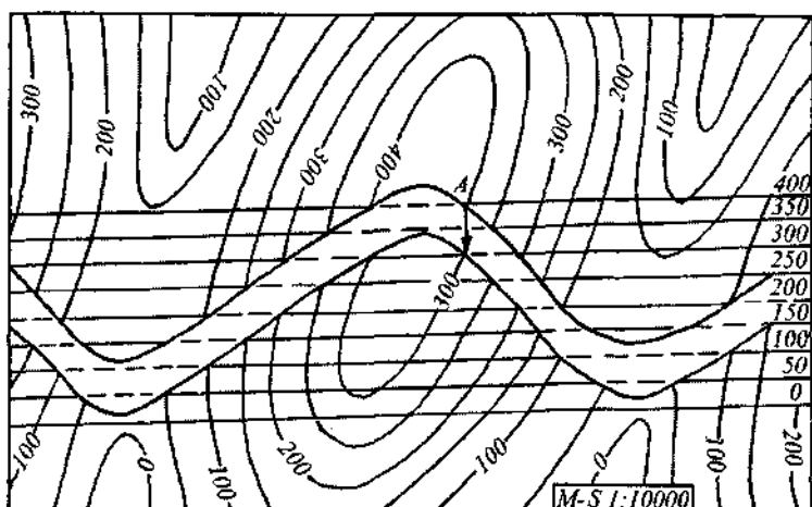
127-rasm. Uzilma orqali murakkablashgan struktura xartasining umumiy ko'rinishi.
