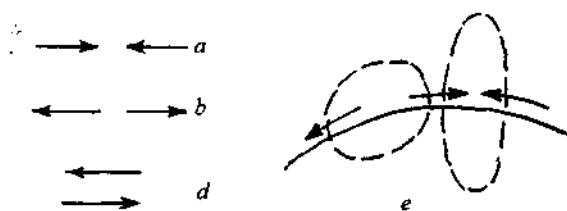
69-rasm. Tektonik kuchlarning harakat yo'nalishi va turlari: a-siquvchi; b-cho'zuvchi; d-parakuchlar; e-sfera yuzasida tektonik kuchlar ta'sirida siqilish va cho'zilish maydonlarining hosil bo'lishi.
