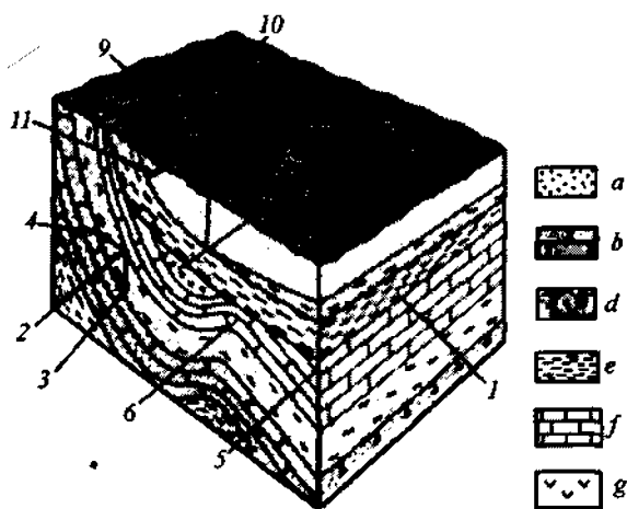
20-rasm. Qatamlarning yotish elementlari. a-qumlar, b-qumtoshlar; d-alevrolitlar; e-gillar; f-ohaktoshlar; g-gips; 1-gil qatlamining ostki yuzasi (ohaktosh qatlamining ustki yuzasi); 2-haqiqiy qalinlik; 3-vertikal qalinlik; 4-gorizontal qalinlik; 5-ohaktosh qatlami qalinligining oshishi; 6-ohaktosh qatlami qalinligining kamayishi; 7-alevrolit qatlamining tugashi (tamom bo'lishi); 8-gips linzasi; 9-yo'nalish chizig'i; 10-yotish yo'nalishi; 11-yotish burchagi.
