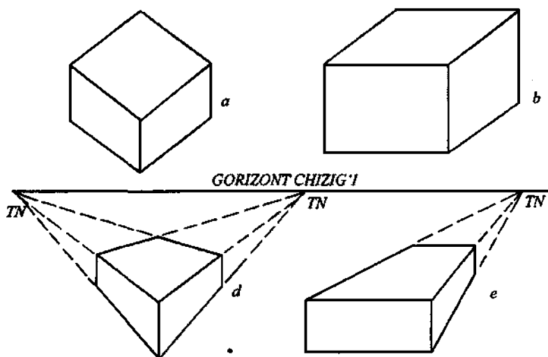
129-rasm. To'g'ri burchakli (a), qiyshiq burchakli (b) aksonometrik proyeksiyasi va qo'sh tutash nurli (d), yakka tutash nurli (e) perspektiv proyeksiyalarning blok-diagrammalari.
