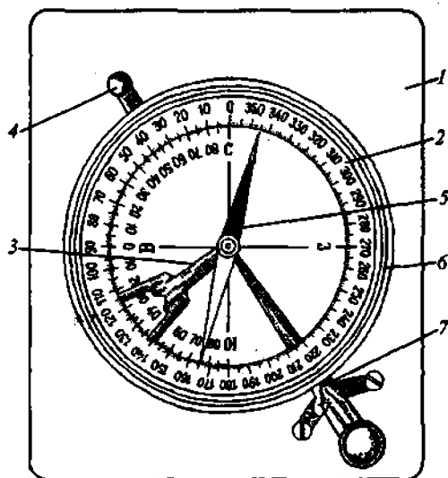
34-rasm. Tog‘ kompassi. 1-kompas asosi; 2-limbl kompas qutisi; 3-klinometr; 4-klinometrni mahkamlash mexanizmi; 5-magnit mili; 6-qoplovchi oynani tutib turuvchi prujina; 7-magnit milini mahkamlash mexanizmi.
