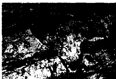
83-rasm. Ikkita uzilmali strukturadan tashkil topgan grabenning fotosurati.
