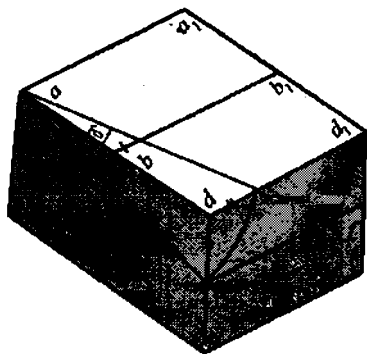
37-rasm. Qatlarning xaritada yotish burchagini aniqlash. a-a , qatlarning yoʻnalish chizigʻi, b-b , va d-d , l - qatlam yoʻnalish chiziqlarining gorizont tekislikdagi proyeksiyalari, a-e - qatlarning yotish chizigʻi, a-d - yotish chizigʻining gorizont tekislikdagi proyeksiyasi, \alpha - qatlarning yotish burchagi, \alpha_1 - yotish burchagining gorizont tekislikka koʻchirilgan vaziyati, aef - qatlarning oʻzaro perpendikulyar vertikal tekisliklardagi oʻrni.
