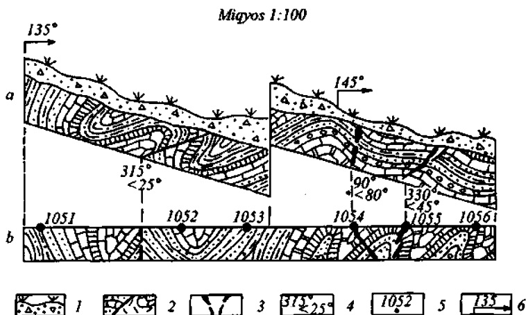
138-rasm. Kanavani hujjatlash namunasi. 1-delyuvial qoplama jinrlar; 2-tub jinrlar; 3-tomirlar; 4-yotish elementlari; 5-namuna olingan nuqtalar; 6-yo'nalish azimuti.
