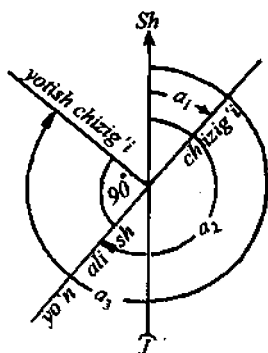
33-rasm. Planda qatlarning yotish elementlari orasidagi munosabat. a_1 va a_2 - yo'nalish chizig'ining azimutlari, a_3 - yotish chizig'ining azimuti.
