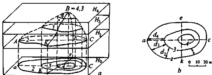
10- a rasmda. Topografik yuzani proyeksiyalash.
