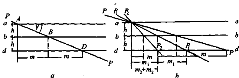
40-rasm. Qatlam qadimini aniqlovchi qurilma. \gamma - qatlamning yotish burchagi, RR - qatlamning vertikal kesmadagi holati, aa, bb, dd - gorizontall tekisliklar, h - gorizontall tekisliklar orasidagi vertikal masofa, A, B, D - gorizontall tekisliklar bilan qatlam yuzasining kesishish nuqtalar, m - qatlam qadami.
