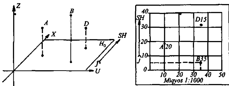
7-rasm. Fazoviy nuqtalarni proyeksiyalash.
