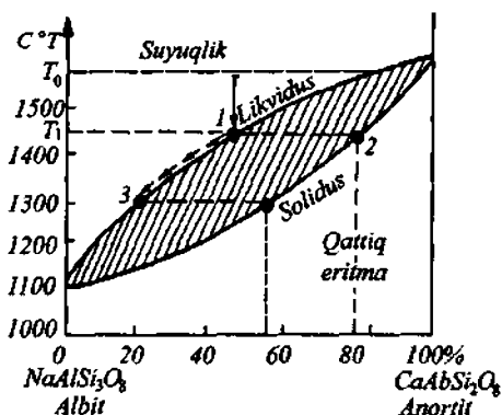
102-rasm. Plagioklaz qatoridagi qattiq eritmalar uchun suyuqlanish diagrammasi (N. Bouen bo'yicha). Shrixlar bilan belgilangan maydonda kristallar va suyuqlikning birga mavjud bo'lishi ko'rsatilgan. Suyuqlikdan ajralib chiquvchi kristallar tarkibi absissa o'qida aniqlanadi. 1-3-suyuqlikning kristallanish bosqichlari rivojlanishi.
