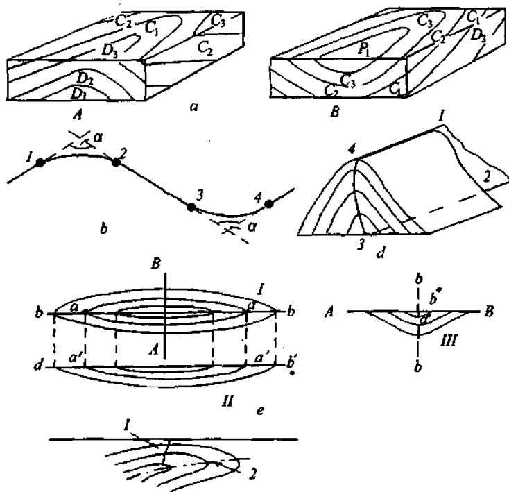
50-rasm. Burma va uning elementlari. (A) antiklinal va sinklinal (B) burmalar; b-burma qanotlari va gulfi; d-burma o'q tekisligi; I-planda, II-bo'ylama kesmada va III-ko'ndalang kesmada ko'rinishi; e - burma o'rkachi, 1-o'rkach tekisligi, 2-o'q tekisligi (A.Ye. Mixaylov bo'yicha).
