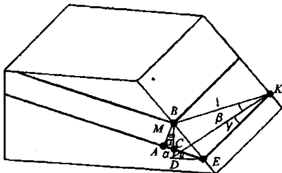
46-rasm. Qatlarning yotishi va relyef qiyaligi bir tomonga yo'nalganda (qatlarning yotish burchagi relyef qiyaligidan kichik bo'lganda) qatlarning haqiqiy qalinligini aniqlash.
