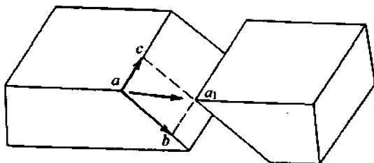
78-rasm. Uzilma-siljima aralash strukturaning ko'rinishi va uning elementlari: aa_1 - blokning harakat yo'nalishi, ac - yer yorig'ining yo'nalish chizg'i, ab - uning yotish burchagi.
