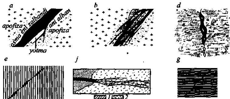
119-rasm. Tomirli ma'dan shakllari (Smirnov, 1969, Bogdanovich, 1913): a-oddiy, b-murakkab (o'zgarigan jinslar maydoni nuqtalar bilan kirsatilgan), d-zanjirsimon, e-tasbehimon, f-shoxlangan (1-qo'ng'ir gneys, 2-kvarsli porfir), g-kamerasimon.
