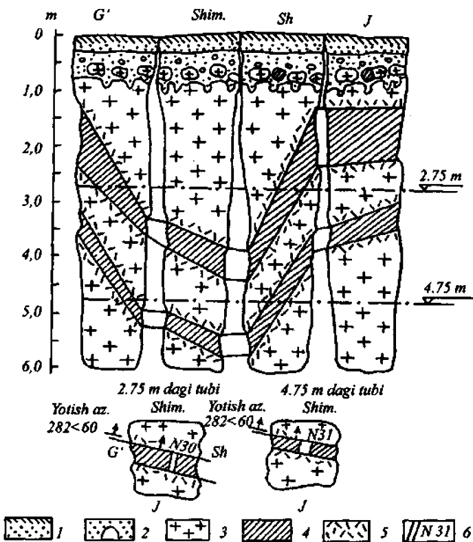
139-rasm. Shurfai hujjatlash namunasi. 1-delyuvial qoplama jinslar; 2-elyuviy jinslari; 3-magmatik jinslar; 4-o'zgargan zonalar; 5-kontakt o'zgarishi; 6-namuna olingan joylar.
