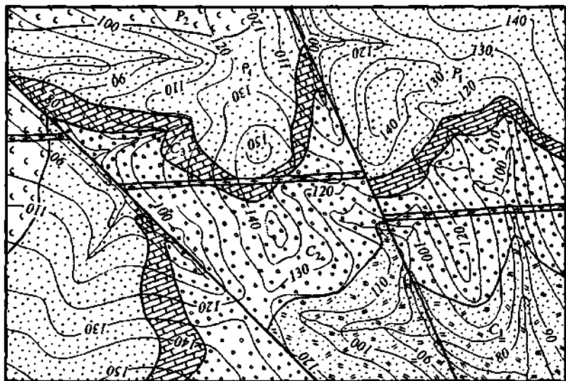
100-rasm. Surilmali yer yoriqlari rivojlangan maydonning geologik xaritasi. C_1 -quyi karbon tuf yotqizilari, C_2 -o'rtta karbon gravelitlari, C_3 -yuqori karbon ohaktoshlari, P_1 -quyi perm qumtoshlari, P_2 -yuqori perm effuzivlari. Surilmali yer yoriqlari yo'g'on qora chiziqlar bilan tasvirlangan.
