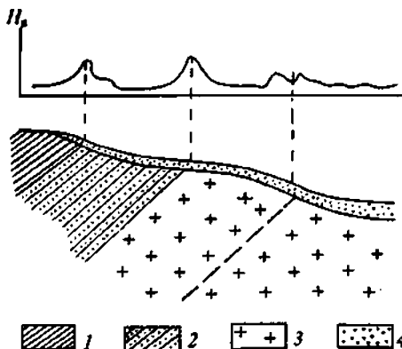
14-rasm. Geologik kesma ustidagi radiokip chizmasi (A.D.Frolov bo'yicha) 1-slanestlar, 2-rogoviklar; 3-granitlar; 4-to'rtlamchi davr yotqiziqdari.
