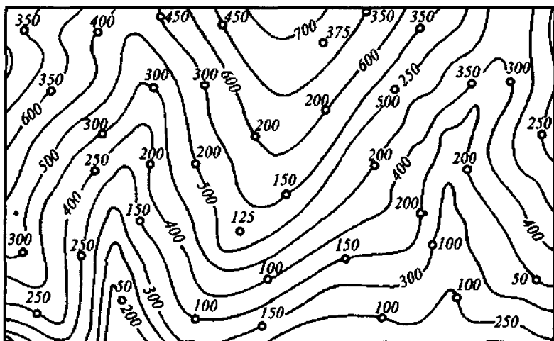
124-rasm. Burg'i quduqlari qazilgan maydonning topografik xartasi. Xaritada burg'i quduqlarining o'rni va tayanch gorizonti yuzasigacha bo'lgan vertikal chuqurligi ko'rsatilgan.
