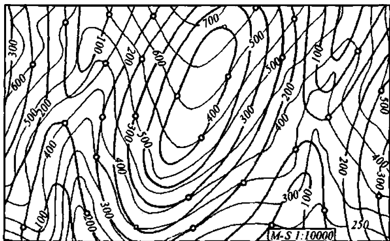
126-rasm. Burg'i quduqlaridan olingan ma'lumotlarga asosanib tuzilgan struktura xartasining umumiy ko'rinishi.
