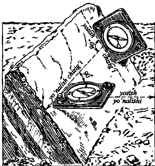
35-rasm. Yotish elementlarini tog' kompassi yordamida aniqlash.
