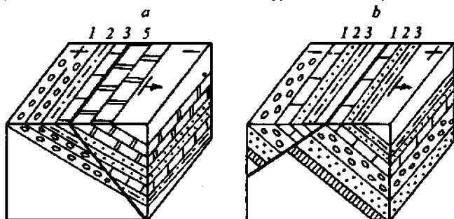
86-rasm. Yer yorig'ining yo'nalish chizig'i qatlamlarnikiga parallel o'tgandagi vaziyat tasviri.
