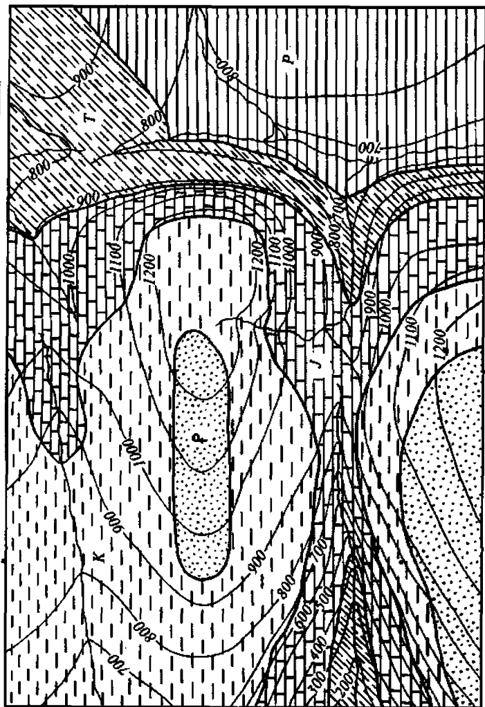
48-rasm. Qatlamlarning qiya yotishi (geologik xarita). 1-perm yotiqizlari (gillar), 2-trias mergellari, 3-yura ohaktoshlari, 4-bo'y alevrolitlari, 5-paleogen qumtoshlari.
