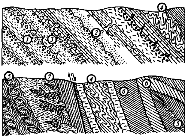
117-rasm. Kuchsiz metamorflashgan qatlamlarning to'ntarilganligini aniqlash belgilari: 1-qattam ritmiyligi, 2-simmetrik to'qin ryabi, 3-qurish yoriqlari va tosh kemiruvchilar izlari, 4-oqish teksturalari, 5-budinaj, 6-klivaj, 7-migmatitlar (V.N.Pavlinov bo'yicha).
