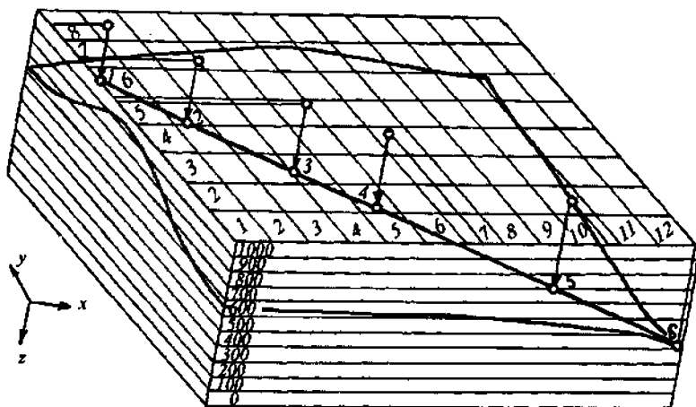
132-rasm. Qiyshiq burchakli aksonometrik proyeksiyalı paralelepipedning ko'rinishi. 1-6 yer yorig'i bo'yicha olingan tayanch nuqtalari va ularning koordinatalari yordamida blok-diagrammaga tushirish tartibi. Parallelepipedning yon tomonlarida gorizontal tekisliklarning sathi ko'rsatilgan.
