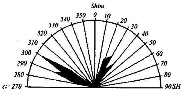
68-rasm. Darzliklar yo'nalishining gul-diagrammasi. Miqyosning bir bo'limi bitta darzlikka to'g'ri keladi (A.Ye.Mixaylov bo'yicha).
