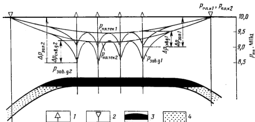
Рис. 102. Изменение \Delta p_{зал} , \Delta p_{скв.д} и p_{пл.тек} при снижении p_{заб.г} .
