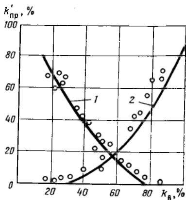
Рис. 9. Зависимость относительных проницаемостей k'_{пр} пористой среды для жидкости (1) и газа (2) от водонасыщенности k_v пустотного пространства в песчанниках (а) и пористых известняках и доломитах (б) (по Ш. К. Гиматудинову)
