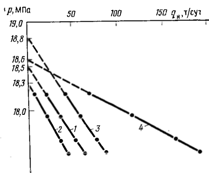
Рис. 103. Индикаторные диаграммы нефтяных пластов I (1), II (2), III (3) и эксплуатационного объекта в целом (4).
