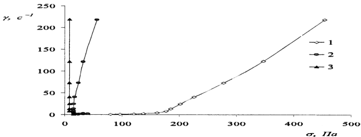
Рис. 1. Зависимость градиента скорости ( \gamma ) напряжения сдвига ( \sigma ) для мази «Ханделии» при различной температуре: 1 – 25 °С; 2 – 40 °С; 3 – 55 °С. напряжения сдвига с ростом температуры.
