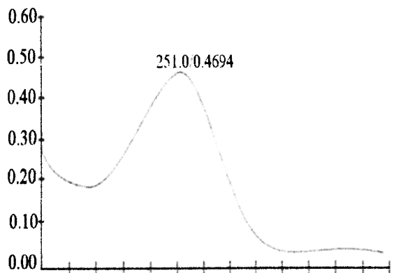
Рис. 1. УФ-спектр РСО глицирризиновой кислоты
