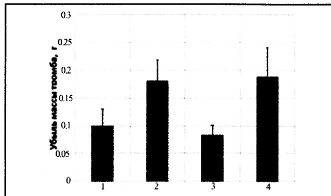
Рис. 1. Убыль массы искусственного тромба при действии ядов. 1 - гюрза, 2 - эфа, 3 - гадюка обыкновенная, 4 - гадюка степная
