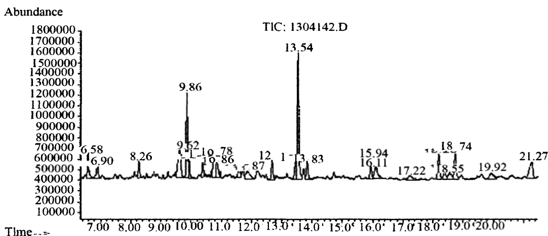
Рис 1. Хроматограмма летучих веществ капсул «СЕДАРЕМ»
