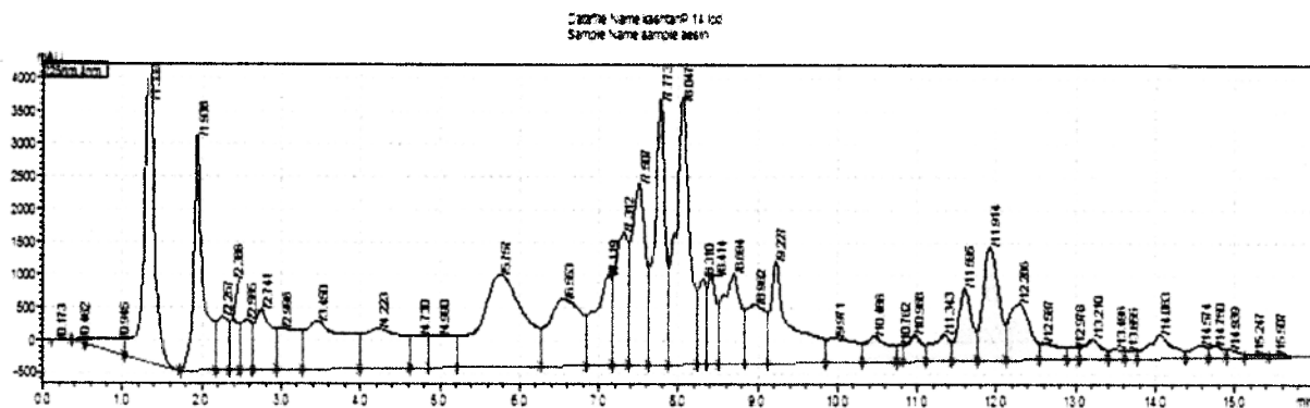
Рис.1. ВЭЖХ-МС водно-спиртового экстракта семян конского каштана. Пики сапонинов окрашены
