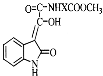
Коэффициенты распределения метиловых эфиров N-[(2-оксоиндолиниден-3)-2-оксиацетил]аминокислот в системе октанол-1 – вода
