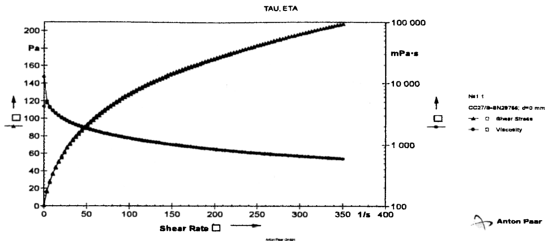
Рис. Зависимость напряжения сдвига ( \tau , Па) и вязкости ( \eta , Па) от градиента скорости ( \dot{\gamma} , \text{с}^{-1} ) экспериментальных образцов геля на основе ГМЦ
