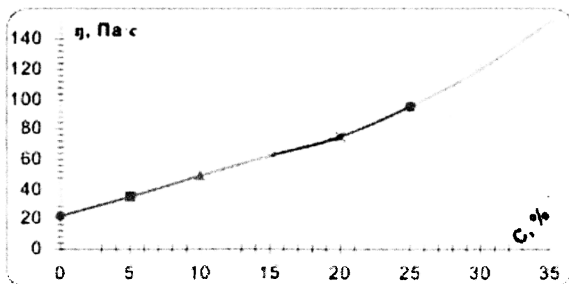
Рис.1. Зависимость структурной вязкости модельных образцов от концентрации масляной фазы
