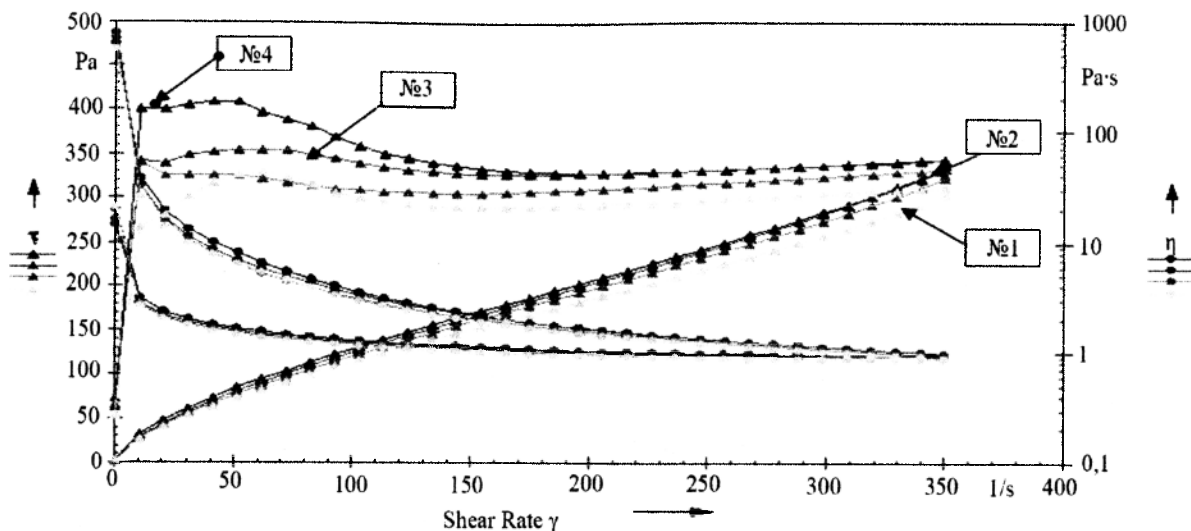
Рисунок 1. Реограммы течения полиэтиленоксидных мазевых основ и графики зависимости структурной вязкости от градиента скорости сдвига.
