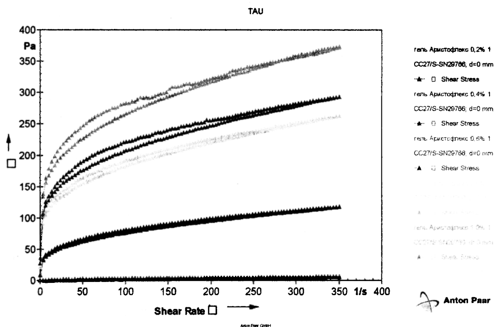
Рисунок 1. Реограммы гелей Aristoflex®AVC
