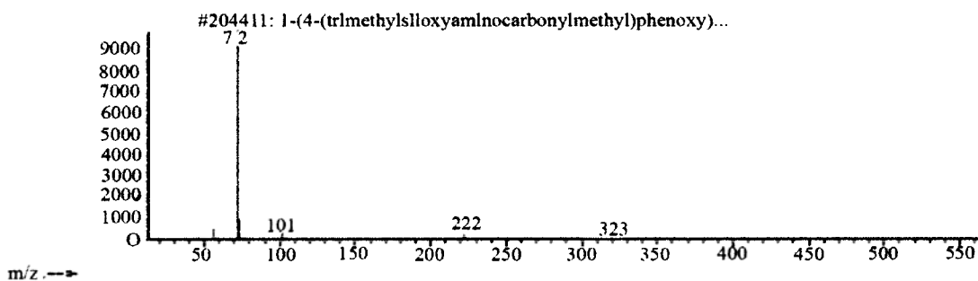
Рис. 1. ГХ/МС профил субстанции ателолола (5 мг в 1 мл)
