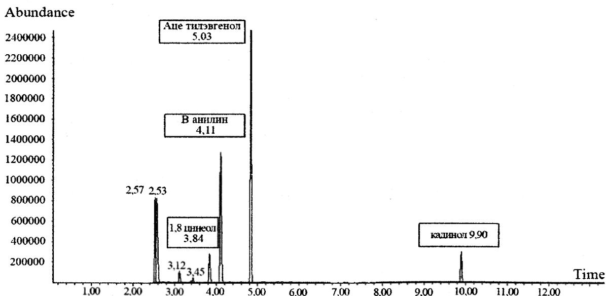
Хромато-масс-спектр материала «Кариосан» фирмы «Омега Дент».
