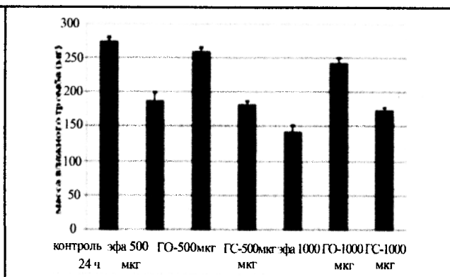
Рис. 2. Действие ядов эфы, гадюк обыкновенной (ГО) и степной (ГС) на тромбы из донорской крови.
