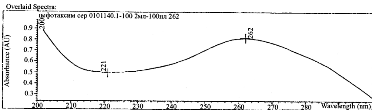
Рис.3 Спектрофотометрия Цефотаксима.
