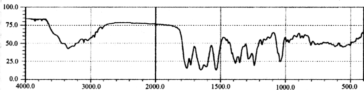
Рис.2 ИК-спектрометрия Цефотаксима.
