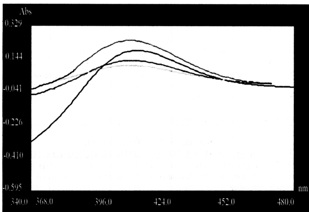
1-расм. Полимер пардадаги флавоноидларнинг УФ – спектрофотометрда олинган натижалари
