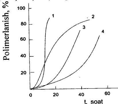
17-rasm. Kaliy laurat konsentratsiyasining izoprenni 50^{\circ}\text{C} da emulsion polimerlanish tezligiga ta'siri. Sovun konsentratsiyasi: 1 - 0,5 M, 2 - 0,1 M, 3 - 0,04 M, 4 - 0,01 M.
