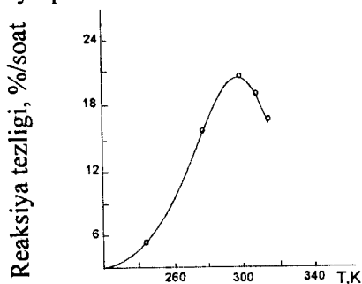
122-rasm. Xlorometil reaksiyasi boshlang'ich tezligining haroratga bog'liqligi.
