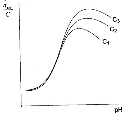
82 – rasm. Har xil konsentrat-siyali polikislota eritmasi keltirilgan qovushqoqligining muhit pH iga bog'liqligi ( c_1 > c_2 > c_3 ).
