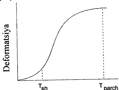
107-rasm. To'rsimon amorf polimerning termomexanik egri.
