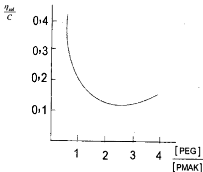
83-rasm. Polimetakril kislotasi bilan polietilenglikol aralashmasi suvli eritmalari keltirilgan qovushqoqligining tarkib bilan o'zgarishi.
