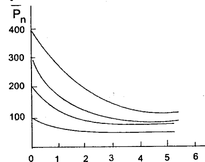
Destruksiyalovchi konts., mol. % 27-rasm. Turli xil polimerlanish darajasiga ega polimerning destruksiyanishi.
