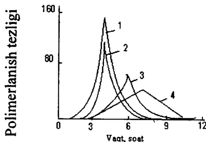
29-rasm. Kaprolaktamning suv ishtirokidagi polimerlanish tezligi 1- 1,96%; 2-1,56%; 3-0,76%; 4-0,5% H 2 O.
