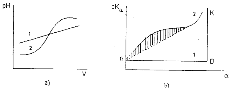
79-rasm. Potensiometrik titrlash egri chiziqlari.
