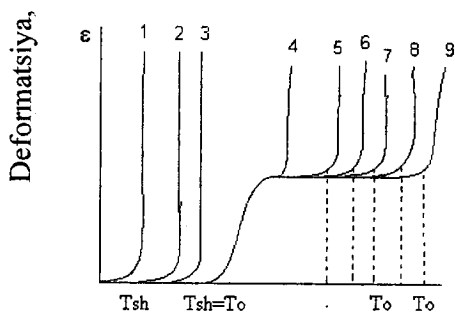
106- rasm. Chiziqsimon polimergomologlar qatorining egri chiziqlari. Egri chiziqdagi raqamlarning ortib borishi polimerlanish darajasining oshishiga mos keladi.
