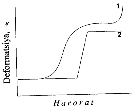
88-rasm. Polimerlarning termomechanik egri chiziqlari;
