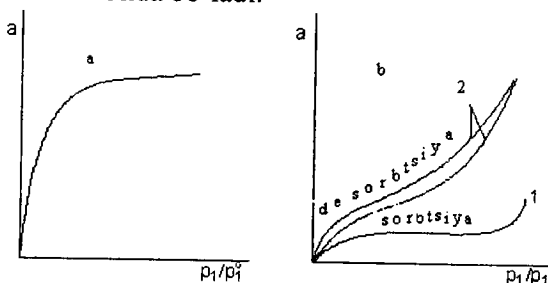
128-rasm. Bir jinsli mayda g'ovakli sorbentlar (a), g'ovaksiz (b, 1 egri chiziq) va ko'chuvchan g'ovakli sorbentlarda (b, 2 egri chiziq) bug'lar sorbsiyasining tipik izotermalari.
