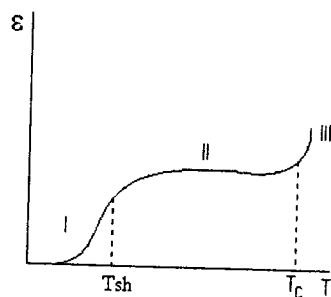
105 – rasm. Amorf polimerning termomexanik egri chizig'i. 1-shishasimon holat; 2 – yuqori elastik holat va 3– qovushqoq – oquvchan holat oraliqlari.
