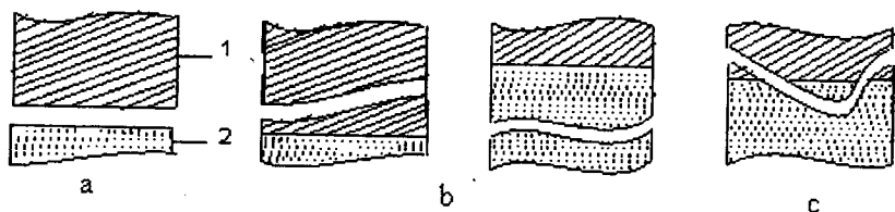
119 – rasm. Adgezion birikmaning emirilish sxemasi: 1 – adgeziv; 2 – substrat; a – adgezion emirilish; b – kogezion emirilish; c – aralash emirilish.
