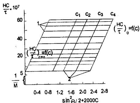
72-rasm. Nur yoyish yordamida olingan natijalarni ekstrapolatsiya qilish uchun qo'llaniladigan B. Zimm diagrammasi. (Sellyuloza nitratining atsetondagi eritmasi), c ni 2000 marta oshirish chizmani chizishni osonlashtirish uchun qilingan. 1 - o'zgarmas \theta larda C = 0 gacha ekstrapolatsiya qilish natijalari; 2 - o'zgarmas c larda \theta = 0 gacha ekstrapolatsiya qilish natijalari.
