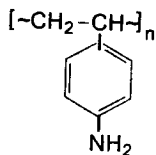
poli-n-aminostirol
