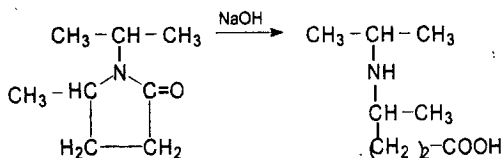
N-izopropil- \gamma - valerolaktam
