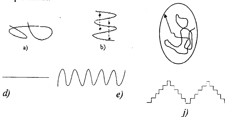
87-rasm. Makromolekulalarning konformatsion turlari: a – statistik g‘ujum; b – spiral (• - o‘zaro vodorod bog‘lari bilan bog‘langan o‘rinbosarlar); c – globula; d – tayoqcha; e – taxlama; j – tirsakli val.
