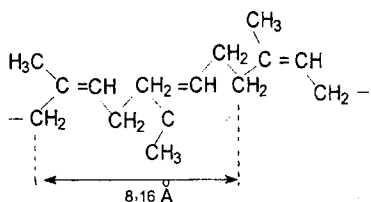
Sis-izomer (kauchuk)
