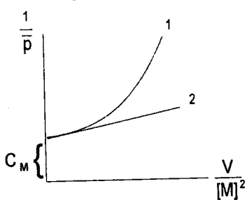
5-rasm. \frac{1}{\bar{P}} - \frac{V}{[M]^2} bog'liklik grafigi; 1 - initsiator zanjir uzatilishda ishtirok etadi; 2 - initsiator zanjir uzatilishda ishtirok etmaydi.
