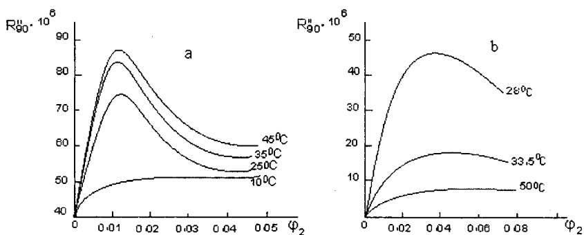
76-rasm. Ortiqcha yorug'lik yoyishning ( R''_{90} ) eritmadagi polimerning hajmiy ulushiga bog'liqligi: a – polistirol yaxshi erituvchi – benzolda; b – polistirol yomon erituvchi – siklogeksanda.
