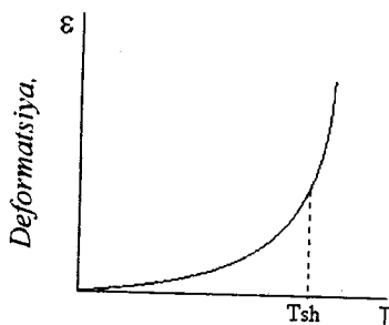
104 – rasm. Quyimolekulyar shishalanuvchi suyuqlikning termomexanik egri chizig'i.
