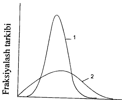
Molekulyar massa 1-rasm. Molekulyar massa bo‘yicha taqsimlanish egrilari
