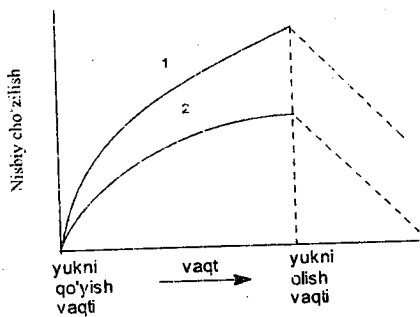
109-rasm. Doiniy kuch taʼsirida polimer namunasi nisbiy uzayishining oʻzgarishi (B-kuch qoʻyilish daqiqasi; A-kuchning olinish vaqti). 1-chiziqsimon polimer; 2-toʻrsimon polimer.
