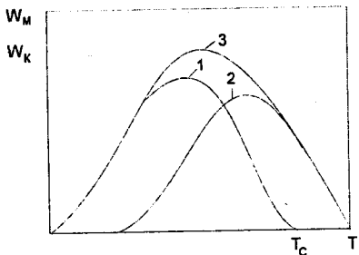
90-rasm. Kristallanish murtagi hosil bo'lish tezligining haroratga bog'liqligi: 1- kristallanish murtaklarining hosil bo'lishi; 2- suyuqlamani o'ta sovutish darajasidan kristallar o'sishi; 3- T_{sh} dan past haroratda murtak hosil bo'lish tezligi.
