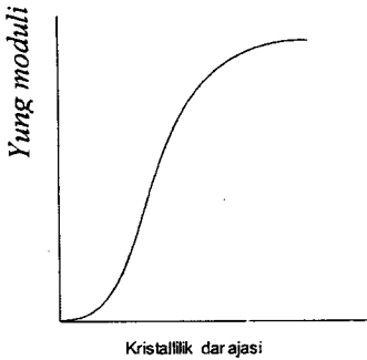
102 – rasm. Yung modulining tabiiy kauchuk namunasi uchun kristallilik darajasiga bog'liqligi.
