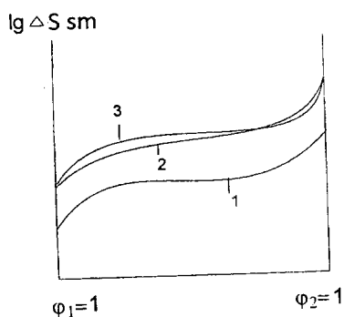
52-rasm. Tabiiy kauchuk-benzol sistemasi uchun aralashis entropiyasining eritma tarki-biga bog'liqligi: 1-ideal aralashish entropiyasi; 2- chin aralashish entropiyasi; 3-nazariy hisoblangan aralashish entropiyasi.
