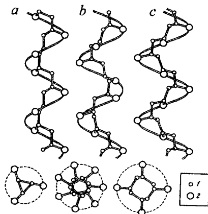
96 - rasm. Izotaktik vinil polimerlarning spiral strukturasi. a - 3_1 -spiral; b - 7_2 -spiral; c - 4_1 -spiral; 1 - asosiy zanjirni hosil qiluvchi uglerod atomlari; 2 - takroriy uglerod atomlariga birikkan R-o'rindosh. Tasvirni soddalashtirish uchun uglerod atomlariga birikkan vodorod atomlari ko'rsatilmagan.
