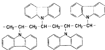
94 - rasm. Polivinilkarbazol strukturasi.
