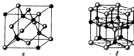
Р и с. 198. Кристаллическая структура с тетраэдро-тетраэдрической координацией атомов:
