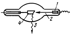
Рис. 86. Схема рентгеновской трубки
