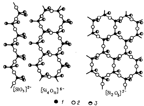
Р и с. 179. Полимерные оксосиликатные ионы:
