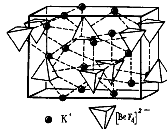
Р и с. 201. Структура \text{K}_2\text{BeF}_4
