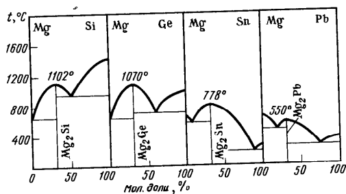
Рис. 180. Диаграмма плавкости систем Mg—Si, Mg—Ge, Mg—Sn, Mg—Pb
