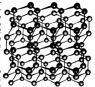
Р и с. 67. Структура льда. Каждая молекула тетраэдрически связана с соседними
