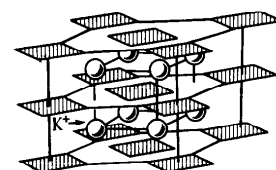
Р и с. 247. Структура \text{K}_2[\text{PtCl}_4]
