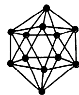
Р и с. 184. Икосаэдрическая группировка атомов \text{B}_{12}
