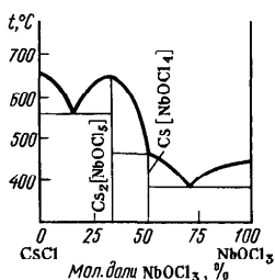
Р и с. 231. Диаграмма плавкости системы \text{CsCl} - \text{NbOCl}_3
