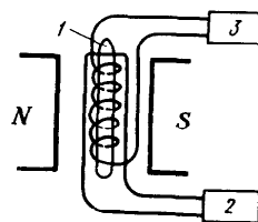
Рис. 94. Схема радиоспектроскопа для исследования ЯМР:
