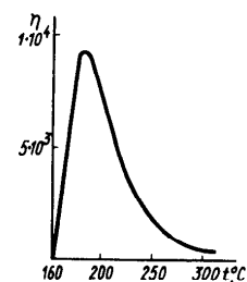
Р и с. 154. Изменение относительной вязкости жидкой серы ( \eta = 1 при 100°C) при повышении температуры
