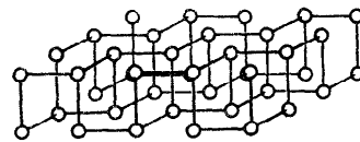
Рис. 164. Расположение атомов в кристалле черного фосфора
