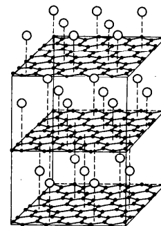
Р и с. 175. Структура фторида графита CF
