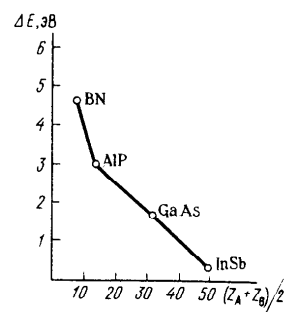
Р и с. 199. Зависимость ширины запрещенной зоны \Delta E в соединениях типа A^{III}B^V от среднего атомного номера
