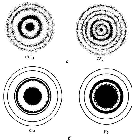
Р и с. 105. Электронограммы: а – газов; б – кристаллов
