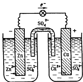
Р и с. 122. Схема гальванического элемента
