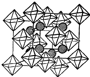
Рис. 68. Кристаллическая решетка соединений типа: \text{M}_2^+[\text{Э}(\text{Hal})_6] или [\text{M}^+(\text{NH}_3)_6]\text{X}_2 :
