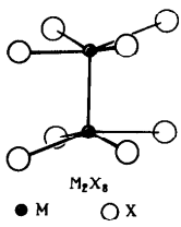
Рис. 235. Структура двухъядерного кластера типа M_2X_8 на примере K_2[Re_2Cl_8] \cdot 2H_2O
