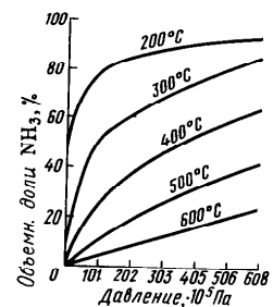
Рис. 159. Равновесная концентрация аммиака в азотоводородной смеси ( 3\text{H}_2 + \text{N}_2 ) как функция давления и температуры
