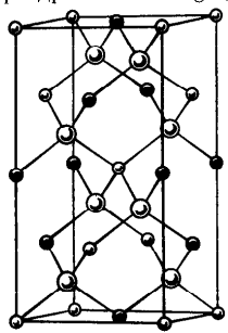
Рис. 135. Кристаллическая решетка халькопирита \text{CuFeS}_2
