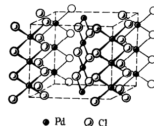
Р и с. 245. Структура PdCl 2
