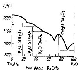
Р и с. 229. Диаграмма плавкости системы \text{Ta}_2\text{O}_5 - \text{K}_2\text{O}
