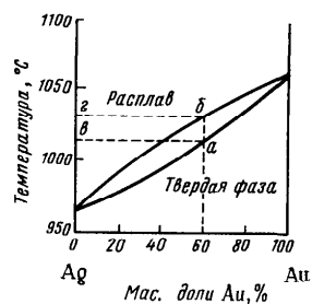
Р и с. 83. Диаграмма плавкости твердого раствора
