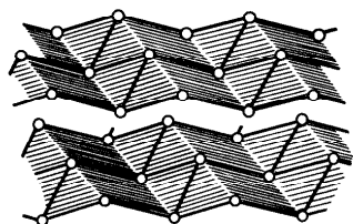
Рис. 169. Слоистая структура мышьяка, сурьмы, висмута
