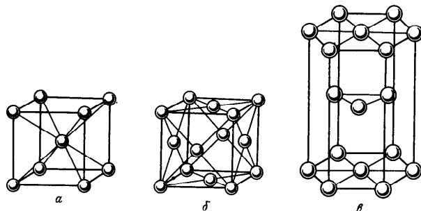
Р и с. 125. Кристаллические решетки металлов:
