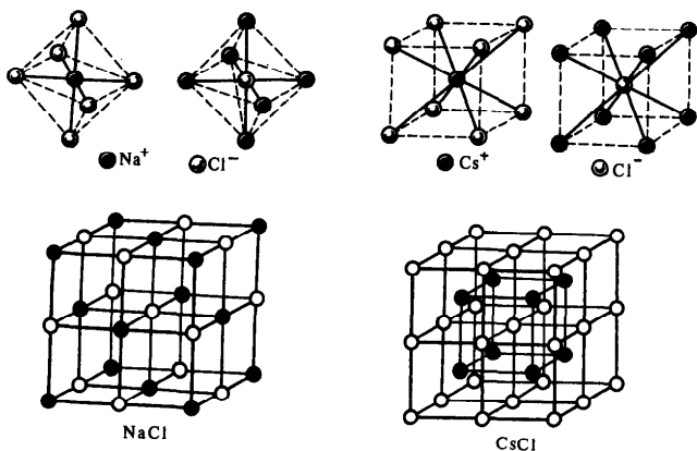
Р и с. 57. Структурный тип хлорида натрия NaCl
