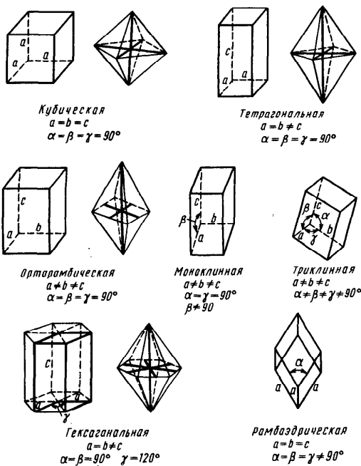
Р и с. 64. Основные системы кристаллов
