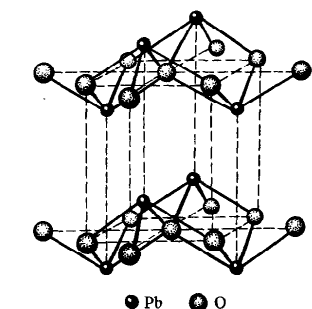
Р и с. 183. Структура PbO
