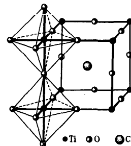
Рис. 70. Структура перовскита CaTiO_3
