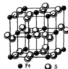
Р и с. 155. Кристаллическая решетка пирита FeS_2
