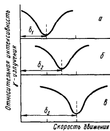
Р и с. 98. \gamma -Резонансный спектр поглощения SnI_4 (а), SnBr_4 (б) и SnCl_4 (в). Источник излучения ^{119}Sn в SnO_2
