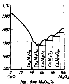
Р и с. 192. Диаграмма плавокости системы CaO – Al 2 O 3
