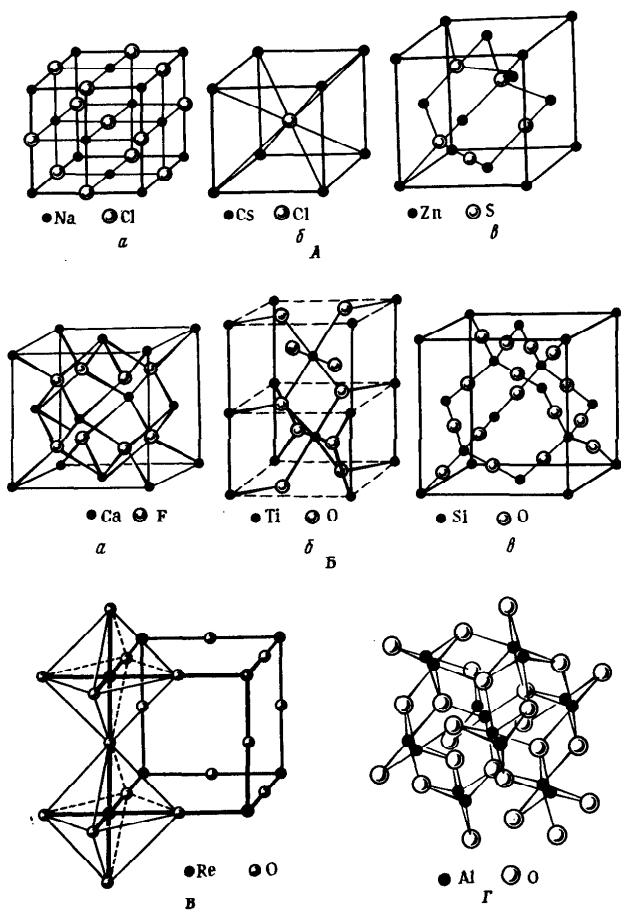
Р и с. 69. Важнейшие типы координационных решеток кристаллов: А – состав АВ, структурный тип: а – NaCl; б – CsCl; в – ZnS (сфалерит); Б – состава АВ 2 , структурный тип: а – CaF 2 (флюорит); б – TiO 2 (рутил); в – SiO 2 (кristобалит); В – состава АВ 3 , структурный тип ReO 3 ; Г – состава А 2 В 3 , структурный тип α-Al 2 O 3 (корунд)
