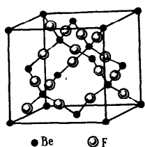
Рис. 60. Структура кристалла фторида бериллия \text{BeF}_2
