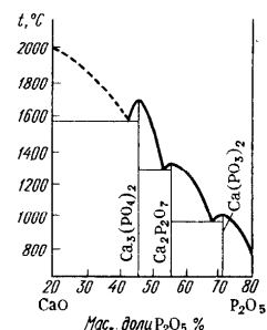
Р и с. 167. Диаграмма плавления системы CaO - P_2O_5
