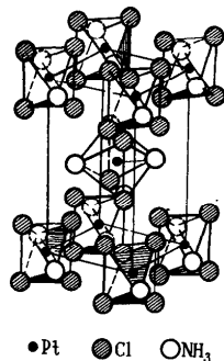
Рис. 249. Строение кристалла [\text{Pt}(\text{NH}_3)_2\text{Cl}_4]
