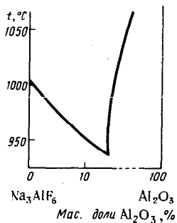
Рис. 190. Фрагмент диаграммы плавкости системы \text{Na}_3\text{AlF}_6 - \text{Al}_2\text{O}_3
