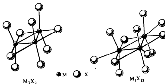
Рис. 234. Структура треугольных кластеров со связью металл–металл типа M_3X_9 и типа M_3X_{12}
