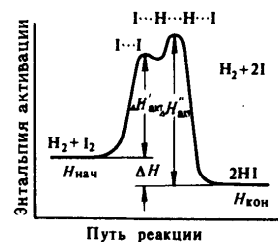
Р и с. 118. Энергетическая схема хода реакции \text{H}_2(\text{r}) + \text{I}_2(\text{r})
