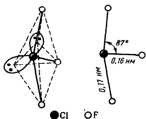
Р и с. 146. Строение молекулы \text{ClF}_3
