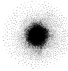
Рис. 2. Электронное облако
