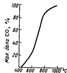
Рис. 177. Влияние температуры на состояние равновесия CO_2(g) + C(s) \rightleftharpoons 2CO(g)
