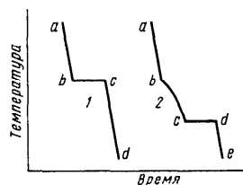
Рис. 78. Кривые охлаждения:
