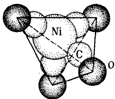
Рис. 242. Строение молекулы тетракарбонила никеля Ni(CO) 4
