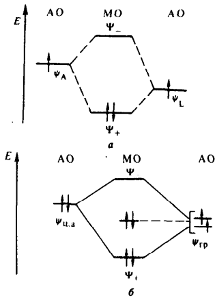
Р и с. 145. Энергетическая диаграмма орбиталей для двухэлектронного двухэлектронного (а) и трехэлектронного четырехэлектронного взаимодействия (б)
