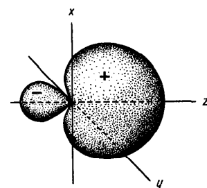
Р и с. 47. Форма sp -гибридной орбитали
