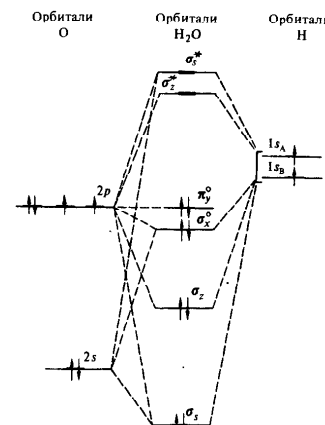
Рис. 151. Энергетическая диаграмма орбиталей молекулы H_2O
