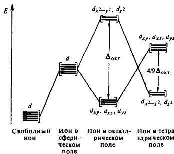
Р и с. 212. Расщепление d -уровня кристаллическим полем разной симметрии
