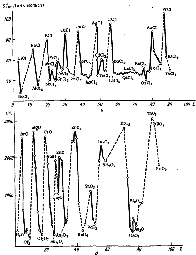
Р и с. 131. Зависимость свойств бинарных соединений от атомного номера элемента с положительной степенью окисления: а — стандартной энтропии кристаллических хлоридов; б — температуры плавления оксидов; в — энтальпии образования хлоридов; г — энергии Гиббса образования хлоридов
