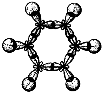
Рис. 52. \sigma -Связи в молекуле бензола
