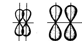
Р и с. 147. Влияние межъядерного расстояния на степень перекрывания p-p -связей
