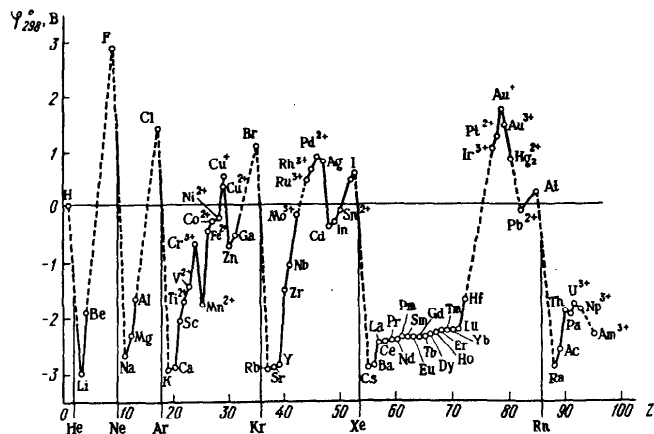
Рис. 129. Зависимость стандартных электродных потенциалов простых веществ в водном растворе от атомного номера элемента и окислителем, и восстановителем, а также выступает в качестве лиганда в процессах комплексообразования (гидратации ионов).
