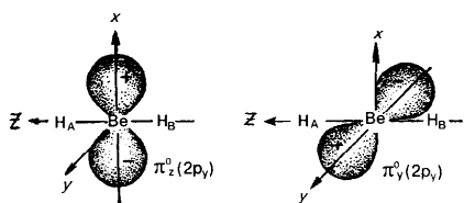
Р и с. 36. Несвязывающие \pi^o -орбитали молекулы \text{BeH}_2
