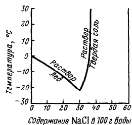
Р и с. 80. Диаграмма плавкости системы H_2O - NaCl
