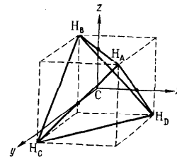
Р и с. 42. Взаимное расположение атомов в молекуле \text{CH}_4 (рис. 43, а) приводит к образованию пятицентровых молекулярных \sigma_s - и \sigma_s^* -орбиталей.
