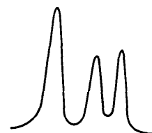
Рис. 95. Спектр ЯМР (протонов) этанола \text{C}_2\text{H}_5\text{OH}
