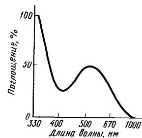
Р и с. 223. Спектр поглощения комплекса [Ti(OH_2)_6]^{3+}
