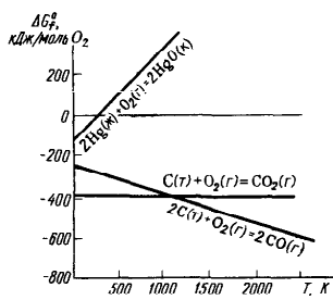
Рис. 113. Зависимость \Delta G_f^0 ряда оксидов от температуры
