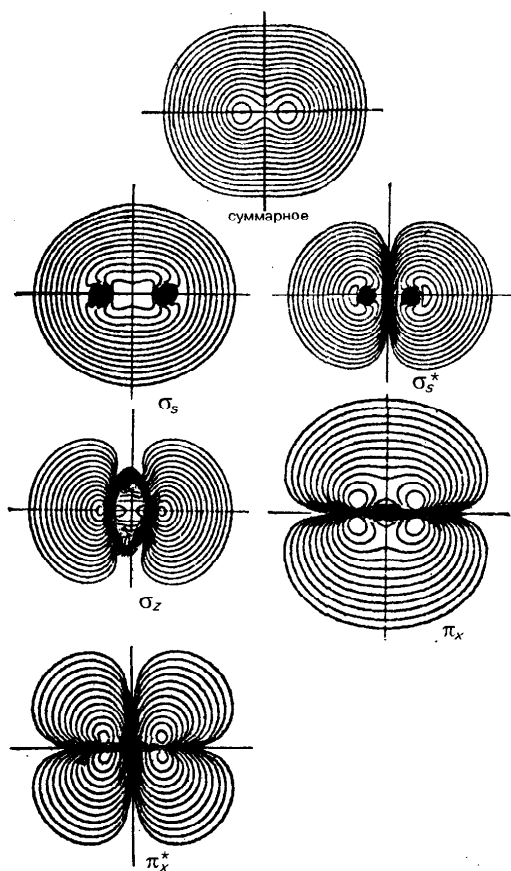
Р и с. 29. Распределение электронной плотности в молекуле O_2 по орбитали \sigma_s и \sigma_s^* , \sigma_z , \pi_x и \pi_x^*
