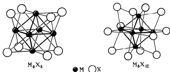
Рис. 233. Структура октаэдрических кластеров типа M_6X_8 на примере иона [Mo_6Cl_8]^{4+} и типа M_6X_{12} на примере иона [Nb_6Cl_{12}]^{4+}
