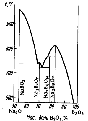
Р и с. 189. Диаграмма плавкости системы Na_2O - B_2O_3
