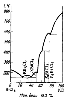
Рис. 170. Диаграмма плавления системы \text{BiCl}_3 — \text{KCl}
