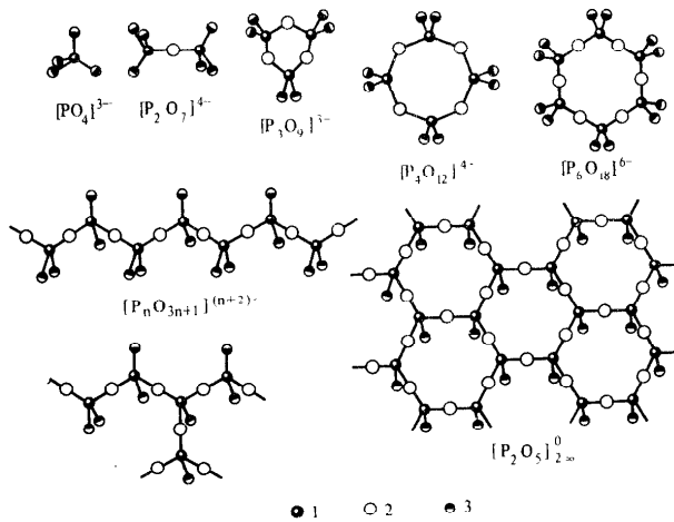
Р и с. 166. Структура оксофосфат (V)-ионов и слоистой модификации P_2O_5 :
