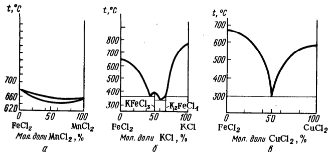
Рис. 136. Диаграммы плавкости систем:
