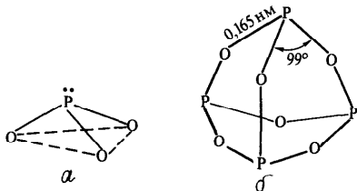
Рис. 165. Пирамидальная структурная единица (а) и строение молекулы \text{P}_4\text{O}_6 (б)
