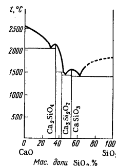
Рис. 178. Диаграмма плавления системы CaO - SiO_2
