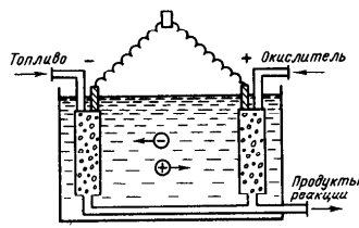
Р и с. 123. Схема топливного элемента
