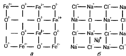
Р и с. 138. Катионный дефект в кристалле \text{FeO} (а) и анионный дефект в кристалле \text{NaCl} , легированном натрием (б)
