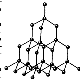
Р и с. 65. Структура алмаза
