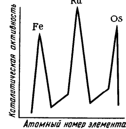
Рис. 160. Зависимость каталитической активности ряда металлов в реакции 2\text{NH}_3 = \text{N}_2 + 3\text{H}_2 ( 800^\circ\text{C}, 1 \cdot 10^5 Па) от атомного номера элемента
