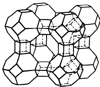
Р и с. 193. Структура цеолита
