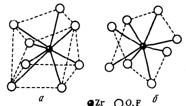
Рис. 227. Взаимное расположение атомов ZrO 2 с примесью HfO 2 в восьмивершинниках оксо- (а) и названных фланитали. Послед- фторпроизводных (б)
