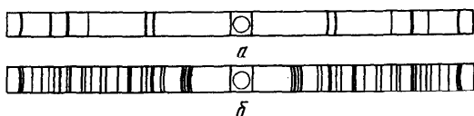
Р и с. 101. Рентгенограммы: а — алмаз; б — графит
