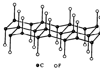
Р и с. 175. Структура фторида графита CF
