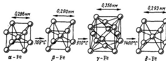
Рис. 239. Полиморфные превращения железа
