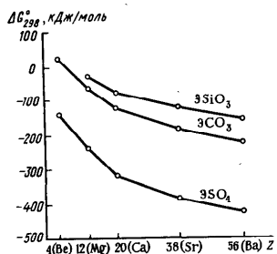
Р и с. 204. Зависимость \Delta G_{298}^{\circ} реакции образования 3\text{SiO}_3 , 3\text{CO}_3 и 3\text{SO}_4 из оксидов ЭО от атомного номера
