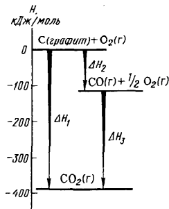
Рис. 109. Энтальпийная диаграмма окисления графита
