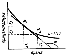
Рис. 114. Изменение концентрации исходных веществ в процессе реакции
