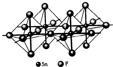
Рис. 182. Структура \text{SnF}_4
