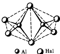
Рис. 194. Строение молекулы Al_2Hal_6
