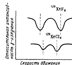
Р и с. 99. \gamma -Резонансные спектры молекул XeCl_4 и XeF_4
