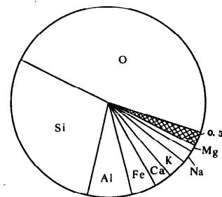
Рис. 124. Распространение химических элементов в земной коре
