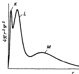
Рис. 11. Распределение электронной плотности в атоме аргона
