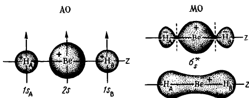
Р и с. 34. Схема образования \sigma_s -связывающей и \sigma_s^* -разрыхляющей орбиталей молекулы \text{BeH}_2
