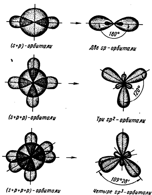
Р и с. 48. Гибридизация валентных орбиталей
