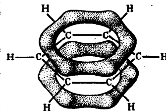
Рис. 54. \pi -Связи в молекуле бензола
