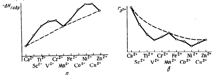
Рис. 215. Изменение энтальпии гидратации (а) и радиусов двухзарядных ионов (б) в ряду \text{Ca}^{2+}-\text{Zn}^{2+}
