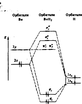
Р и с. 37. Энергетическая диаграмма орбиталей линейной трехатомной молекулы без \pi -связывания на примере \text{BeH}_2
