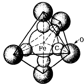
Рис. 240. Структура молекулы пентакарбонила железа \text{Fe}(\text{CO})_5
