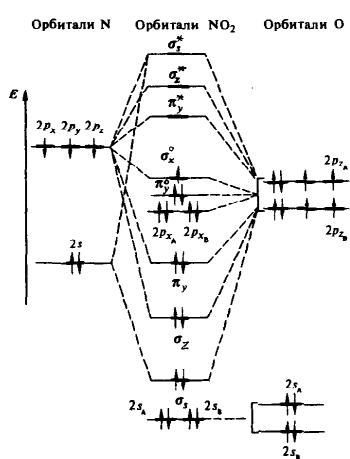
Рис. 163. Энергетическая диаграмма орбиталей молекулы NO 2 и делокализованной \pi -связи ( \pi_y -орбиталь).
