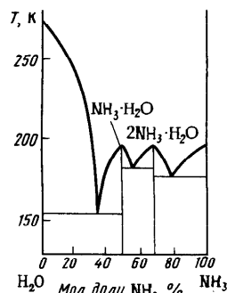
Рис. 158. Диаграмма состояния системы \text{H}_2\text{O} - \text{NH}_3
