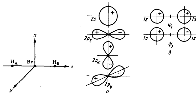
Р и с. 32. Взаимное расположение атомов в молекуле BeH 2
