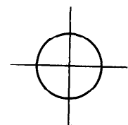
Рис. 3. Сечение граничной поверхности
