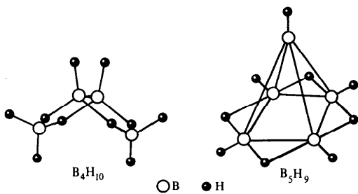
Р и с. 187. Структура тетраборана B_4H_{10} и пентаборана B_5H_9
