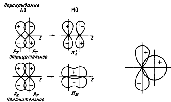
Р и с. 25. Схема образования из p_x -атомных орбиталей связывающей \pi_g и разрыхляющей \pi_g^* молекулярных орбиталей двухатомной гомоядерной молекулы
