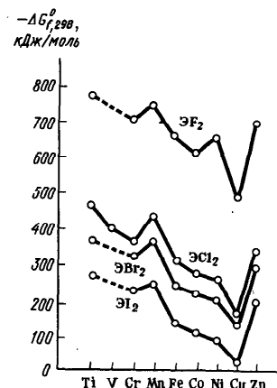
Рис. 150. Энергия Гиббса образования дигалогенидов 3d-элементов
