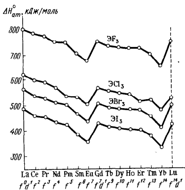
Р и с. 254. Зависимость энthalпии атомизации тригалогенидов лантаноидов от атомного номера лантаноидов
