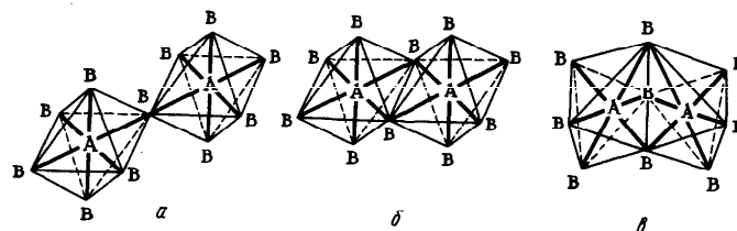
Рис. 61. Двухъядерные комплексы:
