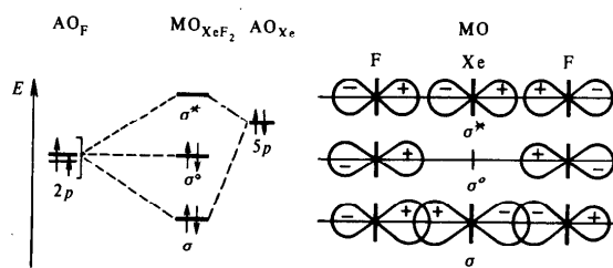
Р и с. 208. Трехцентровые орбитали молекулы XeF 2
