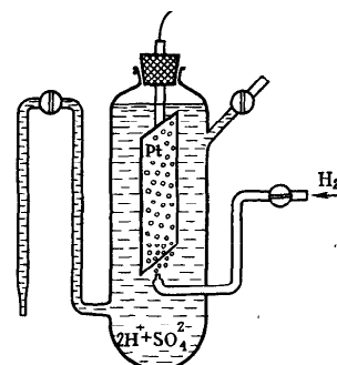
Рис. 121. Схема водородного электрода
