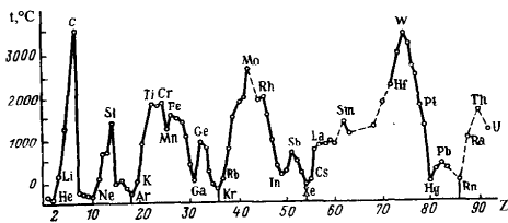
Р и с. 127. Зависимость температуры плавления простых веществ от атомного номера элемента
