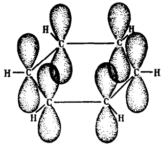
Рис. 53. Расположение p -электронных облаков в молекуле бензола
