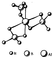
Р и с. 197. Структура \text{Al}(\text{BH}_4)_3
