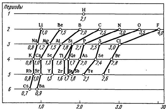
Рис. 13. Шкала электроотрицательностей по Полингу
