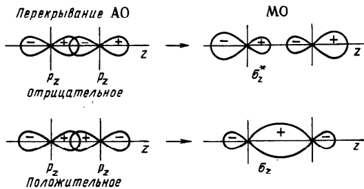
Р и с. 24. Схема образования из p_z -атомных орбиталей связывающей \sigma_g и разрыхляющей \sigma_g^* орбиталей двухатомной гомоядерной молекулы
