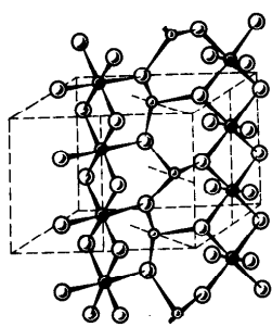
Р и с. 181. Структура сурика \text{Pb}_3\text{O}_4 ( \text{Pb}_2\text{PbO}_4 )
