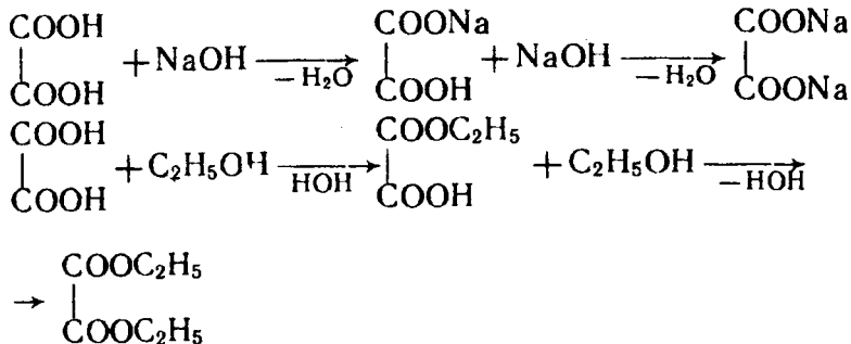
nordon tuz
