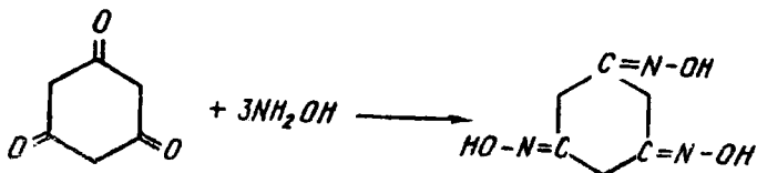
siklogeksantrioksim
