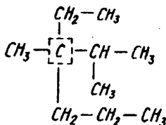
Metan
