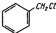
benzilxlorib
