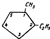
1-metil-2-etil siklopentan
