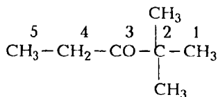
etiluchlamchibutiketon, 2,2-dimetilpentanon-3
