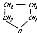
tetragidrofuran
