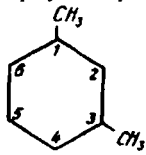
1,3-dimetil-siklogeksan
