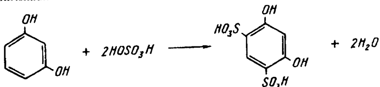
1,3-dioksi-4-6-disulfobenzol
