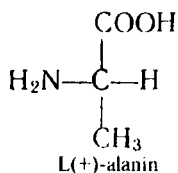
9-rasm. Optik izomerlar – antipodlar.
