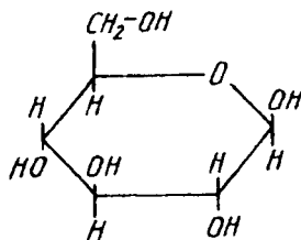
\beta - D -glukoza ( \beta - D -glukonopiranza)
