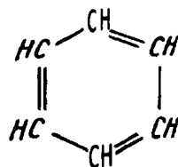
benzol
