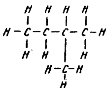
izopentan
