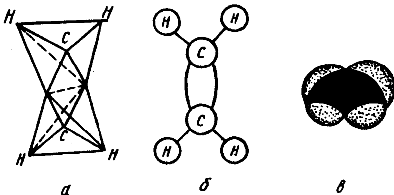
4-rasm. Etilen molekulasining fazoviy modellari: a-tetraedr shaklida, b-shár-sterjen ko'rinishida, v-Styuart-Brigleb modeli bo'yicha ko'rinishi.
