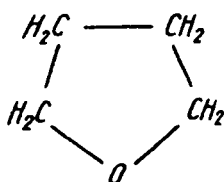
tetragidrofuran
