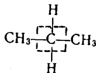
dimetilmetan
