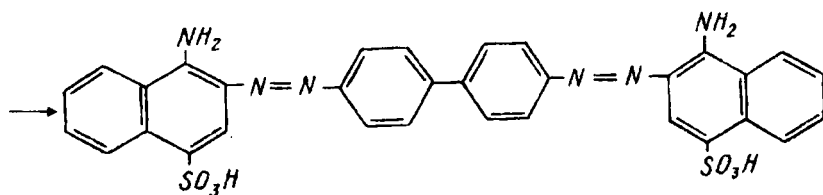
kongo qizil
