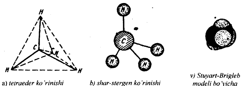
1-rasm. Metan molekulasining fazoviy tuzilish modeli
