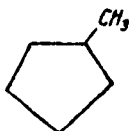
metilsiklopentan
