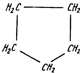
siklopentan
