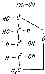
\beta - D -fruktoza (piranoz ko'rinishi)
