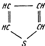
tiofen
