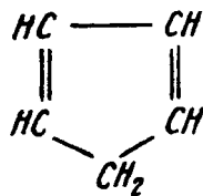
siklopentadien
