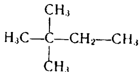
2,2 – dimetilbutan
