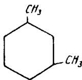
1,3 dimetilsiklogeksan
