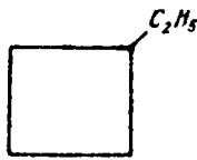
etilsiklobutan
