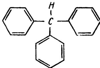
triphenilmetan
