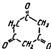
keton
