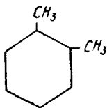
1,2-dimetilsiklogeksan
