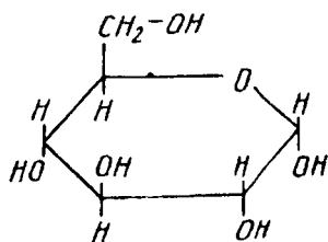
\alpha - D -glukoza ( \alpha - D -glukonopiranza)
