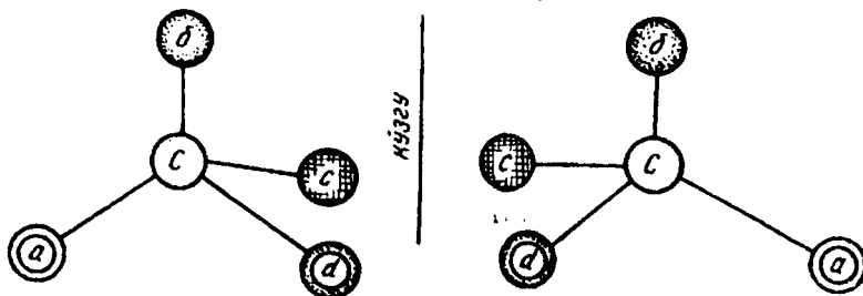
9-rasm. Optik izomerlar – antipodlar.
