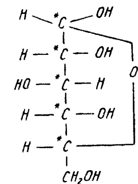
\alpha -D-glukoza ( \alpha -D-glukonopiranoza)
