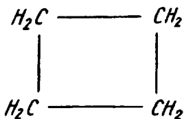
siklobutan
