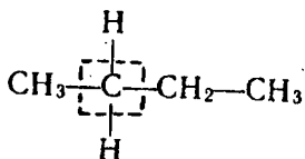
metiletilmetan
