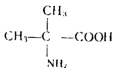
2-amino - 2-metilpropan kislota
