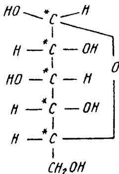
\beta -D-glukoza ( \beta -D-glukonopiranoza)
