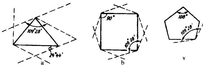
10-rasm. Bayer gipotezasiga ko`ra turli uglevodorodlarning fazoviy modellari:
