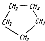
pentametilen (P) siklopantan (C)
