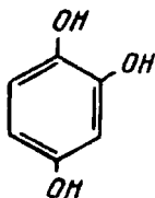
oksigidroxinon
