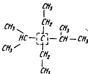
Dietildiizopropilmetan
