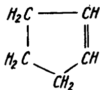
siklopenten
