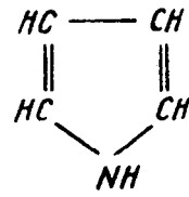
pirrol
