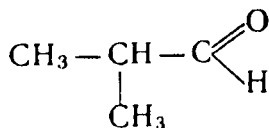
izomoy aldegidi 2-metilpropanal
