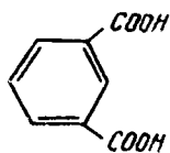
izoftal kislota
