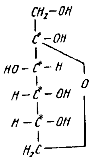
\alpha - D -fruktoza (piranoz ko'rinishi)
