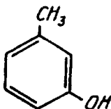
m- krezol
