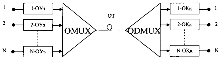
4.9-расм. Оптик сигналлар сатҳидаги вақт бўйича мультиплексорлаш.
