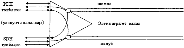
в) ички коммутациялаш режимидаги кириш/чиқишли мультимплексор
