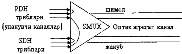
в) ички коммутациялаш режимидаги кириш/чиқишли мультимплексор
