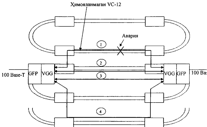
7.5-расм. LCAS технологиясини қўллаган ҳолда Ethernet трафигини ҳимоялашни ташкиллаштиришга мисол.
