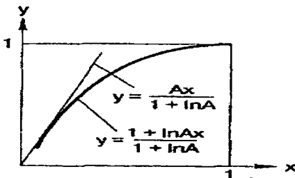
3.6-расм. Компандерлашнинг логарифмик А қонуни.
