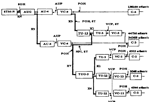
5.7-расм. Триб сигналларидан N-сатҳдаги синхрон транспорт модулининг шаклланиши.
