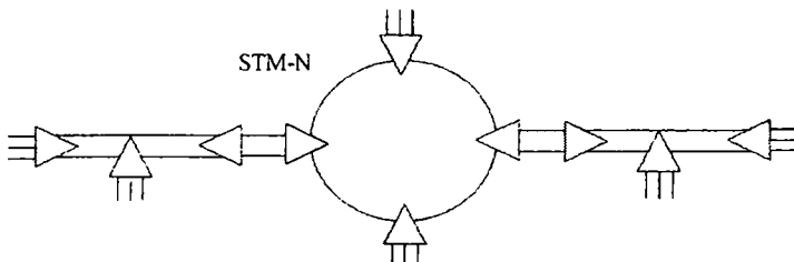
5.16-расм. Нуқта-нуқта ва ҳалқали SDH тармоғи.
