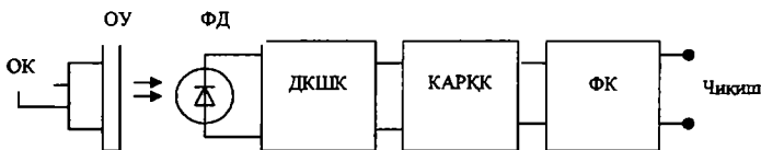
4.11-расм. Оптик қабул қилгичнинг умумий тузилиш схемаси.
