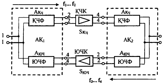
1.30-расм. Юқори ва қуйи частотали йўналтирувчи филтрларга эга икки томонлама икки полосали каналнинг барқарорлиги.
