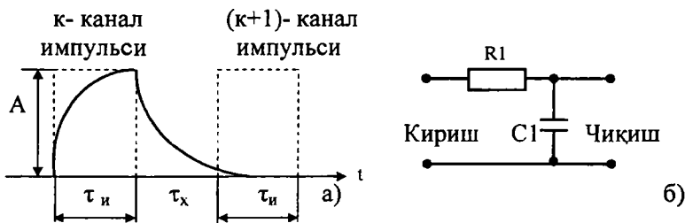
2.19-расм. Гуруҳли сигналнинг бузилмаган ва бузилган импульслари (а); гуруҳли узатиш трактининг юқори частоталар соҳасидаги эквивалент схемаси (б).
