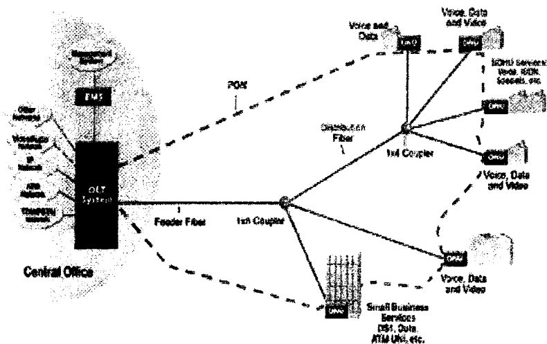
8.15-расм. Пассив тармоқлагичлар орқали охириги миждозларга уланиш
