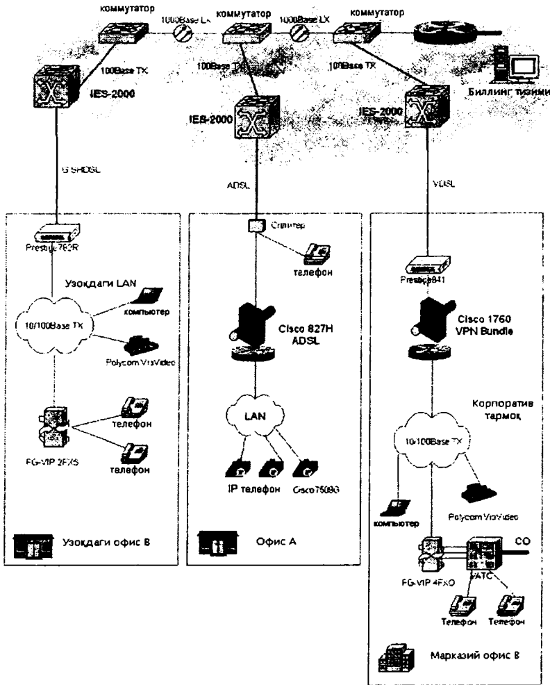
7.3-расм. Тақсимланган мультисервиси тармоқларни ташкил этиш схемаси.
