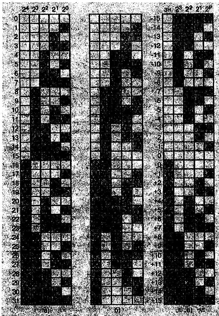
3.9-расм. Иккилик кодларнинг код жадваллари: а-натурал иккилик код; б- Грейнинг рефлекс иккилик коди; в-симметрик иккилик код.
