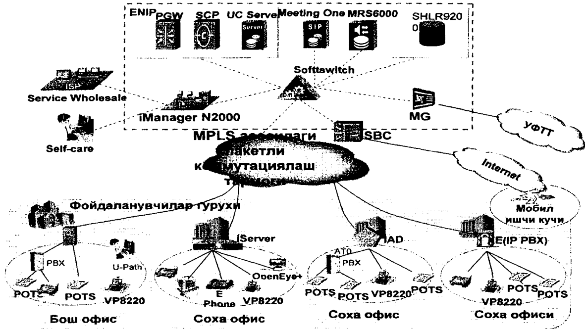
7.16-расм. MPLS технологиясига асосланган корпоратив тармокнинг NGN га уланиши
