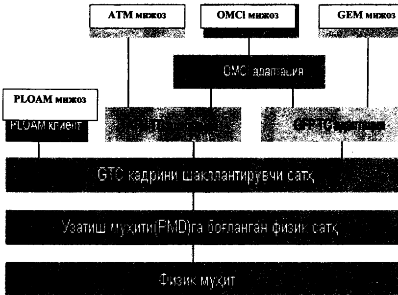
8.23-расм. GPON сатҳларини структураси.
