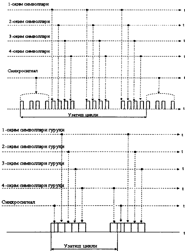
3.23-расм. Рақамли оқимлар символ бўйича (а) ва канал бўйича (б) бирлашаётган рақамли узатиш тизими циклининг тузилиши.
