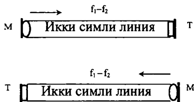
1.18-расм. Икки томонлама телефон алоқани ташкил қилишнинг бир полосали тўрт симли схемаси.
