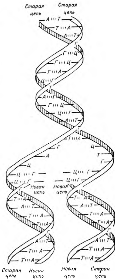
Рис. 2. Модель строения дезоксирибонуклеиновой кислоты (ДНК).
