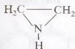
aziridin (azairidin) etilenimin
