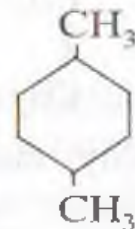
1,2-dimetilsiklogeksan 1,3-dimetilsiklogeksan 1,4-dimetilsiklogeksan
