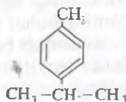
1-metil-4-izopropil benzol, simol
