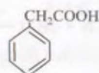
fenil sirka kislota
