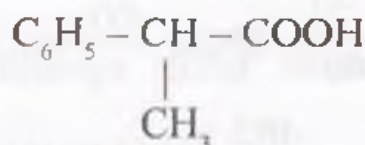
metilfenil sirka kislota; 2-fenilpropan kislota
