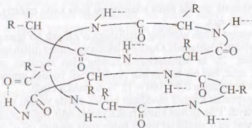
Oqsil molekulasining ikkilamchi tuzilishi.
