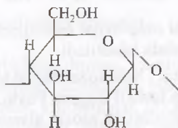
Selluloza zvenosining tuzilishi
