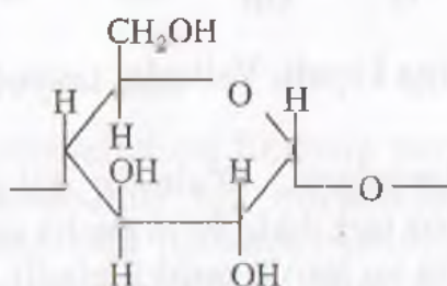
Kraxmal elementlar zvenosining tuzilishi
