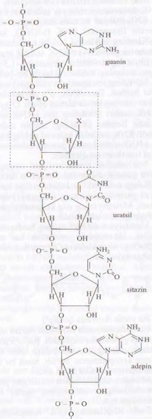
RNK zanjiri eruvchi qismining tuzilishi
