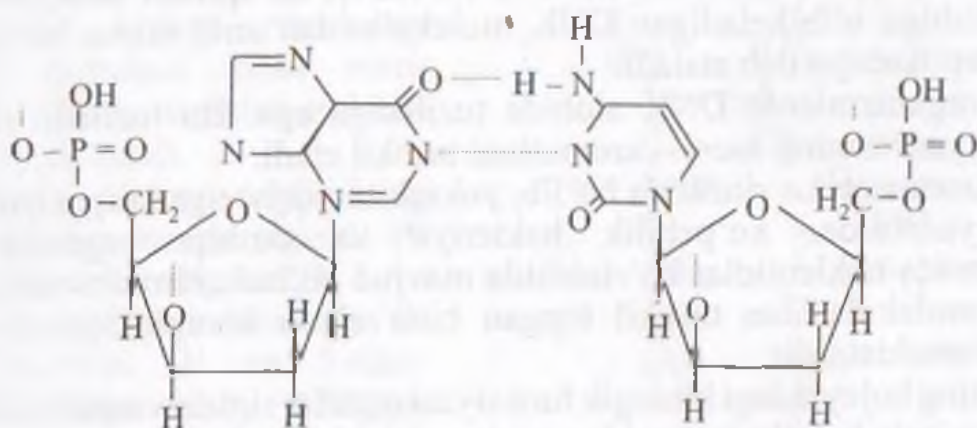
I Nukleotid zanjiri
