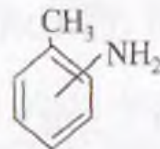
o-, m- va p-aminotoluollar
