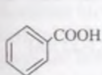
benzoy kislota benzen karbon kislota
