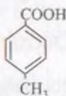
n-toluil kislota n-toluen karbon kislota
