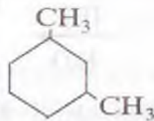
1,2-dimetilsiklogeksan 1,3-dimetilsiklogeksan 1,4-dimetilsiklogeksan
