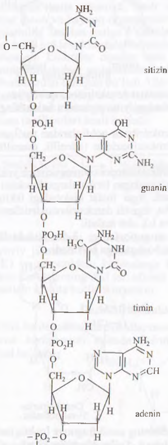
DNK zanjirining bir qismi
