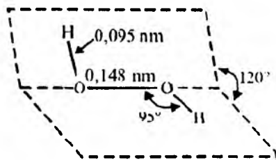
34-rasm. Vodorod peroksid molekulasiining tuzilishi.
