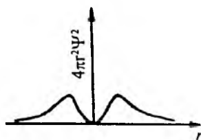
10-rasm. 2p- elektronlarning radial taqsimlanish ehtimolligini ko'rsatuvchi egri chiziqlar.
