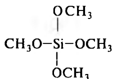
ortokremniy kislotasining tetrametil efiri
