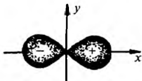
11-rasm. 2p- elektron bulutning ko'rinishi.
