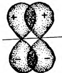
14-rasm. \pi -bog' hosil bo'lishida elektron bulutlarining qoplanishi.
