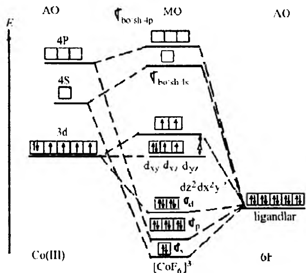
27 rasm. Molekular orbitalar usulida past spinli [Co(NH_3)_6]^{3+} va yuqori spinli [CoF_6]^{3-} komplekslarining energetik diagrammalari tuzilishi.
