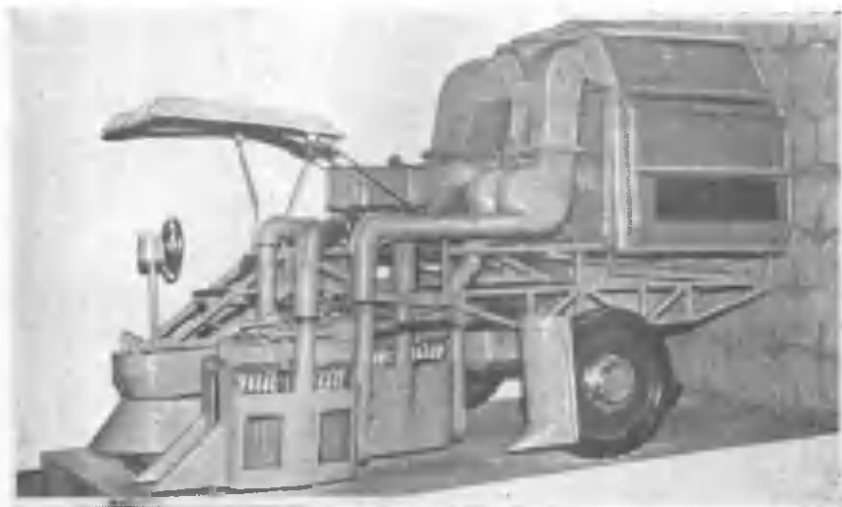
ХВС-1,2 пахта териш машинасининг ҳаракатланувчи модели.
