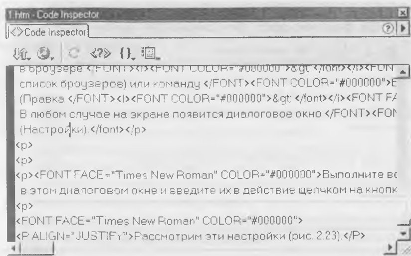
2.3-rasm. Hujjatning belgili rejimida ko'rinishi.
