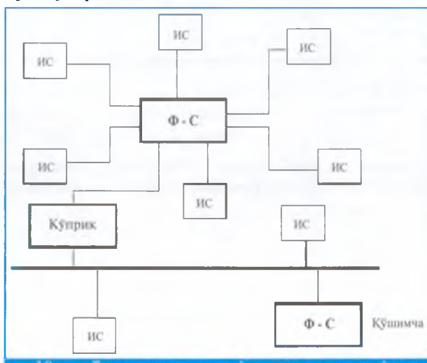
3.9-расм. Тармоқларнинг жисмоний имкониятларини кенгайтириш
