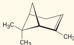
α-Pinene (turpentine)
