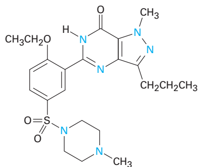
Sildenafil (Viagra)
