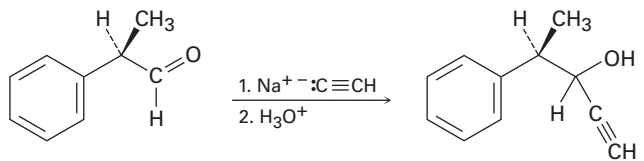
( R )-2-Phenylpropanal
