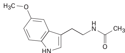
Melatonin
