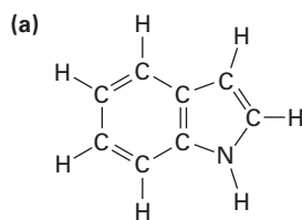
Indole
