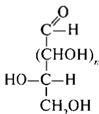
L-monosaxarid
