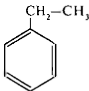
etilbenzol
