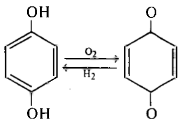
gidroxinon
