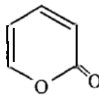
\alpha - piron
