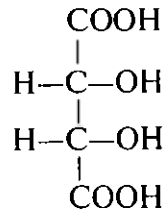
mezovino kislotasi
