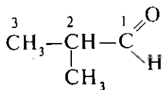
2-metilpropanal
