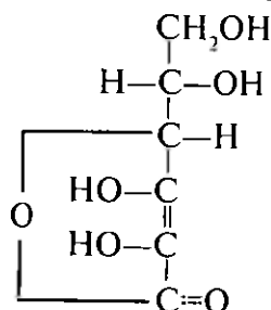
askorbin kislota
