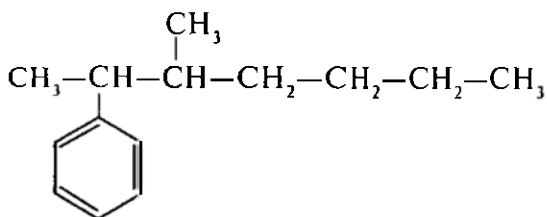
2-fenil-3-metilgeptan
