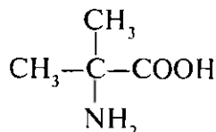
2-amino-2-metilpropan kislota
