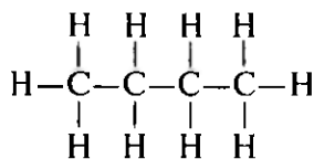
butan
