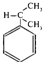
izopropilbenzol
