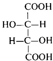
L(-)-vino kislotasi
