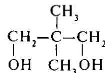
2,2-dimetilpropandiol-1,3
