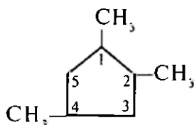
1,2,4-trimetilsiklopentan
