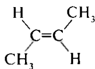
trans-2-buten
