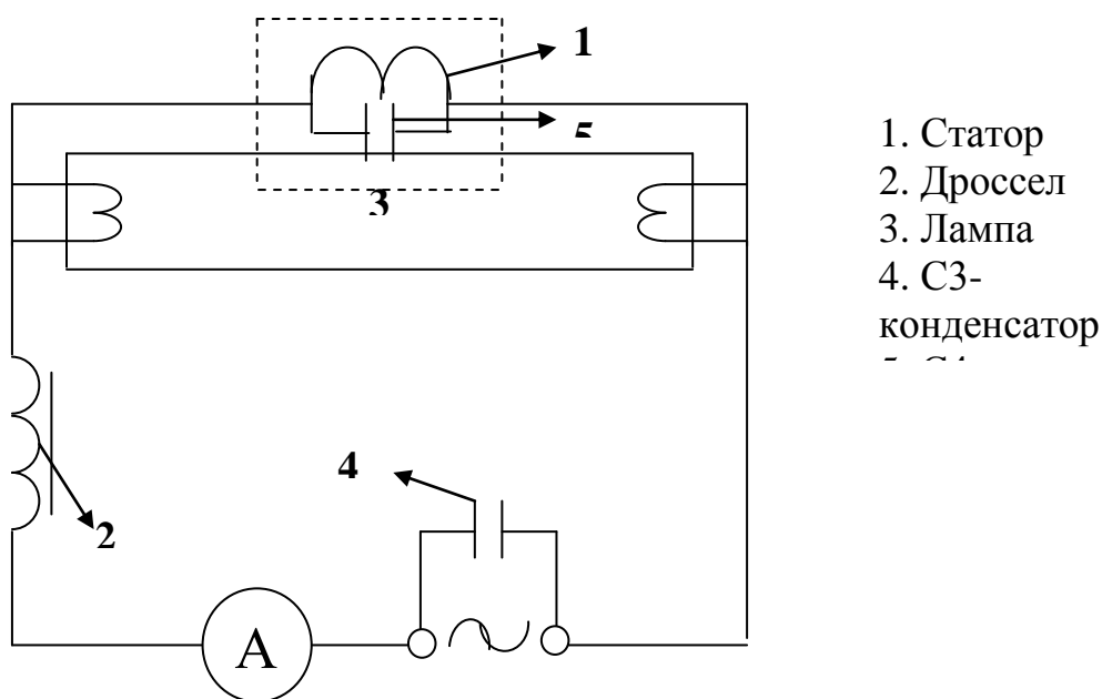
Рис 1.2 Статорное зажигание люминесцентных ламп.
