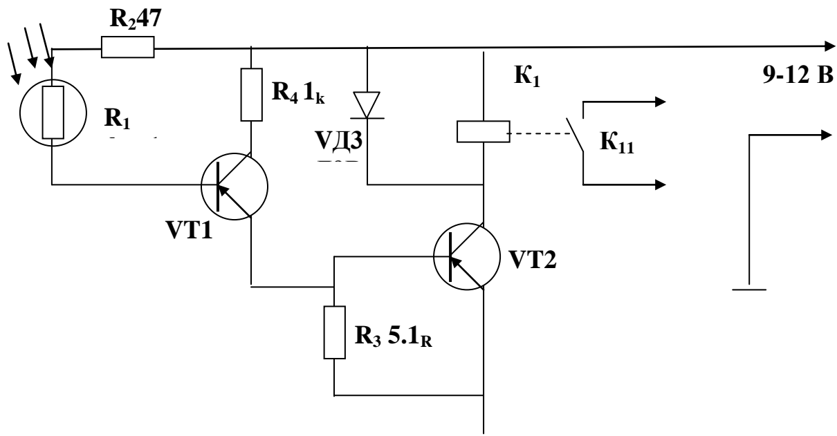
Рис. 3.3 Фоторезисторный фотореле.
