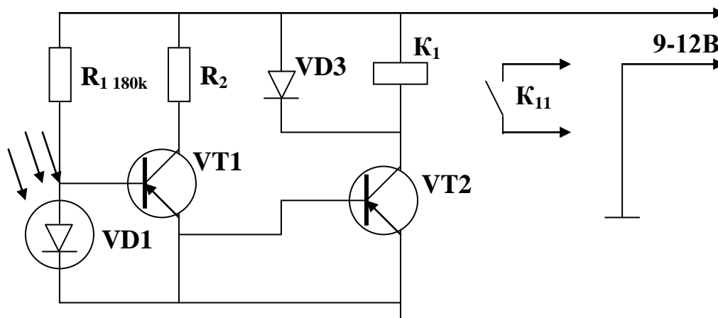
Рис. 2.4 Фотодиодное фотореле
