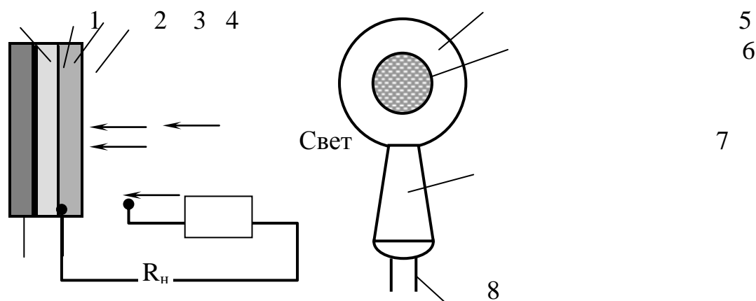
Фотоэлемент с запирающим слоем.
