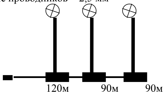
Рис. 5.18. Расчет питающей и групповой сети на минимум проводникового материала
