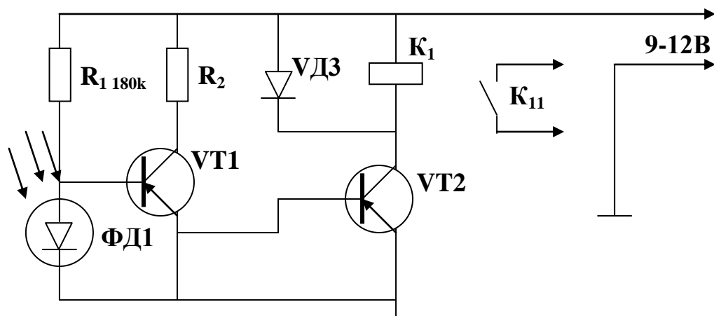
Рис. 3.4 Фотодиодный фотореле
