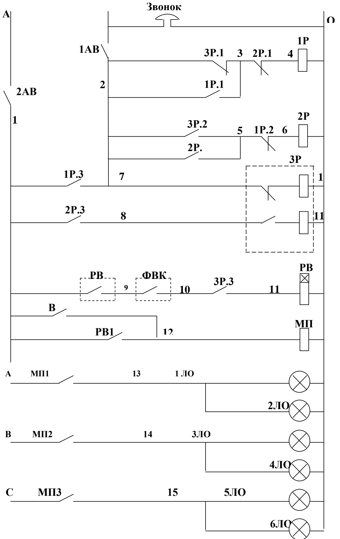
Рис.3.1. Схема автоматического программного управления освещением реакций и коридоров в школах.
