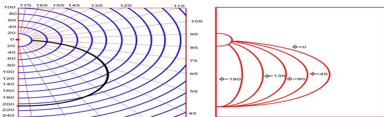
Продольная кривая распределения силы
