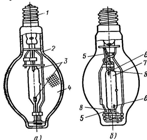
Рис.11.1 Газоразрядные лампы типа ДРЛ а - двух электродная, б - четырех электродная 1-цоколь, 2-внешний баллон, 3-электрод, 4-люминофор, 5-сопротивление, 6-основной электрод, 7-кварцевая горелка, 8-дополнительный электрод.
