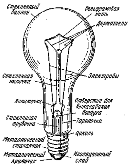
Рис.1.1. Элементы ламп накаливания.
