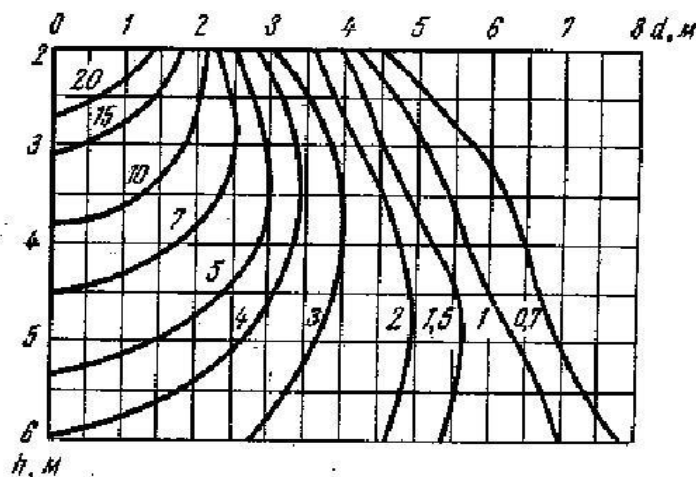
Рис. 4.3. Пространственные изолюксы условной горизонтальной освещенности от «Люцетты» цельного стекла
