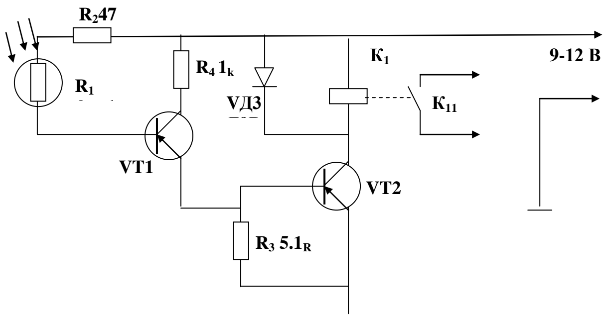
Рис. 2.3 Фоторезисторное фотореле.
