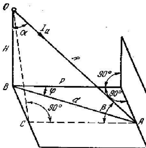
Рис. 17-4. Схема к расчету освещенности точки в вертикальной плоскости.
