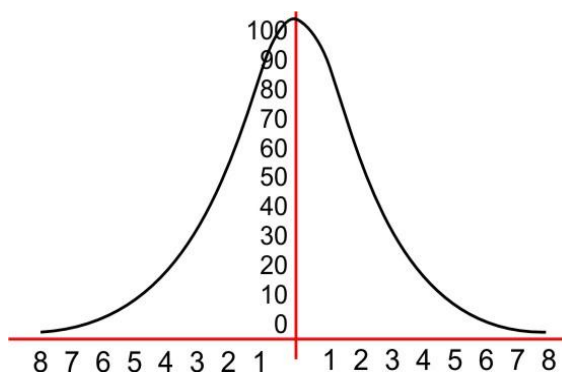
Кривая распределения силы света в прямоугольных координатах (прожекторы и светосигнальные приборы).
