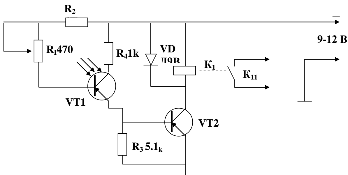
Рис.2.2 Фототранзисторное фотореле
