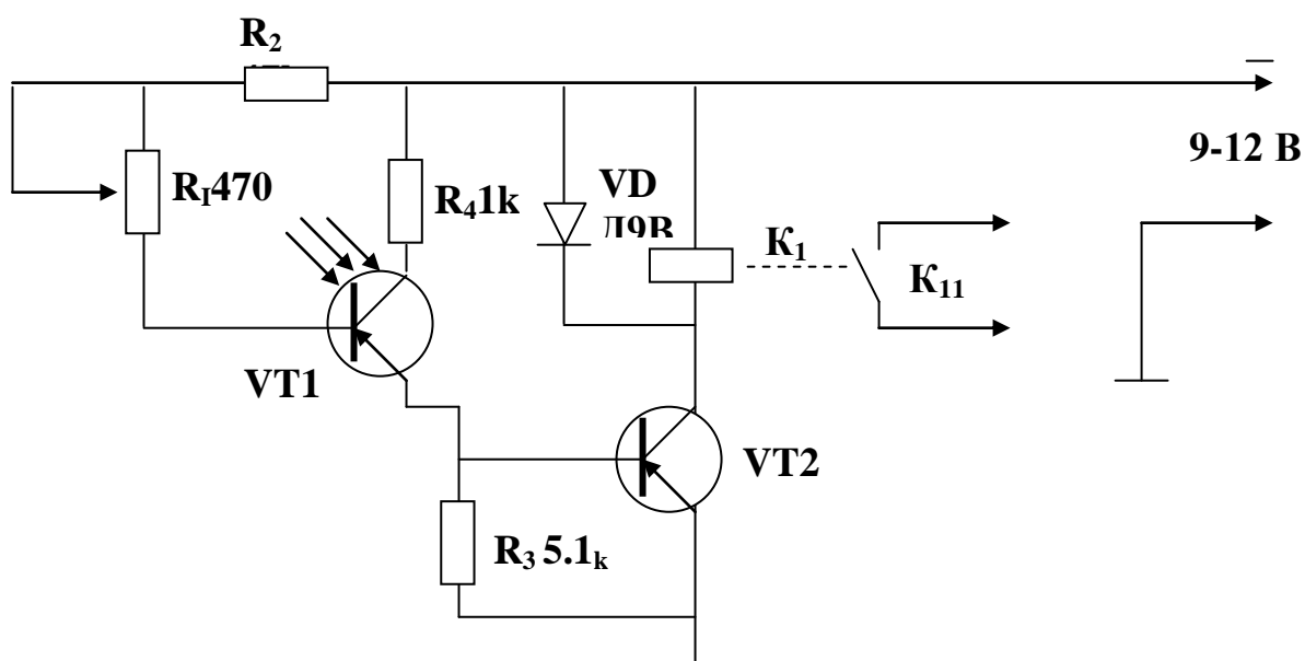
Рис.2.2 Фототранзисторное фотореле
