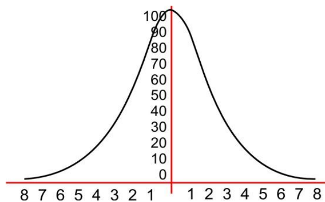
Кривая распределения силы света в прямоугольных координатах (прожекторы и светосигнальные приборы).
