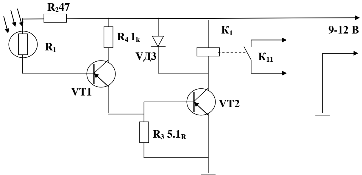
Рис. 3.3 Фоторезисторный фотореле.
