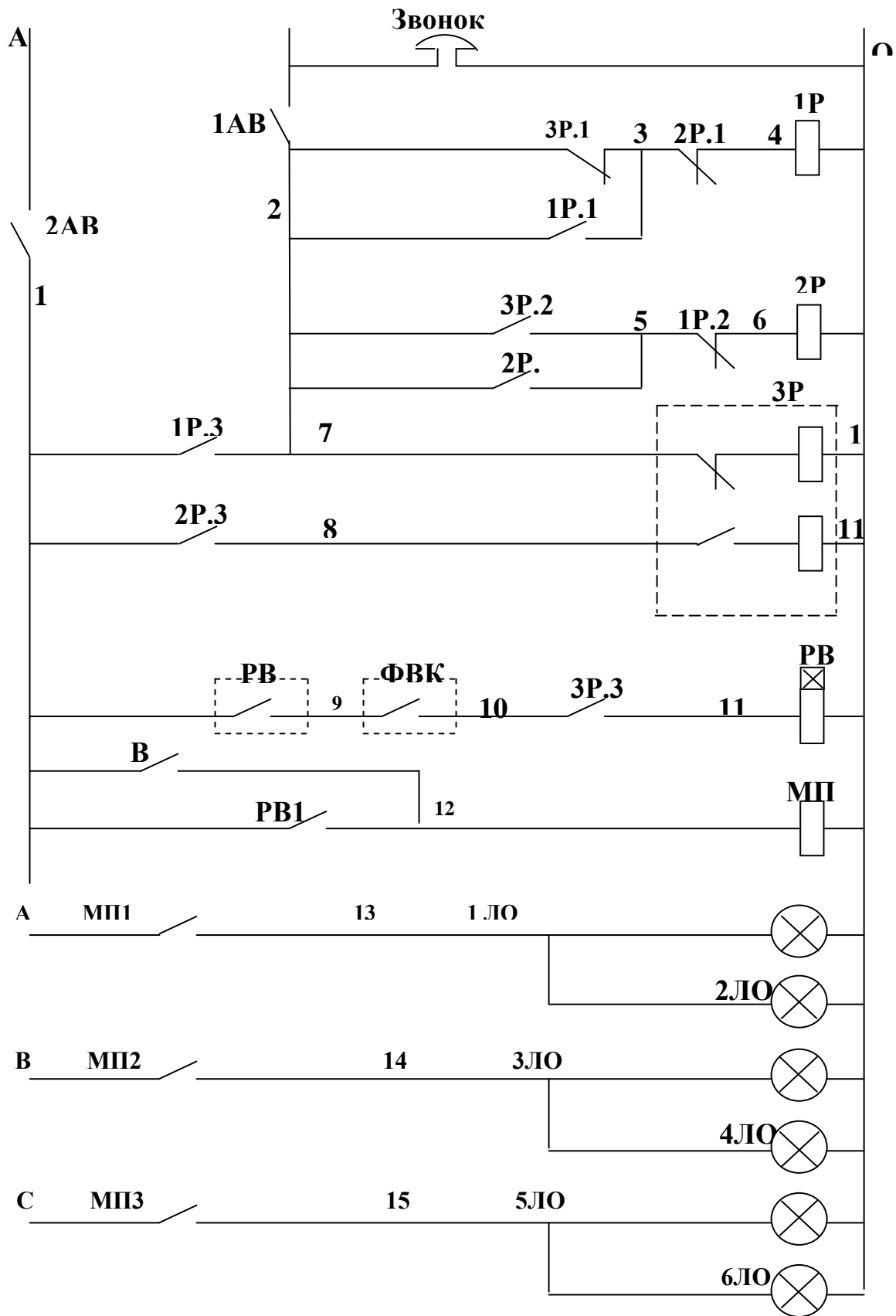
Рис 4.2 Схема автоматическое управление освещение школьных коридоров в зависимости от звонка.
