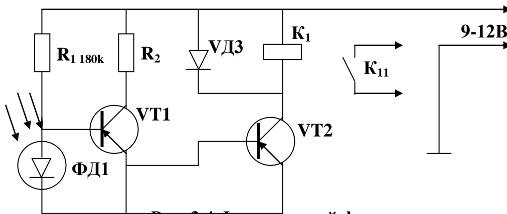
Рис. 3.4 Фотодиодный фотореле
