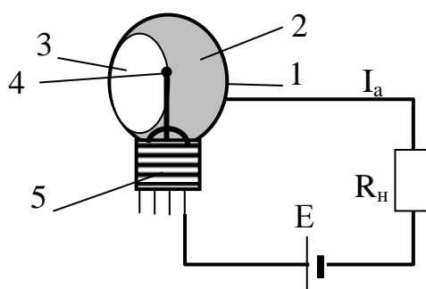
Фотоэлемент с внешним фотоэффектом типа ЦВ-1.
