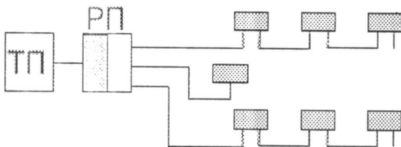
Рис.10.3 - радиально-магистральными
