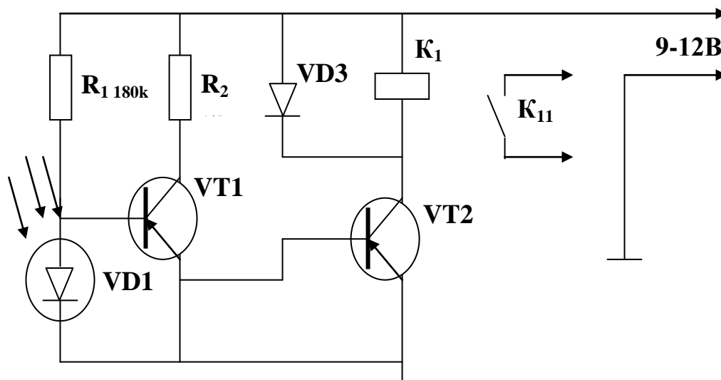
Рис. 2.4 Фотодиодное фотореле
