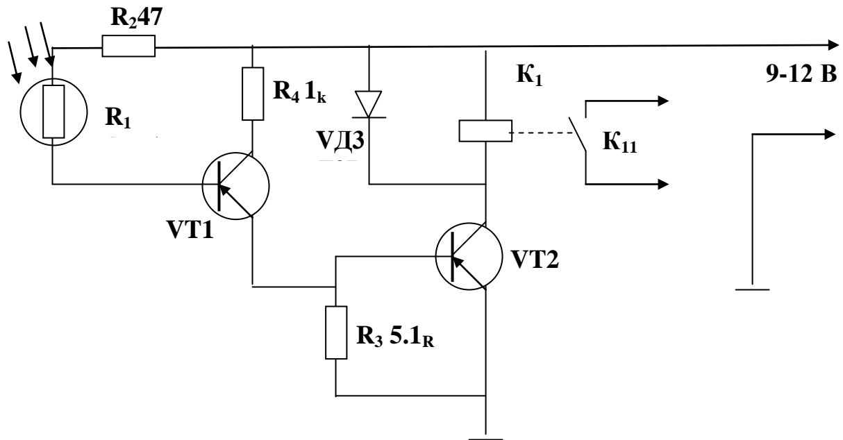
Рис. 2.3 Фоторезисторное фотореле.
