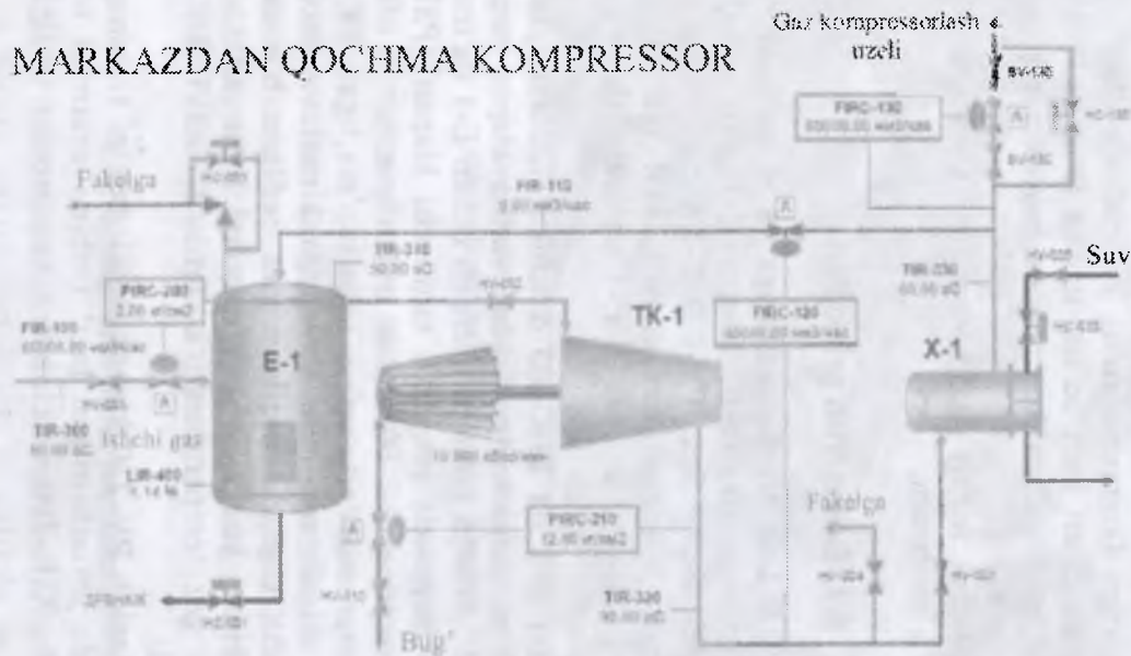
5.4-rasm. Kompressorlash tugunlari sxemasi
