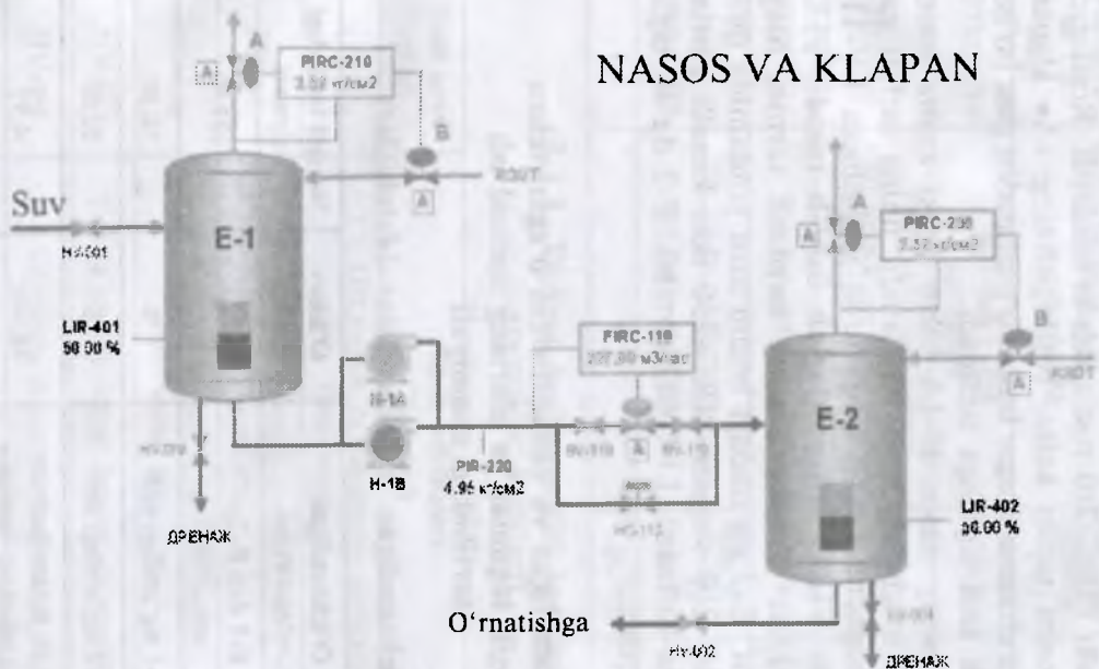
3.9-rasm. Ikkita sig'imdan iborat texnologik quriima
