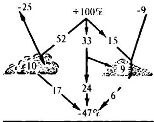
9-расм. Қисқа тўлқинли радиация кучининг атмосферадан ўтишида камайиши (Дажо, 1975).
