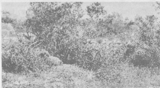
4-rasm. Abiotik omillar. Havo, suv, tuproq, quyosh, temperatura va iqlim – yerdagi butun hayotga ta'sir etuvchi omillar.
