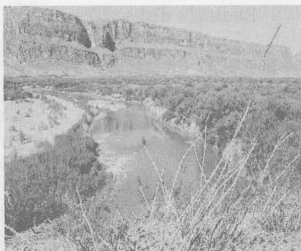
4-rasm. Abiotik omillar. Havo, suv, tuproq, quyosh, temperatura va iqlim – yerdagi butun hayotga ta'sir etuvchi omillar.
