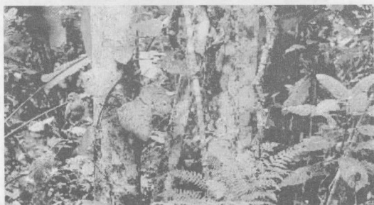
5–6-rasmlar. Suv ekologik omili. Fotosintez jarayoni. Cho'ldagi hayot turlarning uzoq vaqt davomida suvsiz yashashi bilan tasvirlanadi. Minglab turlar yomg'ri o'rmonda yashashga moslashgan.
