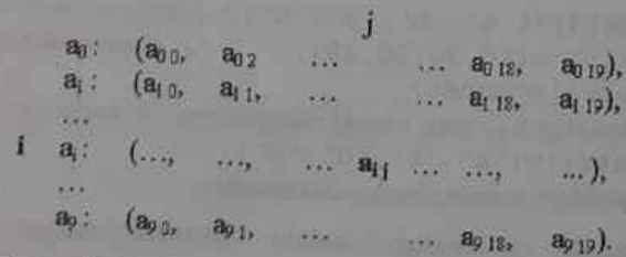
7.2-rasm. Ikki o'lchamli massivning xotiradagi joylashuvi
