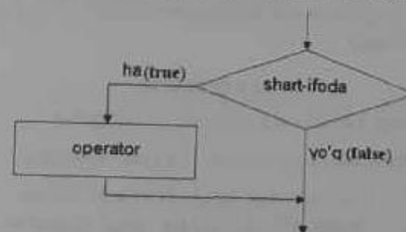
4.1-rasm. if () shart operatorining blok sxemasi
