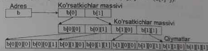
7.3-rasm. Uch o'lchamli massivning xotirada tashkil bo'lishi
