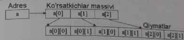
7.3-rasm. Ikki o'lchamli massiv elementlariga murojaat
