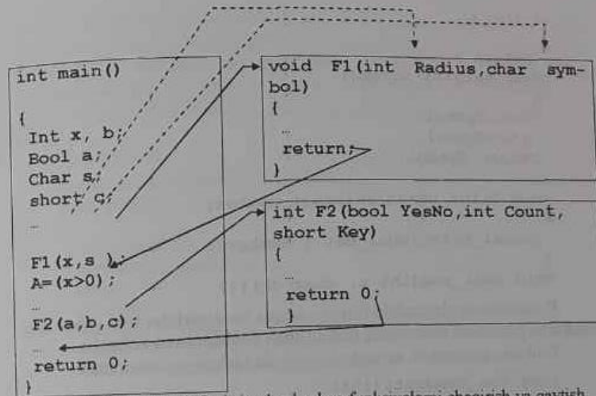
5.1-rasm. Bosh funksiyadan boshqa funksiyalarni chaqirish va qaytish
