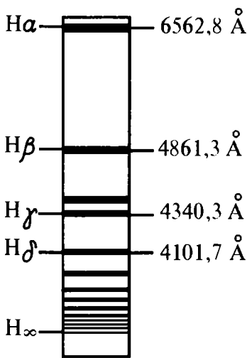
11.5 - расм. Кўзга кўринадиган водород спектри ва унга яқин бўлган ультрабинафша спектр соҳаси (Бальмер серияси).
