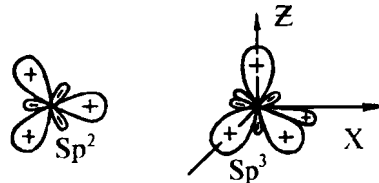
IV.12 - расм. sp^2 ва sp^3 - гибрид орбиталларининг ҳосил бўлиши.
