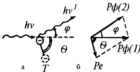
II.8 - расм. Комптон эффектани тушунтириш схемаси:
