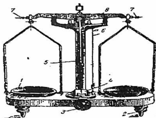
Texnik kimyoviy tarozisi
