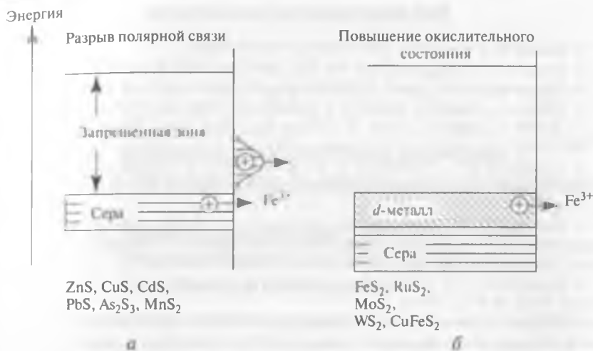
Рис. 11.6. Энергетические характеристики сульфидов, способных за счет удаления электронов разрывать связи в валентной зоне (а) или увеличивать окислительное состояние d -металла (б)
