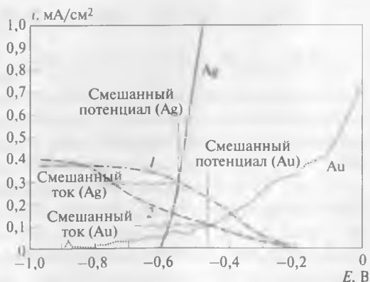
Рис. 13.17. Сравнение процессов растворения золота и серебра в цианидном растворе ( [\text{CN}] = 0,01 \text{ моль/дм}^3 ) и относительное расположение кривых, характеризующих восстановление кислорода: 1 — кислород (Ag + воздух); 2 — кислород (Au + воздух)
