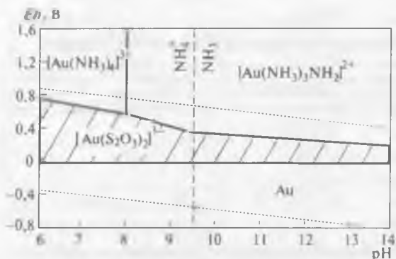
Рис. 16.7. Диаграмма Eh - pH для системы Au(0) - Au(I) - Au(III) - NH_3 - S_2O_3^{2-} - H_2O при [Au(I)] = 10^{-6} моль/дм 3 , [NH_3/NH_4^+] = 1 моль/дм 3 , [Na_2S_2O_3] = 0,1 моль/дм 3 , температуре 25 °С
