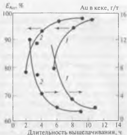
Рис. 17.13. Извлечение золота при последовательном применении выщелачивания и сорбции (1) и при сорбционной хлоринации (2).
