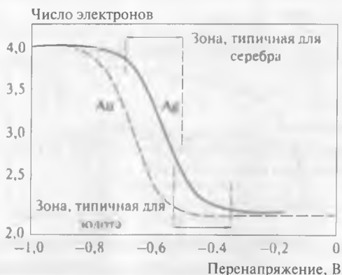
Рис. 13.21. Соотношение между числом электронов, участвующих в процессе растворения золотого и серебряного электродов. Цианидные растворы насыщались воздухом, \omega = 300 \text{ мин}^{-1} , температура 24^\circ\text{C}
