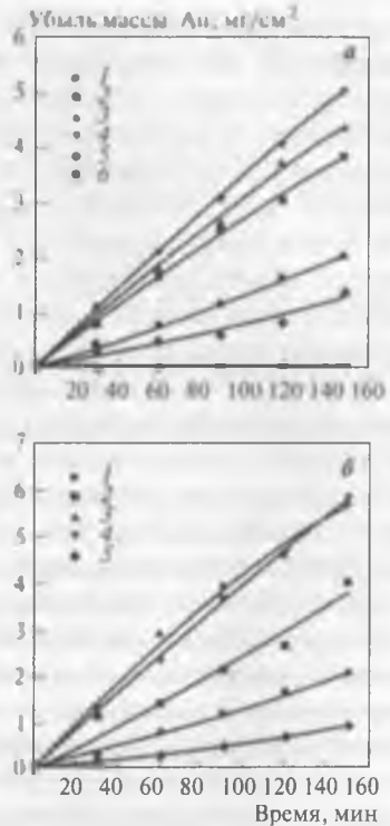
Рис. 4.10. Влияние сульфидных минералов на скорость электрохимического растворения золота в растворах, насыщенных воздухом (а) и кислородом (б) [68]:
