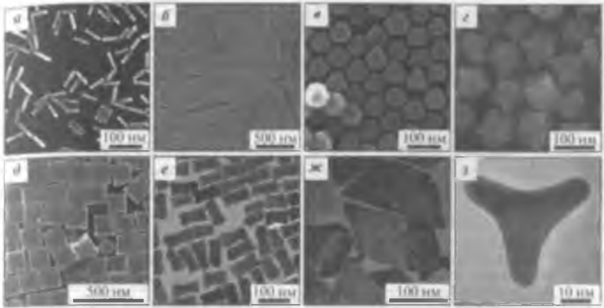
Рис. 6.6. SEM 1 - (a–d) и ТЕМ-изображения (e–z) наночастиц золота с различной морфологией, образованных при использовании СТАВ [6]
