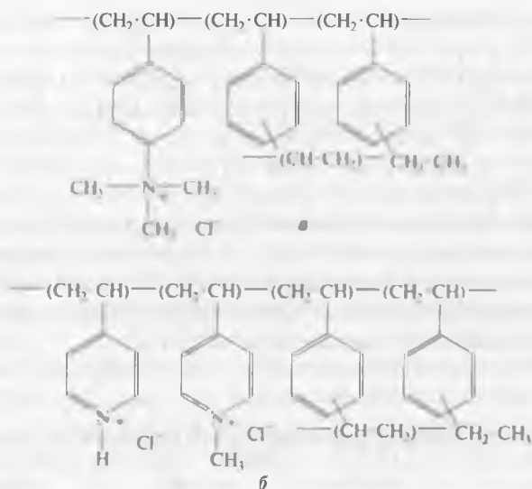
Рис. 21.5. Строение сильноосновных ионообменных смол Ionac A-641 (а) и Reillex HPQ (б)
