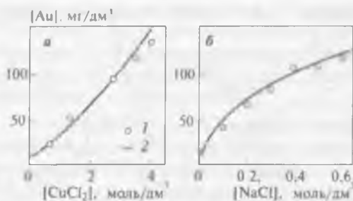
Рис. 17.17. Растворимость золота в системе \text{CuCl}_2 - \text{NaCl} - \text{HCl} при 102^\circ\text{C} : a - [\text{NaCl}] = 3,42 \text{ моль/дм}^3 , [\text{HCl}] = 0,1 \text{ моль/дм}^3 ; b - [\text{CuCl}_2] = 0,6 \text{ моль/дм}^3 , [\text{HCl}] = 0,1 \text{ моль/дм}^3 ; 1 – экспериментальные данные; 2 – расчетные данные
