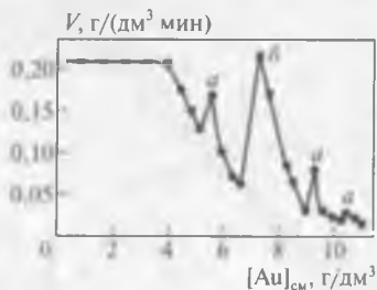
Рис. 21.22. Влияние насыщения слабоосновной смолы МГ-1 на скорость сорбционного извлечения [8]:
