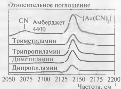
Рис. 21.16. ИКФП-спектры различных ионообменных смол, насыщенных золотом [10]
