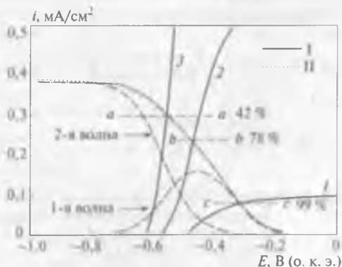
Рис. 13.20. Данные, характеризующие растворение серебра (I), восстановление кислорода (II) и плотности тока в сечениях a–a, b и c–c. Использован вращающийся серебряный электрод при \text{pH} = 11 , \omega = 300 \text{ мин}^{-1} и температуре 24 \text{ }^\circ\text{C} . [\text{NaCN}] , \text{мг/дм}^3 : 1 – 25, 2 – 122, 3 – 490
