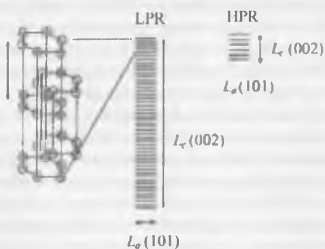
Рис. 24.4. «Сборка» гексагональных графитовых колец в d -направлении и качественное отличие размеров LPR- и HPR-кристаллитов
