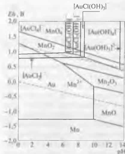
Рис. 17.15. Совмещенная диаграмма Eh – pH для системы Au – Mn – Cl – H 2 O при 298 К, P общ = 101,3 кПа, α Au = 10 -6 , α Mn = 10 -2 , α Cl = 1
