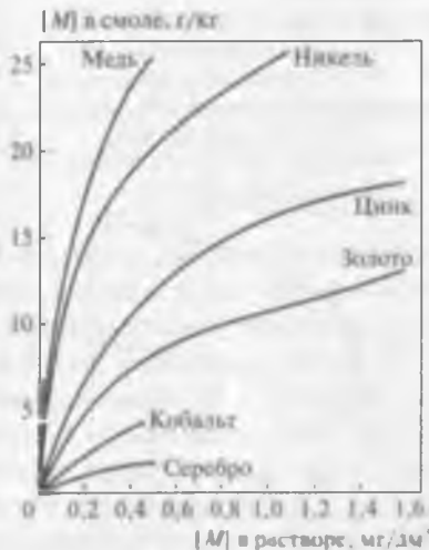
Рис. 21.8. Изотермы сорбции цианидных комплексов цветных металлов и серебра из производственных («Дурбан Дип Родепорт», ЮАР) насыщенных растворов сильноосновной смолы IRA-400 [8].
