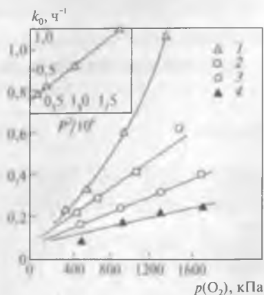
Рис. 10.1. Зависимость константы скорости k_n автоклавного окисления от температуры, °С: 1 – 200; 2 – 190; 3 – 180; 4 – 170
