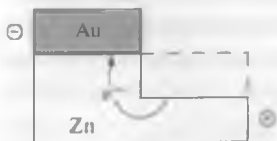
Рис. 19.6. Схема действия микрогальванического элемента при цементации золота цинком
