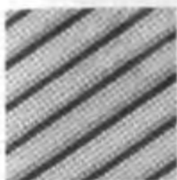
Рис. 7.6. STM-изображение ( 10 \times 10 нм) монослоя молекул этантиола на поверхности золота ( а ) и схема формирования монослоя ( б )
