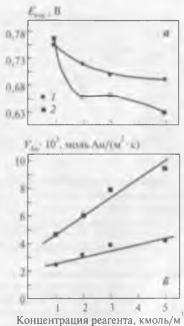
Рис. 17.6. Влияние концентрации иона \text{Cl}^- (1) при \text{pH} = 4 и концентрации \text{HCl} (2) на значение коррозионного потенциала (а) и удельную скорость растворения золота (б).
