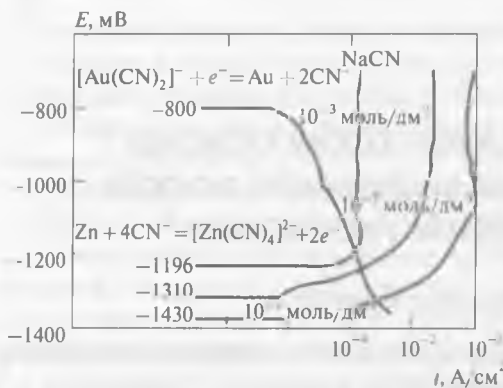
Рис. 19.1. Анодные поляризационные кривые, полученные с помощью вращающегося цинкового дискового электрода в цианидном растворе.
