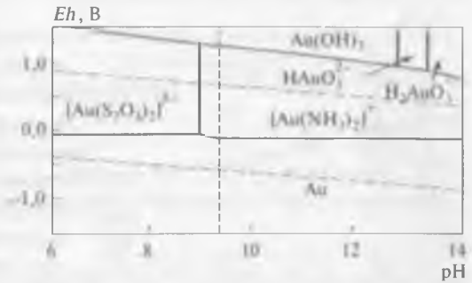
Рис. 16.5. Диаграмма Eh - pH для системы Au(0) - Au(I) - NH_3 - S_2O_3^{2-} - H_2O при [S_2O_3] = 0,2 моль/дм 3 , [NH_3]/[NH_4^+] = 0,4 моль/дм 3 , [Au] = 2,5 \cdot 10^{-3} моль/дм 3 , температуре 25 °C [2]
