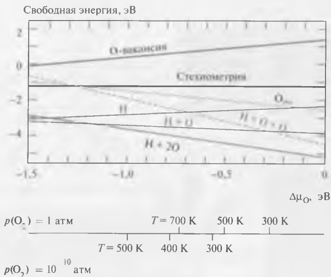
Рис. 7.18. Зависимость свободной энергии системы \text{Au}_7/\text{TiO}_2 от изменения химического потенциала кислорода. \text{O}_{\text{обог}} – система, обогащенная кислородом, зеленые линии относятся к системам, содержащим фрагменты воды и кислород (атомарный и молекулярный). Значение химического потенциала воды выбрано равным -2,96 \text{ эВ} , что соответствует p(\text{O}_2) = 10^{-10} \text{ атм} при 298 \text{ К}
