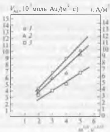
Рис. 17.9. Зависимость удельной скорости растворения золота от частоты вращения дискового электрода \omega и \text{pH} : 1 — \text{pH} = 0 ; 2 — \text{pH} = 2 ; 3 — \text{pH} = 4 . Общая концентрация хлора и других окислителей 2 \text{ моль/м}^3 , [\text{Cl}^-] = 1 \text{ кмоль/м}^3 , T = 295 \text{ К}
