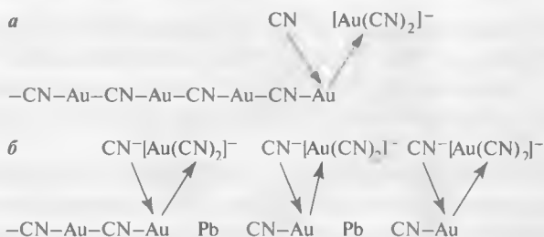
Рис. 13.14. Схема, иллюстрирующая растворение осадка AuCN, образующегося в отсутствие (а) и при наличии (б) Pb (II)
