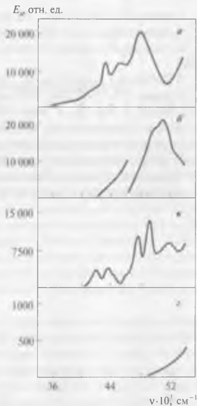
Рис. 2.6. УФ-спектры дicyанокомплексов в водном растворе: а – \text{K}[\text{Cu}(\text{CN})_2] ; б – \text{K}[\text{Ag}(\text{CN})_2] ; в – \text{K}[\text{Au}(\text{CN})_2] ; г – [\text{Hg}(\text{CN})_2]
