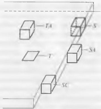
Рис. 4.1. Изменение координационного числа (и, соответственно, энергии) для атомов различного вида на слабо дезорганизованной поверхности металла
