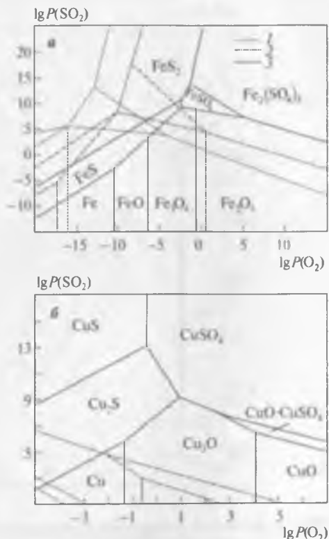
Рис. 9.2. Фазовые диаграммы \lg P(SO_2) - \lg P(O_2) для систем Fe – S – O (а) и Cu – S – O (б) при температурах обжига, К: 1 – 723; 2 – 873; 3 – 1273
