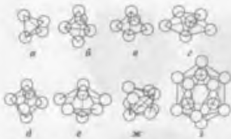
Рис. 5.3. Конфигурации нанокластеров из N плотноупакованных атомов [9]: a – тетраэдр ( N = 4 ); б – тригональная бипирамида ( N = 5 ) как сочетание двух тетраэдров; в – квадратная пирамида ( N = 5 ); г – трипирамида ( N = 6 ), образованная тремя тетраэдрами; д – октаэдр ( N = 6 ); е – пентагональная бипирамида ( N = 7 ); ж – звездообразный тетраэдр ( N = 8 ), образован пятью тетраэдрами – к каждой из четырех граней центрального тетраэдра присоединен еще один тетраэдр; з – икосаэдр ( N = 13 ), содержит центральный атом, окруженный 12 атомами, объединенными в 20 равносторонних треугольников [25]
