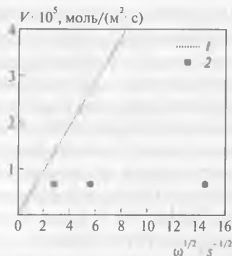
Рис. 13.11. Зависимости скорости растворения золота от интенсивности перемешивания, рассчитанные по уравнению Левича: 1 – для лимитирующей скорости диффузии кислорода; 2 – условия эксперимента Джеффри и Ритчи [1]. [CN^-]_{\text{в.р.}} = 20 \text{ ммоль/дм}^3, t = 25 \text{ }^\circ\text{C}
