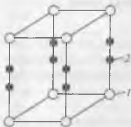
Рис. 2.2. Структура элементарной кристаллической ячейки AuCN : 1 – Au; 2 – CN
