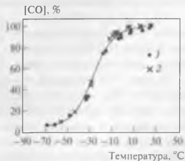
Рис. 7.13. Зависимость конверсии CO в \text{CO}_2 от температуры: 1 – 0,47 % Au/ \text{TiO}_2 ( \text{pH}_{\text{нач}} = 4 , \text{pH}_{\text{кон}} = 9 ); 2 – 0,55 % Au/ \text{TiO}_2 ( \text{pH}_{\text{нач}} = 11 , \text{pH}_{\text{кон}} = 8,5 )
