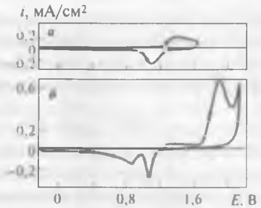
Рис. 4.6. Типичная циклическая вольтамперограмма для поликристаллического золотого электрода в растворе \text{NaOH} (1 моль/ \text{дм}^3 ) при 25 °С и скорости развертки потенциала, мВ/с: а – 50 (от 0 до 1,6 В); б – 10 (от –0,2 до 2,1 В)
