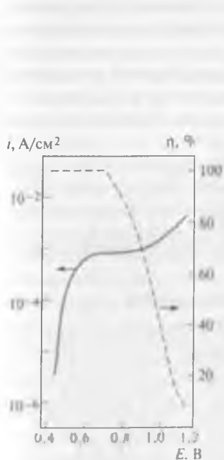
Рис. 15.1. Влияние потенциала E на процесс анодного растворения золота в серноокислом растворе ТМ [3]. [\text{H}_2\text{SO}_4] = 0,1 моль/дм 3 , [\text{SC}(\text{NH}_2)_2] = 0,1 моль/дм 3 ; температура 30 °C
