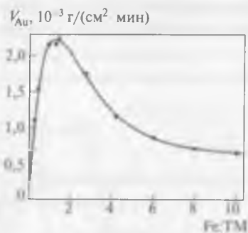
Рис. 15.5. Зависимость скорости растворения золота в ТМ-растворе, содержащем 0,4 моль/дм 3 SC(NH 2 ) 2 , от концентрации Fe 2 (SO 4 ) 3 при рН = 0,5, T = 298 К [16]
