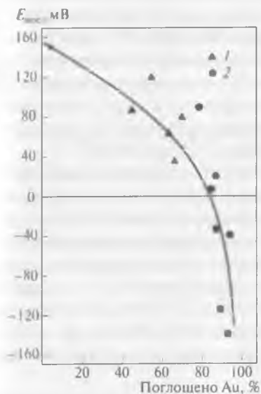
Рис. 23.2. Влияние восстановительного потенциала различных углей на сорбцию золота (1) из цианидных растворов (исходная концентрация золота 250 мг/дм 3 ): 1 – уголь на основе кокосовой скорлупы; 2 – битуминозный уголь
