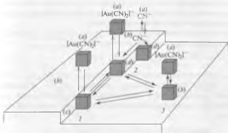
Рис. 13.15. Модель поверхности золота, характеризующая возможные пути протекания реакций при контакте с цианидными растворами: 1 – активный центр у конца структуры (с); 2 – активные центры, расположенные на изломе (d); 3 – адатом (ион) на плоскости (b); атомы в составе электролита (a)
