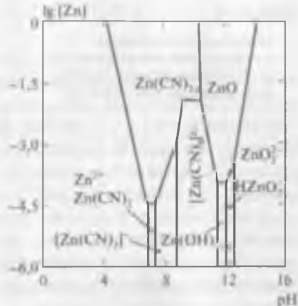
Рис. 19.4. Диаграмма \lg[\text{Zn}] - \text{pH} для системы \text{Zn} - \text{CN} - \text{H}_2\text{O} при 25^\circ\text{C} , E = 0,5 В, [\text{CN}^-] = 10^{-3} моль/дм 3
