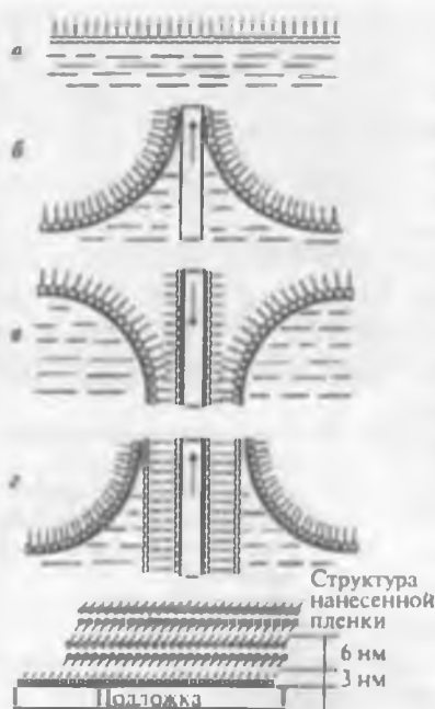
Рис. 7.3. Схема синтеза многослойной лэнгмюровской пленки [4]: а – структурирование пленки силами поверхностного натяжения; б, в, г – нанесение первого, второго и третьего слоев соответственно
