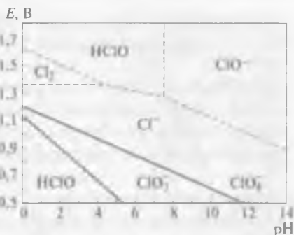
Рис. 17.1. Eh – pH-диаграмма для метастабильной системы хлор – вода (пунктирные линии) при 298 К, активности и парциальном давлении \text{Cl}_2 , равных 1. Сплошные линии соответствуют равновесию при окислении \text{Cl} (I) в составе кислоты \text{HClO} до \text{Cl} (V) и \text{Cl} (VII)
