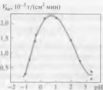
Рис. 15.6. Зависимость скорости растворения золота в растворе, содержащем 0,40 моль/дм 3 SC(NH 2 ) 2 и 0,36 моль/дм 3 Fe 2 (SO 4 ) 3 , от pH при T = 298 \text{ К} [16]
