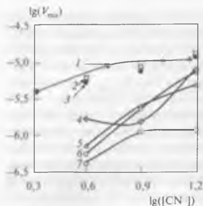
Рис. 4.9. Зависимость удельной скорости электрохимического растворения золота V_{ма} от величины, численно равной концентрации цианида для покрытий различного типа [62]: 1 – без покрытия [63]; 2 – без покрытия, рН = 10,5, 11,5 [64]; 3 – глина, рН = 10,5; 4 – активный уголь, рН = 10,5; 5 – РУВ, рН = 10,5; 6, 7 – графит, рН = 10,5
