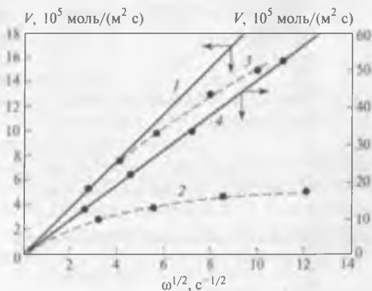
Рис. 16.9. Зависимость удельной скорости растворения от угловой скорости вращения дискового электрода:
