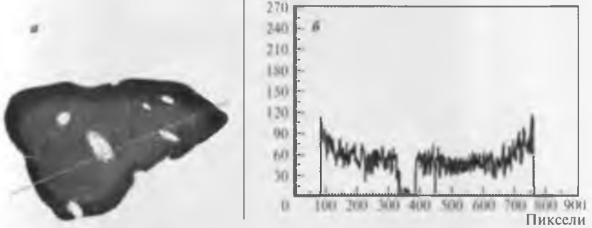
Рис. 23.5. Микротомография среза зерна активного угля «Пика», содержащего 2,5 г Au/кг (насыщение 24 ч): a – осевой разрез; б – распределение золота по площади разреза (1 пиксель = 5,15 мкм)
