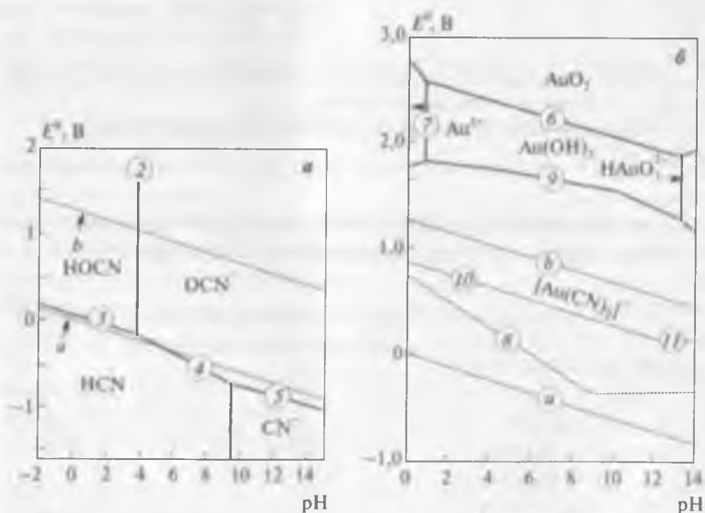
Рис. 12.3. Диаграммы Eh - \text{pH} для систем CN – H 2 O (а) и Au – CN – H 2 O (б) при 25 °С
