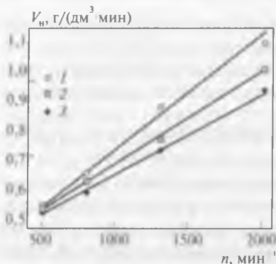
Рис. 21.21. Влияние интенсивности перемешивания на скорость насыщения ( V_n ) сильноосновной смолы IRA-400 в начальный период [8]:
