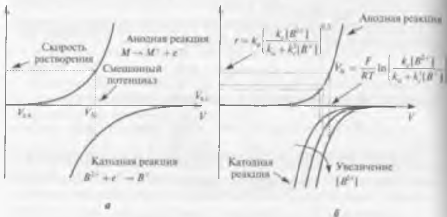
Рис. 2.П.3. Диаграммы, характеризующие электрохимический механизм растворения минералов [3]:
