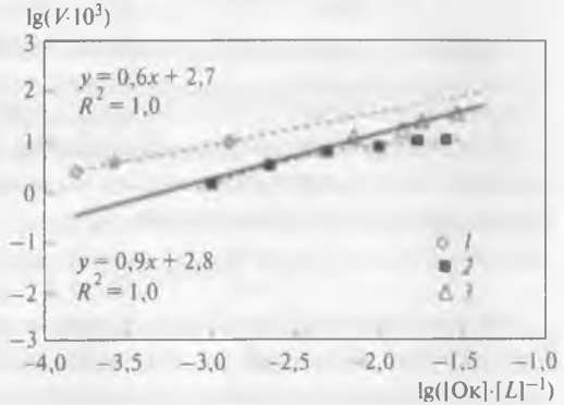
Рис. 16.12. Зависимость скорости растворения золота от концентрации реагентов, определенная методом вращающегося диска: 1 — O 2 /цианид; 2 — Cu 2+ /NH 3 — S 2 O 3 2- ; 3 — Fe 3+ /ТМ
