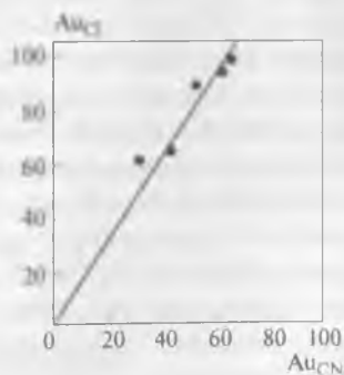
Рис. 23.3. Соотношение между количествами золота, адсорбированного из хлоридного и цианидного растворов активными углями на основе кокосовой скорлупы с разной восстановительной способностью. Содержание в растворе: 800 мг/дм 3 [AuCl_4]^- при pH = 1 в среде HCl; 250 мг/дм 3 Au в составе K[Au(CN)_2]
