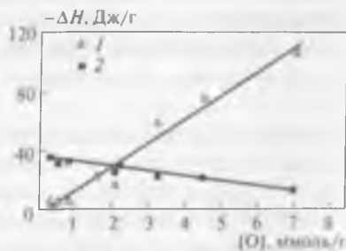
Рис. 22.6. Изменение энтальпии нейтрализации для NaOH (1) и HCl (2) в зависимости от содержания кислорода на поверхности угля
