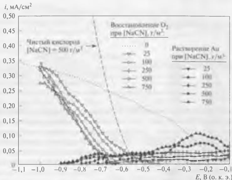
Рис. 13.16. Вольтамперограммы, характеризующие растворение золота и восстановление кислорода при разных концентрациях цианида. Температура 24 °С, pH = 10,5, \omega = 300 \text{ мин}^{-1} при диаметре дискового электрода 1,4 см [23]
