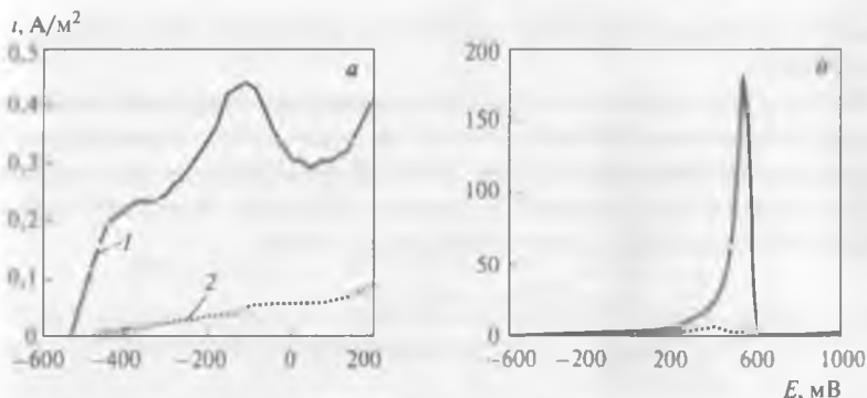
Рис. 13.12. Поляризационные кривые при окислении золота в сверхчистых (1) и ч. д. а. (2) растворах при скорости вращения электрода 300 \text{ мин}^{-1} , скорости изменения потенциала 1 \text{ мВ/с} и t = 25^\circ \text{C} . Концентрация цианида: а – 20 \text{ ммоль/дм}^3 ; б – 100 \text{ ммоль/дм}^3
