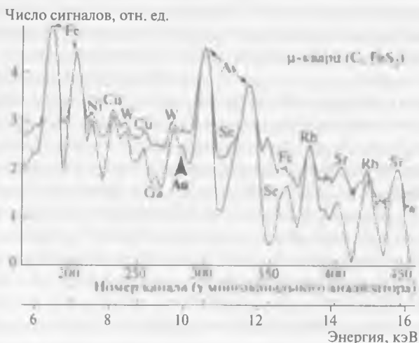
Рис. 25.5. Протон микрозондовый спектр микрокристаллического зерна кварца со следами графитизированного углерода и пирита. Концентрация золота – 20 г/т. Верхний спектр характеризует все выявленные элементы, а нижний спектр очищен от «фона»
