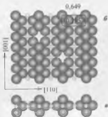
Рис. 7.17. STM-изображение поверхности \text{TiO}_2[110] ( а ) и схематичная структурная модель \text{TiO}_2 ( б – вид сверху; в – вид сбоку)
