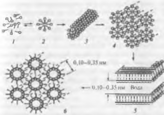
Рис. 7.4. Структуры, возникающие в растворах ПАВ:
