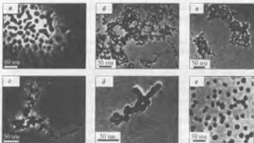
Рис. 6.1. ТЕМ-изображения золотых наночастиц на разных стадиях цитратного синтеза по методу Туркевича [8]
