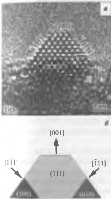
Рис. 7.15. Изображение наночастицы золота диаметром 2 нм на поверхности TiO 2 (а), полученное с помощью электронной микроскопии высокого разрешения, и схематичная трехмерная модель внутренней ориентации нанокристалла (б)
