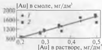
Рис. 21.6. Участок изотермы сорбции [\text{Au}(\text{CN})_2]^- смолой «Миникс»: 1 — по уравнению Фрейндлиха; 2 — анализ
