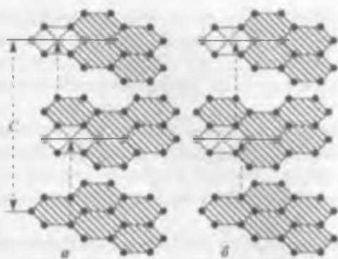
Рис. 22.3. Структура графитовых слоев: a — упорядоченная структура в графите; b — неупорядоченная структура в микрокристаллическом активном углероде
