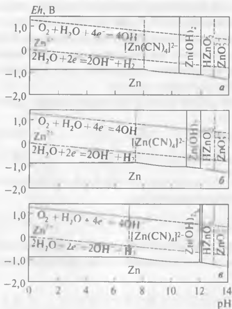
Рис. 19.2. Eh – pH-диаграммы для системы Zn – CN – H 2 O [I] при [Zn(II)] = 1,5 \cdot 10^{-4} моль/дм 3 , [NaCN] , г/дм 3 : а – 0,1; б – 0,3; в – 0,5
