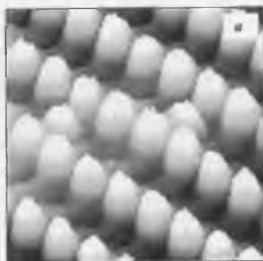
Рис. 7.17. STM-изображение поверхности \text{TiO}_2[110] ( а ) и схематичная структурная модель \text{TiO}_2 ( б – вид сверху; в – вид сбоку)
