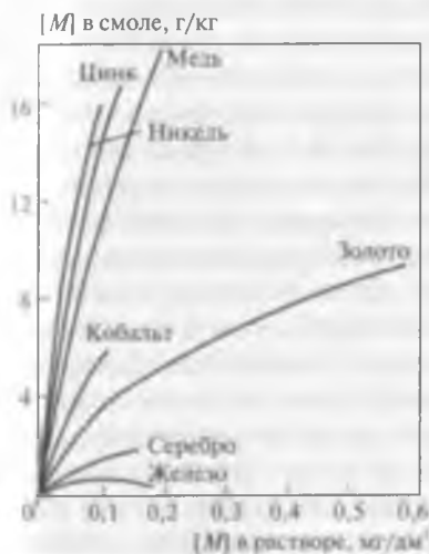
Рис. 21.7. Изотермы сорбции цианидных комплексов цветных металлов, железа и серебра из производственных («Грутвлей», ЮАР) насыщенных растворов сильноосновной смолы A101-DU [8].
