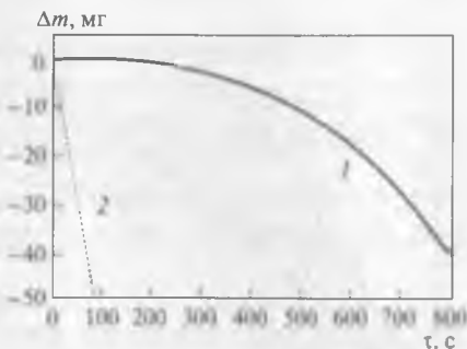
Рис. 16.8. Скорость растворения золота (1) и серебра (2) при [\text{S}_2\text{O}_3^{2-}] = 0,4 \text{ моль/дм}^3 , [\text{NH}_3] = 0,84 \text{ моль/дм}^3 , [\text{Cu}^{2+}] = 25 \text{ ммоль/дм}^3
