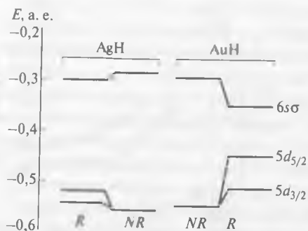
Рис. 3.3. Релятивистские ( R ) и нерелятивистские ( NR ) орбитальные энергии ( E ) молекул AuH и AgH [11]
