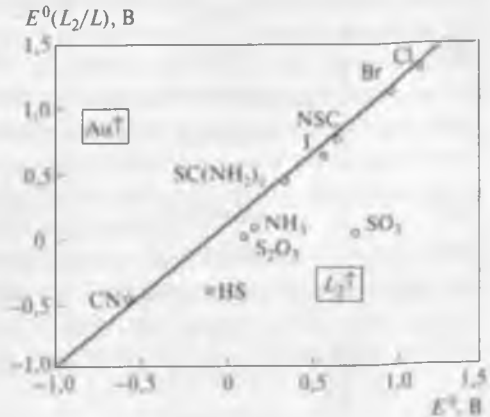
Рис. 14.2. Корреляция между значениями стандартных восстановительных потенциалов пары Au(I)/Au(0) и пар L_2/L : Au^+ — область большей устойчивости Au(I) ; L_2^+ — область большей устойчивости лигандов
