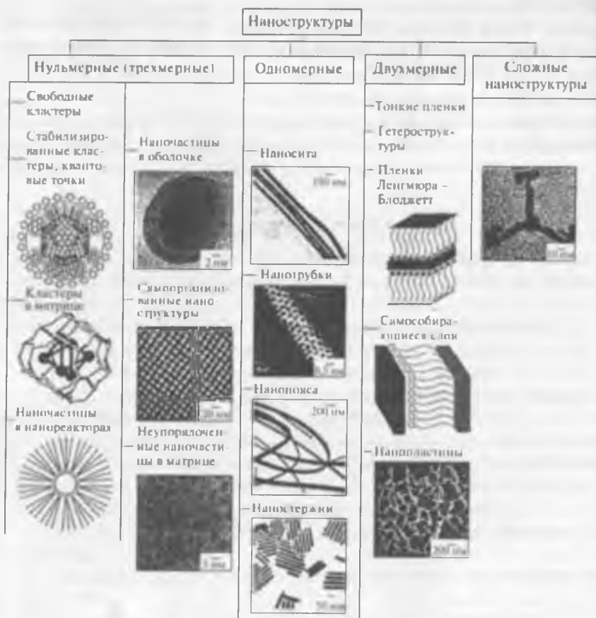
Рис. 7.1. Классификация наноструктур [1]
