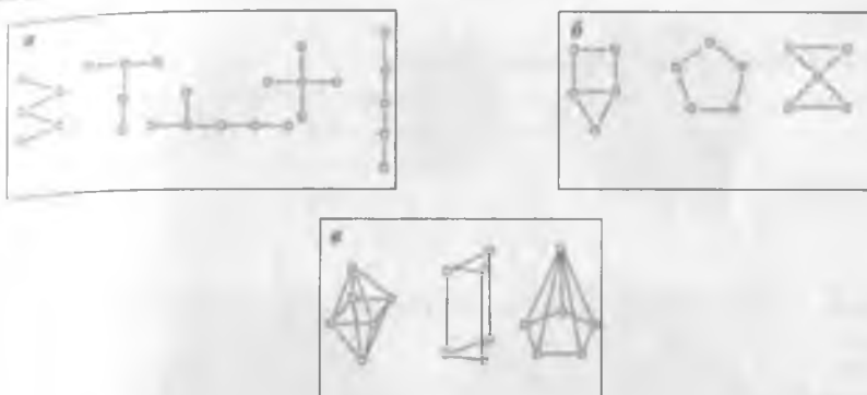
Рис. 5.1. Типы структур кластерного остова: a – цепочечные; b – кольцевые; c – полиэдральные
