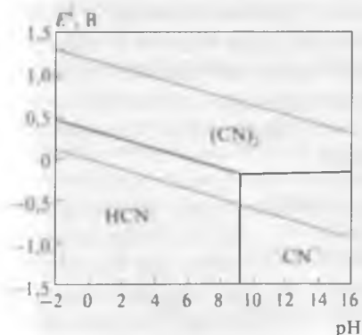
Рис. 12.4. Диаграмма Eh – pH для системы CN – H 2 O при допущении стабильности (CN) 2 . Активности всех соединений равны единице, p(\text{CN})_2 = 98 \text{ кПа} , температура 25 °С
