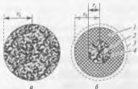
Рис. 9.1. Исходная сферическая частица твердого вещества радиусом r_0 (а) и частица радиусом r_c после окислительного обжига в течение времени t (б): 1 – огарок; 2 – остаток ядра; 3 – внешний слой газа; 4 – кислород
