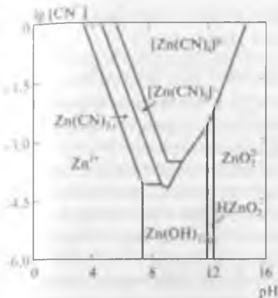
Рис. 19.3. Диаграмма \lg[\text{CN}^-] - \text{pH} для системы \text{Zn} - \text{CN} - \text{H}_2\text{O} при 25^\circ\text{C} , [\text{Zn}] = 10^{-4} моль/дм 3 , E = 0,5 В
