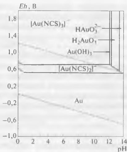
Рис. 18.2. Eh – pH-диаграмма для системы Au – NCS – H 2 O при 25 °С, \alpha_{\text{Au}} = 10^{-1} , \alpha_{\text{SCN}} = 10^{-5}
