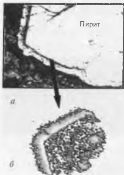
Рис. 25.3. Микрофотография участка зерна FeS_2 с оболочкой мышьяковистого пирита, полученная электронным сканированием (а), и изображение зон, обогащенных мышьяком (выделены красным цветом, б)
