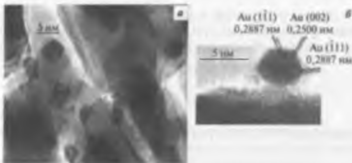
Рис. 7.14. ТЕМ-изображения наночастиц золота на поверхности оксидных подложек: а – Fe 2 O 3 , размер частиц Au – 2–5 нм; б – ZnO, размер частиц Au – 5 нм
