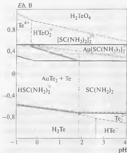
Рис. 15.8. Диаграмма Eh – pH для системы AuTe_2 - SC(NH_2)_2 - H_2O при 298 К. Активности растворенных соединений для золота – 10^{-5} , теллура – 10^{-4} , SC(NH_2)_2 – 10^{-4} , HSC(NH_2)_2^+ – 10^{-2} , [SC(NH_2)_2]_2^+ – 10^{-1}
