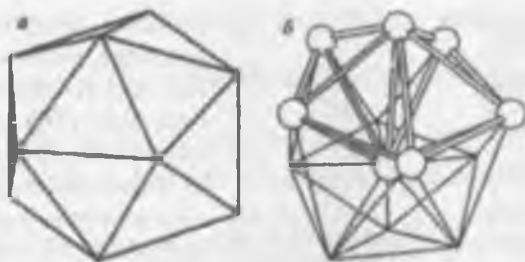
Рис. 6.11. Двадцатигранный квазикристалл (а) и соответствующее этой конфигурации расположение атомов (б) в кластере с N = 13 (показана часть атомов)
