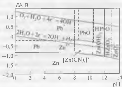
Рис. 19.7. Eh - pH -диаграмма для системы Zn - Pb - CN - H_2O [1].
