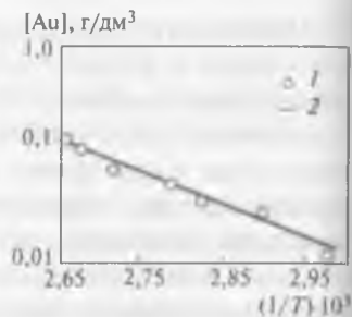
Рис. 17.18. Растворимость золота в хлоридном растворе как обратная функция от температуры: 1 – экспериментальные данные; 2 – расчетные данные. [\text{NaCl}] = 3,42 \text{ моль/дм}^3 , [\text{CuCl}_2] = 0,6 \text{ моль/дм}^3 , [\text{HCl}] = 0,1 \text{ моль/дм}^3
