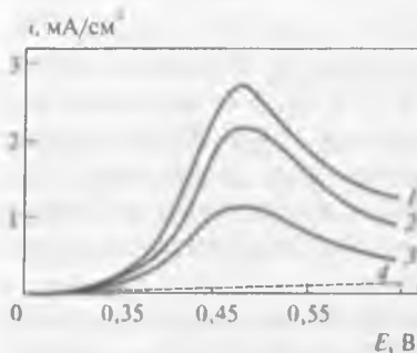
Рис. 15.4. Поляризационные кривые, полученные при растворении золота в растворе, содержащем 0,1 моль/дм 3 SC(NH 2 ) 2 и по 0,5 моль/дм 3 H 2 SO 4 и Na 2 S, 10 -5 моль/дм 3 : 1 – 4; 2 – 2; 3 – 1; 4 – 0
