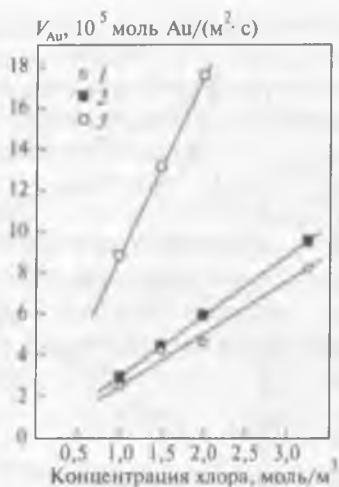
Рис. 17.7. Зависимость удельной скорости растворения золота от концентрации \text{Cl}_2 в растворе: 1 — [\text{HCl}] = 1 \text{ кмоль/м}^3 , T = 295 \text{ К} , частота вращения дискового электрода 240 \text{ мин}^{-1} ; 2, 3 — теоретические значения скорости растворения по Левичу [21] (2 — в виде [\text{AuCl}_4]^- ; 3 — в виде [\text{AuCl}_2]^- )
