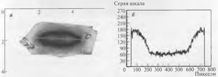
Рис. 23.6. Микротомография среза зерна активного угля «Пика», содержащего 25,0 г Au/кг (насыщение 24 ч): a – осевой разрез; б – распределение золота по площади разреза (1 пиксель = 5,15 мкм)
