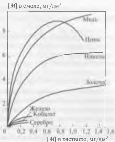
Рис. 21.11. Изотермы сорбции цианидов железа, благородных и цветных металлов из производственных растворов завода «Дурбан Дип Родепорт» (ЮАР) с помощью слабоосновной смолы А-7 [8]. Отношение объемов раствор:смола = 1000:1, \text{pH} = 7 , t = 20^\circ\text{C}
