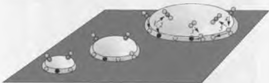
Рис. 7.19. Схема роста термодинамической стабильности окисленного состояния кластеров золота при увеличении их размера [43]: 1 – \text{CO} -атака на \text{O} в кольцевой зоне окисленного золота; 2 – образование вакансии и \text{CO}_2 ; 3 – адсорбция \text{O}_2 на вакансии; 4 – \text{CO} -атака на \text{O}_2 ; 5 – образование \text{CO}_2 и реокисление золота
