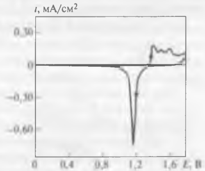
Рис. 4.3. Типичная вольтамперограмма, записанная для поликристаллического золотого диска в растворе H_2SO_4 (1 моль/дм 3 ) при 25 °С. Скорость развертки потенциала 50 мВ/с (от 0 до 1,8 В)
