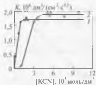
Рис. 19.11. Зависимость констант скорости реакций цементации серебра (1) и золота (2) от концентрации свободного цианида калия
