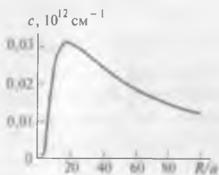
Рис. 5.7. Зависимость плотности дефектов c в кластере от его относительного размера R/a
