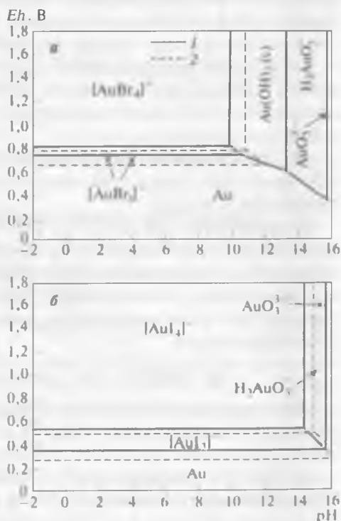
Рис. 18.1. Eh - \text{pH} -диаграммы для систем \text{Au} - \text{Br}_2 - \text{H}_2\text{O} (а) и \text{Au} - \text{I}_2 - \text{H}_2\text{O} (б) при 25^\circ\text{C} : 1 - \alpha_{\text{Au}} = 10^{-3} , \alpha_{\text{Br}^-} = \alpha_{\text{I}^-} = 1 ; 2 - \alpha_{\text{Br}^-} = \alpha_{\text{I}^-} = 5
