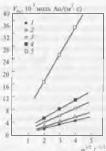
Рис. 17.8. Зависимость удельной скорости растворения золота от частоты вращения дискового электрода: 1–3 — [\text{HCl}] = 1 \text{ кмоль/м}^3 , [\text{Cl}_2] = 2 \text{ моль/дм}^3 (1 — \text{pH} = 4 ; 2 — \text{pH} = 2 ; 3 — \text{pH} = 0 ); 4, 5 — расчетные значения скорости по Левичу [21] при массопереносе, контролируемом восстановлением \text{Cl}_2 (4 — образование [\text{AuCl}_4]^- ; 5 — образование [\text{AuCl}_2]^- )
