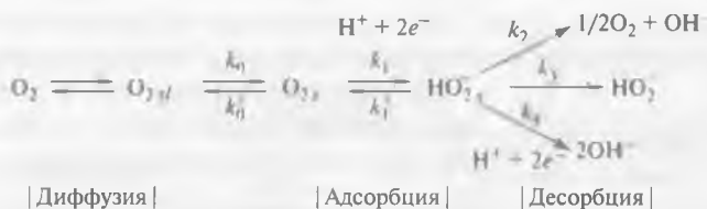
Рис. 13.18. Схема массопереноса кислорода при двух- и четырехэлектронной реакциях [37, 38]: \text{O}_{2,ст} – кислород в водной фазе у поверхности металла; \text{O}_{2,с} и \text{HO}_2^- – адсорбированные состояния; k_0-k_2 , k_0-k_3 – константы двухэлектронного процесса; k_0-k_4 – константы четырехэлектронного процесса
