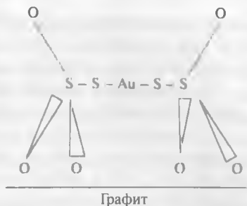
Рис. 16.13. Стереорасположение тиосульфатного комплекса золота на поверхности графита
