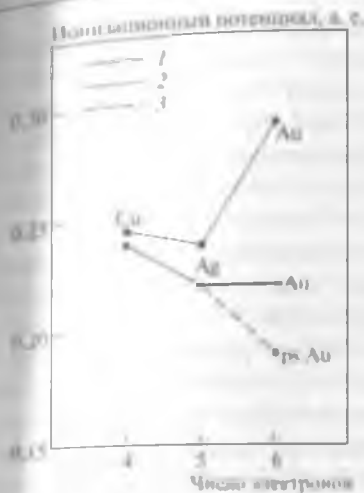
Рис. 3.1. Относительные значения ионизационных потенциалов металлов подгруппы меди [13, 14]: 1 – с учетом релятивистских эффектов; 2 – без учета релятивистских эффектов; 3 – псевдопотенциал ( \psi_s ), без учета f -электронов
