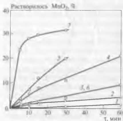
Рис. 17.14. Скорость растворения \text{MnO}_2 в кислотных хлоридных растворах (график построен по данным [30]) при 25 (1–5) и при 70 °С (6, 7): 1 – \text{HCl} (1 моль/дм 3 ) + \text{MnO}_2 ; 2 – \text{HCl} (1 моль/дм 3 ) + \text{MnO}_2 + \text{PbS} ; 3 – \text{HCl} (8 моль/дм 3 ) + \text{MnO}_2 ; 4 – \text{HCl} (8 моль/дм 3 ) + \text{MnO}_2 + \text{ZnS} ; 5 – \text{HCl} (8 моль/дм 3 ) + \text{MnO}_2 + \text{CuFeS}_2 ; 6 – \text{HCl} (4 моль/дм 3 ) + \text{MnO}_2 ; 7 – \text{HCl} (8 моль/дм 3 ) + \text{MnO}_2 + \text{ZnS}
