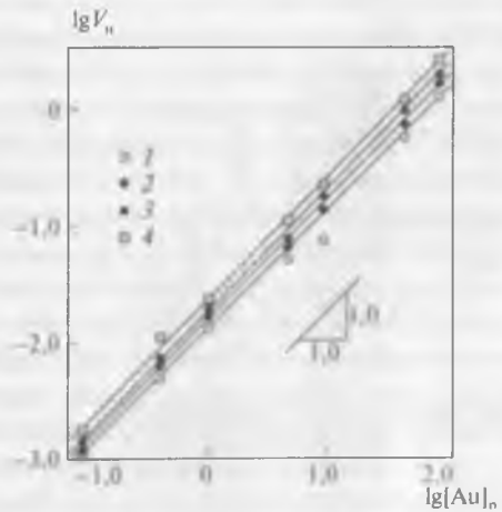
Рис. 21.20. Влияние концентрации золота в растворе на скорость насыщения смолы IRA-400 в начальный период [8] при скорости перемешивания, мин -1 : 1—500; 2—800; 3—1300; 4—2000. Размер зерен смолы 0,85–1,0 мм, pH = 6, ионная сила раствора - 0
