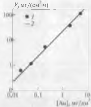
Рис. 19.10. Влияние концентрации золота на скорость цементации: 1 – экспериментальные данные; 2 – расчет
