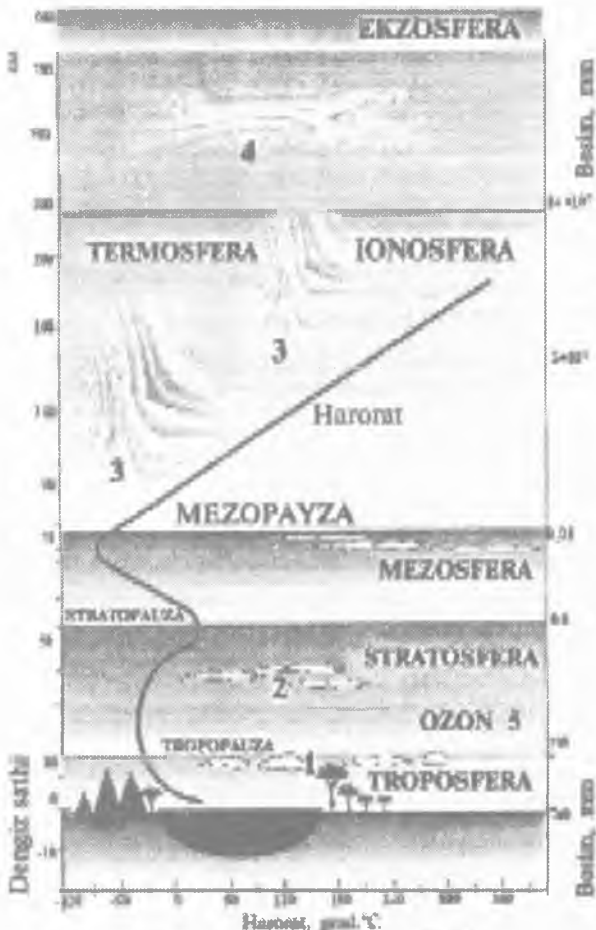
Atmosfera ning vertikal tuzilishi namunasi 1-joyvatqiy va passimon bulutlar; 2-uzdofalmoq bulutlar; 3-quyi sonozferadagi qutb yog'ulalar; 4-yuqori kionozferadagi qutb yog'ulalar. 3-ozon miqdori eng ko'p qatlam.
