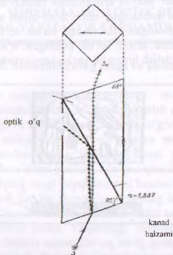
1.8-rasm. Nikol prizmasidagi nur yo'li.
