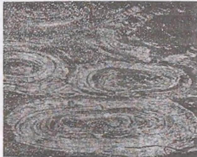
5.63-rasm. Marganes ma'dani. Psilomelan va piroluzitning oolitli ma'dan donalari. Chiaturi koni. Nik.II, A.G.Betextindan olingan.
