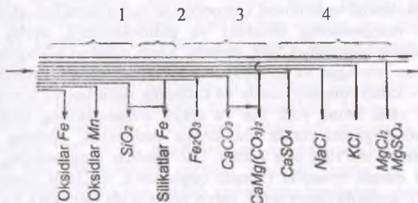
5.6-rasm. L.V. Pustovalov (1940) bo'yicha moddalarning kimyoviy cho'kish - differentsiatsiyalanish sxemasi:
