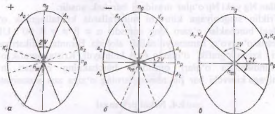
1.7-rasm. Kristallar indikatriyasining optik o'qlar tekisligi bo'yicha kesimi: a – optik musbat; b – optik manfiy; v – neytral. A_1 va A_2 – optik o'qlar; K_1 va K_2 – ularga to'g'ri keladigan doira kesimi.
