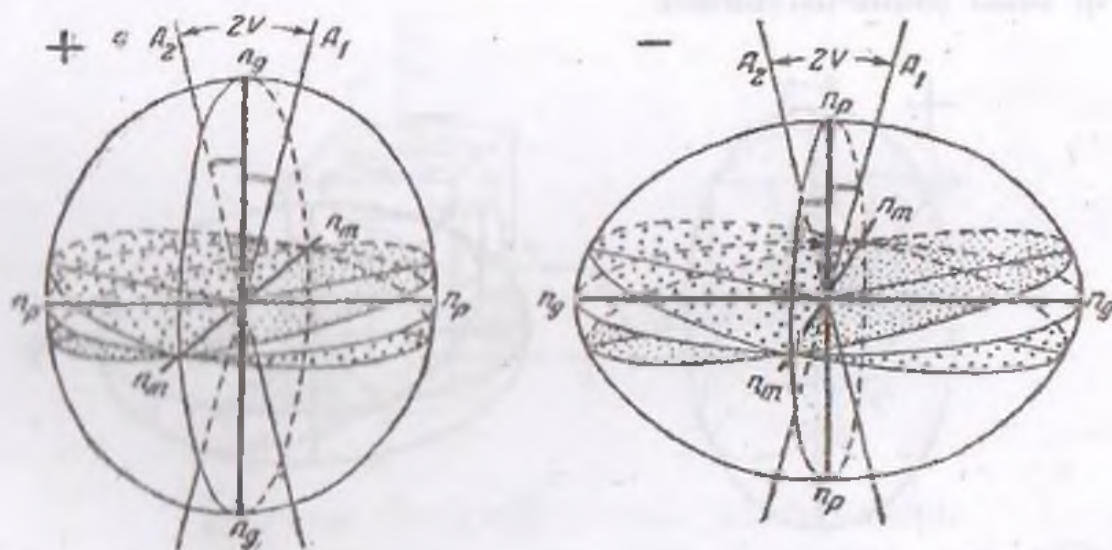
1.6-rasm. Ikki o'qli kristallarning musbat (+) va manfiy (-) optik indikatrasi.
