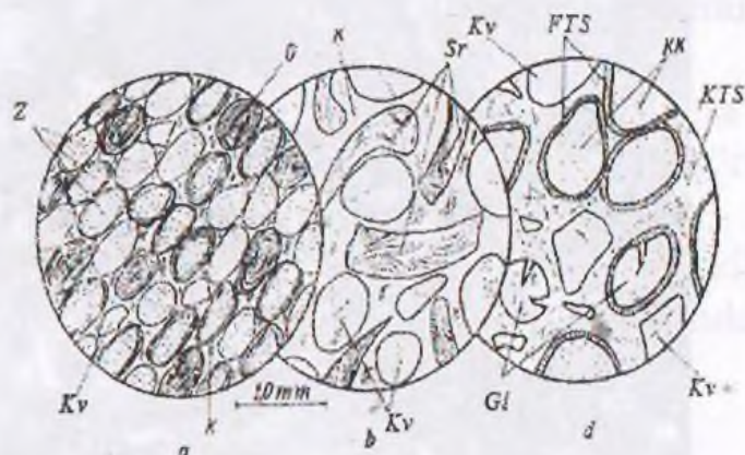
5.59- rasm. Qatlamli fosforitlar:
