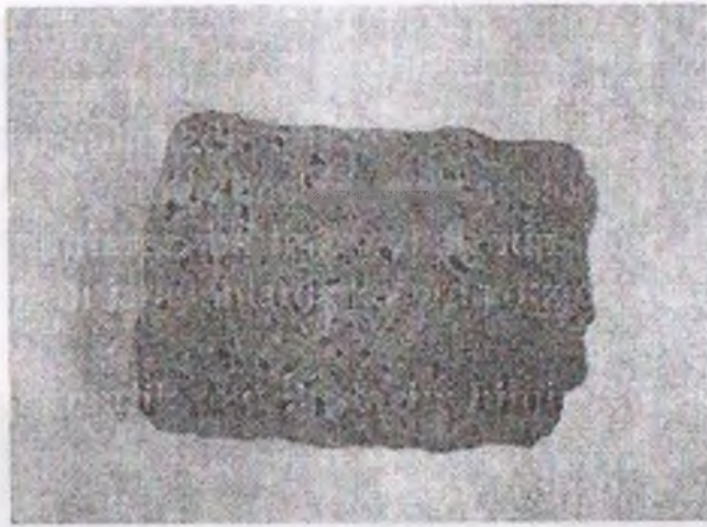
4.18-rasm. Porfirli struktura.
