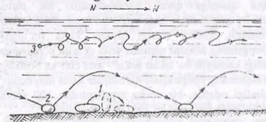
5.3- rasm. Bo'laklarning suv ( yoki havo) oqimida ko'chirilishi.
