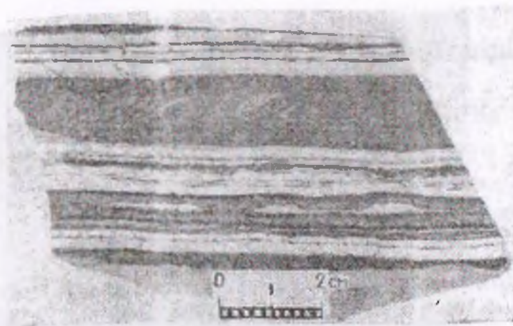
6.24-rasm. Yo'l-yo'l teksturali kvarsit.
