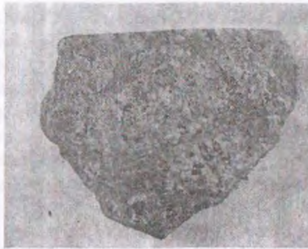
4.105-rasm. Nefelinli sienit.
