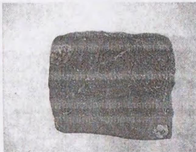
4.20-rasm. Afir struktura.
