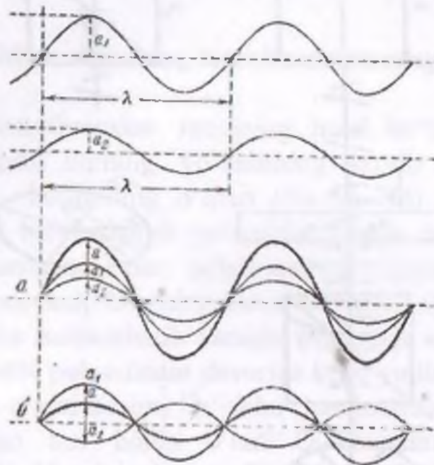
3.2-rasm. Monoxromatik yorug'lik qutblangan to'lqinlarining interferensiya sxemasi.
