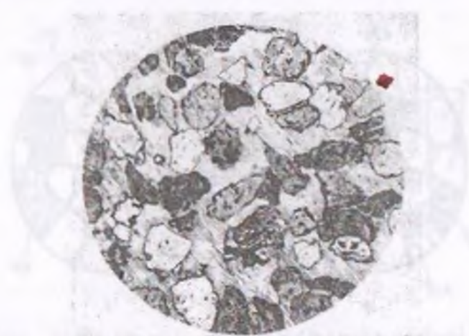
5.24-rasm. Polimiktli qumtosh (yirik donali bazal turidagi gipsli sementatsiya bilan). G.N.Yershova. Nikol II; kattal. 42
