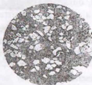
5.31-rasm. Gidroslyudali gildagi qoldiq pepla strukturasi. Gil massasi psammo - pelitli struktura. Dolomitning rombik donalari porfiroblast holida. M.F. Vikulova, Nikol 1.
