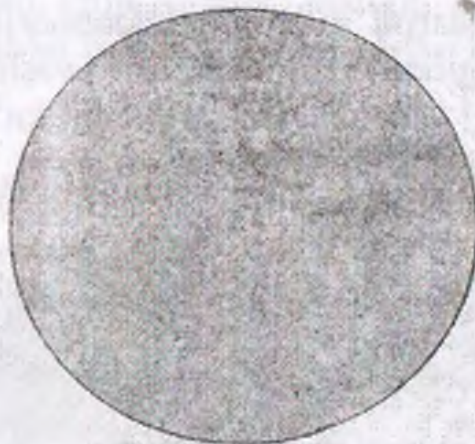
5.29-rasm. Mayin pelit strukturali va xol-xol mikroteksturali gil. Jins gidroslyudadan tashkil topgan ( < 0,001 mm). O'rta devon. Leningrad obl. M.F Vikulova koll. A.S Dyorin chizgan. Nikol 1.
