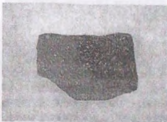
4.51-rasm. Kvarsli porfir.
