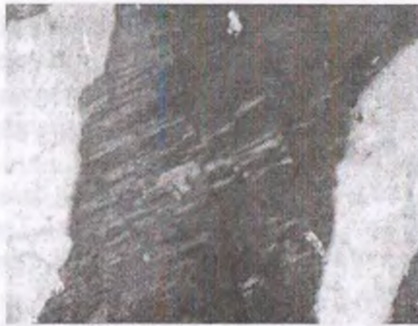
4.28-rasm. Pegmatitli struktura. Nikollar +
