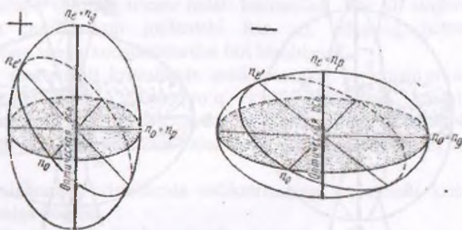
1.5-rasm. Bir o'qli kristallarning musbat (+) va manfiy (-) optik indikatrisoni.
