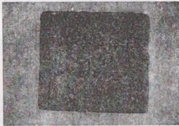
4.7-rasm. O'рта donali struktura.
