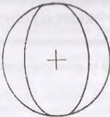
1.2 - rasm. Geksagonal singoniyali mineralda nurning tarqalish sirti.
