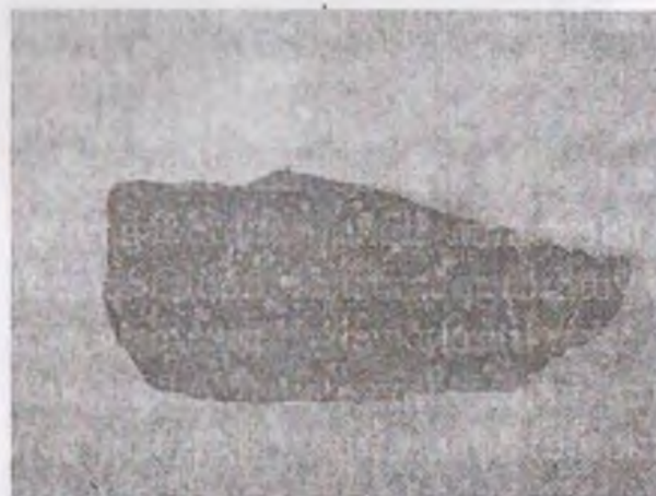
4.40-rasm. Granodiorit porfir.
