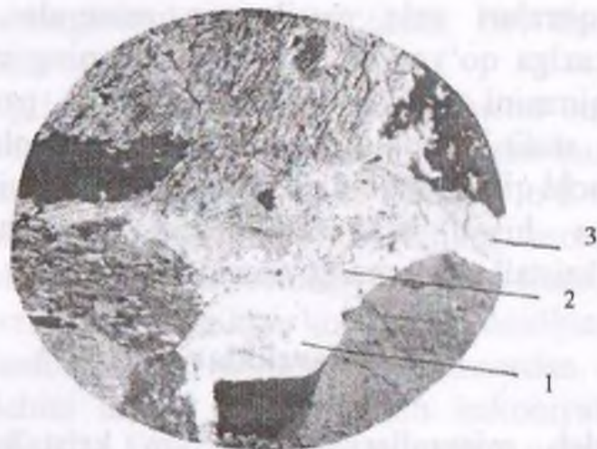
2.1- rasm. Minerall donalarining shakli: 1 – idiomorf; 2 – gipidiomorf; 3 – ksenomorf.
