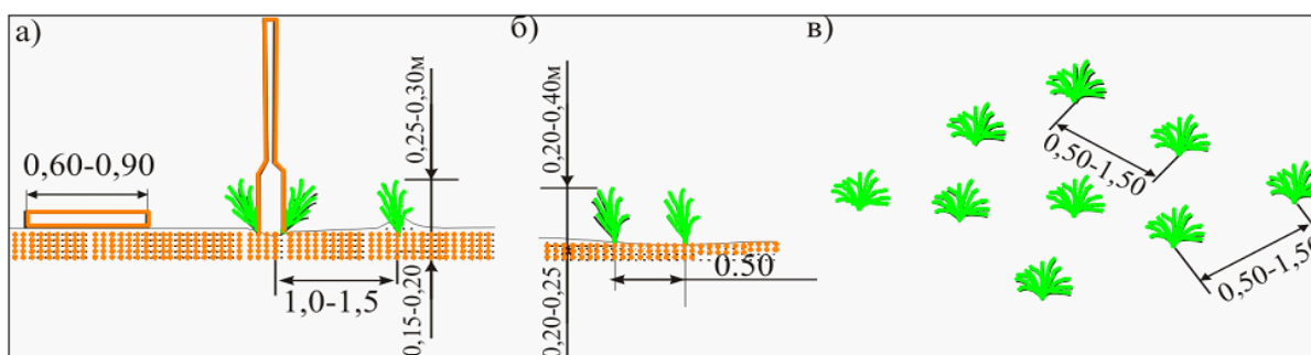
2.11 – rasm. Siqiluvchan va tik o‘sovchi himoya. a – siqiluvchan himoyalarni o‘rnatish ketma-ketligi; b – tebranuvchi himoyani o‘rnatish; v – bog‘lamlarni joylashishi.
