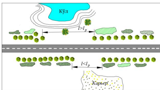
1.12 – rasm. Yo‘ldagi ekinlarning uzilgan joyi kengligini aniqlashga misol.
