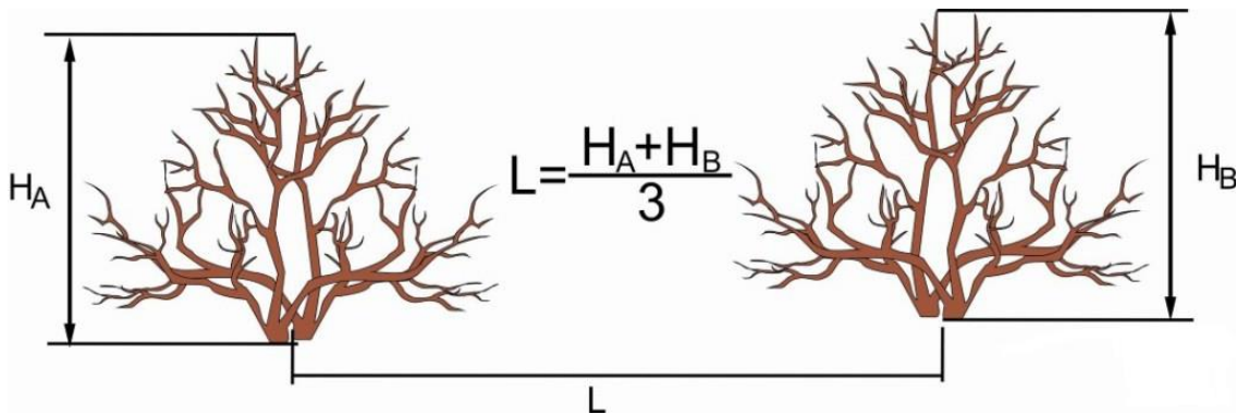
Butalarni ekish joylarini oralig'ini hisoblash
