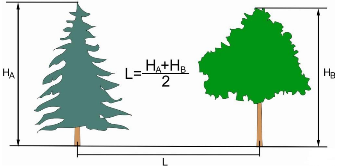
Daraxtlarni ekish joylarini oralig'ini hisoblash (tik kolonna shaklda o'sadigan daraxtlardan tashqari)
