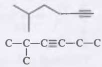
2-metilgeksin-3
