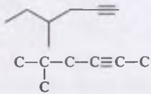
5-metilgeksin-2
