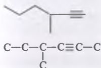
4-metilgeksin-2
