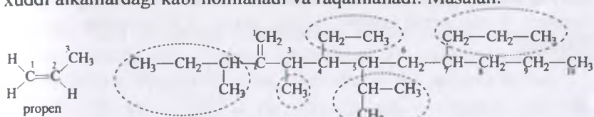
2-ikkilamchibutil-3-metil-5-izopropil-7-propil-4-etildetsen-1
