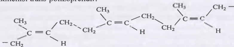
trans-polizopren
