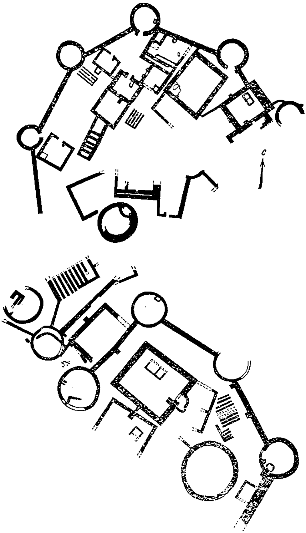
28-расм. Жанубий Туркманистондаги энеолит даври маконларининг плани (Муллалитепа, Ялонгочтепа)
