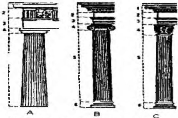
60-rasm. Me'morchilik uslublari: A-doriy; B-ioniy; C-korinf.
