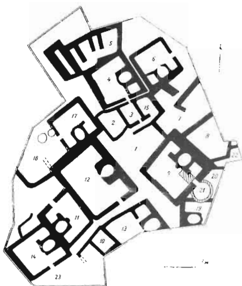
10-расм. Чағаллитепа. Неолит даври уй-жойларининг тузилиши.
