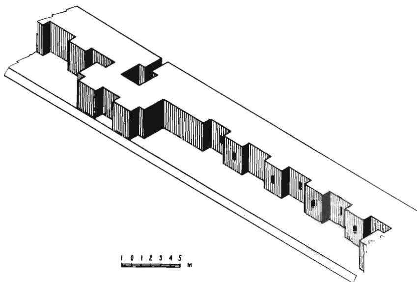
41-расм. Узунқир мудофаа деворлари (тикланган).
