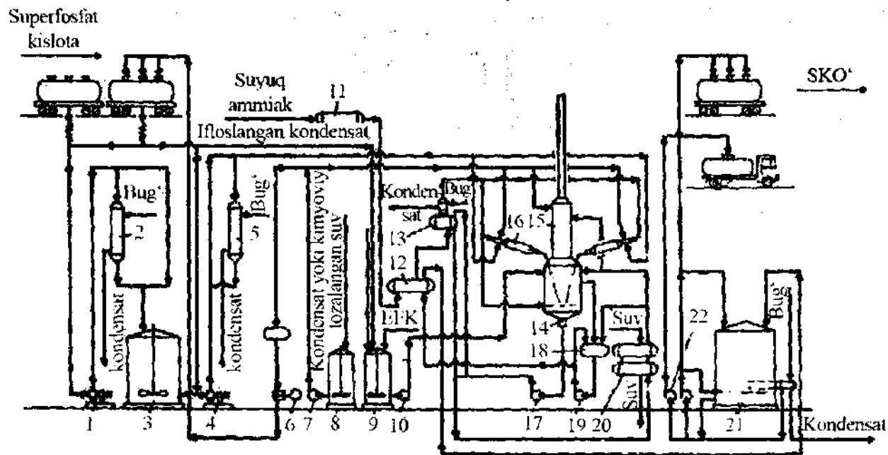
5.11-rasm. Polifosfat kislotalar asosida suyuq kompleks o'g'itlar ishlab chiqarish sxemasi:
