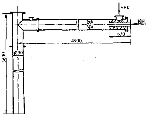
5.13- rasm. SFKni ammoniyash uchun quvurli reaktor sxemasi.
