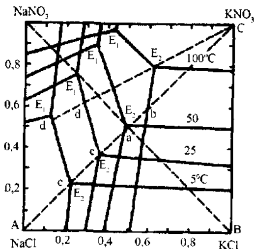
2.1- rasm. 5, 25, 50 va 100^\circ C haroratdagi KCl + NaNO_3 = NaCl + KNO_3 suvli sistemasida eruvchanlik izotermasi.
