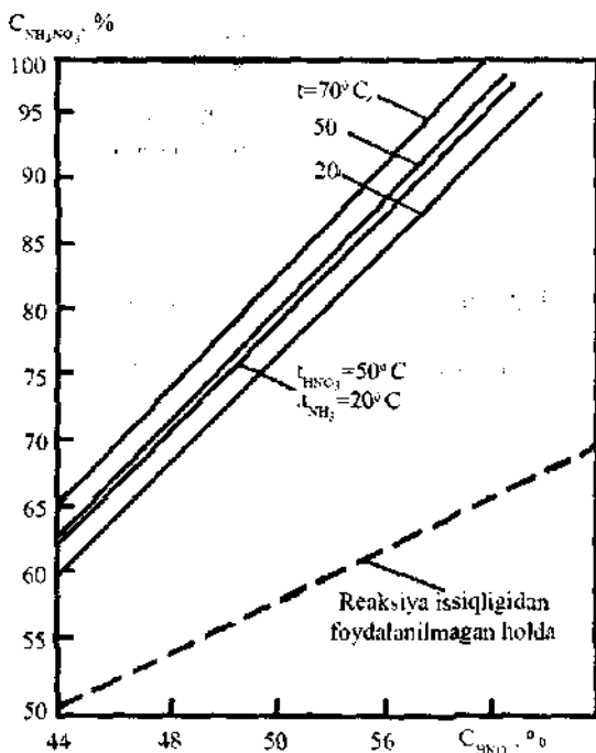
4.3-rasm. Reaksiya issiqligidan foydalanilganda olinadigan \text{NH}_4\text{NO}_3 eritmasi konsentratsiyasining reagentlar harorati turlicha bo'lganda nitrat kislota konsentratsiyasiga bog'liqligi (issiqlik yo'qotilishi 3% atrofida deb olinadi).
