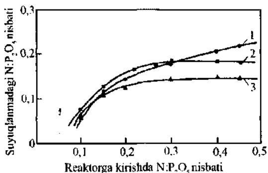
5.6- rasm. Reaktorga kirishdagi ammiak va fosfat kislota nisbatining suyuqlanmadagi N:P 2 O 5 nisbatiga ta'siri: boshlang'ich kislota konsentratsiyasi: 1 – 53,2; 2 – 62,5; 3 – 69,2.
