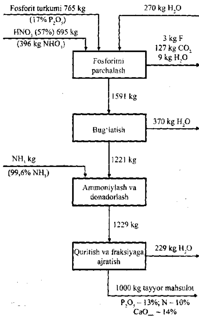
3.22- rasm. Nitrokalsiyfosfat ishlab chiqarish moddiy balansi.
