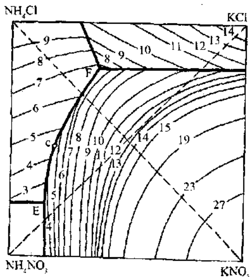
2.3- rasm. \text{KCl}-\text{NH}_4\text{NO}_3-\text{KNO}_3-\text{NH}_4\text{Cl} sistema izotermasi ( 0^\circ\text{C} ).
