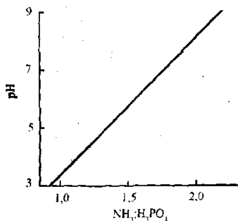
3.4- rasm. 65–75°C haroratdagi ammoniy fosfatlar to'yingan eritmaları pH qiymatining \text{NH}_3:\text{H}_3\text{PO}_4 molar nisbatiga bog'liqligi.
