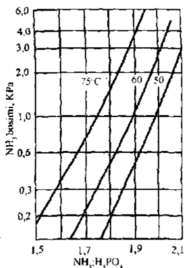
3.3- rasm. Ammoniy fosfatlar to'yingan suvli eritmaları ustidagi ammiak bosimining \text{NH}_3:\text{H}_3\text{PO}_4 molar nisbatiga bog'liqligi.
