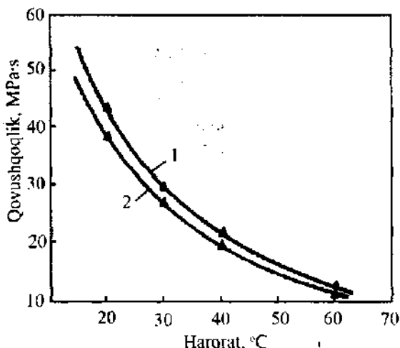
5.2- rasm. SKO' qovushqoqligining haroratga bog'liqligi, P_2O_5 konversiya darajasi: 1 – 56,9%; 2 – 68,7%.
