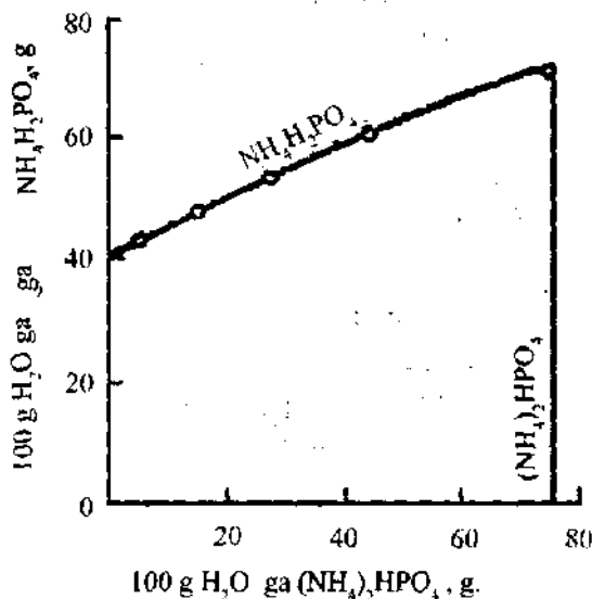
3.2-rasm. 25°C haroratdagi NH_4H_2PO_4 - (NH_4)_2HPO_4 - H_2O sistemadagi eruvchanlik izotermasi.
