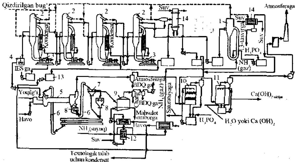
3.7- rasm. Ammofos suspensiyasini bug'latish va BDQ jihazida donadorlash orqali ammofos ishlab chiqarish sxemasi:
