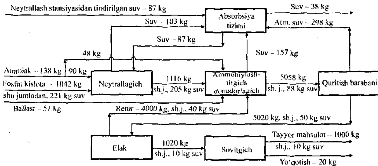
3.12-rasm. Ammofos ishlab chiqarish moddiy balansi.
