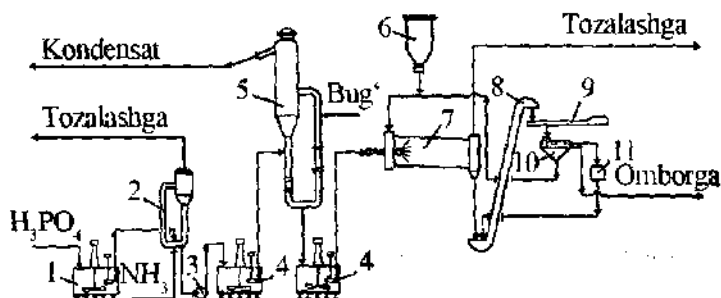
4.7- rasm. Karboammofos olish texnologik sxemasi:
