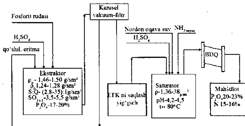
3.17- rasm. Ammoniy sulfatfosfat o'g'iti ishlab chiqarishning prinsipl texnologik sxemasi.
