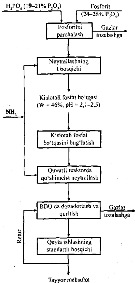
3.13-rasm. Ammofosfat ishlab chiqarish blok-sxemasi
