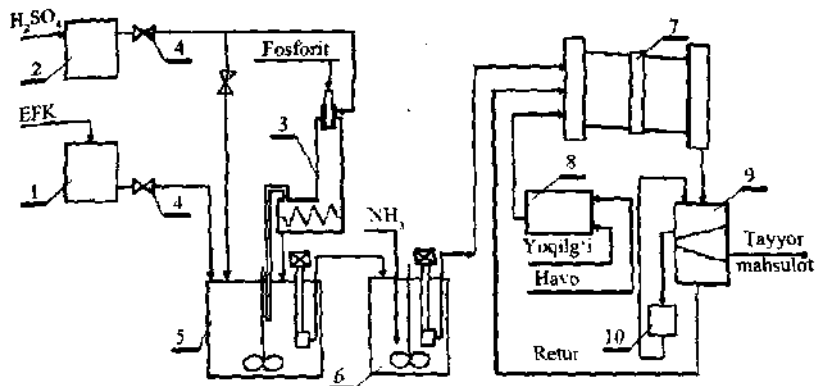
3.24-rasm. PS-Agro o'g'itini ishlab chiqarish texnologiyasining printsiplal sxemasi:
