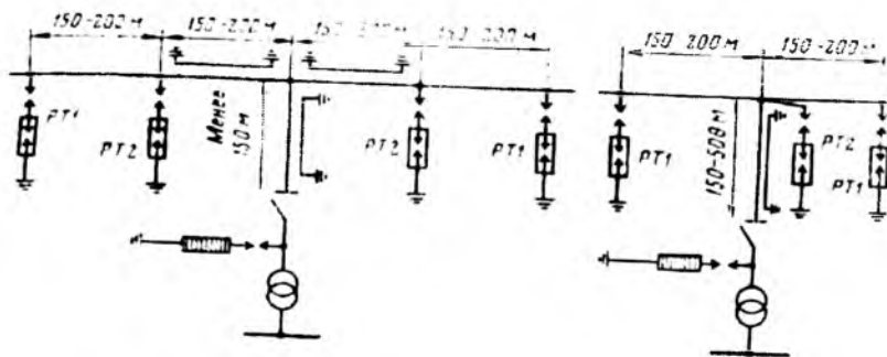
Рис. 4.2.18. Схемы защиты от грозовых перенапряжений ПС, присоединенных к ВЛ ответвлениями длиной до 150 и более 150 м.
