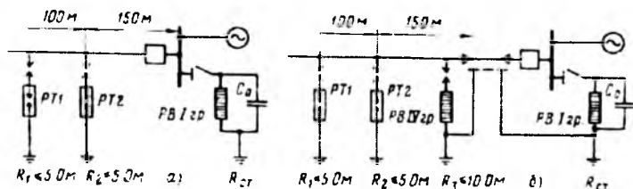
Рис. 4.2.21. Схемы защиты электродвигателей мощностью до 3 МВт: при подходе ВЛ на деревянных опорах
