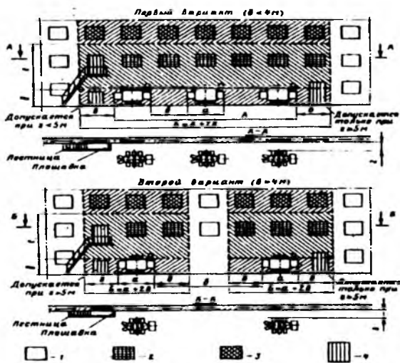
Рис. 4.2.13. Требования к открытой установке маслонаполненных трансформаторов у зданий с производствами категорий Г и Д (по противопожарным нормам)
