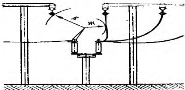
Рис. 4.2.11. Наименьшие расстояния от контактов и ножей разъединителей в отключенном положении до заземленных и токоведущих частей.
