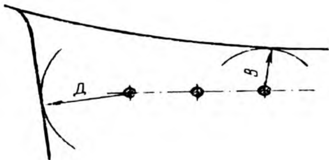
Рис. 4.2.8. Наименьшие расстояния между токоведущими частями разных цепей, расположенных в различных плоскостях, с обслуживанием нижней цепи при неотключенной верхней.
