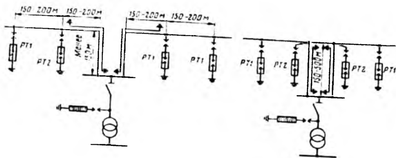
Рис. 4.2.19. Схемы защиты от грозовых перенапряжений ПС, присоединенных к ВЛ с помощью заходов длиной до 150 и более 150 м.
