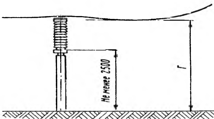
Рис. 4.2.6. Наименьшие расстояния от неогражденных токоведущих частей и от нижней кромки фарфора изоляторов до земли
