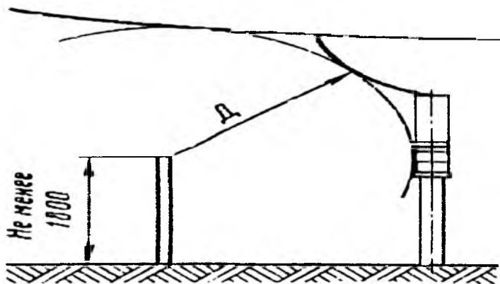
Рис. 4.2.10. Наименьшие расстояния от токоведущих частей до верхней кромки внешнего ограждения
