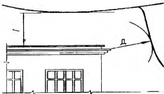
Рис. 4.2.12. Наименьшие расстояния между токоведущими частями и зданиями и сооружениями
