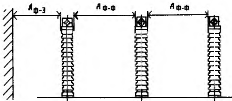
Рис. 4.2.3 Наименьшие расстояния в свету при жестких шинах между токоведущими и заземленными частями ( A_{\phi-з} ) и между токоведущими частями разных фаз ( A_{\phi-\phi} )
