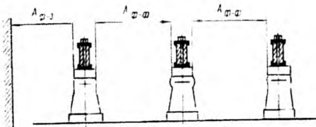
Рис. 4.2.14. Наименьшие расстояния в свету между неизолированными токоведущими частями разных фаз в ЗРУ и между ними и заземленными частями (по Таблице 4.2.8)
