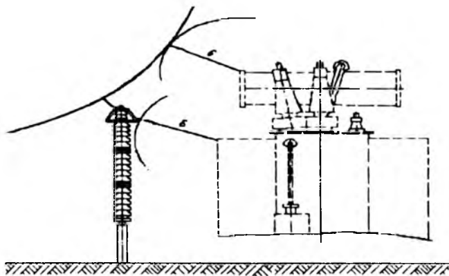
Рис. 4.2.7. Наименьшие расстояния от токоведущих частей до транспортируемого оборудования
