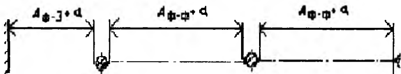
Рис. 4.2.4 Наименьшие расстояния в свету при гибких шинах между токоведущими и заземленными частями и между токоведущими частями разных фаз, расположенными в одной горизонтальной плоскости
