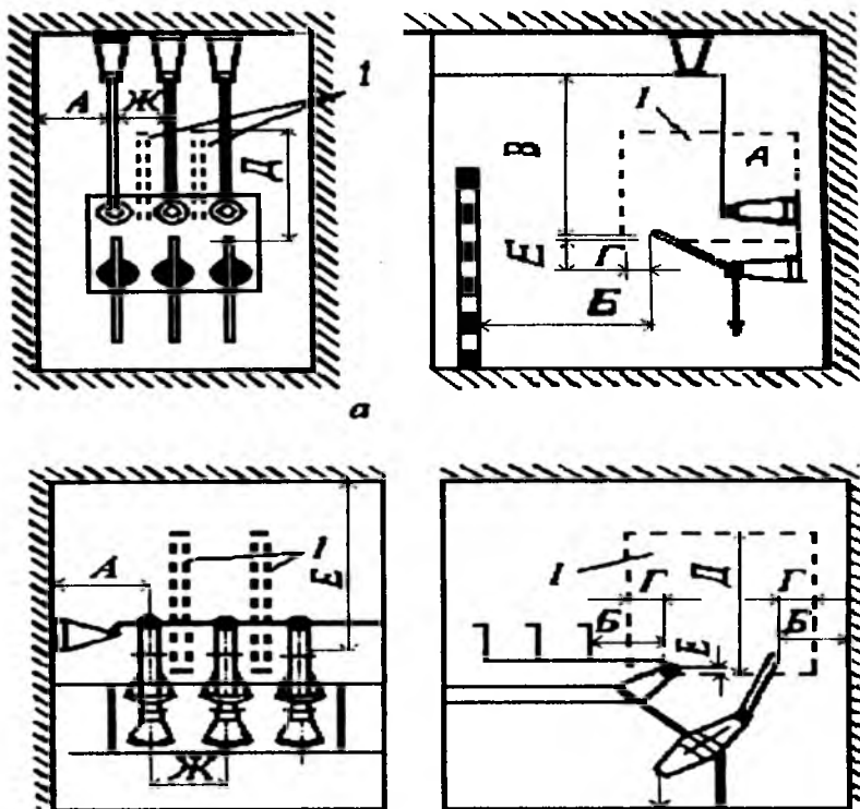
Рис. 4.2.2. Установка разъединителя (отделителя)
