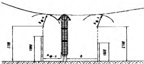
Рис. 4.2.5. Наименьшие расстояния от токоведущих частей и элементов изоляции, находящихся под напряжением, до постоянных внутренних ограждений
