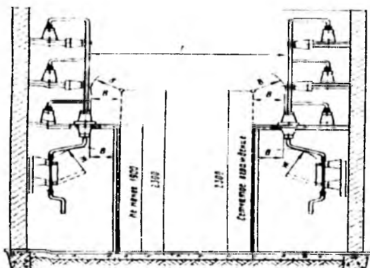
Рис 4 2 16. Наименьшие расстояния от неизолированных токоведущих частей в ЗРУ до сетчатых ограждений и между неогражденными неизолированными токоведущими частями разных цепей (по Таблице 4.2.8)
