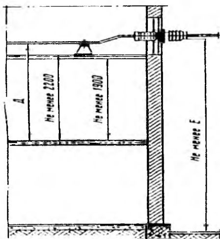
Рис 4 2 17. Наименьшие расстояния от пола до неогражденных неизолированных токоведущих частей и до нижней кромки фарфора изолятора и высота прохода в ЗРУ. Наименьшее расстояние от земли до неогражденных линейных выводов из ЗРУ вне территории ОРУ и при отсутствии проезда транспорта под выводами
