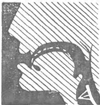
18-rasm. S, Z, tovushlari artikulatsiyasi profili.
