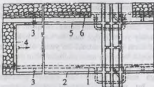
7.3-rasm. Stolbani maydon lahimlari yordamida tayyorlash: 1 - yuk tashuvchi maydon shtreki; 2 - qatlamli konveyerli shtrek; 3 - gezenk yoki oraliq qvershlag, 4 - lava; 5 - qatlamni shamollatuvchi shtrek; 6 — shamollatuvchi maydon shtreki.
