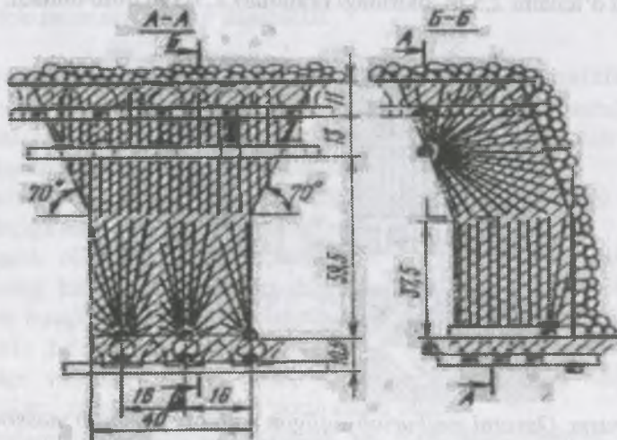
5.18-rasm. «Apatit» kombinatida qo'llaniladigan, qavatni majburan qulatilish varianti
