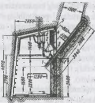
2.17-rasm. Ikki sektorli zatvor o'rnatilgan lyuk: 1-lyukning tagi (asosi); 2-lyukning zatvorlari; 3-lyukning borlari; 4-lyukning peshonasi; 5-rama va lyuk zatvorini ochib-yopuvchi yuritma
