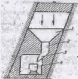
2.15-rasm. Rudani blokdan o‘z og‘irlik kuchi ta‘sirida tushirish sxemasi: 1-voronka; 2-ruda tushiruvchi lahim; 3-lyuk; 4-vagonetka.
