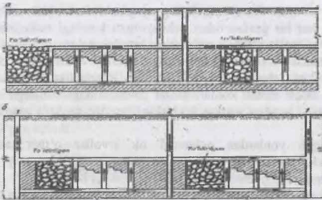
2.1-rasm. Markazlashtirilgan va diagonal shamollatish sxemalari: 1 - yordamchi stvol; 2 - bosh stvol.
