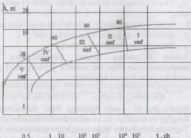
4.6-rasm. Kon lahimining ushlab turuvchi oralig'ining kattaligi uning ish vaqtiga bog'liqligi (I – V – tog' jinsi sinflari).
