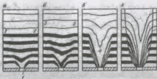
5.10-rasm. Rudani qulatilgan tog' jinslari ostidan chiqarishda harakatlanish sxemasi.
