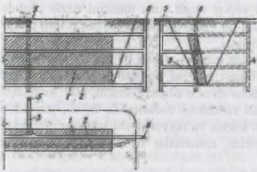
2.2-rasm. Vertikal stvollar bilan ochish sxemasi:
