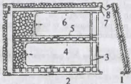
7.6-rasm. O'ta qiya qatlamlarda qavatni nimqavatlariga ajratib qaziydigan stolbali qazish tizimi: 1 - oraliq kvershlag, 2 — qatlamli yuk tashuvchi shtrek; 3 - sirpanma; 4 - oraliq shtrek; 5 - parallel shtrek; 6 - shamollatuvchi shtrek; 7 - shamollatuvchi tutashma; 8- shamollatuvchi kvershlag.
