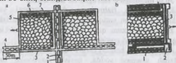
7.8-rasm. Lava-qavatli sidirg'asiga qazish tizimi: a — qavat shtreklarini saqlovchi butunliklar bilan muhofaza qilish va tashuvchi shtrek kavjoyini lavadan uzdirib o'tkazish sxemasi (1 — kapital bremsberg, 2 — ishchilar yo'lagi; 3 — qavat tashuvchi shtreki; 4 — prosek; 5 — lava; 6 — qavat shamollatuvchi shtreki; 7 — qulatilgan kesuvchi pechi; b — qavat shtreklarini toshdevorlar bilan muhofaza qilish va tashuvchi shtrekn lavadan kechiktirib o'tqazish sxemasi (1 — qavat tashuvchi shtreki; 2 - raskoska; 3 - lava; 4 - qavat shamollatuvchi shtreki).
