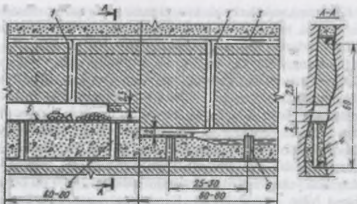
6.6-rasm. Gorizontl qatlamlab gidroto'ldirgich materiallar qo'llab, yuzasini beton bilan qoplab qazish tizimi: 1-blok vosstayushiysi, 2-ikki bo'limdan iborat ruda tushirish va kishilar harakatlanishiga xizmat qiluvchi vosstayushiy, 3-suyuq to'ldiruvchi materiallarni yetkazib beruvchi quvur, 4-gidro to'ldirgich, 5-beton to'shama, 6-drenaj quvuri.
