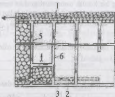
7.4-rasm. Yakka lavalalar bilan ko'tarilish yo'nalishi bo'yicha uzun stolbali qazish tizimi: 1 va 2 - bosh yuk tashuvchi va shamollatuvchi maydon shtreklari; 3 - prosek; 4 va 5 - konveyerli va shamollatuvchi uklonlar.
