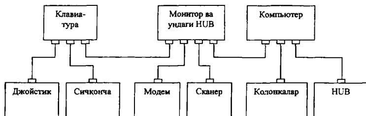
12.10-расм. Ташқи қурилманинг USB тармоққа уланишга мисол.
