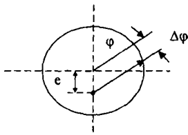
5.2-расм. Секундомер стрелкаси ўқининг эксцентриситетига боғлиқ хато: e – стрелканинг шкала марказига нисбатан кўчиши (эксцентриситет); \phi – стрелканинг бурилиш бурчаги.
