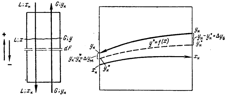
Рис. X-8. К определению средней движущей силы процесса массопередачи.
