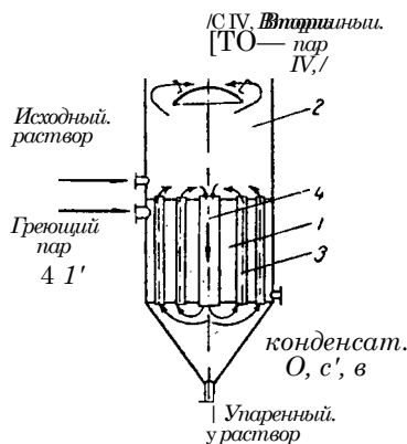
Рис. 1X-1. Схема устройства одиночного (однокорпусного) выпарного аппарата:
