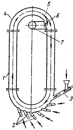
Рис. XVШ1-18. Схема струйной мельницы с трубчатой помольной камерой:
