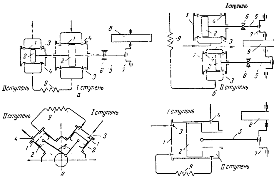
Рис. 1У-6. Схема многоступенчатых поршневых компрессоров:
