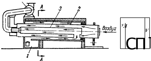
Рис. XV-34. Барабанная контактная сушилка:
