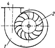
Рис. IV-11. Схема вентилятора низкого давления:
