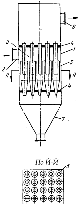
Рис. \M1. Батарейный циклон:
