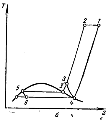
Рис. XVII-18. Соединенные циклы низкого давления — дроссельный и детандерный (регенеративный):
