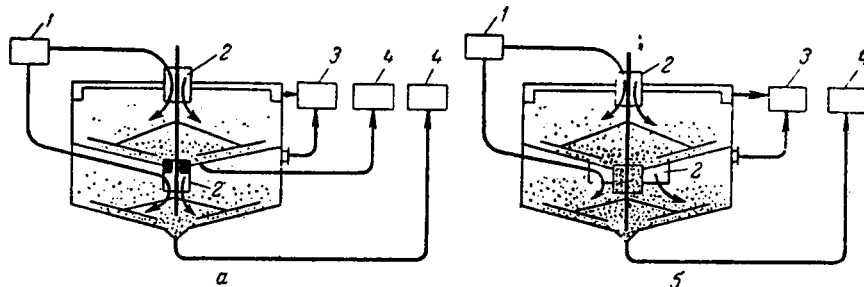
Рис. У-6. Многоярусные отстойники закрытого (а) и сбалансированного (б) типов:
