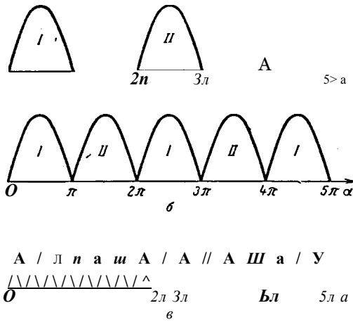
Рис. 111-15. Диаграммы подачи поршневых насосов:
