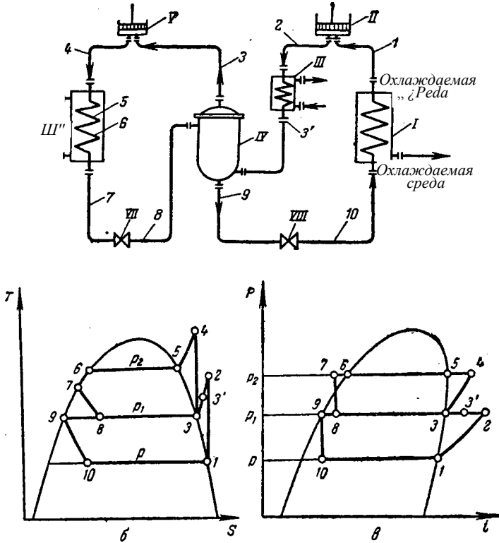
Рис. XVII-8. Двухступенчатая компрессионная холодильная машина.
