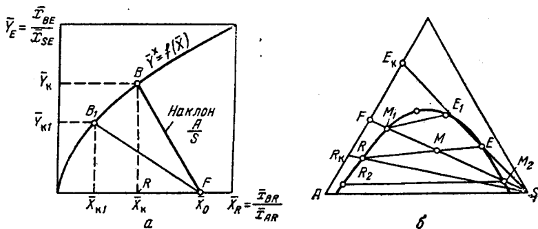
Рис. XIII-9. Изображение процесса одноступенчатой экстракции:
