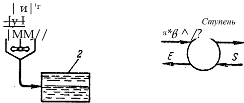
Рис. XIII-8. Схема одноступенчатой экстракции:
