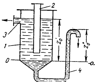
Рис. 11-5. К определению высоты гидравлического затвора в непрерывно действующем жидкостном сепараторе.
