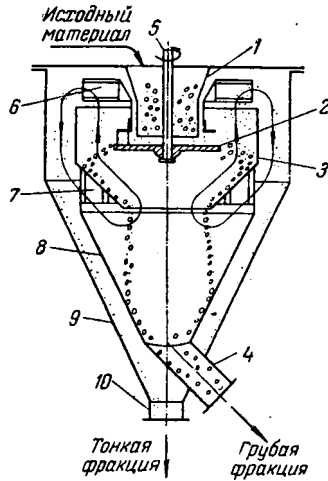
Рис. XIX-9. Схема воздушно-циркуляционного сепаратора:
