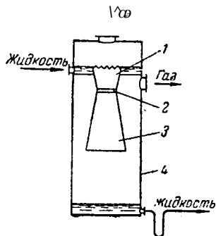
Рис. X1-29. Распыливающий абсорбер Вентури:
