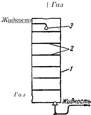
Рис. XI-25. Колонна с тарелками без сливных устройств:
