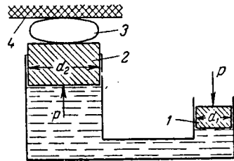
Рис. П-7. Схема гидравлического пресса.
