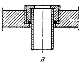
Рис. VI П-23. Закрепление труб в трубных решетках:
