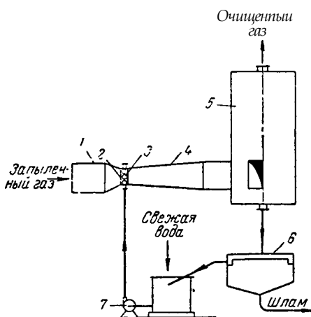
Рис. \M8. Схема скруббера Вентури;
