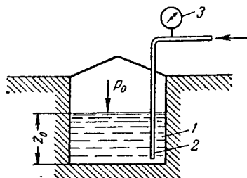
Рис. 11-6. Пневматический измеритель уровня жидкости.
