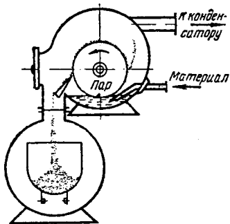
Рис. XV-32. Одновальцовая сушилка.
