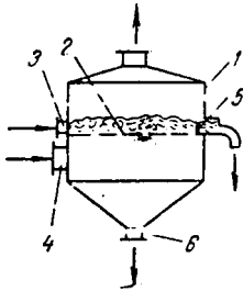
Рис. У-49. Барботажный (пенный) пылеуловитель:
