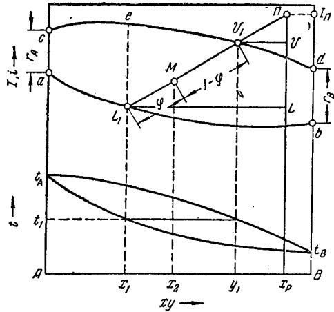
Рис. XI-26. Расчет ректификации бинарных смесей с помощью диаграмм t-x-y (сверху) и t-x-y (снизу).
