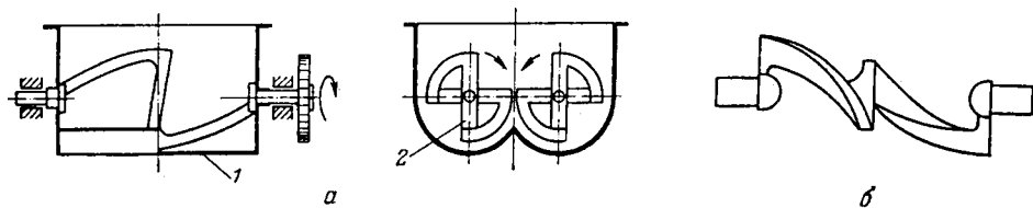
Рис. XX-2. Схема двухвального смесителя:
