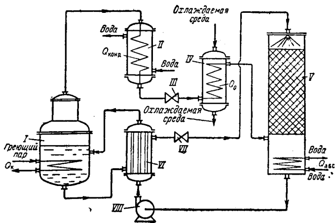
Рис. XVII-10. Схема водноаммиачной абсорбционной холодильной машины.
