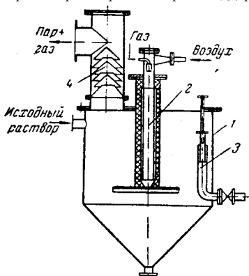
Рис. IX-20. Выпарной аппарат с погружной горелкой:
