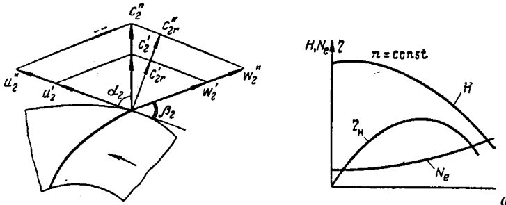
Рис. Ш-5. Подобие параллелограммов скоростей при изменении числа оборотов колеса от n до n' . Рис. Ш-6. Характеристика центробежного насоса,
