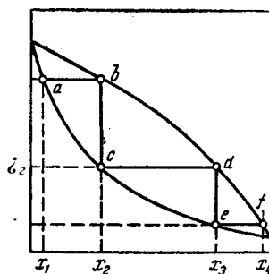
Рис. XII-13. Изображе- ние би^рной^шеси^Тутем ректификации на диа- грамме <—x—y.
