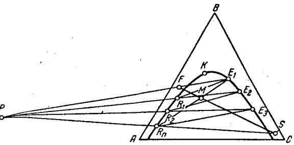
Рис. XIII-13. Определение числа теоретических ступеней при противоточной многоступенчатой экстракции.
