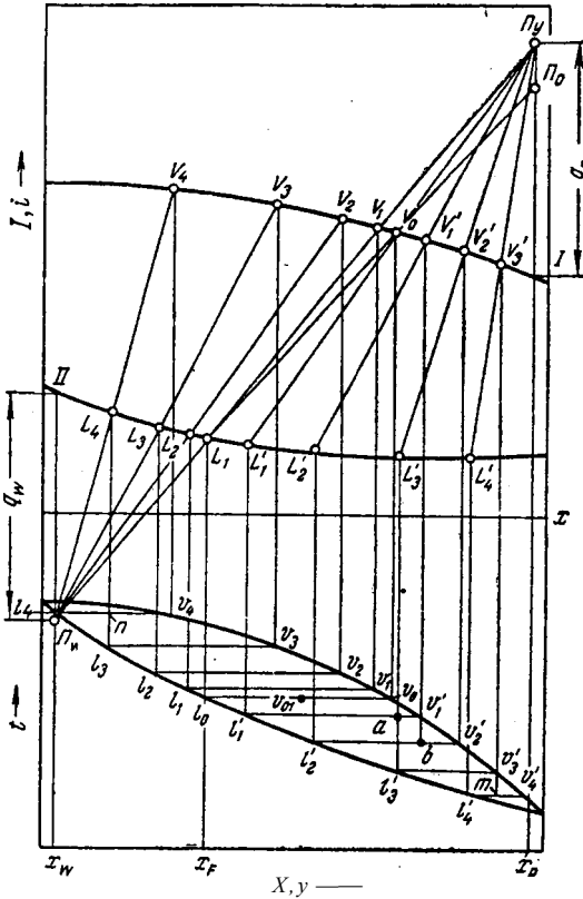
Рис. XII-27. К расчету ректификационной колонны с помощью энтальпийной диаграммы.
