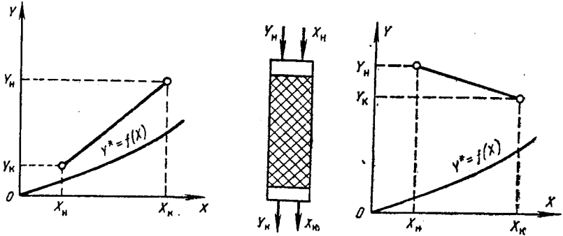
Рис. X1-31. Схема противоточной абсорбции. Рис. X1-32. Схема проточной абсорбции.
