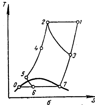
Рис. XIII-17. Соединенные циклы дроссельный и детандерный без регенерации:
