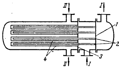
Рис. VIII-15. Кожухотрубчатый теплообменник с двойными трубами:
