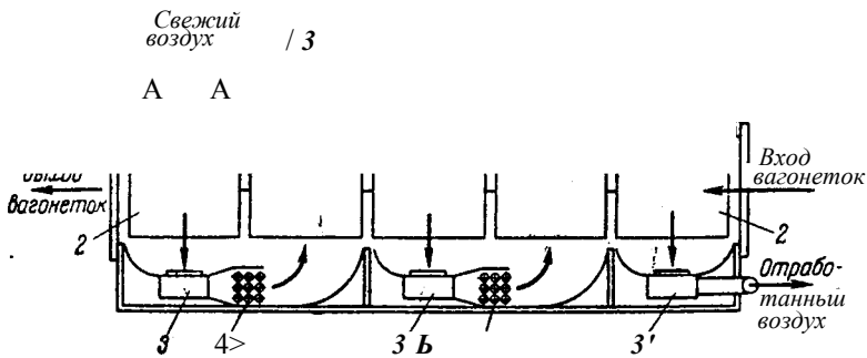
Рис. ХУ-19. Туннельная сушилка:
