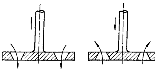
Рис. У1-13. Устройство дисков вибрационных мешалок.
