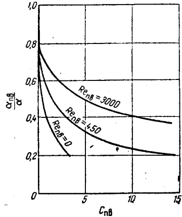
Рис. УН-13. Влияние примеси воздуха на относительный коэффициент теплоотдачи для водяного пара при p = 0,8 бар, M = 10 °С.
