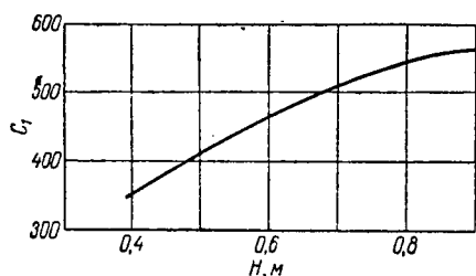
Рис. X1-17. К определению предельной скорости газа в абсорбере с ситчатыми тарелками.
