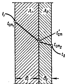
Рис. 15 к выводу уравнения теплопередачи через плоскую стенку.
