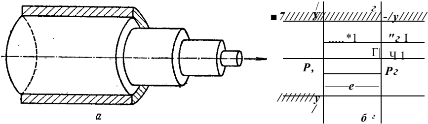
Рис. П-9. К определению распределения скоростей и расхода жидкости при ламинарном движении.
