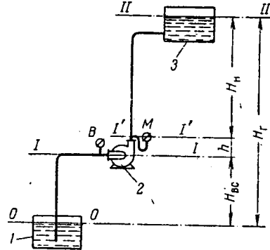
Рис. 111-1. Схема насосной установки:
