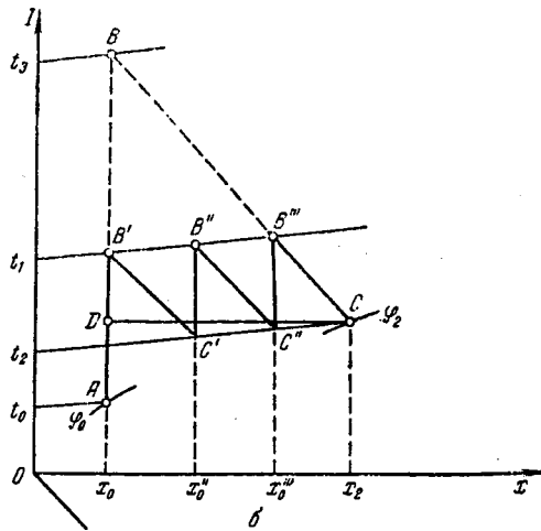
Рис. ХУ-9. Сушилка с промежуточным подогревом воздуха по зонам:
