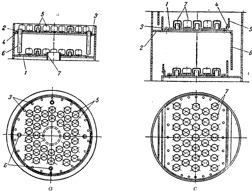
Рис. X1-21. Колпачковая тарелка с различными переливами жидкости: а — радиальный перелив; 1 — диск; 2 — прокладка; 3 — болты; 4 — опорное кольцо; 5 — колпачки; 6 — периферийные переливные трубки; 7 — спиральная сливная трубка; б — диаметральный перелив; 1 — диск; 2 — опорный лист; 3 — приемный порог; 4 — сливной порог; 5 — сменная гребенка; 6 — перегородка; 7 — колпачки.
