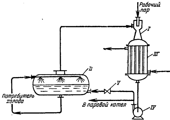
Рис. XVII-1. Принципиальная схема пароводяной эжекторной холодильной машины:
