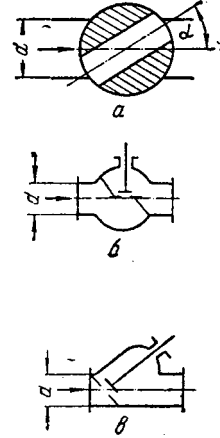
Рис. 11-25. Некоторые запорно-регулирующие устройства: а — пробковый кран; б — стандартный вентиль; в — прямоугольный вентиль с наклонным шпинделем.
