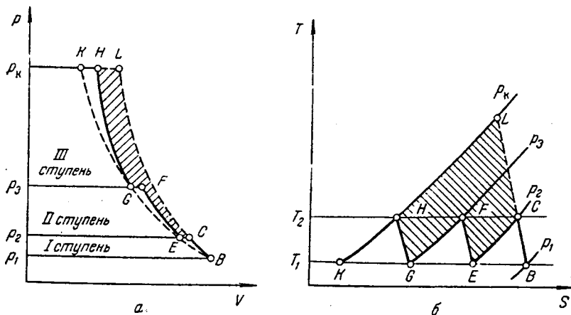
Рис. 1У-7. Индикаторная (а) и энтропийная (б) диаграммы многоступенчатого сжатия газа.
