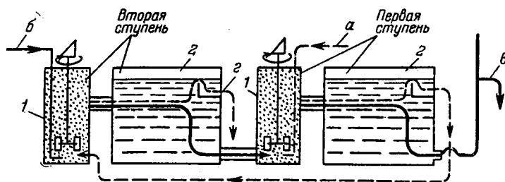
Рис. ХШ-17. Схема смесительно-отстойного экстрактора:
