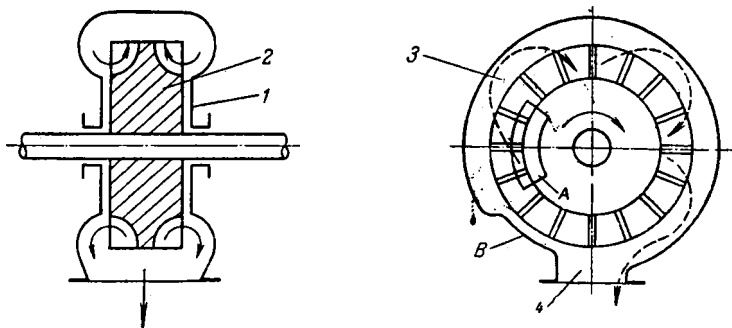
Рис. Ш-23. Схема вихревого насоса;
