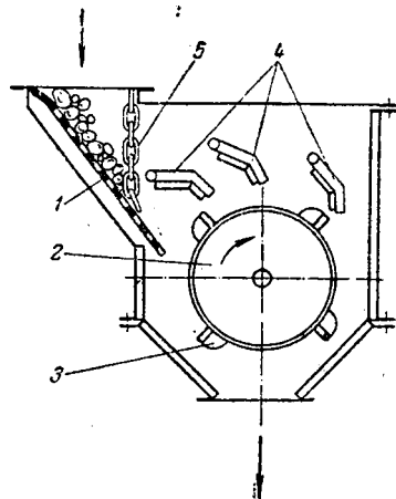
Рис. XVIII-10. Схема отражательной дробилки:
