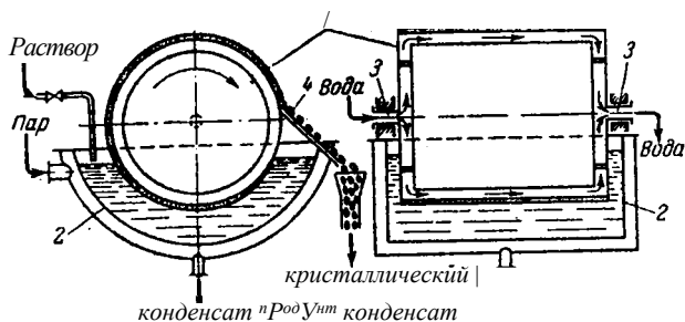
Рис. XVI-9. Вальцовый кристаллизатор:
