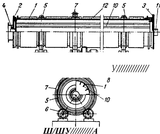
Рис. XIII-32. Барабанный-экстрактор:
