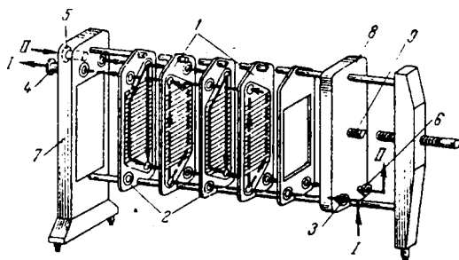
Рис. УП-19. Схема пластинчатого теплообменника:
