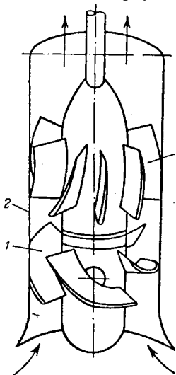
Рис. Ш-22. Схема пропеллерного насоса:
