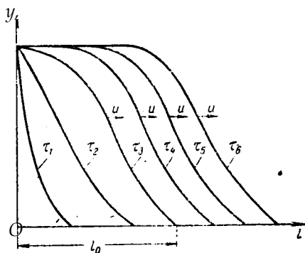
Рис. X1Y-2. Изменение фронта адсорбции во времени.
