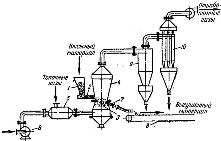
Рис. ХУ-24. Однокамерная сушилка с кипящим слоем:
