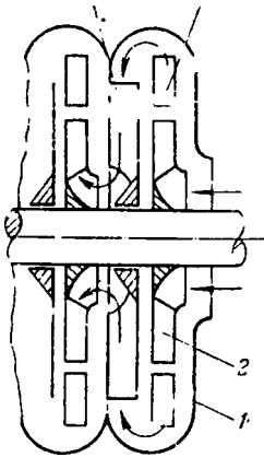
Рис. IV-13. Схема многоступенчатой турбогазодувки:
