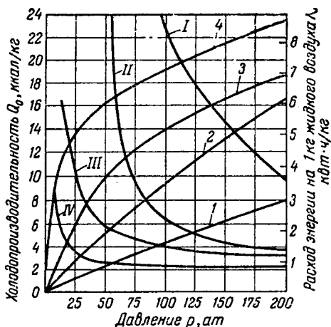
Рис. XVII-22. Сравнительная характеристика основных холодильных циклов при получении жидкого воздуха
