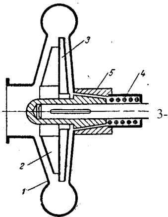
Рис. 111-19. Схема бессальникового насоса:
