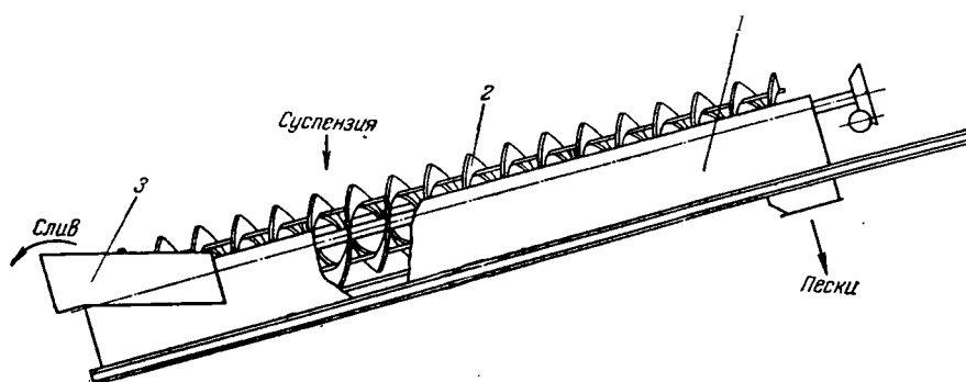
Рис. XIX-6. Схема спирального-классификатора:
