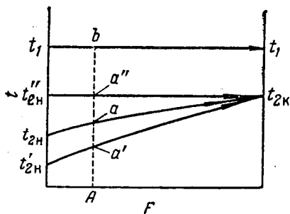
Рис. УП-19. Влияние перемешивания на среднюю движущую силу процесса теплообмена.
