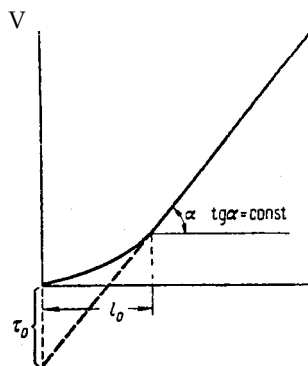
Рис. X1Y-3. Зависимость времени защитного действия от длины слоя поглотителя.
