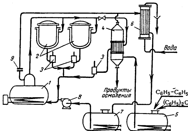
Рис. VIII-7. Схема обогрева парама ВОТ:
