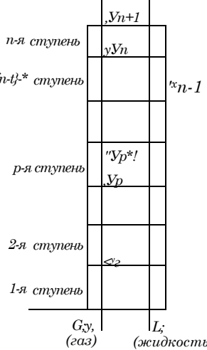
Рис. X-13. Схема противоточного «ступенчатого» массообменного аппарата.
