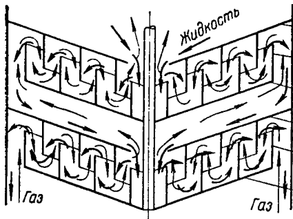
Рис. XI-30. Роторный центробежный абсорбер:
