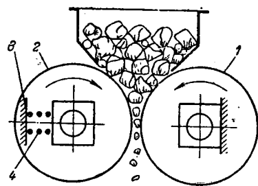
Рис. XVIII-7. Схема валковой дробилки:
