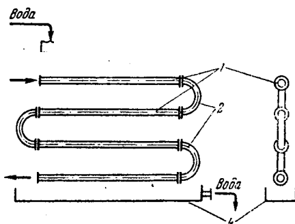
Рис. VIII-18. Оросительный теплообменник:
