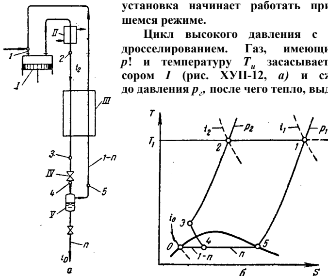
Рис. ХУП-12. Регенеративный цикл высокого давления с однократным дросселированием:
