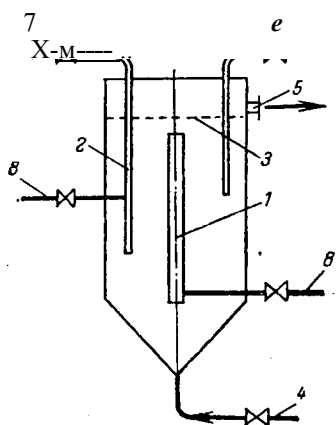
Рис. ХУ1-13. Ионообменная колонна с пневматическим перемешиванием:
