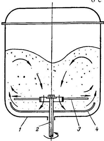
Рис. XX-6. Схема смесителя с псевдооживлением материала вращающимся ротором:
