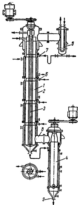
Рис. ХН-24. Схема роторно-пленочной ректификационной колонны:
