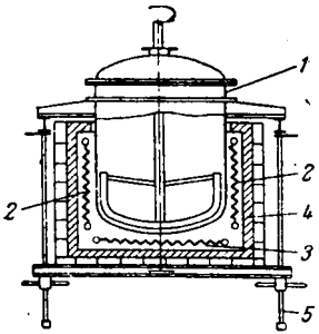
Рис. УП1-9. Электропечь сопротивления:
