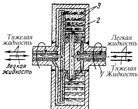
Рис. XII-25. Схема устройства центробежного экстрактора:
