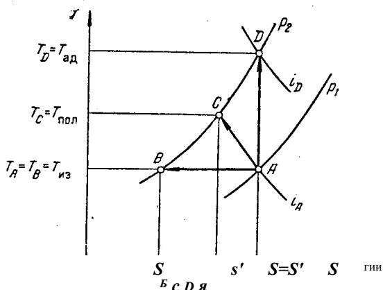
Рис. IV-2. Изображение процессов сжатия газа К и П р о ц е с с на T-S -диаграмме.
