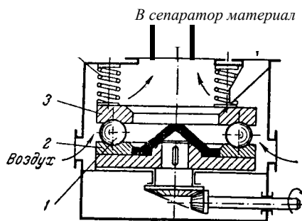
Рис. ХУШ-15. Схема шаровой кольцевой мельницы:
