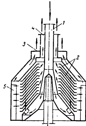
Рис. У-34. Жидкостный сепаратор тарельчатого типа:
