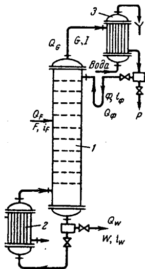
Рис. XII-20. К составлению теплового баланса непрерывно действующей ректификационной колонны:
