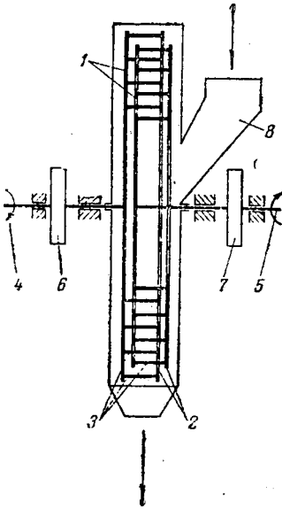
Рис. XV111-9. Схема дезинтегратора:
