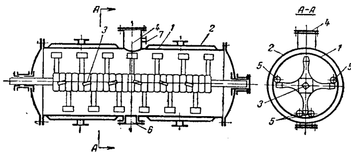
Рис. ХУ-30. Гребковая вакуум-сушилка:
