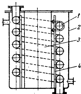
Рис. УШ-17. Змеевиковый теплообменник:
