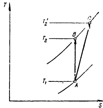
Рис. 1У-14. Энтропийная диаграмма сжатия газа в турбогазодувке.
