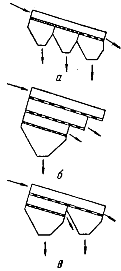
Рис. XIX-1. Способы грохождения:
