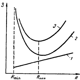
Рис. XII-18. К определению действительного (оптимального) флегмового числа:
