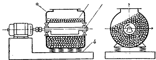
Рис. XVI П-16. Схема вибрационной мельницы инерционного типа:
