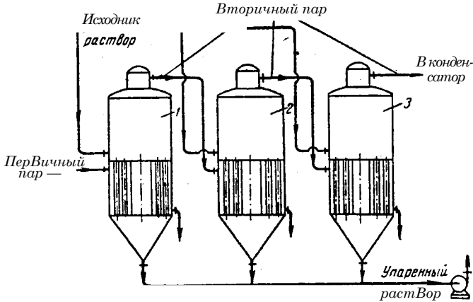
Рис. 1X-4. Многокорпусная выпарная установка с параллельным питанием корпусов (1—3).
