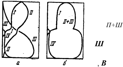
Рис. XII-29. Действительное (а) и приближенное (б, в) распределение концентраций компонентов I—IV по высоте колонны.
