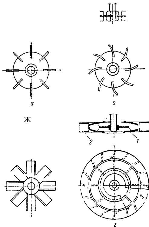
Рис. \П-10. Турбинные мешалки:
