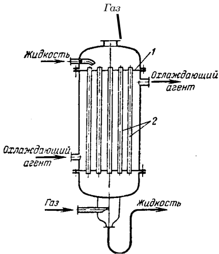
Рис. XI-9. Трубчатый абсорбер:
