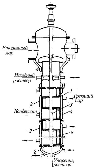
Рис. IX-16. Роторный прямоточный выпарной аппарат:
