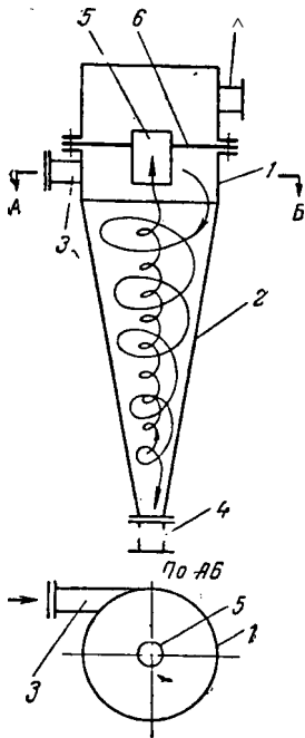
Рис. У-37. Гидроциклон:
