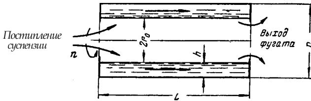
Рис. У-27. Схема действия отстойной центрифуги.
