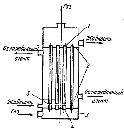
Рис. X1-11. Абсорбер с восходящим движением жидкой пленки:
