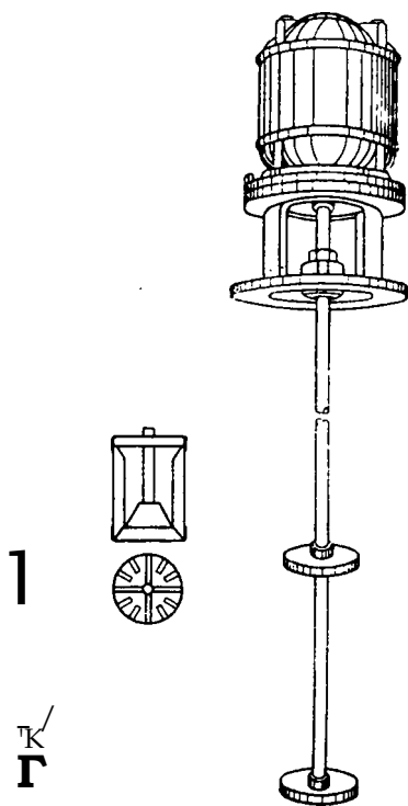
Рис. У1-11. Барабанная мешалка.
