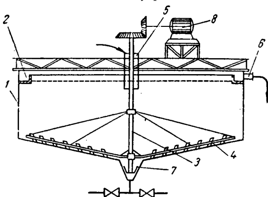
Рис. У-4. Отстойник непрерывного действия с гребковой мешалкой:
