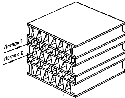
Рис. VIII-23. Схема устройства пластиночато-ребристого теплообменника.
