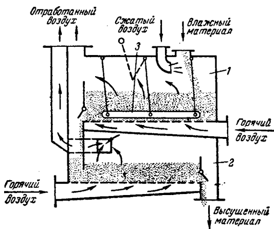
Рис. ХУ-25. Двухкамерная сушилка с кипящим слоем: 1 — верхняя камера; 2 — нижняя камера; 3 — раз* рыхлитель.
