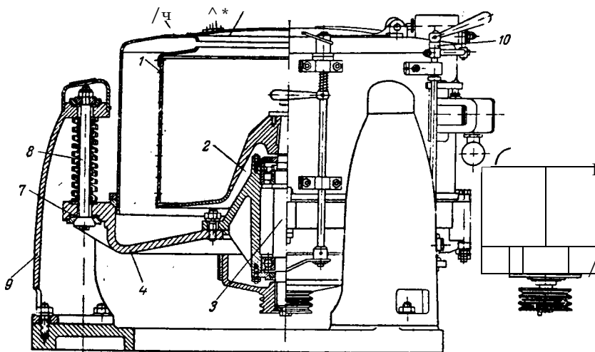
Рис. У-28. Трехколонная центрифуга:
