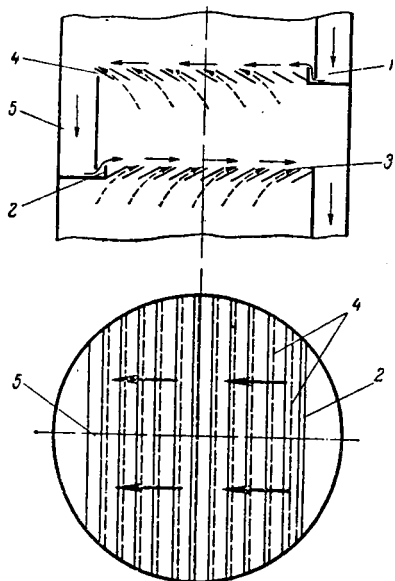
Рис. X1-24. Пластинчатая тарелка:
