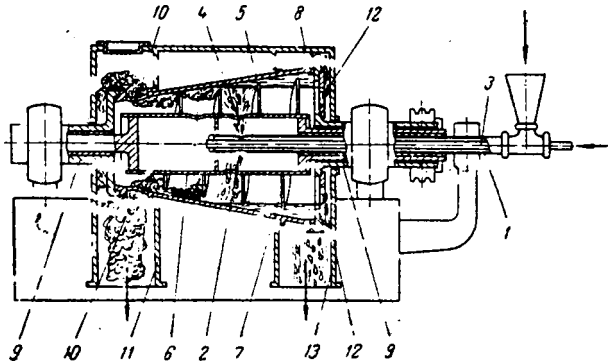
Рис. У-32. Центрифуга со шнековым устройством для выгрузки осадка:
