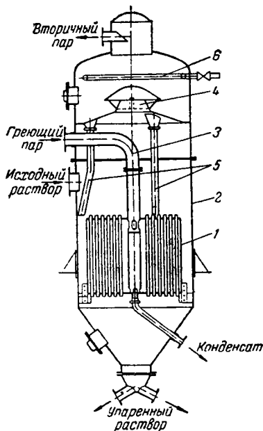
Рис. 1X-10. Выпарной аппарат с подвесной нагревательной камерой:
