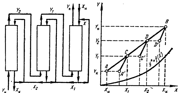
Рис. XI-34. Схема многоступенчатой противоточной абсорбции с рециркулирующей жидкостью в каждом абсорбере.
