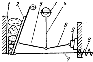
Рис. XVIII-3. Схема щековой дробилки с верхним подвесом щеки
