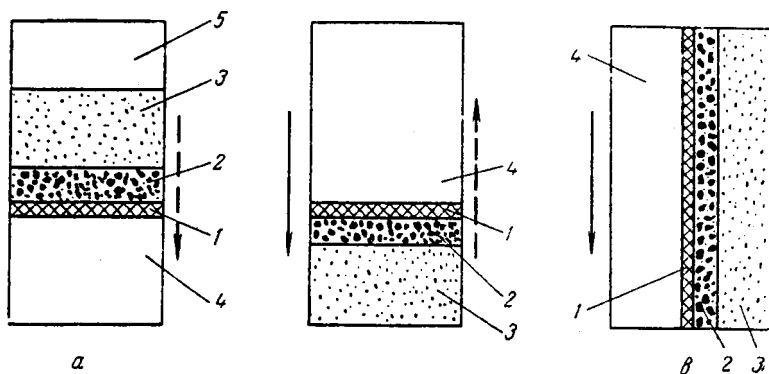
Рис. У-Ю. Взаимные направления действия силы тяжести и движения фильтрата в фильтрах:
