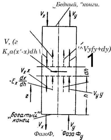
Рис. X-12. К составлению материального баланса массообменного аппарата с учетом обратного перемешивания.
