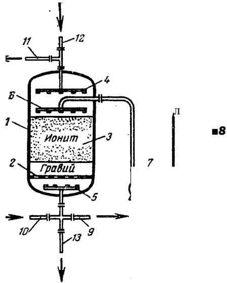
Рис. XIV-12. Схема ионообменной установки периодического действия:
