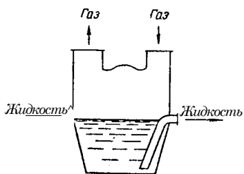
Рис. X1-6. Поверхностный абсорбер.
