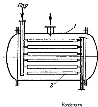
Рис. XV-29. Вакуум-сушильный шкаф:
