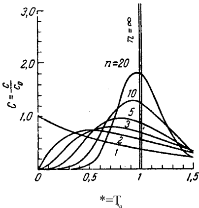
Рис. П-38. К ячеечной модели структуры потока:
