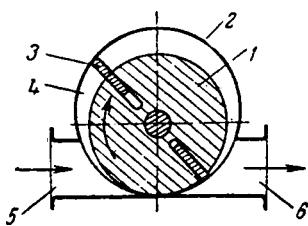
Рис. Ш-27. Схема пластинчатого ротационного насоса:
