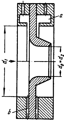
Рис. П-18. Мерное сопло.
