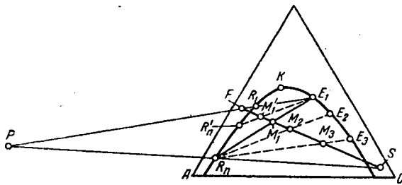
Рис. XIII-14. К определению удельного расхода экстрагента.
