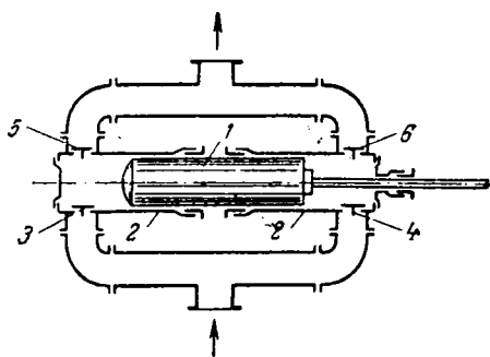
Рис. Ш-12. Схема горизонтального плунжерного насоса двойного действия:
