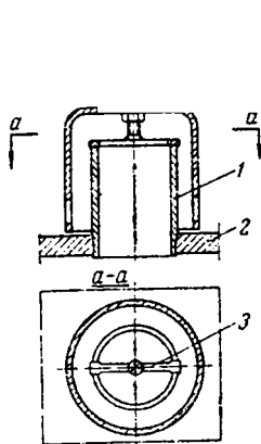
Рис. XI-22. Устройство капсульного колпачка:
