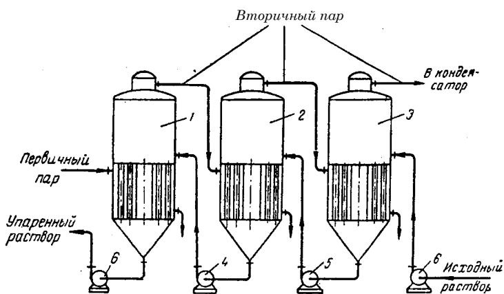
Рис. 1X-3. Многокорпусная противоточная выпарная установка:
