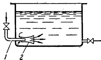
Рис. VIII-3. Бесшумный сопловой подогреватель:
