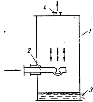
Рис. У-54. Установка для предварительной акустической коагуляции частиц при газоочистке:
