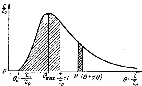
Рис. П-37. Функция распределения времени пребывания (кривая отклика) в безразмерных координатах для аппарата промежуточного типа.
