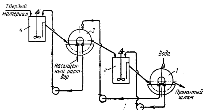
Рис. ХШ-29. Схема противоточной промывки осадка (шлама) на барабанных вакуум-фильтрах:
