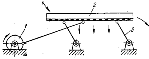
Рис. XIX-3. Схема качающегося грохота: 1 — эксцентрик; 2 — корпус; 3 — опорная стойка.
