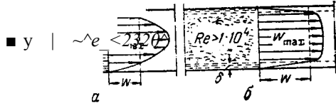
Рис. П-10. Распределение скоростей при различных режимах движения:
