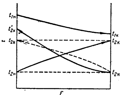
Рис. УП-21. Сравнение прямотока и противотока теплоносителей.
