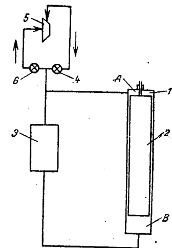
Рис. XVII-21. Принципиальная схема холодильного цикла с тепловым насосом:
