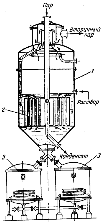
Рис. XV1-4. Выпарной аппарат-кристаллизатор с подвешенной греющей камерой и нутч-фильтрами:
