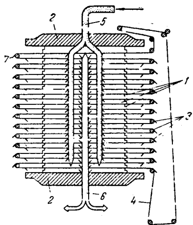
Рис. У-20. Схема действия автоматизированного фильтрпресса с горизонтальными камерами:
