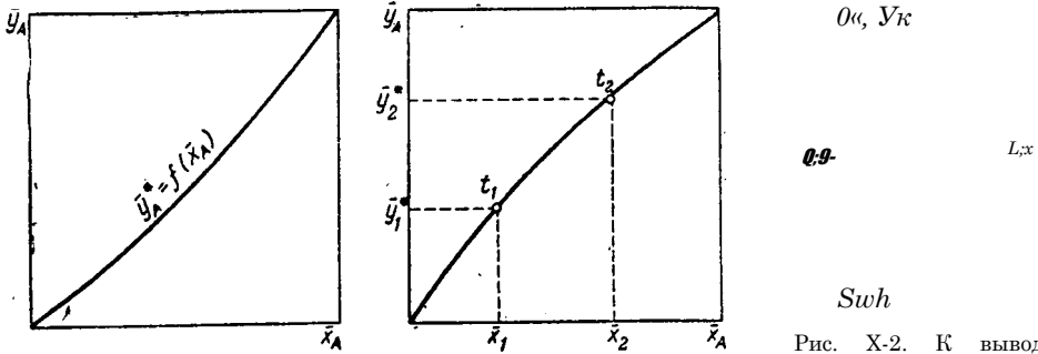
Рис. X-2. К выводу уравнения материального баланса противоточного массообменного аппарата
