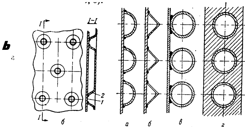
Рис. VII-25. Аппарат с рубашкой:
