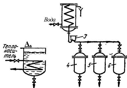
Рис. XII-8. Схема установки для фракционной перегонки:
