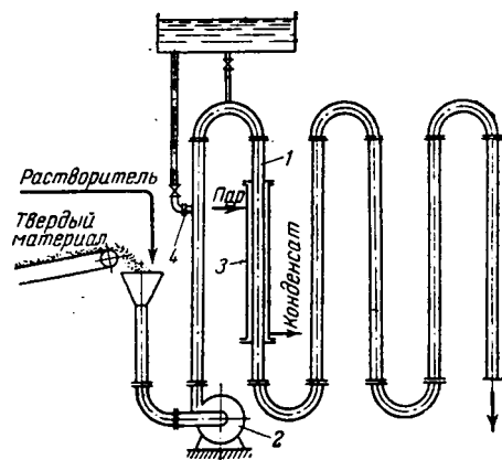
Рис. XIII-33. Трубчатый экстрактор:
