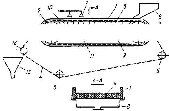
Рис. У-25. Ленточный вакуум-фильтр'
