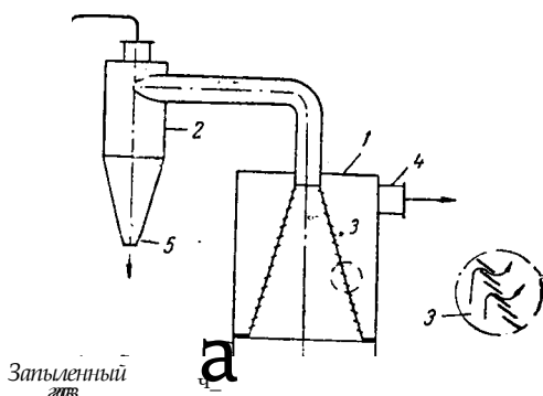
Рис. У-39. Инерционный жалюзийный пылеуловитель:
