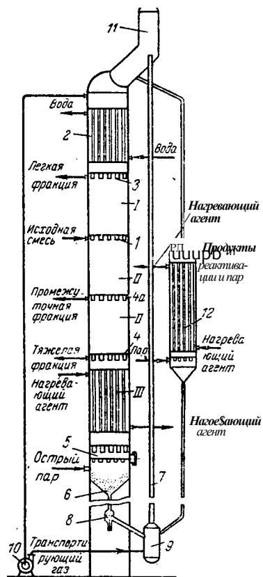
Рис. XIV-7. Схема адсорбционной установки с движущимся слоем активного угля:
