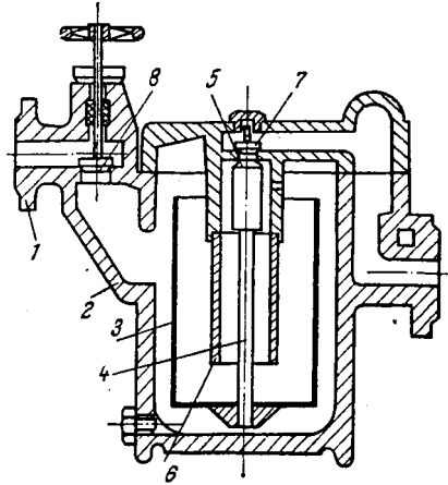
Рис. УП1-2. Конденсатоотводчик с открытым поплавком:
