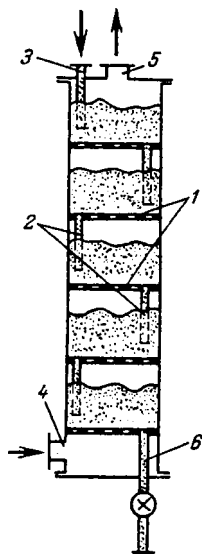
Рис. X1Y-9. Многокамерный адсорбер с кипящим слоем поглотителя:
