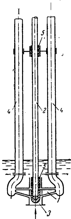
Рис. Ш-20. Схема погружного насоса:
