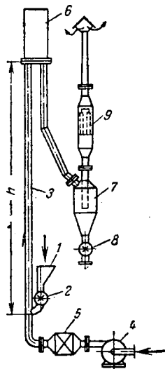
Рис. XV-28. Пневматическая сушилка:
