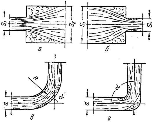
Рис. 11-24. Некоторые местные сопротивления: а — внезапное расширение; б — внезапное сужение; в — плавный поворот на 90° (отвод); з — резкий поворот на 90° (колени).
