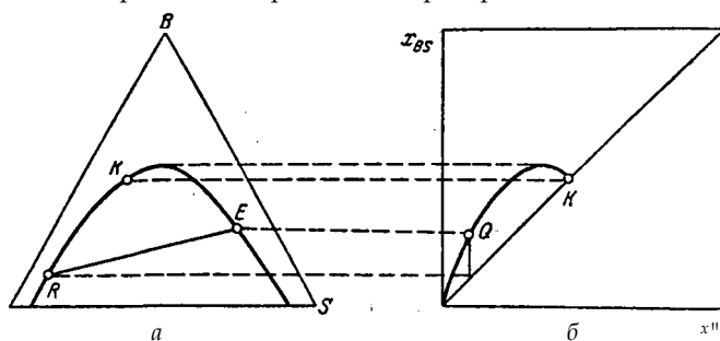
Рис. XIII-7. Треугольная диаграмма (а) и кривая распределения (б) для системы с одной парой частично смешивающихся компонентов.
