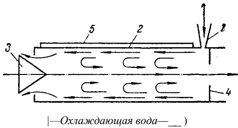
Рис. XVII-4. Вихревая труба:
