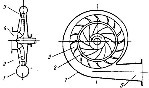
Рис. 1У-12.. Схема турбогазодувки: 1 — корпус; 2 — рабочее колесо; 3 — направляющий аппарат; 4 — всасывающий патрубок; 5 — нагнетательный патрубок.
