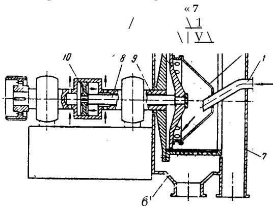
Рис. У-31. Центрифуга с пульсирующим поршнем для выгрузки осадка: ■
