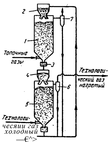
Рис. УШ-8. Нагревательная установка с падающей насадкой:
