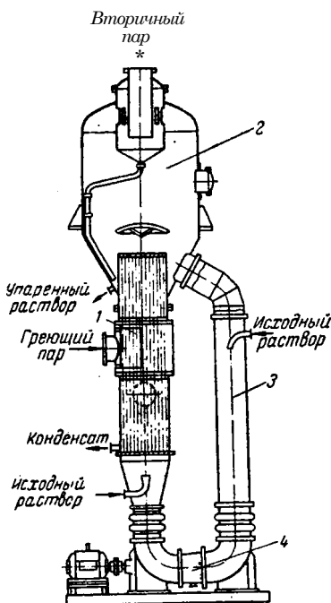
Рис. IX-17. Выпарной аппарат с принудительной циркуляцией:
