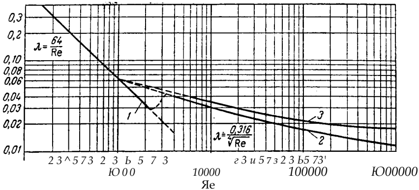
Рис. П-22. Зависимость \lambda от критерия \text{Re} :
