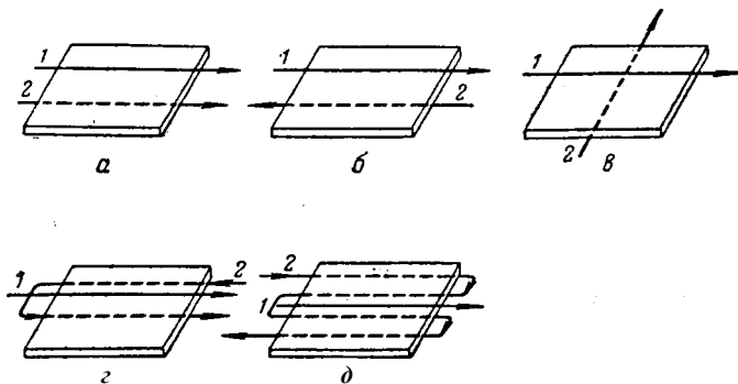
Рис. УП-16. Схемы направления движения жидкостей I и 2 при теплообмене:
