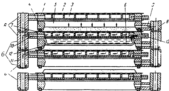
Рис. V-19. Автоматизированный фильтрпресс с горизонтальными камерами (ФПАКМ):
