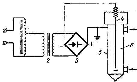
Рис. У-51. Принципиальная схема установки для электрической очистки газов:
