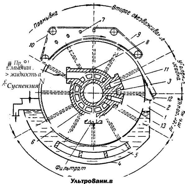
Рис. У-21. Схема действия барабанного вакуум-фильтра с наружной поверхностью фильтрования:
