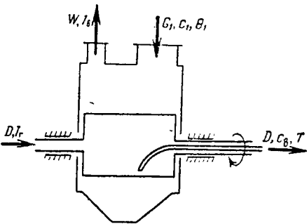
Рис. XV-6. Принципиальная схема контактной сушилки непрерывного действия.
