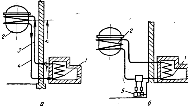
Рис. VIII-5. Принципиальные схемы установок с естественной (а) и принудительной (б) циркуляцией жидкого промежуточного теплоносителя:
