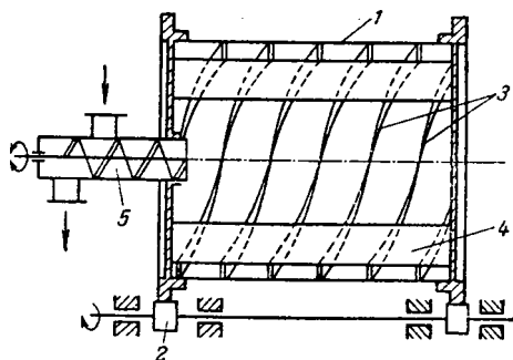
Рис. XX-1. Схема смесового барабана:
