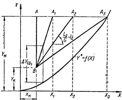
Рис. XI-2. К определению удельного расхода абсорбента.
