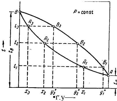
Рис. XII-2. Зависимость температур кипения и конденсации от состава фаз (диаграмма I-x-y ).
