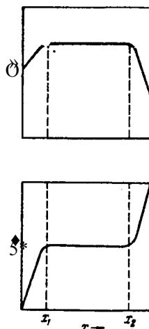
Рис. XII-7. Диаграммы p-x и y-x для смесей жидкостей, ограниченно растворимых друг в друге.
