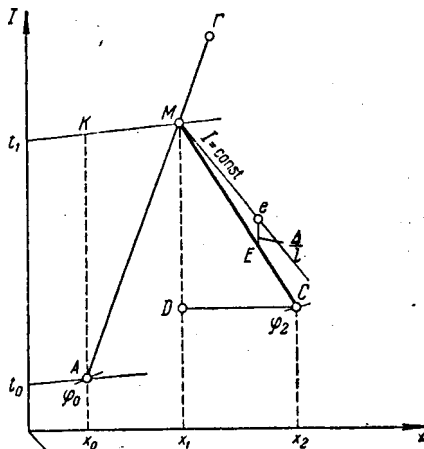
Рис. XV-13: Построение на t-x -диаграмме процесса сушки топочными газами (основной вариант процесса сушки).
