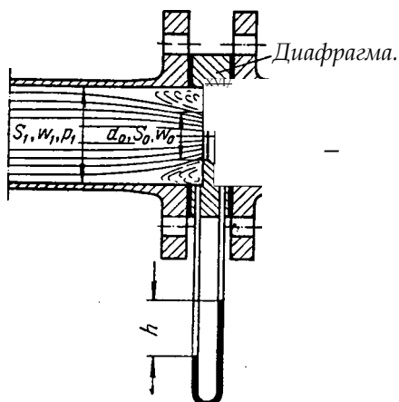
Рис. П-17. Мерная диафрагма.
