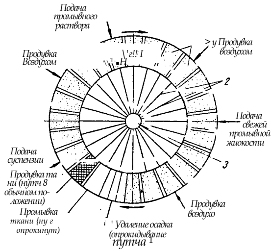
Рис. У-24. Схема карусельного фильтра в плане:
