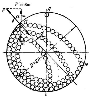
Рис. XVIII-12. К определению числа оборотов шаровой мельницы.
