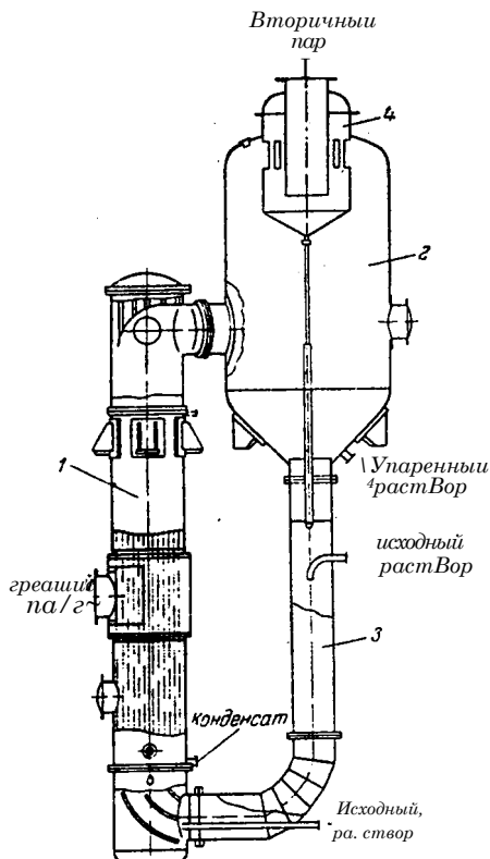
Рис. 1X-12. Выпарной аппарат с выносной нагревательной камерой:
