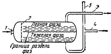
Рис. У-8. Отстойник непрерывного действия для разделения эмульсий:
