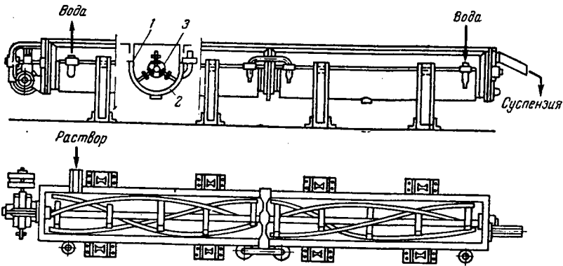
Рис. XVI-7. Кристаллизатор с ленточной мешалкой:
