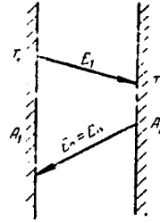
Рис. VII-7. К выводу закона Кирхгофа.
