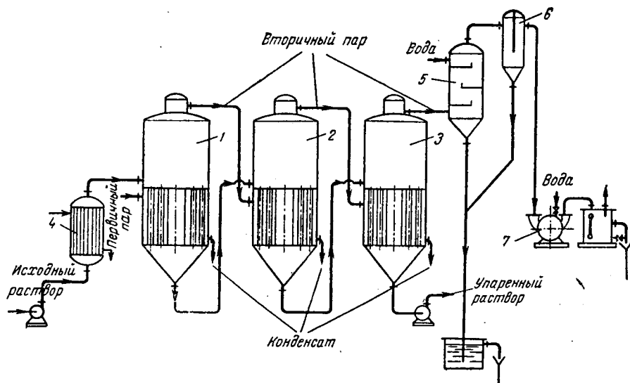
Рис. 1X-2. Многокорпусная прямоточная вакуум-выпарная установка:
