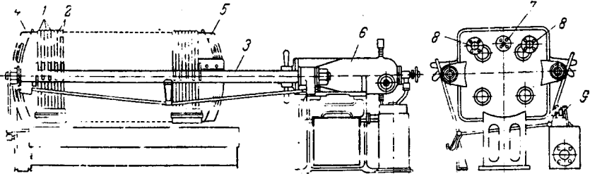
Рис. \M4. Фильтрпресс с вертикальными рамами (плиточно-рамный фильтрпресс):
