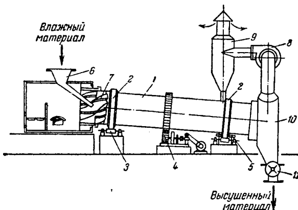
Рис. ХУ-22. Барабанная сушилка:
