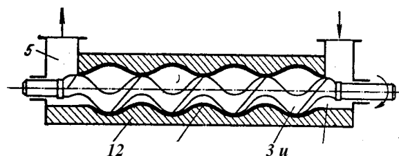
Рис. Ш-26. Схема одновинтового (героторного) насоса:
