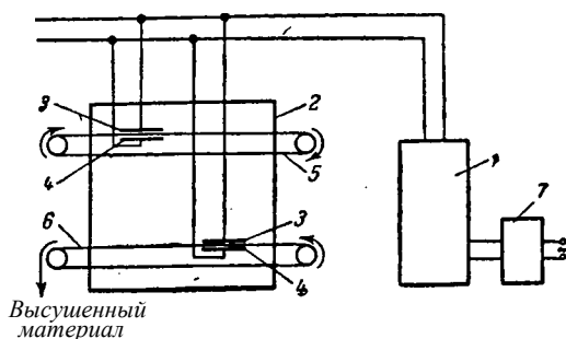
Рис. ХУ-36. Высокочастотная (диэлектрическая) сушилка:
