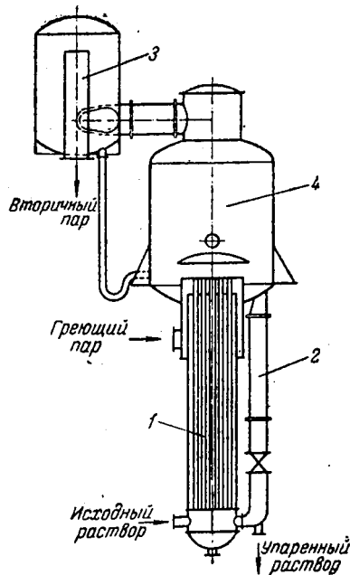
Рис. 1X-11. Выпарной аппарат с выносной циркуляционной трубой:
