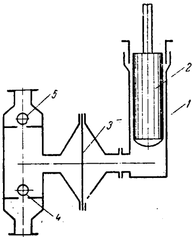
Рис. 111-18. Схема диафрагмового (мембранного) насоса:
