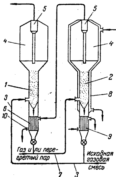
Рис. X1Y-10. Схема установки для адсорбции и десорбции в псевдооживленном слое поглотителя:
