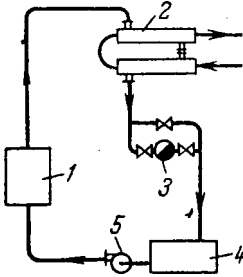
Рис. УП1-1. Схема нагрева глущим паром:
