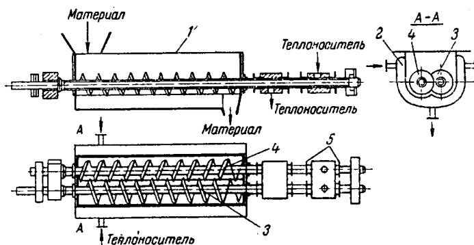
Рис. VII1-28. Шнековый теплообменник:
