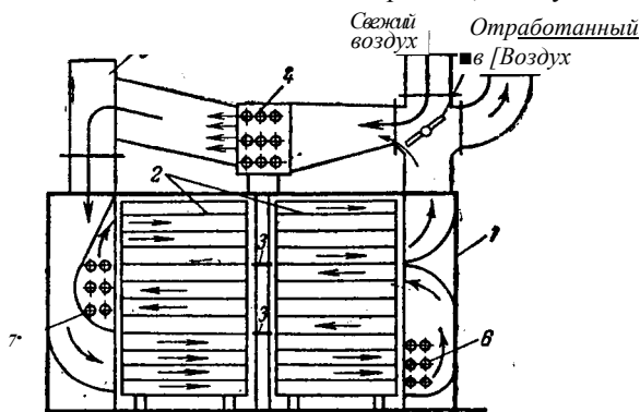
Рис. XV-18. Камерная сушилка:
