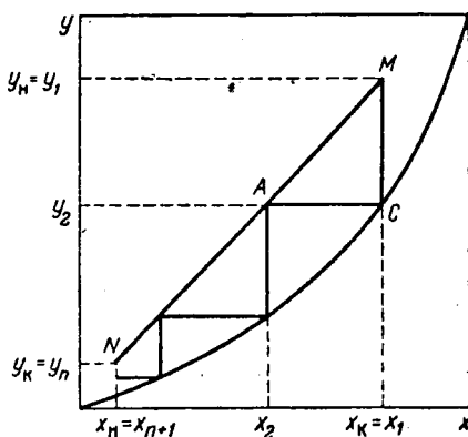
Рис. X-15. Определение числа теоретических ступеней графическим методом.
