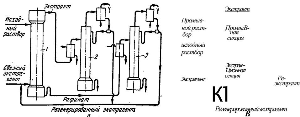
Рис. ХИМ. Принципиальные схемы процесса экстракции в системах жидкость—жидкость:
