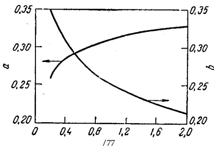
Рис. 11-27. Значения констант в уравнении (11,95а).
