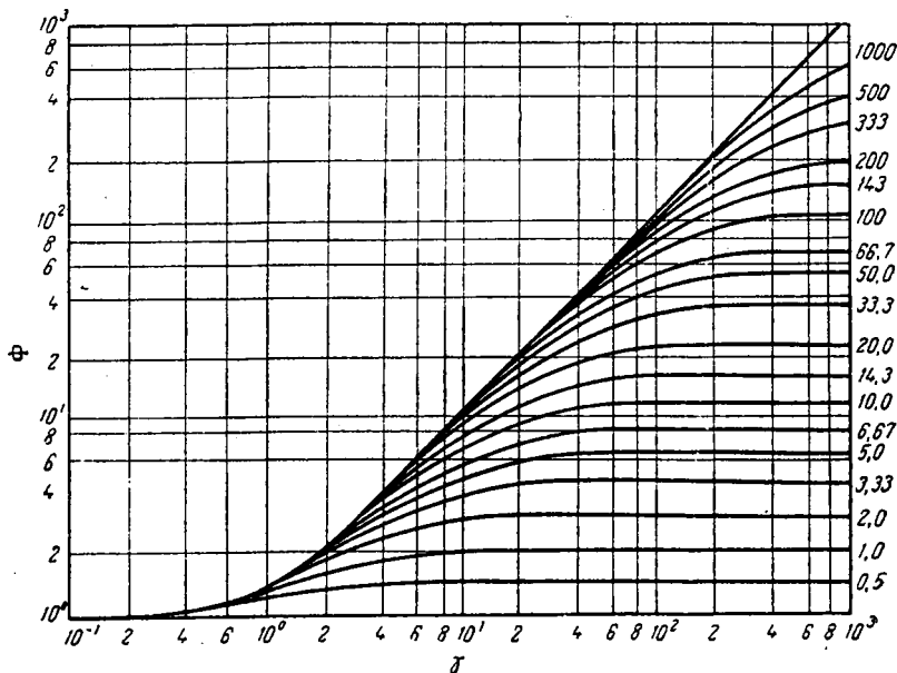
Рис. X1-5. Зависимость фактора ускорения \Phi от комплексов u и N .
