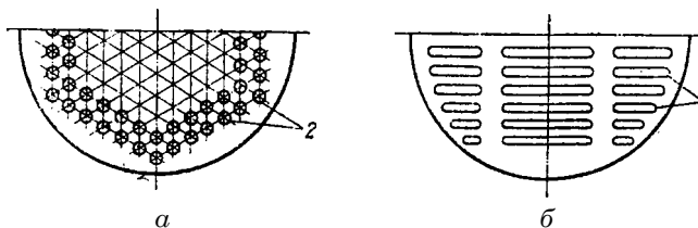
Рис. XI-27. Провальные тарелки:
