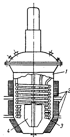
Рис. УШ-Ю. Аппарат с внешними индукционными катушками:
