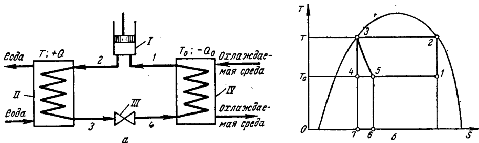
Рис. XVII-5. Компрессионная холодильная машина:
