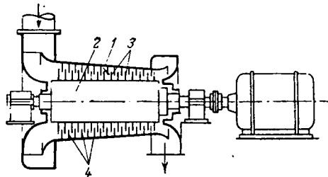
Рис. 1У-17. Схема осевого компрессора:
