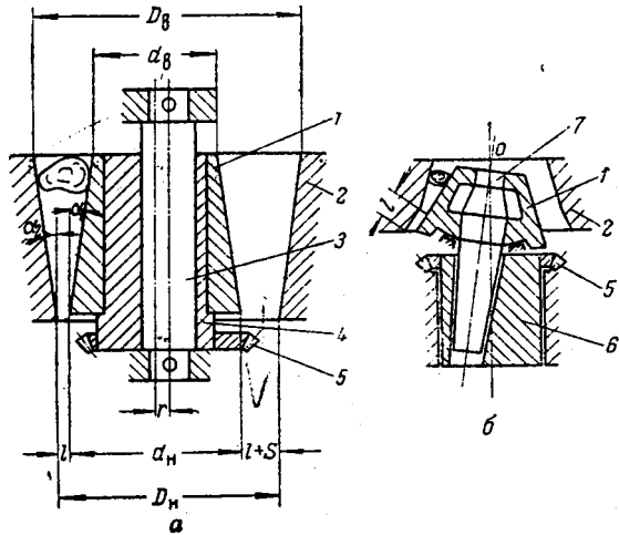
Рис. XVI [1-6. Схемы конусных дробилок:
