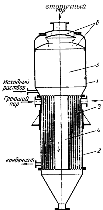
Рис 1X-9. Выпарной аппарат с внутренней нагревательной камерой и центральной циркуляционной трубой:
