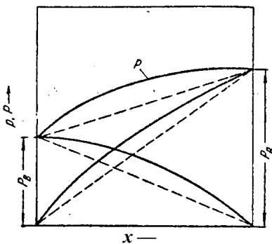
Рис. XII-4. Диаграмма p-x для смеси с положительным отклонением от закона Рауля (пунктиром показаны соответствующие линии для идеального раствора).
