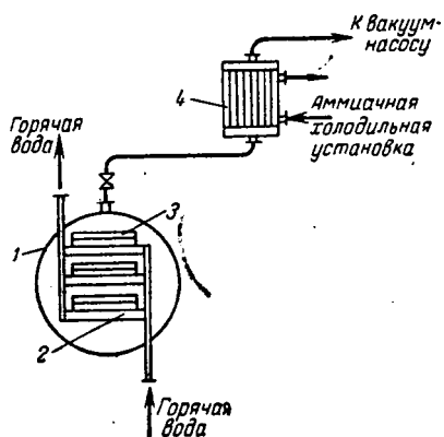
Рис. ХУ-737. Принципиальная схема сублимационной сушилки:
