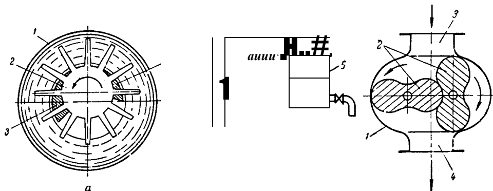
Рис. 1У-9. Схема ротационного водокольцевого компрессора (а) Рис. 1У-10. Схема ротационной газодувки:
