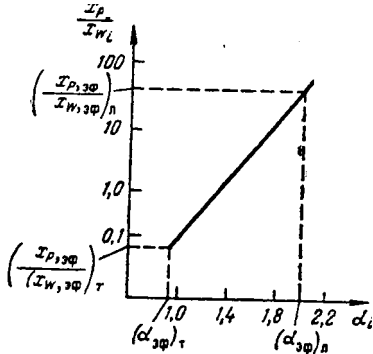
Рис. XII-28. К составлению материального баланса процесса многокомпонентной ректификации.
