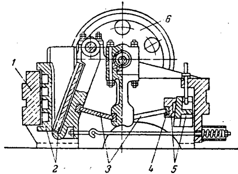
Рис. XVIII-4. Общий вид щековой дробилки: 1 — корпус; 2 — сменные плиты; 3 — распорные плиты; 4 — вкладыш; 5 — регулировочные клинья; 6 — маховик.
