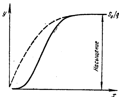
Рис. XIII-2. Типичная изотерма экстракции для извлечения неорганических веществ.
