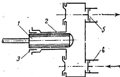
Рис. Ш-11. Схема горизонтального плунжерного насоса простого действия:
