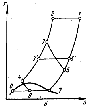
Рис. XV11-16. Соединенные дроссельный и детандерный регенеративный циклы:
