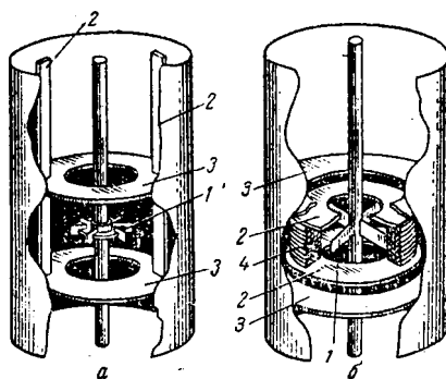
Рис. XIII-23. Устройство секций непрерывно действующих колонных экстракторов с механическими мешалками:
