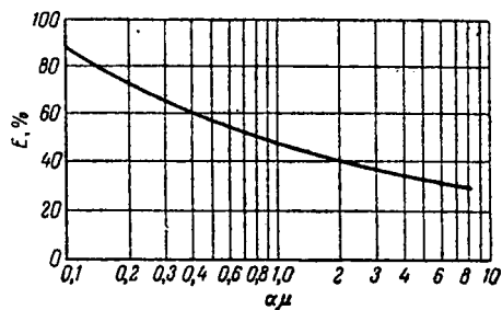
Рис. XII-25. График для определения средней эффективности колонны E в зависимости от произведения летучести компонентов a на среднемолярную вязкость жидкости питания \mu (в cm^3 ).
