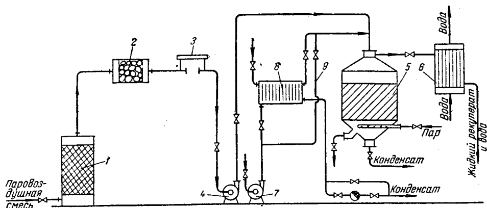
Рис. X1У-6. Схема промышленной углеадсорбционной установки для улавливания (рекуперации) паров органических веществ из их смеси с воздухом:
