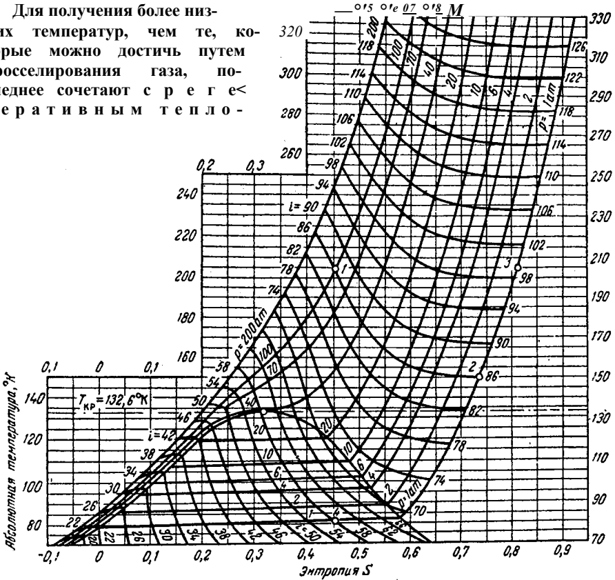
Рис. XVII-3. Диаграмма T—S для воздуха.
