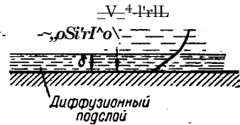
х 6 Структура пограничного слоя
