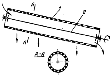
Рис. XIX-2. Схема барабанного грохота: 1 — барабан; 2 — центральный вал.
