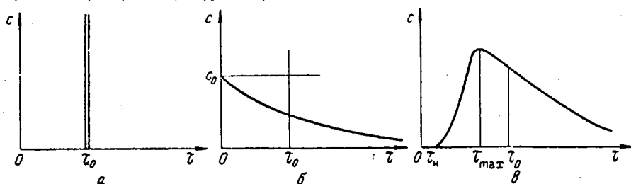
Рис. 11-36. Кривые отклика при мгновенном вводе индикатора: а — аппарат идеального вытеснения; б — аппарат идеального смешения; в — аппарат промежуточного типа.
