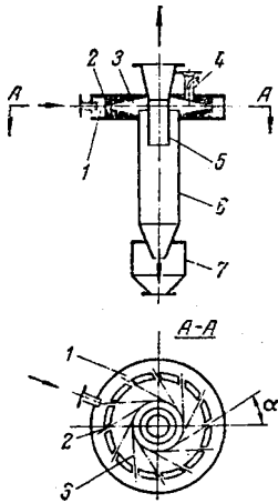
Рис. XVШ1-17. Схема струйной мельницы с плоской помольной камерой:
