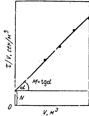
Рис. У-12. К определению удельного сопротивления осадка и сопротивления фильтровальной перегородки.
