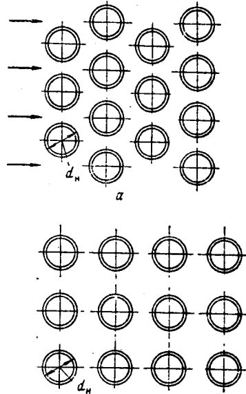
Рис. УП-Ю. Движение теплоносителя при обтекании трубного пучка:
