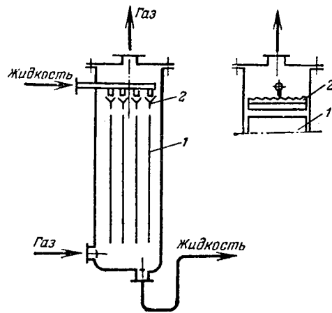
Рис. XI-10. Абсорбер с плоскопараллельной насадкой:
