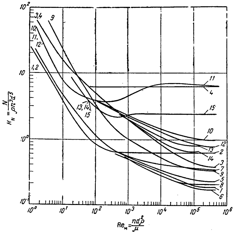
Рис. VI-2. Зависимость критерия мощности K_{\Sigma} от критерия Рейнольдса Re_m для мешалок нормализованных типов:
