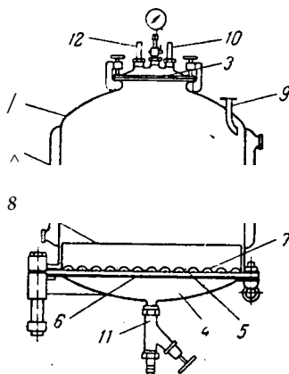
Рис. У-13. Нутч, работающий под давлением до 3 ат:
