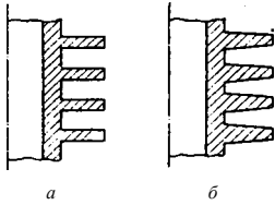
Рис. VIII-21. Элементы оребренного теплообменника:
