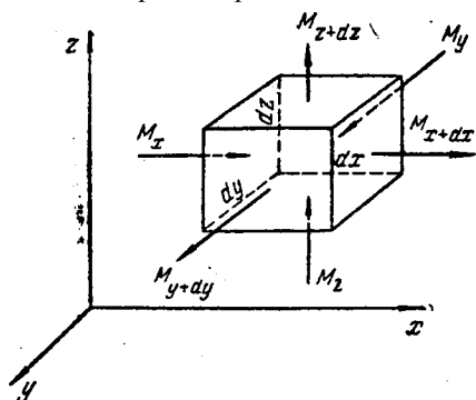
Рис. П-12. К выводу дифференциального уравнения неразрывности потока.
