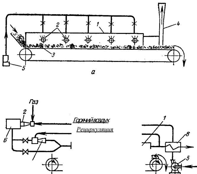
Рис. XV-35. Терморрадиационные сушилки с газовым обогревом:
