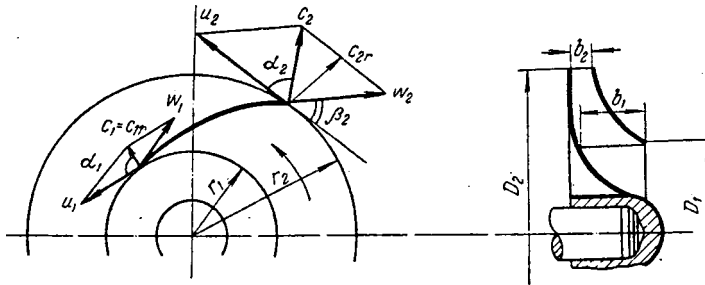
Рис. Ш-4. К выводу основного уравнения центробежных машин.
