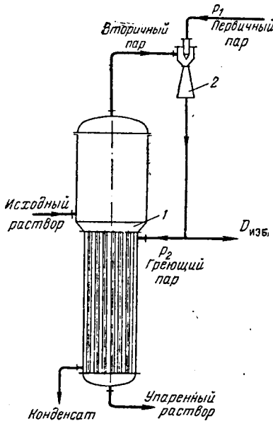
Рис. 1X-18. Схема однокорпусной выпарной установки с тепловым насосом:
