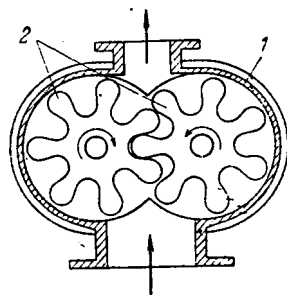
Рис. Ш-24. Схема шестеренного насоса:
