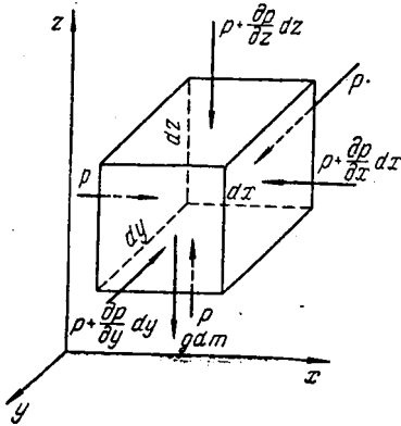
Рис. 11-2. К выводу дифференциальных уравнений равновесия Эйлера.
