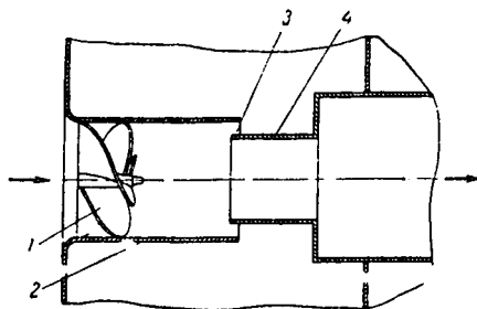
Рис. У-43. Элемент прямоточного батарейного циклона:
