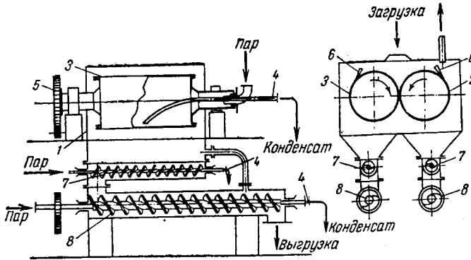
Рис. ХУ-31. Двухвальцовая сушилка:
