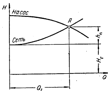
Рис. III-8. Совмещение характери- стик насоса и сети.
