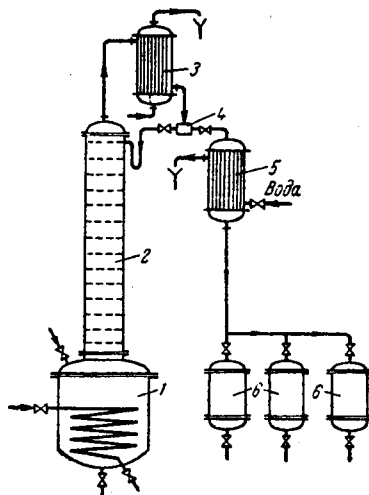
Рис. ХП-15. Схема периодически действующей ректификационной установки:
