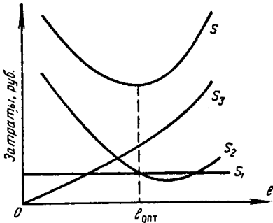
Рис X1-3. К определению оптимального удельного расхода абсорбента.
