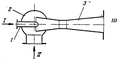
Рис. Ш-28. Струйный насос:
