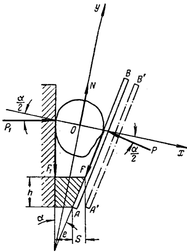
Рис. XV111-5. К расчету угла захвата, числа оборотов и производительности щековой дробилки.
