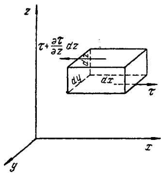
Рис. II-14. К выводу уравнений Навье—Стокса.
