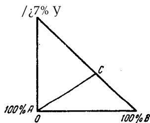
Рис. XIII-35. Треугольная диаграмма (системы твердое тело — жидкость).
