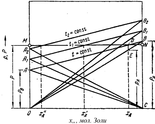
Рис. XII-1. Изотермы парциальных давлений компонентов и общего давления для идеальных растворов (диаграмма p-x ).
