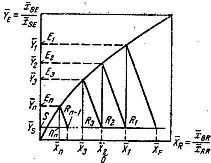
Рис. XIII-10. Схема многоступенчатой экстракции при перекрестном токе (а) и изображение процесса на диаграмме Y - X (б): 1 < 2, 3, ..., n - ступени.
