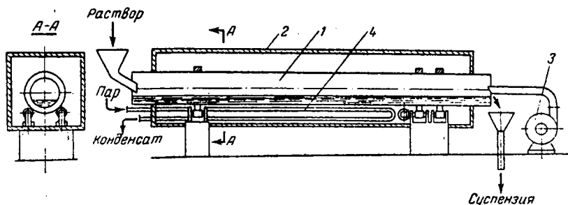
Рис. XVI-8. Барабанный кристаллизатор с воздушным охлаждением:
