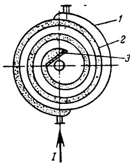
Рис. У1П-24. Спиральный теплообменник:
