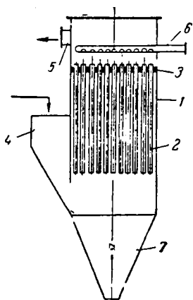
Рис. Y-45. Металлокерамический фильтр:
