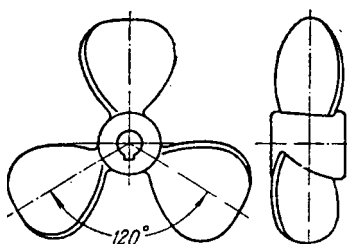
Рис. VI-8. Пропеллерная мешалка.
