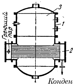
Рис. 1X-8. Выпарной аппарат с горизонтальной трубчатой нагревательной камерой и вертикальным цилиндрическим корпусом:
