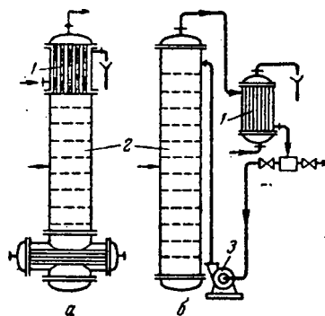
Рис. ХП-23. Варианты установки дефлегматора:
