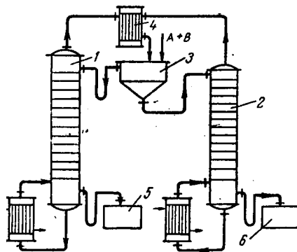
Рис. ХП-33. Схема двухколонной установки для гетероазеотропной ректификации бинарных расслаивающихся жидкостей:
