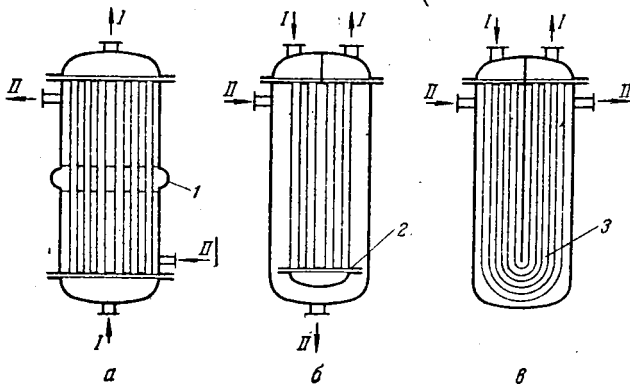
Рис. УПЫ4. Кожухотрубчатые теплообменники с компенсирующими устройствами:
