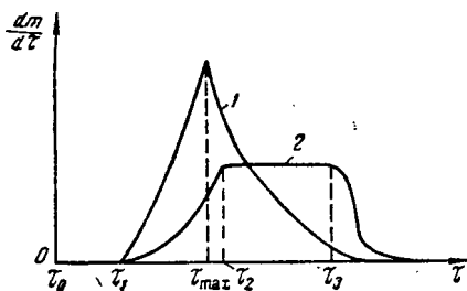
Рис. XVI-3. Изменение скорости кристаллизации ( m ) во времени ( t ):
