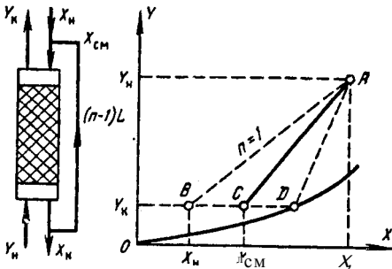
Рис. X1-33. Схема одноступенчатой абсорбции с рециркуляцией жидкости.
