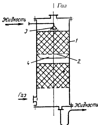
Рис. XI-12. Насадочный абсорбер:
