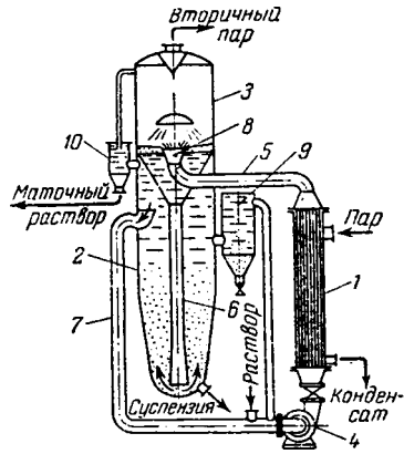
Рис. XV1-11. Выпарной аппарат-кристаллизатор с псевдооживленным слоем и выносной нагревательной камерой:
