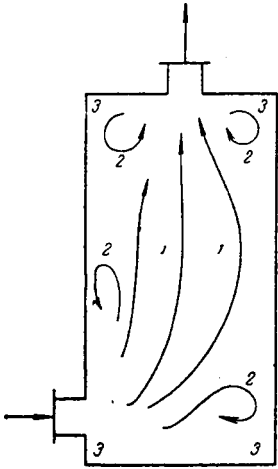
Рис. 11-35. Движение потока в полном аппарате.
