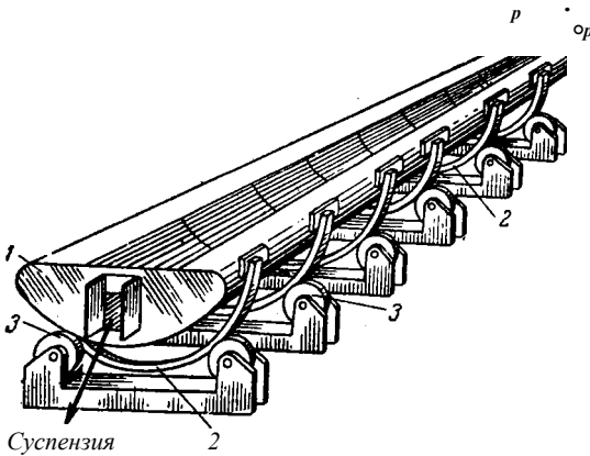
Рис. ХУ1-6. Качающийся кристаллизатор:
