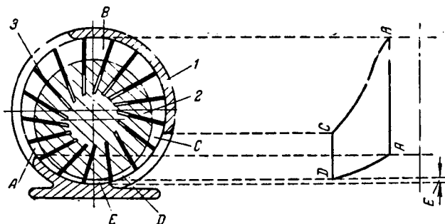
Рис. 1У-8. Схема ротационного пластинчатого компрессора:
