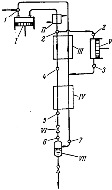
Рис. XIII-17. Соединенные циклы дроссельный и детандерный без регенерации:
