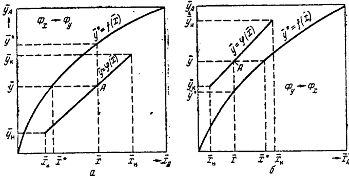
Рис. X-3. Определение направления массопередачи по y-x диаграмме:
