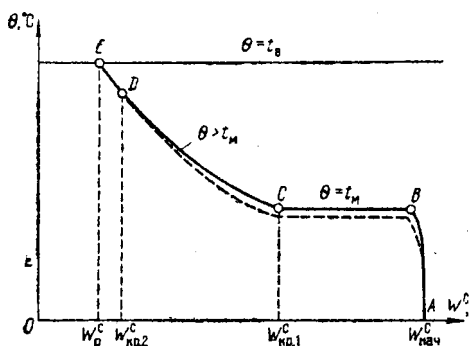
Рис. ХУ-17. Температурная кривая материала.
