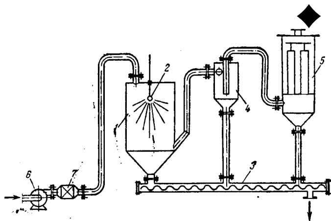
Рис. XV-27. Распылительная сушилка:
