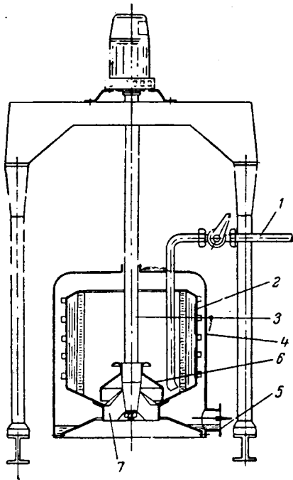
Рис. V-29. Подвесная центрифуга:
