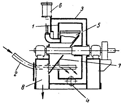
Рис. V-30. Горизонтальная центрифуга
