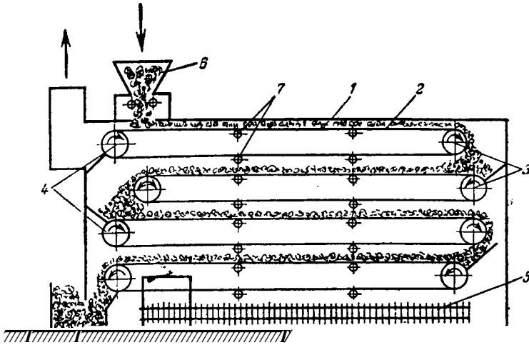
Рис. ХУ-20. Ленточная сушилка:
