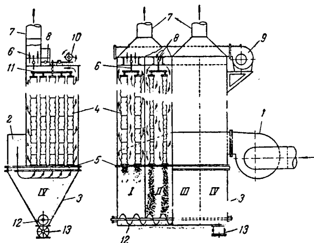
Рис. У-44. Рукавный фильтр с механическим встряхиванием и обратной продувкой ткани:
