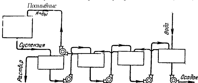
Рис. У-5. Схема непрерывной противоточной отмывки осадка от жидкости.
