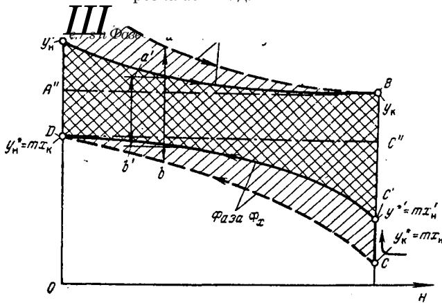
Рис. X-11. Влияние перемешивания на изменение концентраций по высоте (длине) массообменного аппарата.
