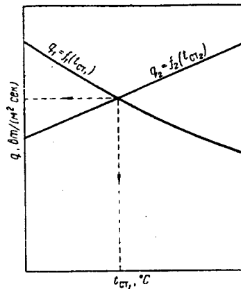
Рис. VIII-31. Построение нагрузочной характеристики теплообменника.
