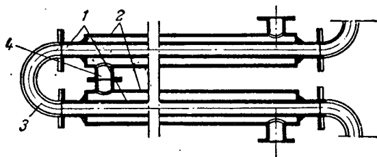
Рис. У1Н-16. Двухтрубчатый теплообменник:
