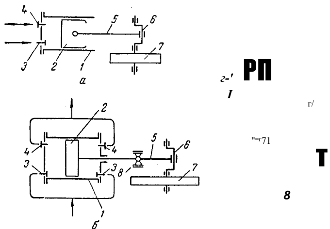
Рис. 1У-3. Схемы одноступенчатых поршневых компрессоров:
