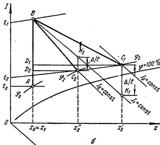
Рис. XV-7. Изображение процессов сушки на l-x -диаграмме: a — теоретическая сушилка; б — действительная сушилка.
