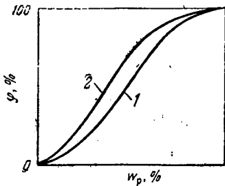
Рис. XV-3. Зависимость равновесной влажности материала от относительной влажности воздуха: 1 -- изотерма десорбции; 2 — изотерма сорбции.
