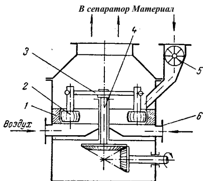
Рис. ХУШ-14. Схема кольцевой роliko-маятниковой мельницы:
