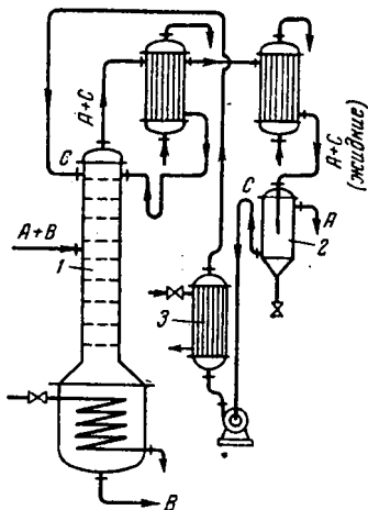
Рис. ХП-32. Схема установки для азеотропной ректификации:
