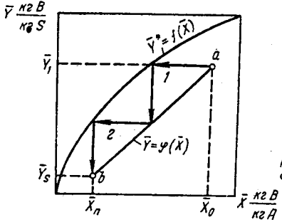
Рис. XIII-12. Изображение процесса многоступенчатой противоточной экстракции на прямоугольной диаграмме P - X (1, 2 - ступени).
