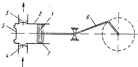
Рис. Ш-10. Схема горизонтального поршневого насоса простого действия:
