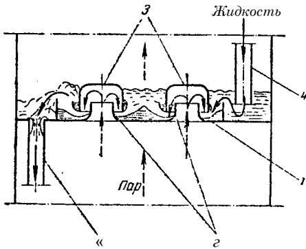
Рис. X1-19. Схема работы колпачковой тарелки: 1 — тарелка; 2 — газовые патрубки; 3 — колпачки; 4 — сливные трубки.
