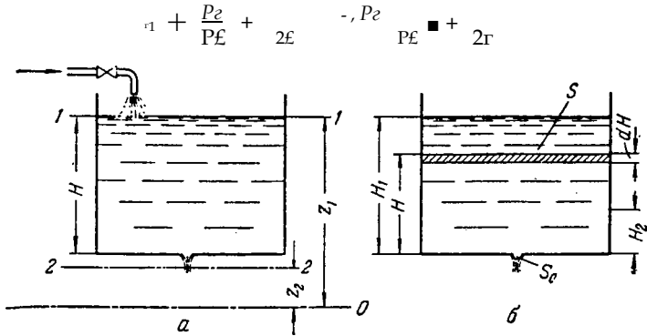
Рис. П-20. Истечение жидкости из сосуда:
