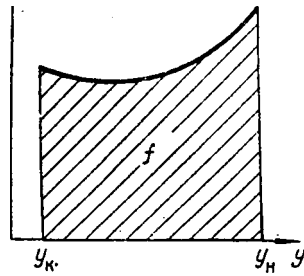
Рис. X-9. Определение числа единиц переноса методом графического интегрирования.
