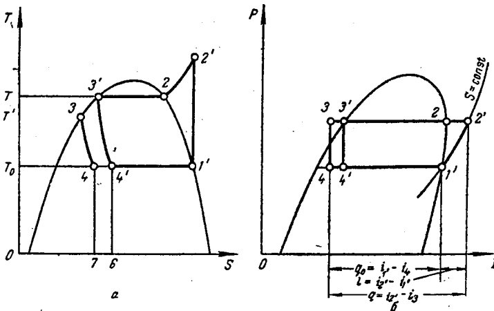
Рис. ХУП-7. Изображение холодильного цикла действительной компрессионной холодильной машины на диаграммах T-i и p-i .
