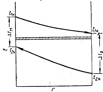
Рис. VII-18. Изменение температуры теплоносителей при движении жидкостей противотоков.
