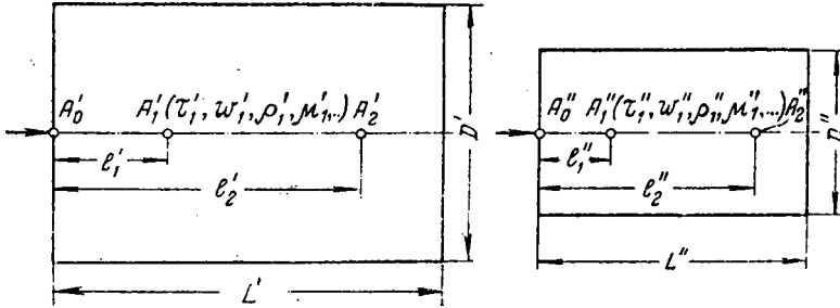
Рис. 11-21. К формулировке условий подобия потоков в натуре и в модели.
