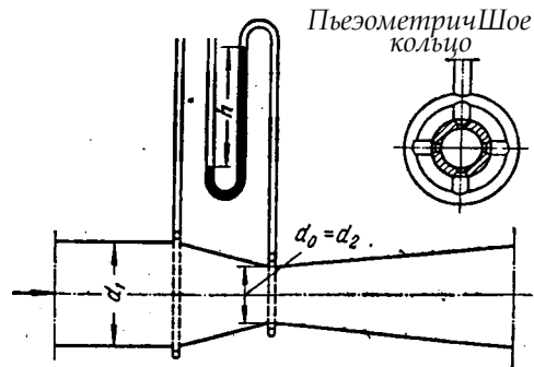
Рис. П-19. Труба Вентури.
