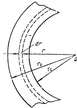
Рис. V-36. К расчету фильтрующих центрифуг непрерывного действия.
