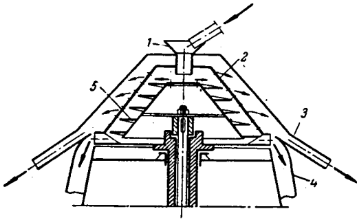
Рис. У-33. Центрифуга с инерционной выгрузкой осадка:
