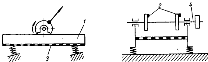
Рис. XIX-5. Схема вибрационного грохота:
