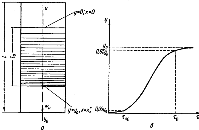
Рис. XIY-4. Массопередача при адсорбции:
