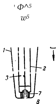
Рис. V-3б. Схема устройства трубчатой сверхцентрифуги:
