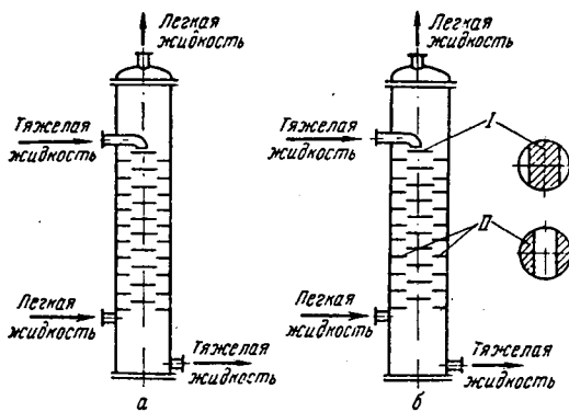
Рис. ХШ-20. Полочные колонные экстракторы:
