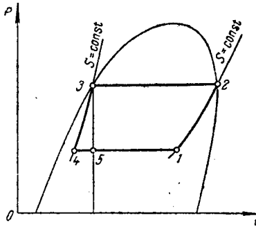
Рис. XVII-6. Изображение холодильного цикла компрессионной холодильной машины на диаграмме p-i .
