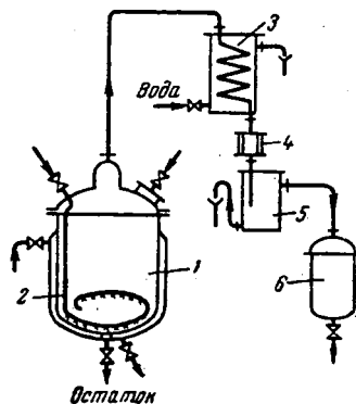
Рис. XII-10. Схема установки для перегонки с водяным паром:
