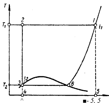
Рис. XVII-2. Работа сжижения газа по идеальному циклу.
