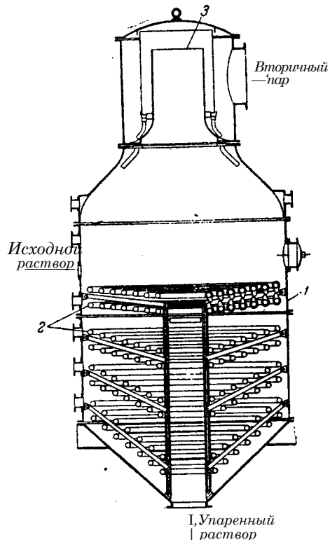
Рис. 1X-7. Змеевиковый выпарной аппарат:
