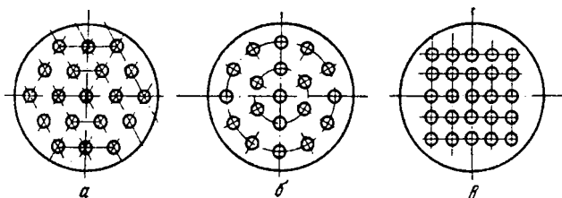
Рис. УШ-12. Способы размещения труб в теплообменниках:
