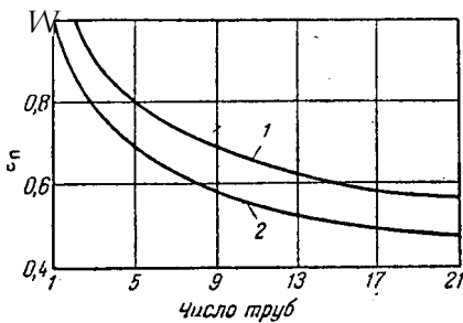
Рис. УП-12. Значение усредненного поправочного коэффициента e_n при различном размещении труб в пучке:
