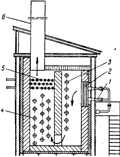
Рис. VIII-4. Печь для нагрева жидких продуктов, работающая на газе:
