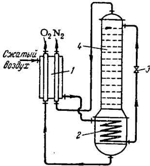
Рис. XII-36. Установка одинарной ректификации для разделения жидкого воздуха:
