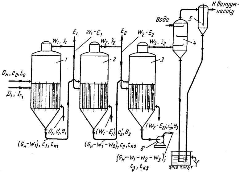
Рис. 1X-5. К составлению теплового баланса многокорпусной выпарной установки:
