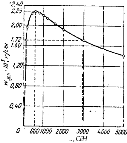
Рис. У-11. Зависимость w'_{удн} от t_{осж} .
