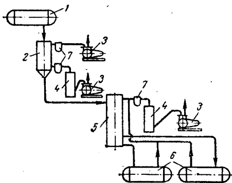
Рис. XII-34. Схема установки для молекулярной дистилляции:
