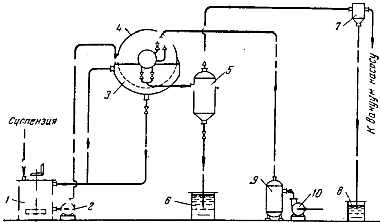
Рис. У-23. Схема установки с барабанным вакуум-фильтром.
