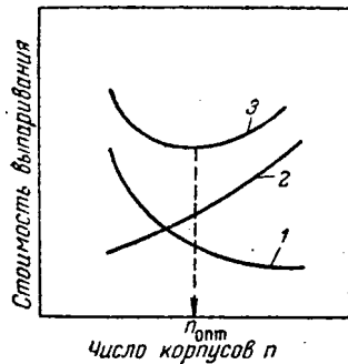
Рис. 1X-6. К определению оптимального числа корпусов многокорпусной выпарной установки:
