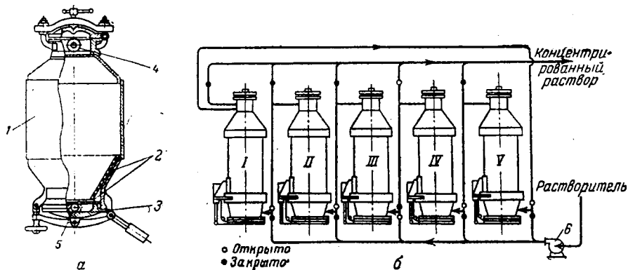
Рис. ХШ-30. Схема экстракции (выщелачивания) в батарее диффузоров: о — диффузор; б — батарея диффузоров (I—V); 1 — корпус; 2 — ложное днище (решетка); 3 — откидное днище; 4 — штуцер для ввода свежего растворителя; 5 — штуцер для отвода конечного (концентрированного) раствора; 6 насос.
