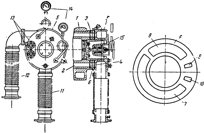
Рис. Ч-22. Распределительное устройство барабанного вакуум-фильтра:
