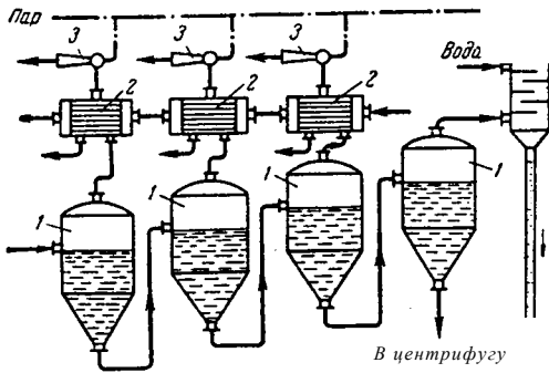
Рис. XVI-10. Многоступенчатая вакуум-кристаллизационная установка:
