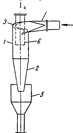
Рис. У-40. Циклон конструкции НИИОгаз:
