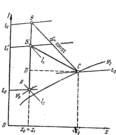
Рис. ХУ-8. Изображение теоретического процесса сушки с частичным подогревом воздуха в сушильной камере на I-x -диаграмме.
