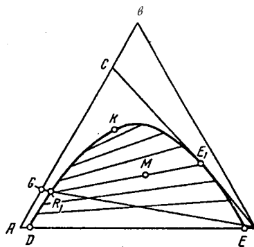
Рис. XIII-6. Треугольная диаграмма тройной системы жидкость-жидкость с одной парой частично смешивающихся компонентов ( A и B ).
