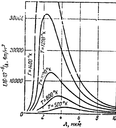
Рис. УП-6. Зависимость от \lambda ч T по уравнению Планка.
