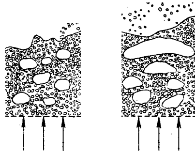
р>нс П-33. Возрастание неравномерности псевдооживления с увеличением скорости газа,
