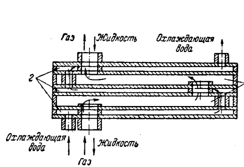
Рис. XI-8. Пластинчатый абсорбер:
