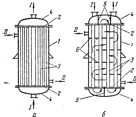
Рис. УШ-11. Кожухотрубчатые одноходовой (а) и многоходовой (б) теплообменники:
