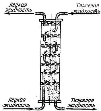
Рис. ХШ-21. Ситчатый колонный экстрактор.
