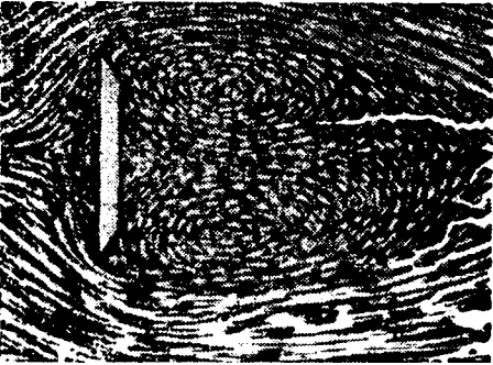
Рис. У1-1. Обтекание плоской пластины с острыми кромками при Re_{\text{кр}} \gg 10
