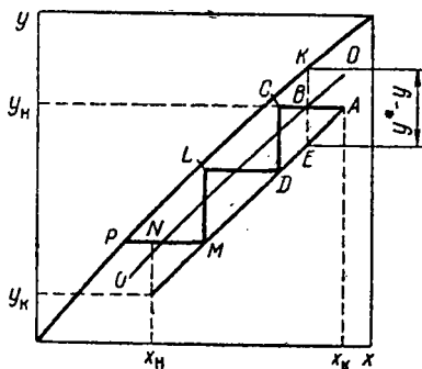
Рис. X-10. Определение числа единиц переноса упрощенным графическим методом.
