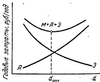
Рис. 11-28. К определению оптимального диаметра трубопровода.
