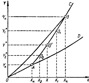
Рис. X1-4. Кривая равновесия при неизотермической абсорбции.
