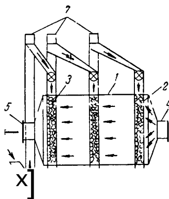
Рис. Y-46. Фильтр непрерывного действия с движущимся слоем зернистого фильтрующего материала:
