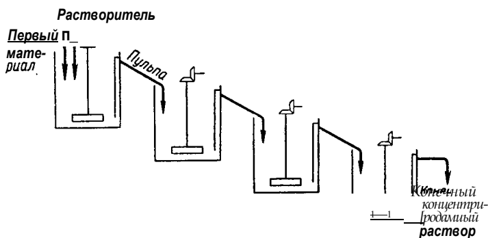
Рис. XIII-28. Схема непрерывного процесса экстракции в каскаде аппаратов с мешалками.
