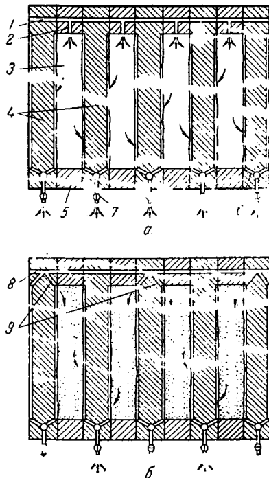
Рис. 1. Схема работы плиточно-рамного фильтрпресса;
