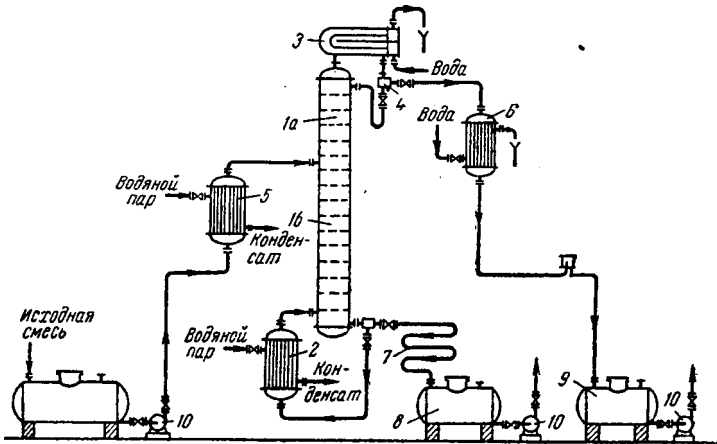
Рис. XII-14. Схема непрерывно действующей ректификационной установки:
