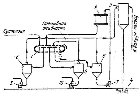
Рис. У-26. Схема противоточной промывки осадка на ленточном вакуум-фильтре:
