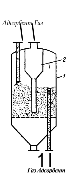
Рис. X1Y-8. Однокамерный адсорбер с кипящим слоем поглотителя:
