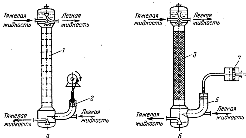
Рис. ХШ-24. Пульсационные колонные экстракторы:
