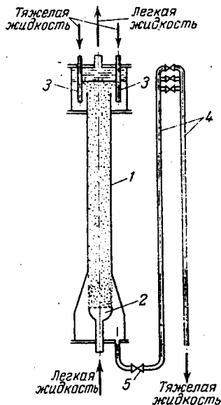
Рис. XII-19. Распылительный колонный экстрактор: 1 - корпус; 2 - распылитель тяжелой жидкости (сплошной фазы); 3 - гидравлический затвор; 4 - гидравлический затвор; 5 - регулирующий вентиль.
