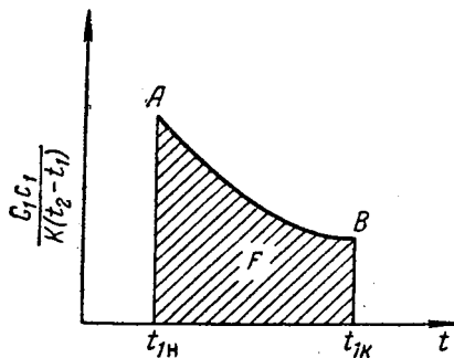
Рис. УП-20. К расчету поверхности теплообмена методом графического интегрирования.
