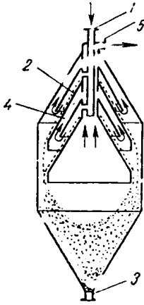
Рис. У-7. Отстойник непрерывного действия с коническими полками:
