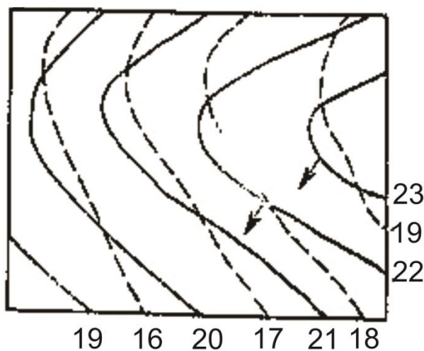
— gorizontal chizig'i - - - gidroizogips chizig'i ↙ yer osti suvlari oqimining yo'nalishi
