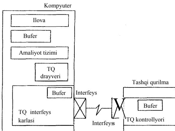
9.7-rasm Kompyuteming tashqi qurilmalar bilan aloqasi.
