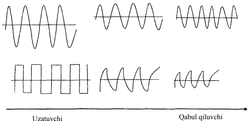
6.5-rasm. Elektr kabellarida signallarning soʻnishi.
