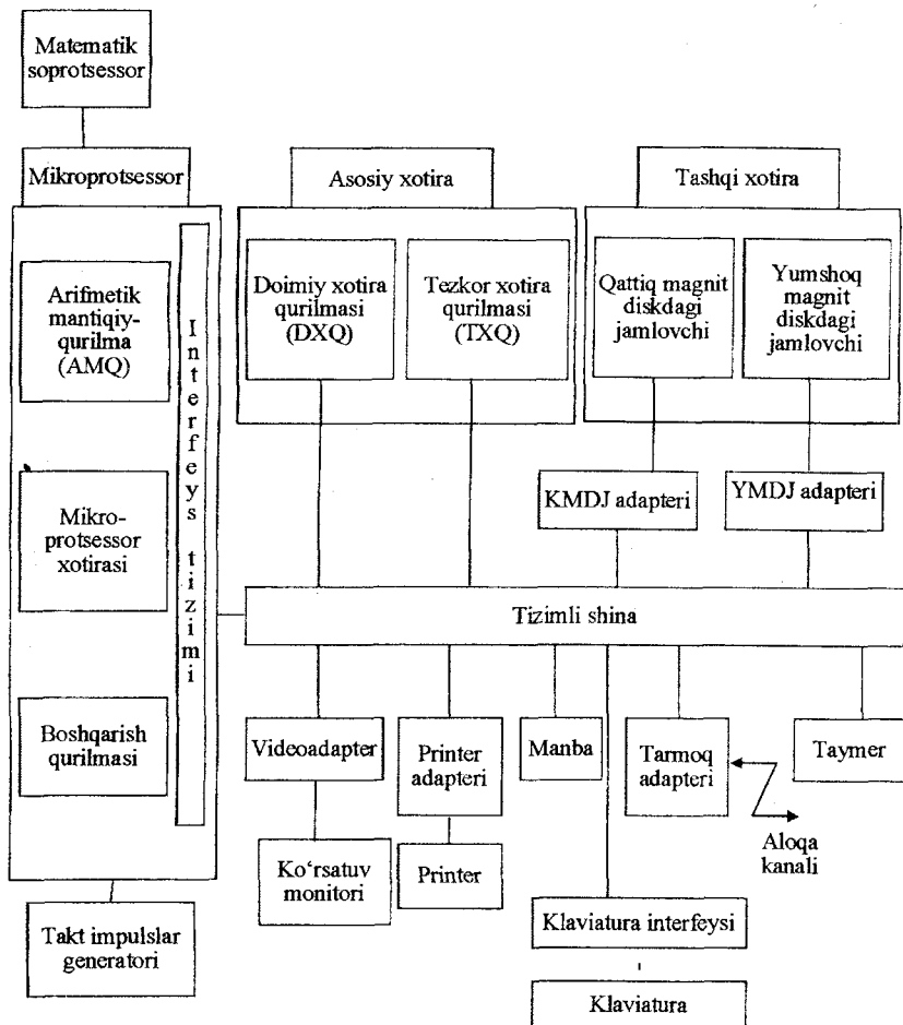
1.9-rasm. Shaxsiy kompyutemning tarkibiy sxemasi.
