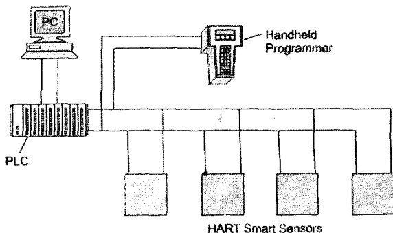
J 5.3-rasm. HART protokolida ko'p nuqtali aloqalar.
