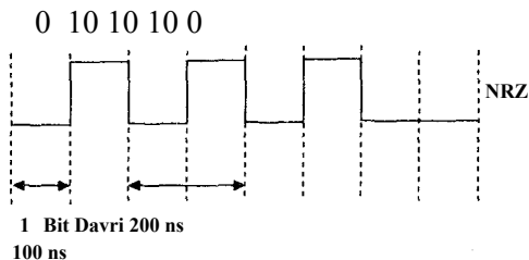
6.11-rasm. NRZ kodida kerakli o'tkazirish imkoniyati va uzatirish tezligi.
