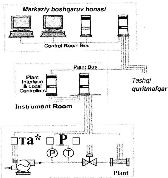
16.1-rasm. Tipik boshqarish tizimlarini bog'lash sxemasi.
