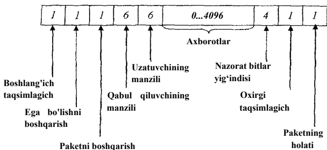
7.10-rasm. Token-Ring tarmoq paketiningoichami (maydon uzunliklari baytda berilgan).
