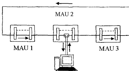
7.6-rasm. Konsentratorlarni birtomonlama aloqa yoki orqali birlashtirish.
