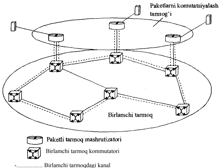
10.1-rasm. Birlamchi tarmoq orqali marshrutizatorlarni ulanishi.
