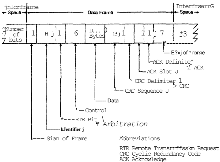
16.10-rasm. CANbus paketi.
