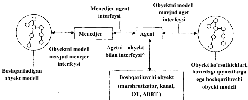
11.5-rasm. “Menejer - agent - boshqariluvchi obyekt” muloqotining sxemasi.
