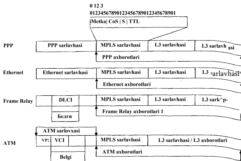
10.13-rasm. Bir necha MPLS texnologiya turlarining sarlavhalari o'ichamlari.
