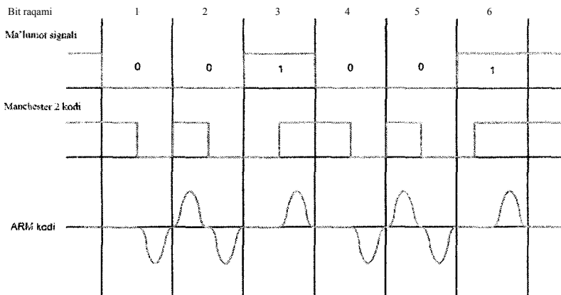
16.6-rasm. 0‘zgaruvchan puls modulatsiyasi.
