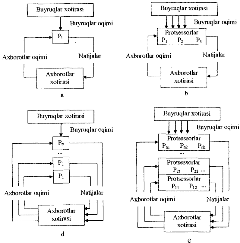
2.5-rasm. Yuqori parallelli MPHT shartli tarkibi.
