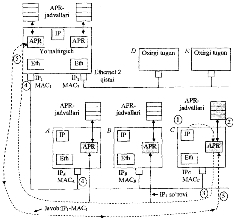
8.5-rasm. ARP protokoli ishlar sxemasi.
