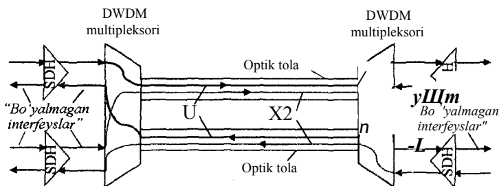
10.4-rasm. Bitta tolada turli uzunlikdagi toiqinlarni multiplesirlash tamoili.
