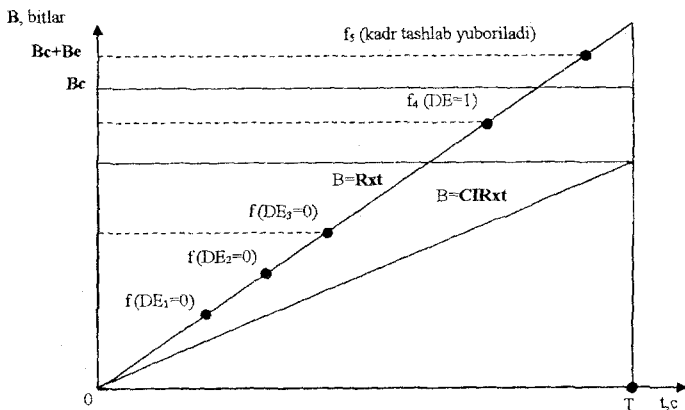
10.6-rasm. Foydalanuvchining xatti-harakatiga tarmoqning javobi.
