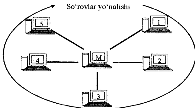
5.18-rasm. Yulduz topologiyali tarmoqda axborot almashinuvini markazlashtirilgan boshqarish usuli.
