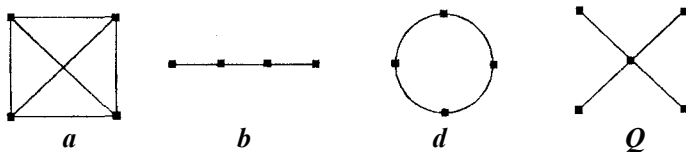
3.4-rasm. Parallel hisoblash tizimlarining asos topologiyalari.
