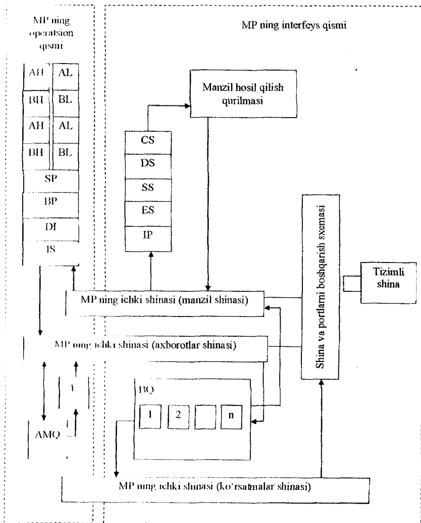
1.13-rasm. Mikroprotessorning soddalashtirilgan sxemasi.
