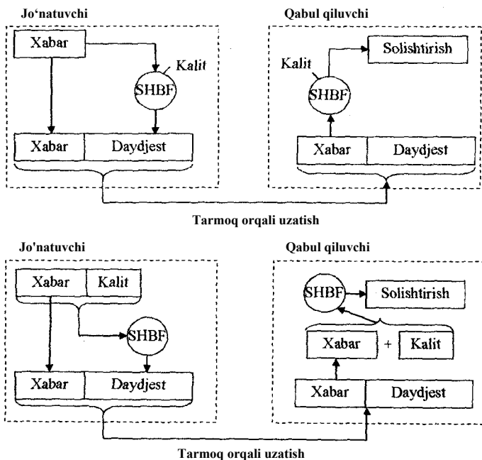
12.4-rasm. Shifrlashning bir tomonlama funktsiyalari.
