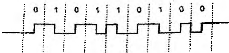
5.17-rasm. Manchester kodi.
