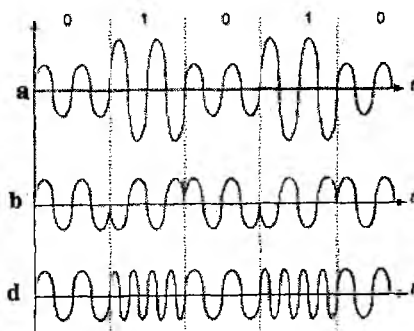
5.14-rasm. Signalning modulatsiya turlari. a- amplitudali; b- fazoliy; d- chastotali.
