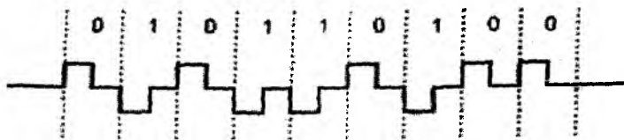
5.16-rasm. RZ raqamli kodlashtirish.
