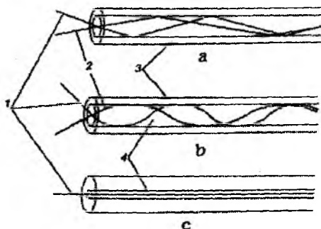
5.2-rasm. Optiktola kabeli xillari:
