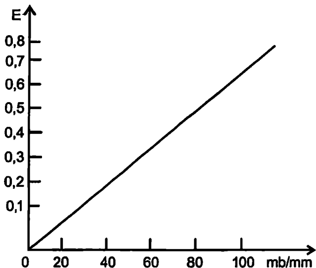
8-rasm. Kalibrlovchi grafik.
