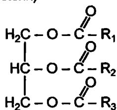
Triasilglitserin
