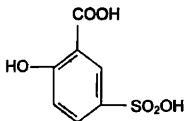
sulfosalitsil kislota
