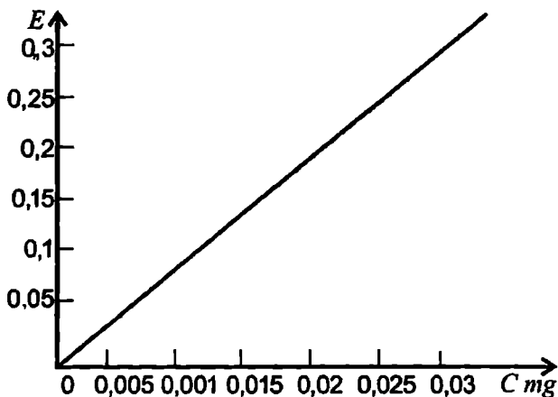
10-rasm. Kalibrlash grafi. Ordinata o'qida optik zichligi ( E ), absissa o'qida esa pirouzum kislotasi (mg da).
