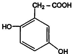
Gomogentizin kislotalari
