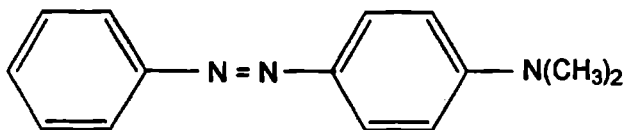
Paradimetilaminoazobenzol
